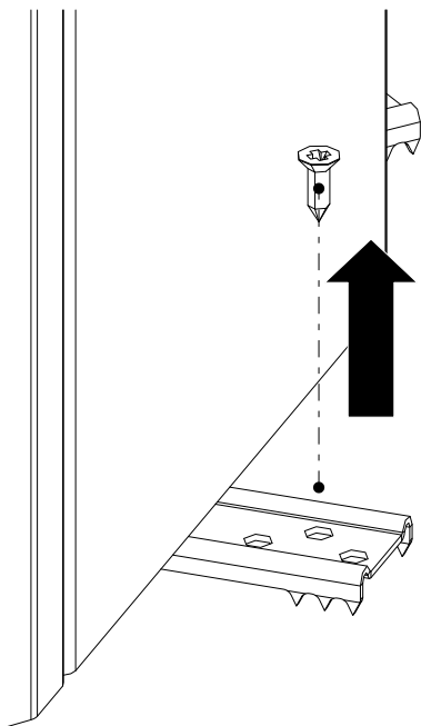
Fig. 7: Dévisser les vis de la plaque
