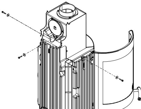
Fig. 49: Enlever les pierres HMS
