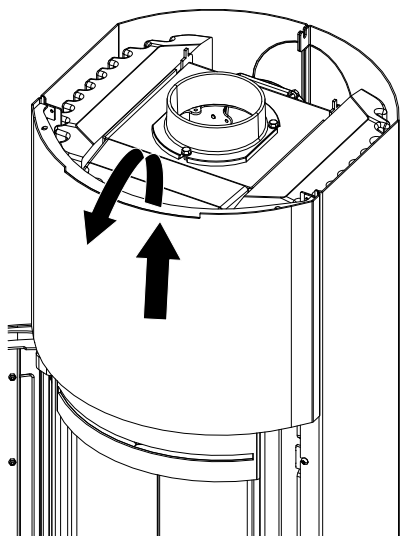
Fig. 13: Enlever le recouvrement supérieur
