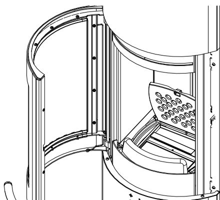
Fig. 44: Chiusura del coperchio
