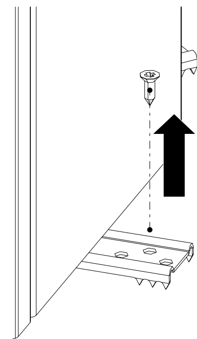
Fig. 7: Montaggio dei collegamenti a vite del pannello
