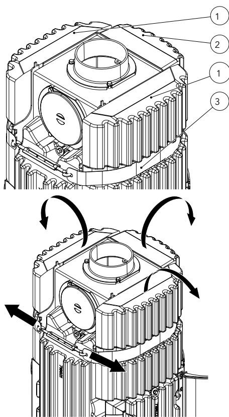
Fig. 48: Rimozione della cinghia di fissaggio e delle pietre HMS superiori
