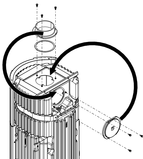
Fig. 23: Sostituzione del coperchio e del pezzo di collegamento
