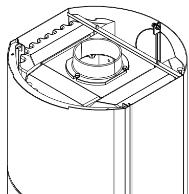
Fig. 29: Rimozione del coperchio
