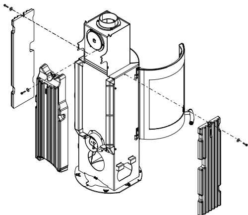
Fig. 26: Montaggio delle pietre HMS
