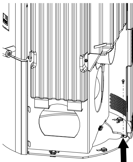
Fig. 18: Svitamento delle viti posteriori del rivestimento laterale
