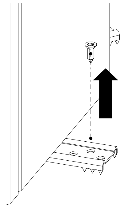
Fig. 7: Montaggio dei collegamenti a vite del pannello
