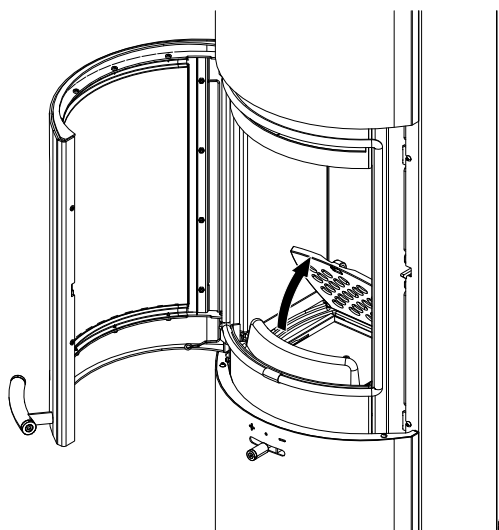
Fig. 42: Sollevamento della griglia
