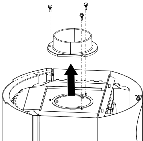
Fig. 32: Smontaggio della presa della canna fumaria
