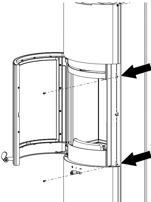
Fig. 16: Apertura della porta e allentamento delle viti all'interno
