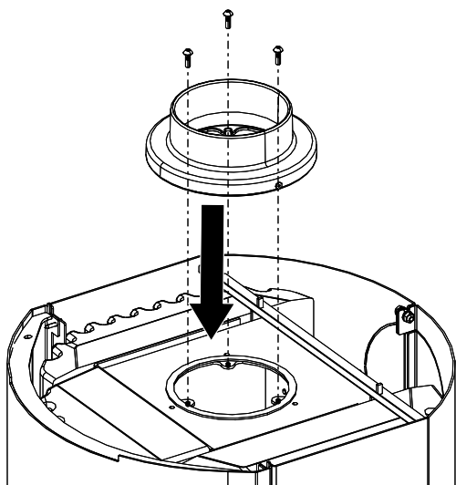
Fig. 34: Montaggio del giunto girevole
