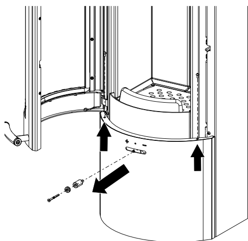
Fig. 14: Rimozione della copertura inferiore
