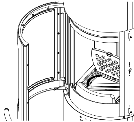
Fig. 43: Coperchio sul box cenere
