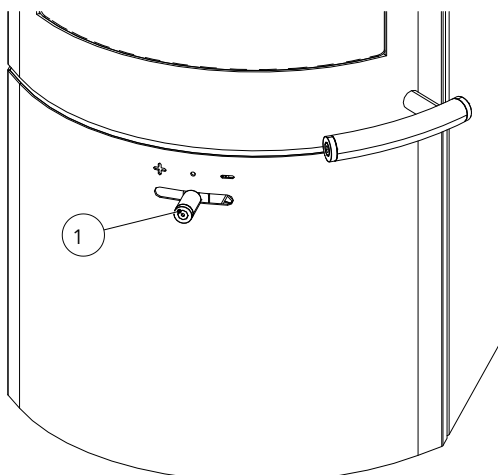
Fig. 38: Regolatore dell'aria primaria/secondaria
