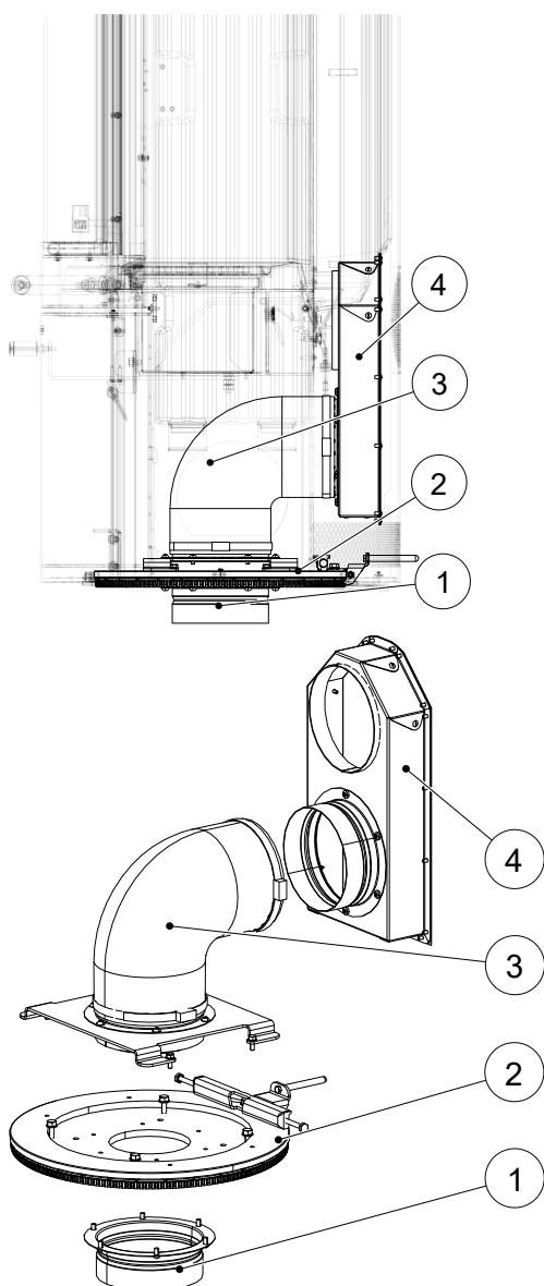
Fig. 36: Montaggio della connessione dell'aria esterna nella parte inferiore
