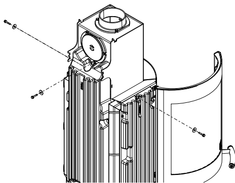
Fig. 49: Rimozione delle pietre HMS
