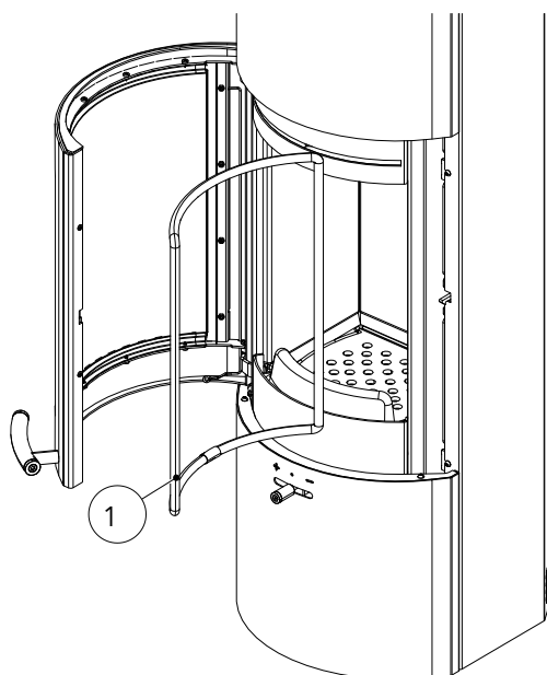
Fig. 41: Sostituzione della guarnizione
