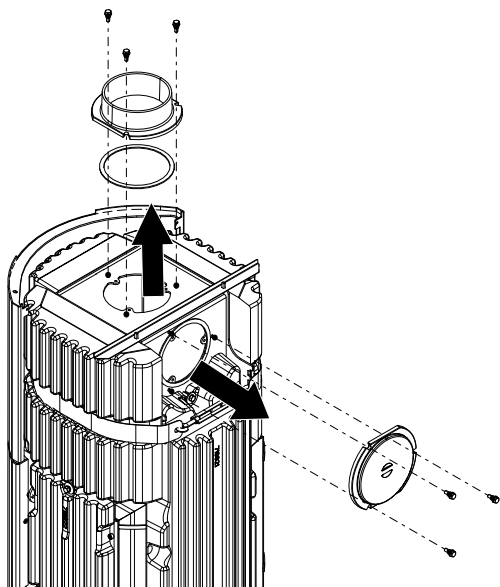
Fig. 22: Smontaggio del coperchio e della presa della canna fumaria
