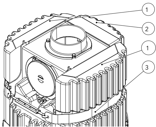
Fig. 27: Collocamento delle pietre superiori
