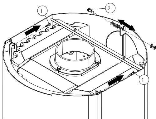
Fig. 12: Svitamento delle viti
