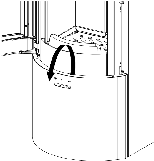
Fig. 15: Rimozione della copertura inferiore
