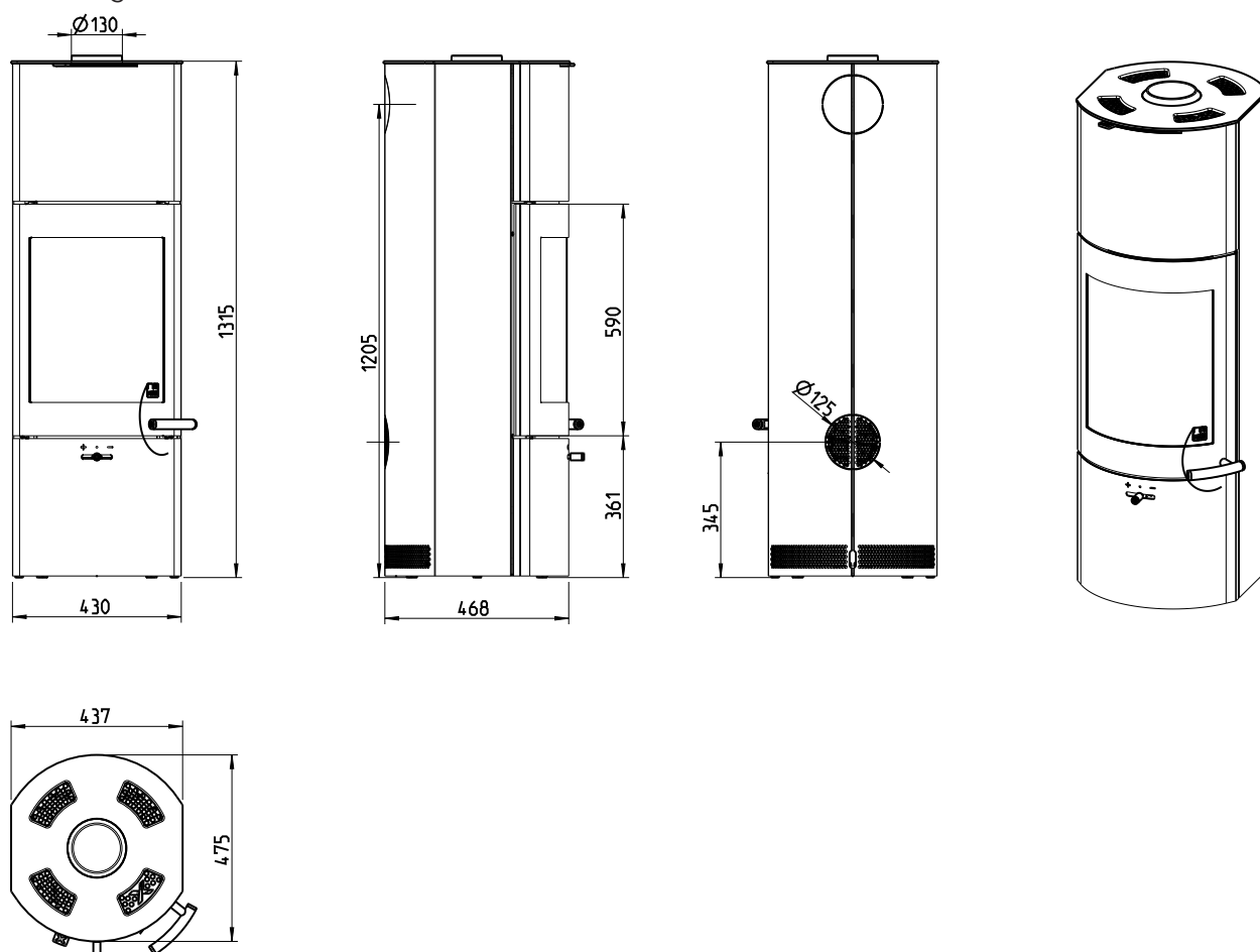
Fig. 1: Dimensioni dell'apparecchio di base
