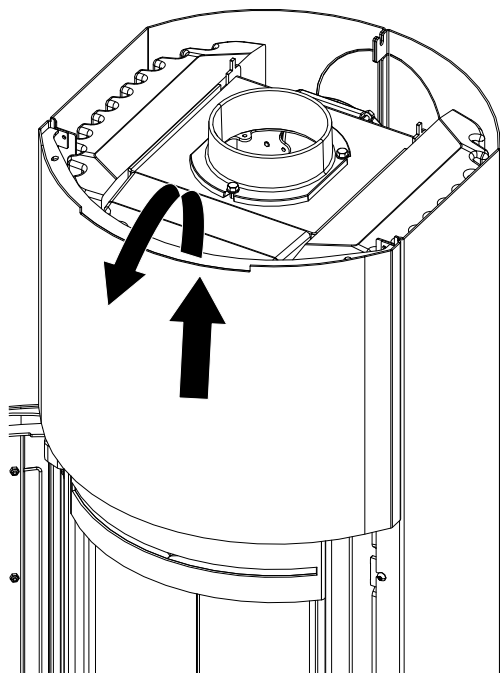
Fig. 13: Rimozione della copertura superiore
