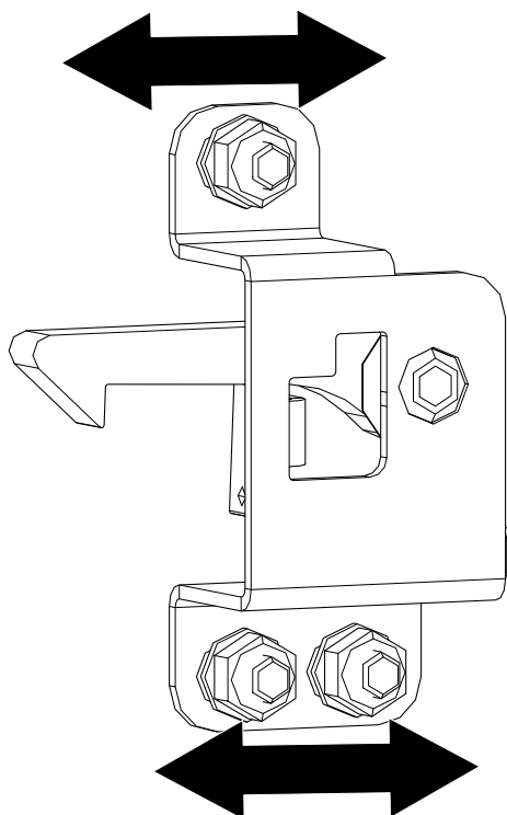
Fig. 37: Regolazione della serratura dello sportello
