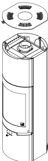
Fig. 11: Rimozione del coperchio
