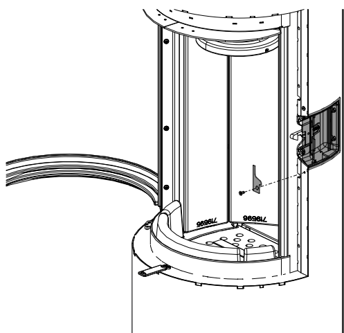
Fig. 40: Rimontaggio della maniglia
