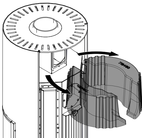
Fig. 53: Smontaggio delle pietre HMS in alto
