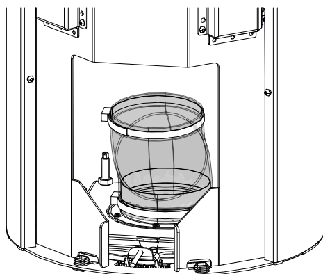
Fig. 26: Fissaggio del tubo
