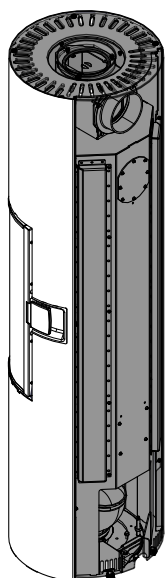
Fig. 13: Rimontaggio della parete posteriore e del coperchio
