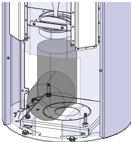
Fig. 15: Fissare il tubo flessibile in alluminio.
