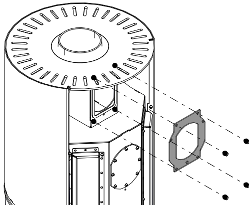
Fig. 29: Smontaggio della guarnizione posteriore
