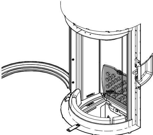
Fig. 47: Sollevamento della griglia
