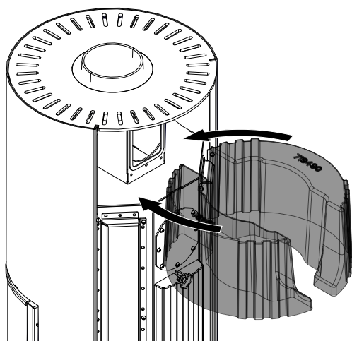
Fig. 32: Montaggio delle pietre HMS in alto
