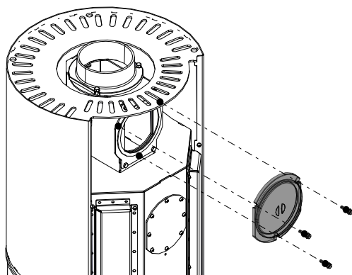
Fig. 28: Smontaggio della copertura posteriore
