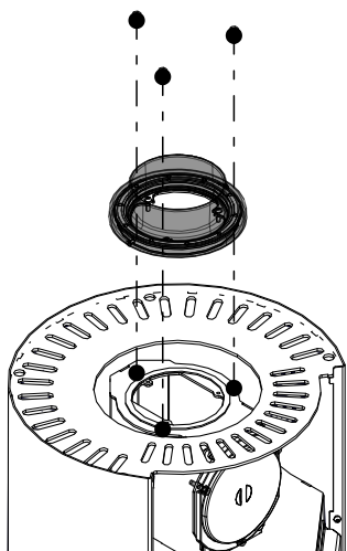
Fig. 19: Montaggio della presa della canna fumaria rotante
