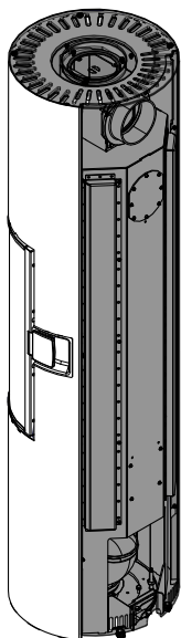
Fig. 55: Rimontaggio della parete posteriore e del coperchio.
