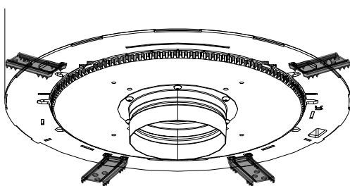
Fig. 7: Rimozione dei fermi di trasporto
