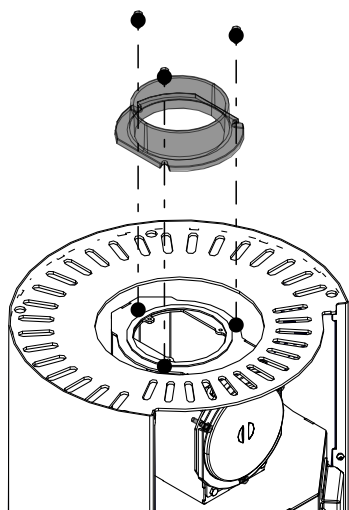
Fig. 22: Smontaggio della presa della canna fumaria
