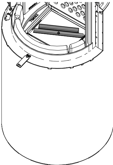
Fig. 48: Coperchio sul box cenere
