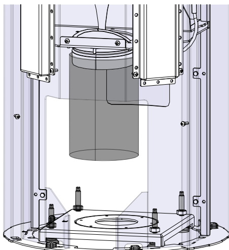
Fig. 16: Fissare il tubo flessibile in alluminio.
