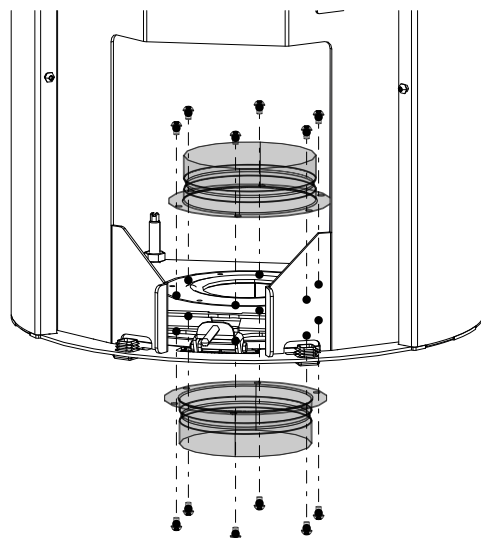
Fig. 25: Montaggio di entrambi i supporti
