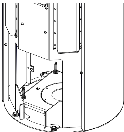
Fig. 34: Allineamento della stufa
