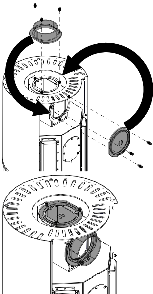
Fig. 11: Sostituzione della presa della canna fumaria e della copertura
