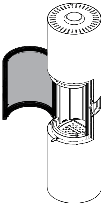
Fig. 37: Apertura dello sportello
