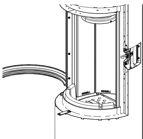
Fig. 39: Regolazione della serratura dello sportello
