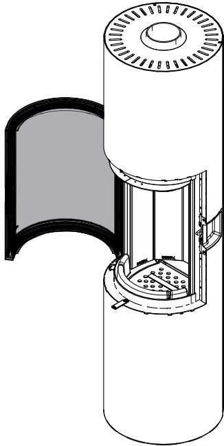
Fig. 41: Apertura dello sportello
