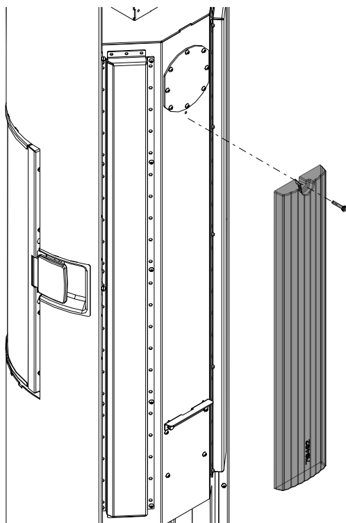
Fig. 54: Smontaggio della pietra HMS
