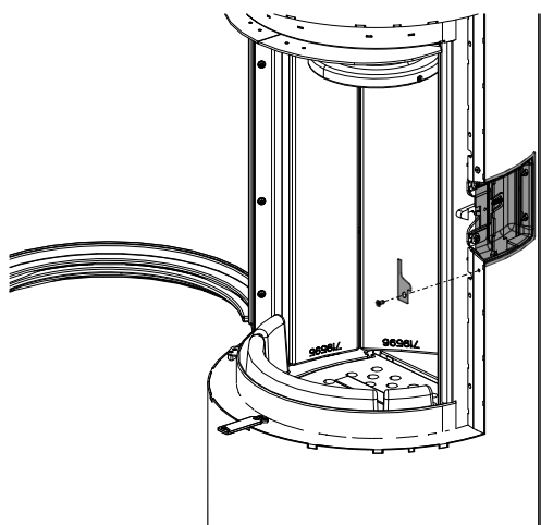
Fig. 38: Smontaggio della maniglia dello sportello
