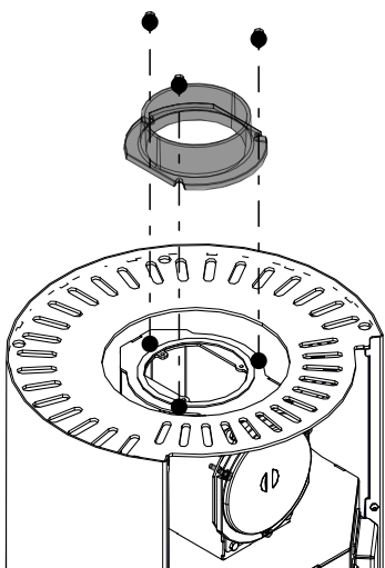
Fig. 18: Smontaggio della presa della canna fumaria
