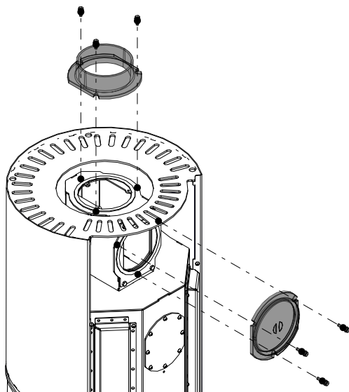
Fig. 10: Rimozione dei pezzi
