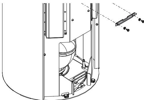
Fig. 30: Montaggio dei supporti dell'HMS
