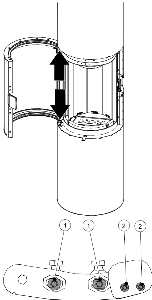
Fig. 36: Viti di registro dello sportello
