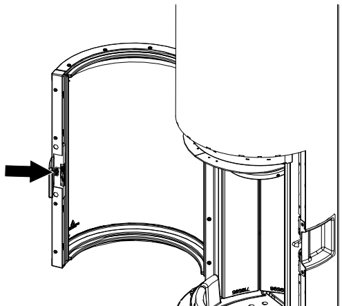
Fig. 42: Regolazione della forza di chiusura dello sportello
