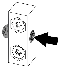
Fig. 43: Regolazione della forza di chiusura dello sportello
