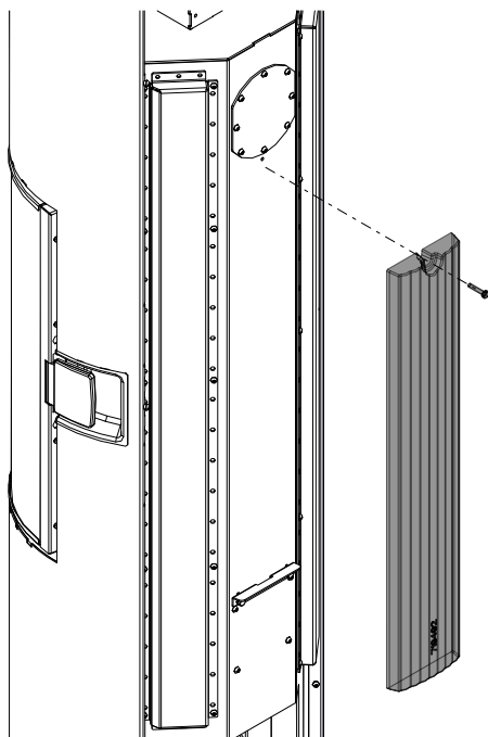
Fig. 31: Montaggio della pietra HMS
