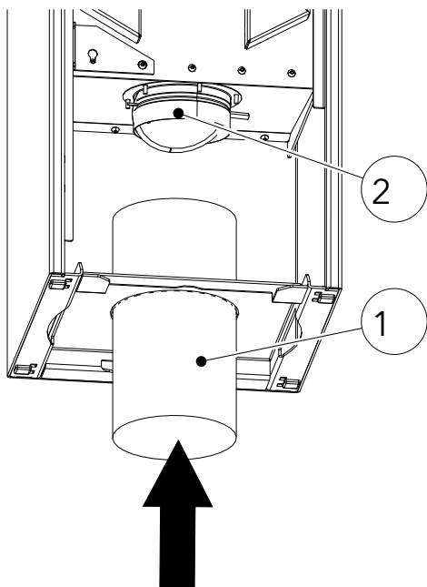
Fig. 18: Attraversamento del tubo
