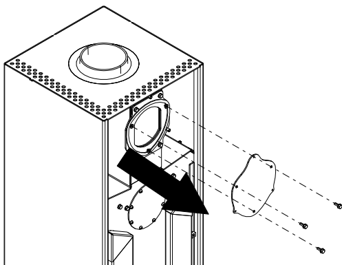
Fig. 10: Smontaggio della copertura del tubo dei fumi posteriore
