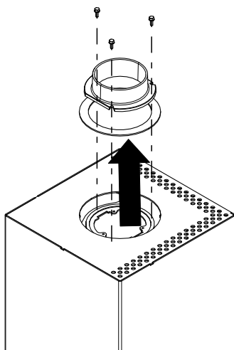
Fig. 31: Smontaggio della presa della canna fumaria.
