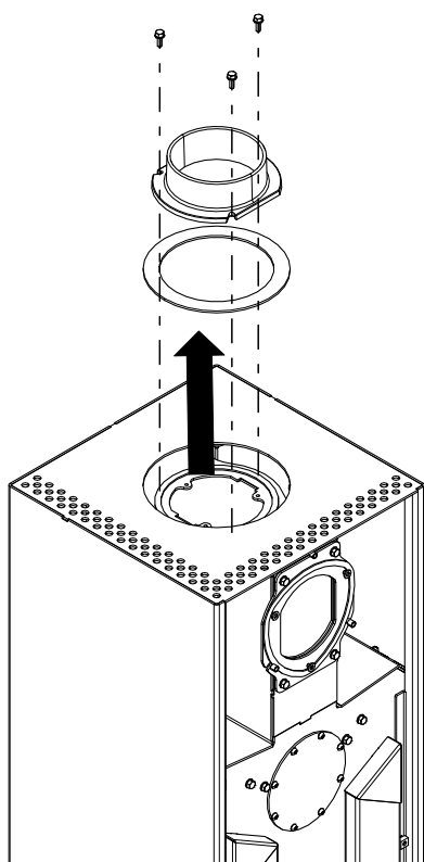
Fig. 11: Smontaggio dell'elemento di collegamento con la guarnizione
