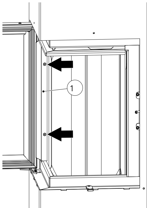
Fig. 50: Apertura dello sportello e svitamento delle viti
