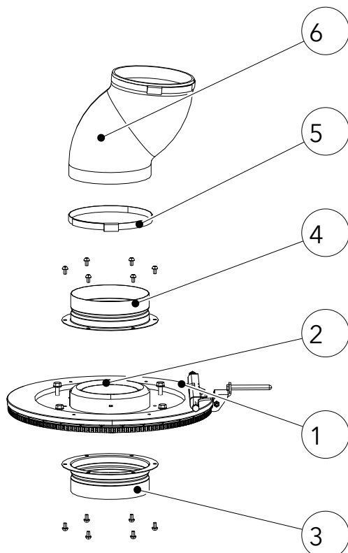
Fig. 35: Piatto girevole con raccordi
