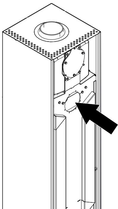
Fig. 45: Aspirare i passaggi dei gas di combustione
