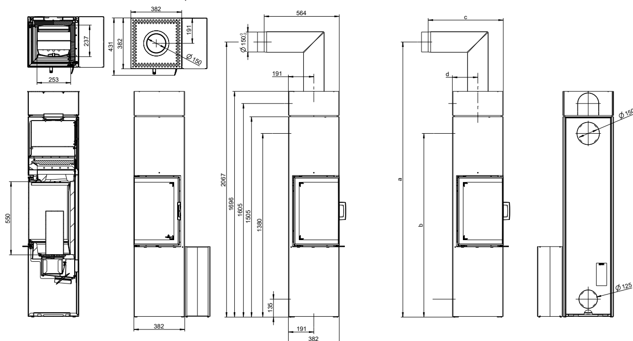
Fig. 1: Dimensioni Slim 4.0
