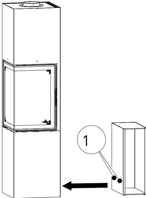
Fig. 25: Montaggio del box laterale
