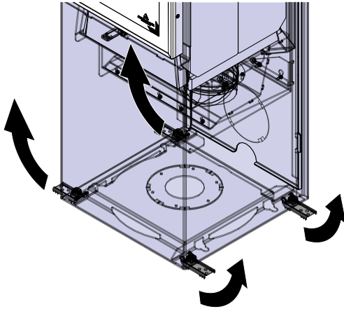
Fig. 6: Rimozione dei fermi di trasporto
