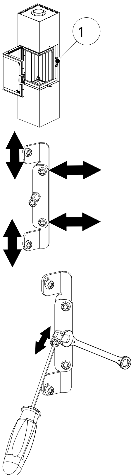
Fig. 37: Regolazione della chiusura
