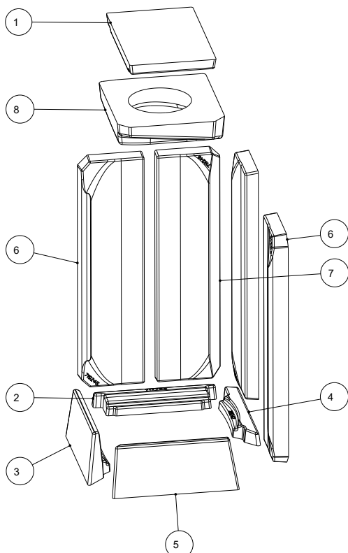
Fig. 19: Montaggio del Keramott - sinistra
