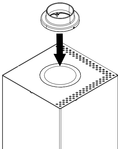
Fig. 33: Montaggio del giunto girevole
