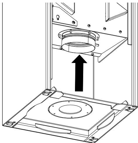
Fig. 15: Montaggio dell'attacco dell'aria esterna posteriore
