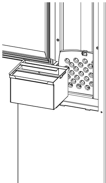
Fig. 49: Rimozione e svuotamento del box cenere
