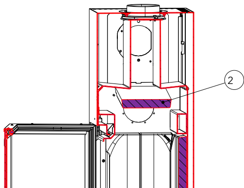
Fig. 58: Estrazione della deviazione in Keramott
