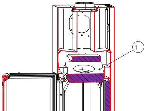
Fig. 57: Rimozione del tagliafiamma in Keramott
