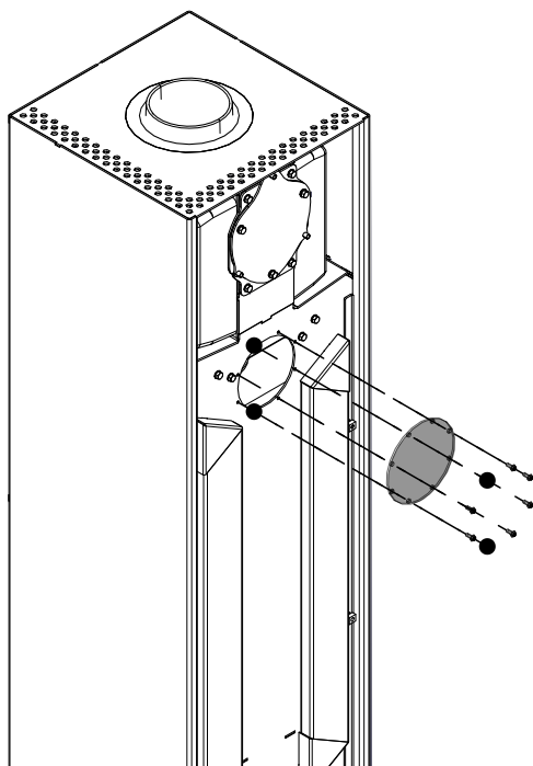
Fig. 44: Rimuovere il coperchio di ispezione
