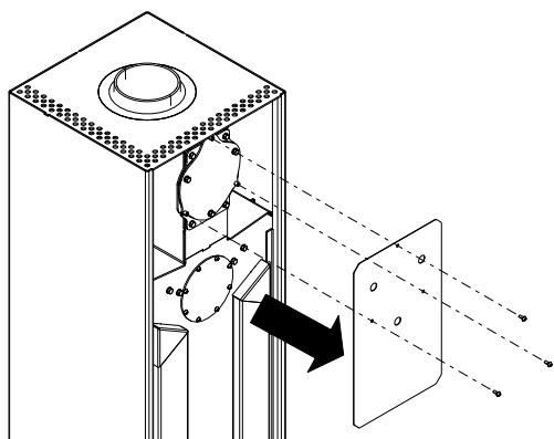
Fig. 21: Smontaggio del pannello di protezione dal calore
