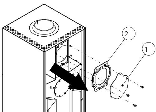
Fig. 22: Smontaggio della copertura del tubo dei fumi posteriore
