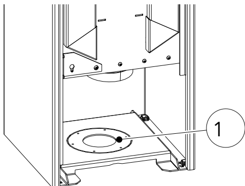
Fig. 17: Rimozione della parte perforata
