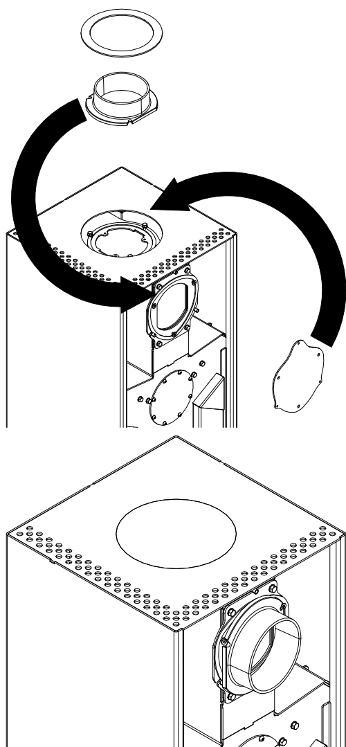
Fig. 12: Sostituzione della copertura e del pezzo di collegamento
