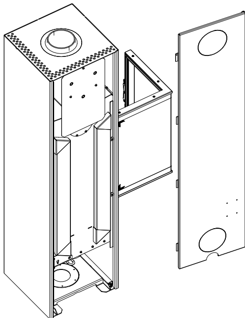
Fig. 53: Smontaggio della parete posteriore
