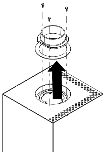
Fig. 26: Smontaggio della presa della canna fumaria.
