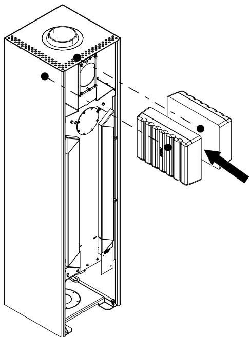
Fig. 23: Inserimento delle pietre HMS
