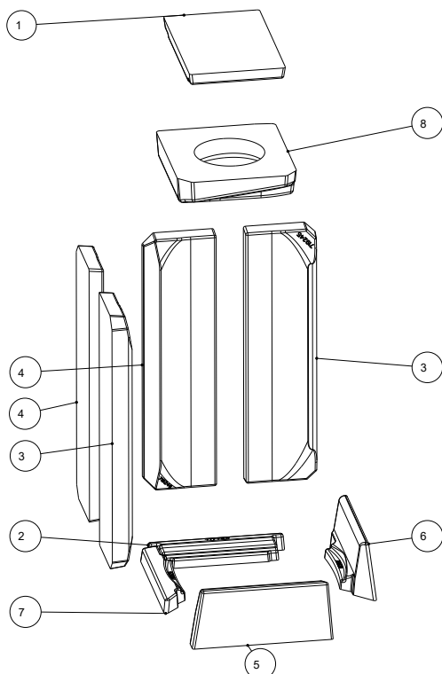
Fig. 20: Montaggio del Keramott - destra
