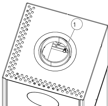
Fig. 7: Rimozione della sicurezza per il trasporto
