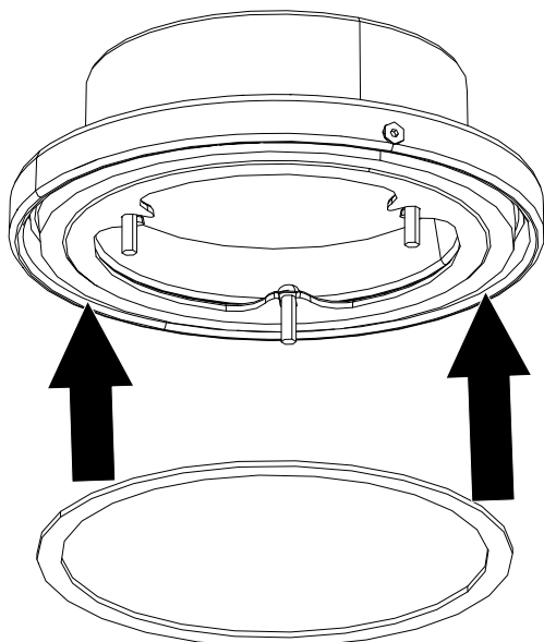
Fig. 27: Montaggio della guarnizione sul giunto girevole
