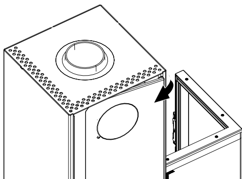
Fig. 52: Apertura della parete posteriore
