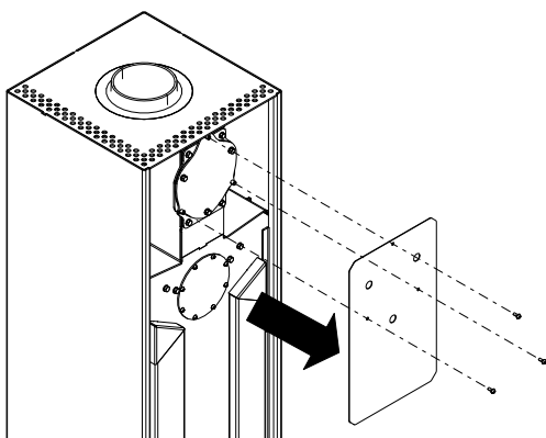
Fig. 9: Smontaggio del pannello di protezione dal calore
