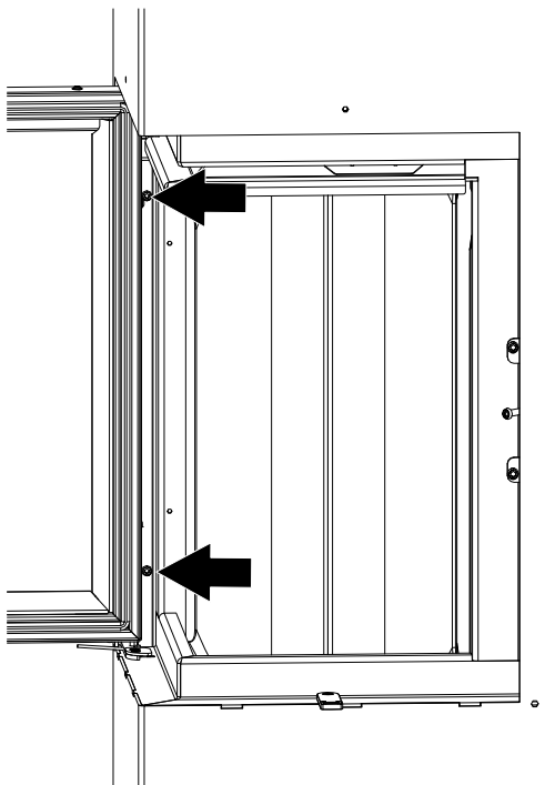
Abb. 53: Schrauben von der Rückwand lösen
