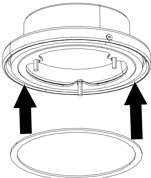
Abb. 34: Dichtung am Drehstutzen anbringen
