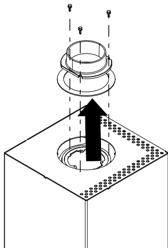
Abb. 28: Rauchrohrstutzen demontieren
