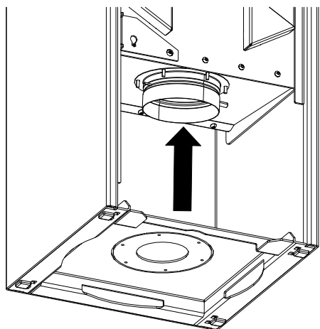
Abb. 17: Externen Luftanschluss hinten montieren
