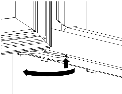
Abb. 57: Feder lösen
