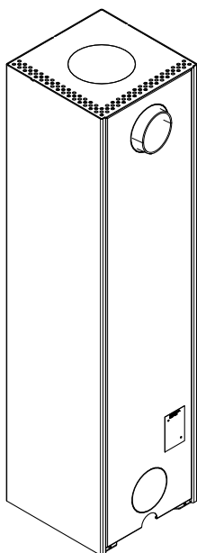
Abb. 15: Rückwand montieren
