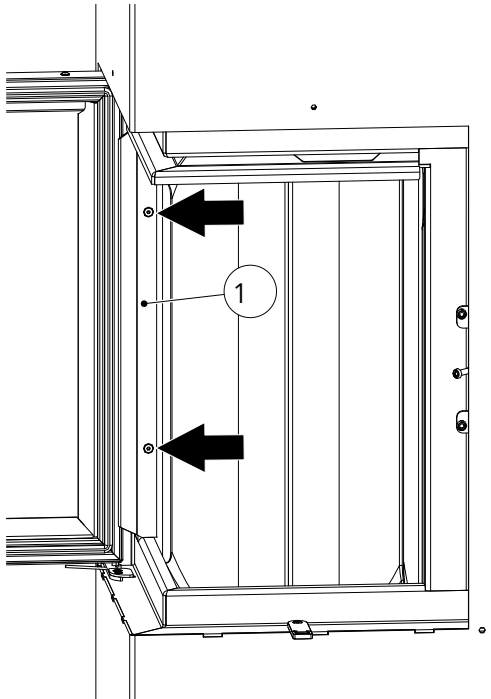
Abb. 52: Tür öffnen und Schrauben lösen
