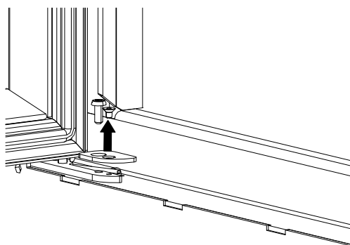
Abb. 56: Feuerraumtür öffnen und Schrauben lösen
