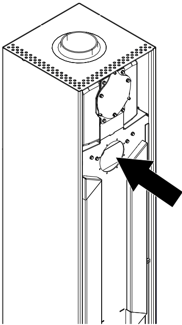
Abb. 47: Rauchgaswege saugen
