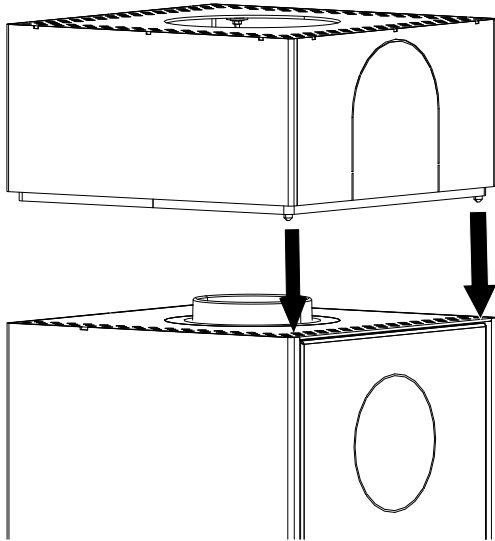
Abb. 26: Aufsatzbox anbringen
