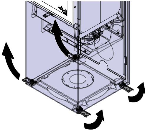
Abb. 8: Transportsicherung entfernen
