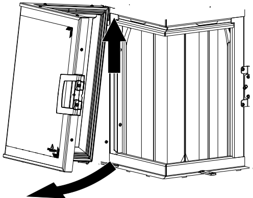
Abb. 58: Feuerraumtür aushängen
