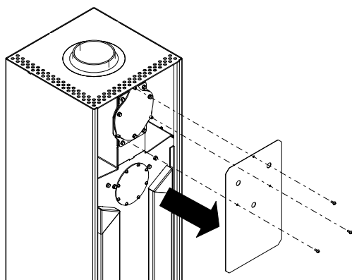
Abb. 23: Hitzeschutz demontieren
