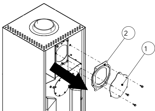
Abb. 24: Hintere Rauchrohrabdeckung demontieren
