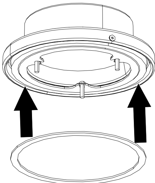
Abb. 29: Dichtung am Drehstutzen anbringen
