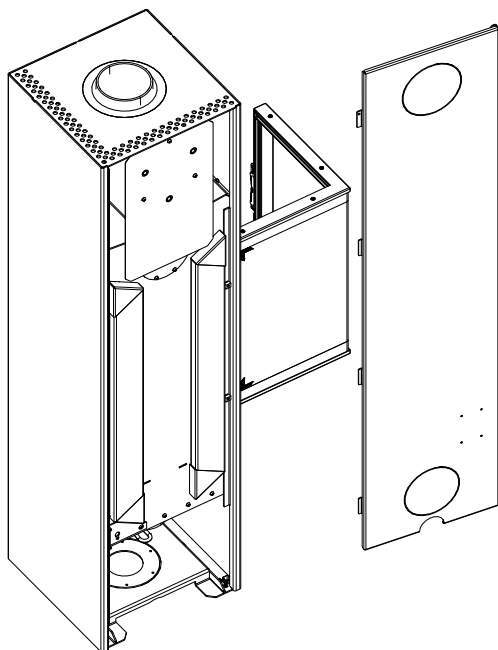
Abb. 55: Rückwand demontieren
