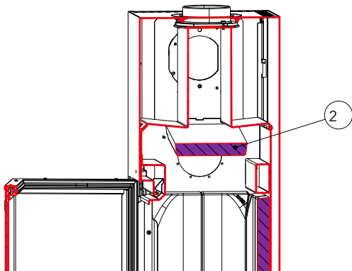
Abb. 60: Keramottumlenkung herausnehmen
