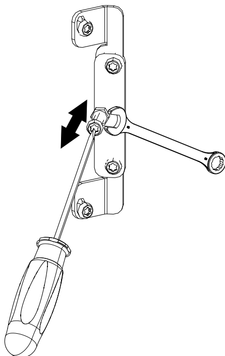
Abb. 39: Verschluss einstellen
