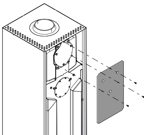
Abb. 45: Schrauben lösen
