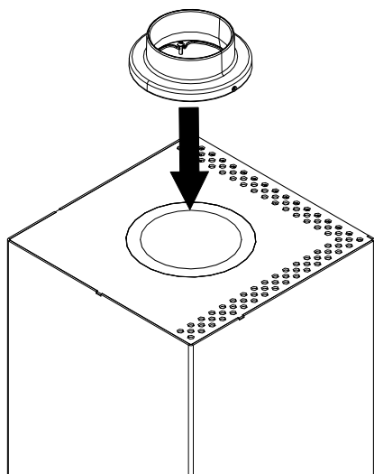
Abb. 30: Drehstutzen montieren
