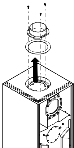
Abb. 13: Stützen mit Dichtung demontieren
