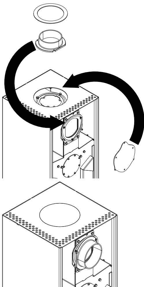
Abb. 14: Abdeckung und Stützen tausche
