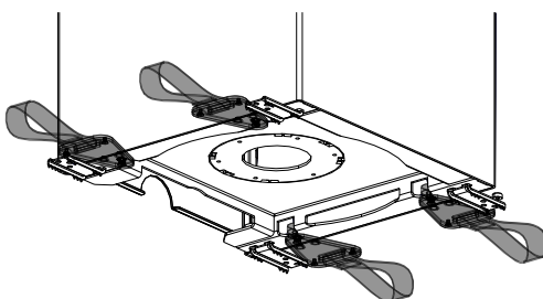
Abb. 7: Transporthilfe
