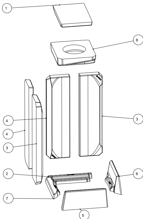
Abb. 22: Keramott einbauen - rechts
