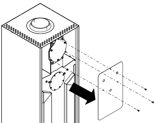
Abb. 11: Hitzeschutz demontieren
