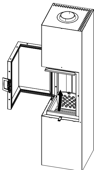
Abb. 48: Rost hochklappen
