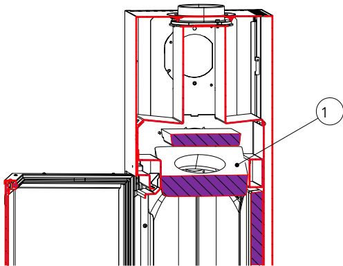
Abb. 59: Keramottzugplatte herausnehmen
