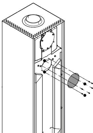
Abb. 46: Revisionsdeckel abnehmen
