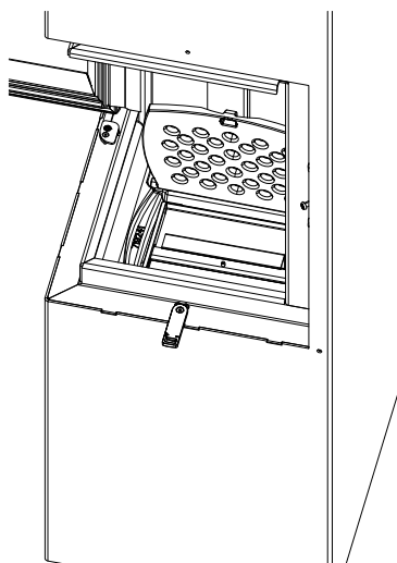
Abb. 50: Deckel zumachen
