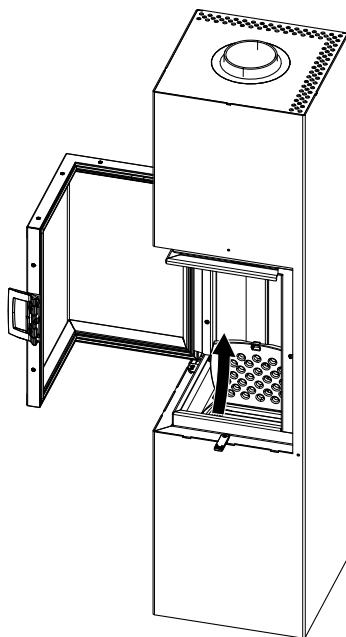
Fig. 49: Relever la grille
