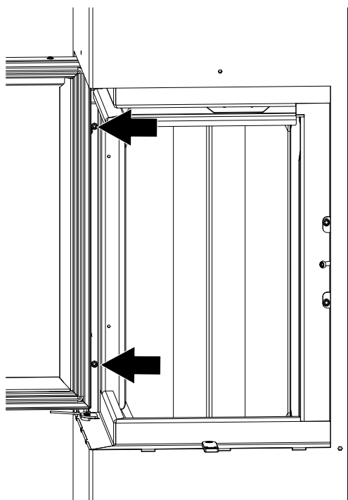
Fig. 54: Dévisser les vis de la paroi arrière
