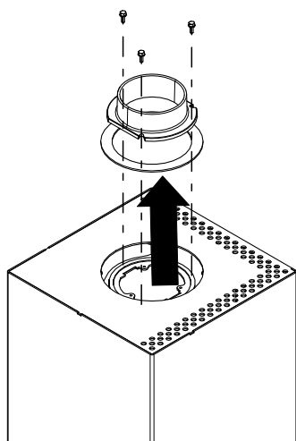
Fig. 31: Démontez la tubulure de fumées
