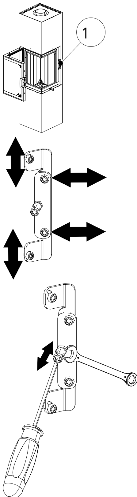
Fig. 36: Régler la serrure
