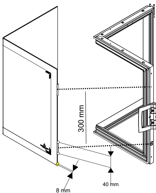
Fig. 47: Installer la vitre de la porte
