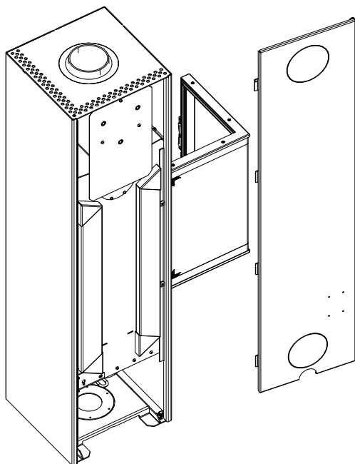
Fig. 56: Déposer la paroi arrière
