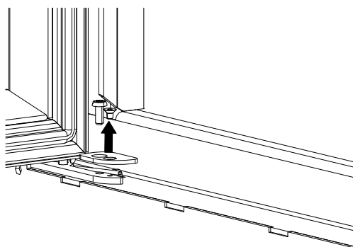
Fig. 57: Ouvrir la porte du foyer et dévisser les vis
