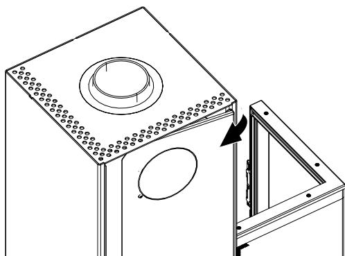
Fig. 55: Ouvrir la paroi arrière
