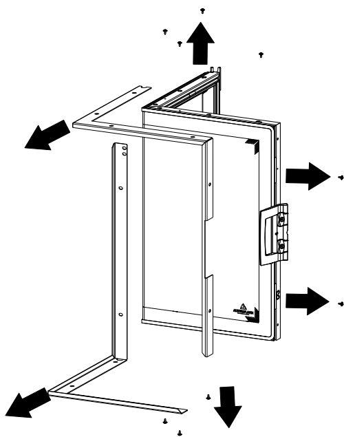
Fig. 45: Déposer les vis et les parcloles
