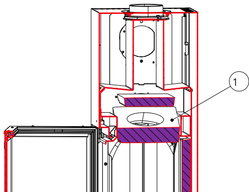
Fig. 60: Extraire la plaque de tirage en Keramott
