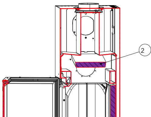
Fig. 61: Extraire le déflecteur en Keramott
