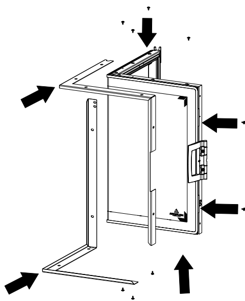
Fig. 48: Remettre les parcloles en place
