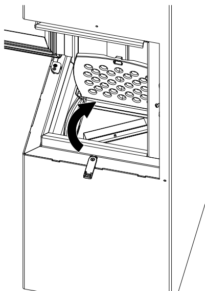
Fig. 50: Mettre le couvercle sur le bac à cendres
