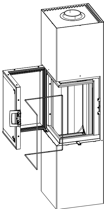
Fig. 44: Remplacer le joint
