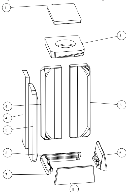
Fig. 21: Installation de la Keramott - droite
