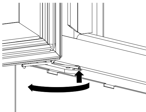
Fig. 58: Libérer le ressort
