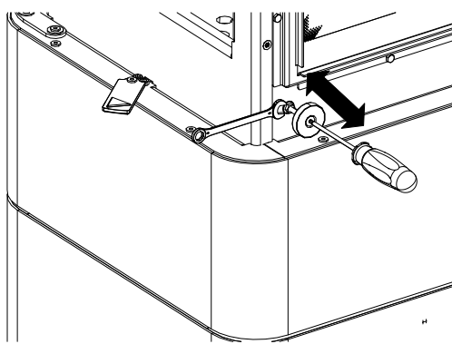
Fig. 38: Pos. 2 Régler la porte
