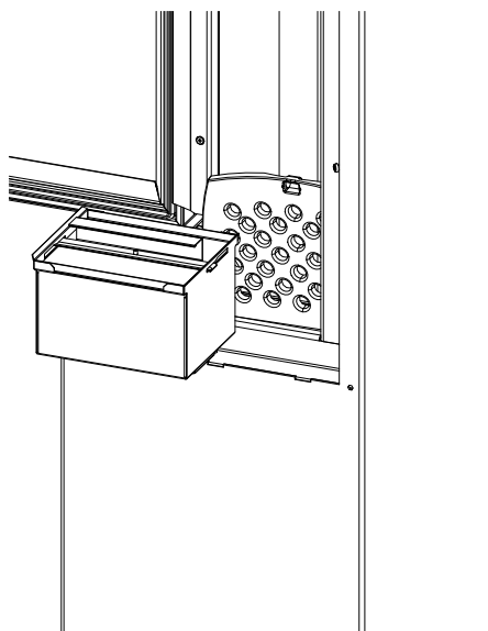
Fig. 52: Enlever et vider le bac à cendres
