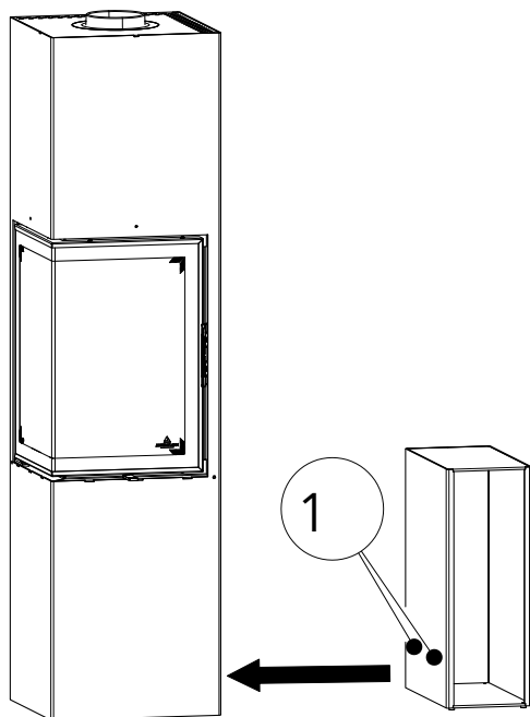
Fig. 26: Installer le module latéral
