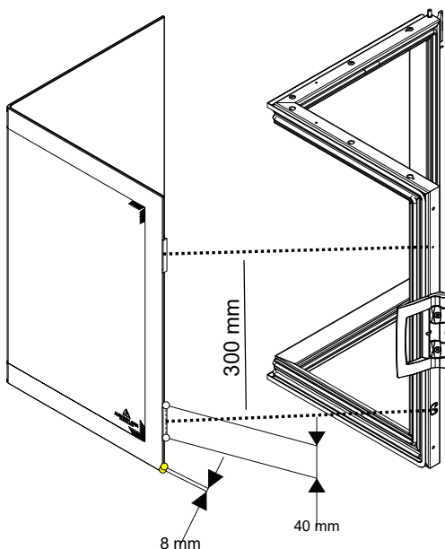
Fig. 44: Installer la vitre de la porte
