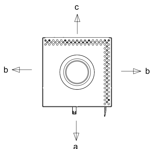
Fig. 8: Distances de sécurité (vue de dessus) en angle
