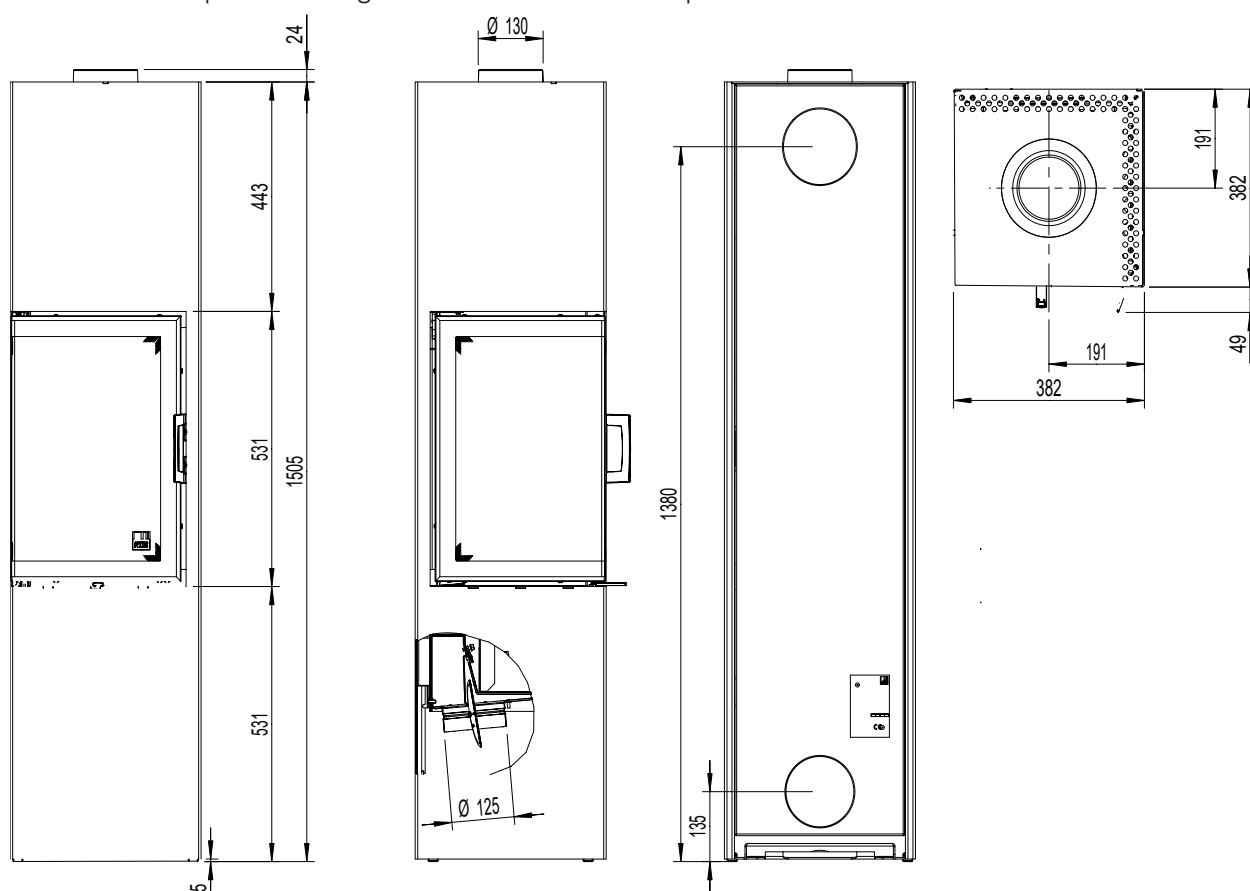
Fig. 1: Dimensions pour Slim gauche
