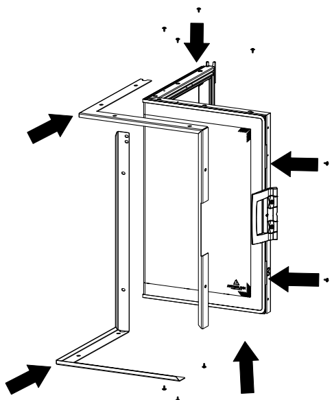
Fig. 45: Remettre les parcloles en place
