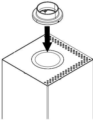
Fig. 33: Installer la tubulure tournante
