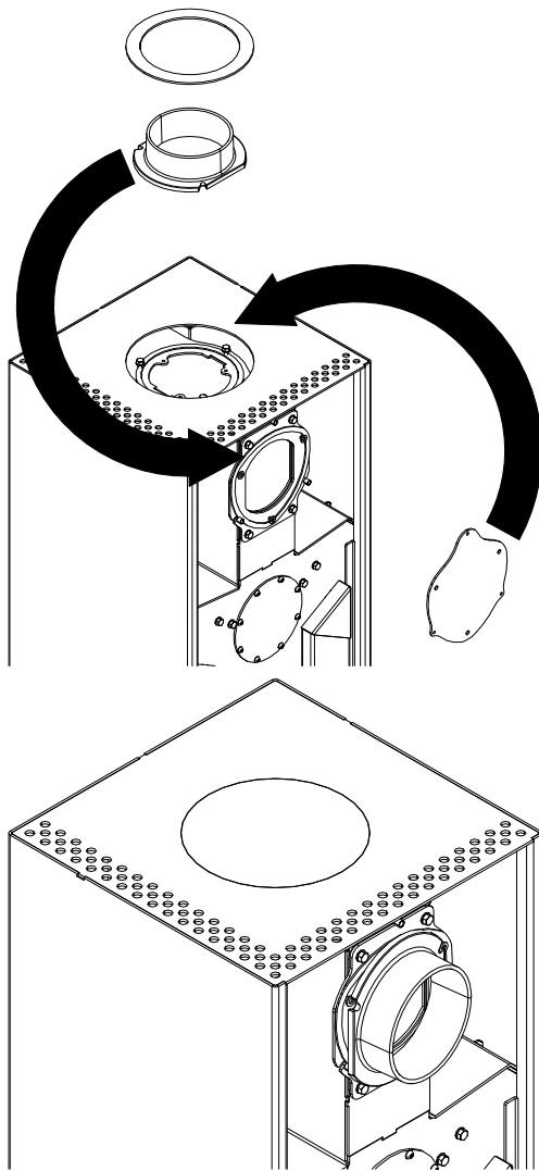
Fig. 13: Interchanger le recouvrement et la tubulure
