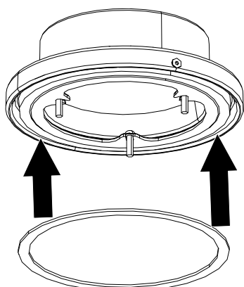
Fig. 32: Poser le joint sur la tubulure tournante
