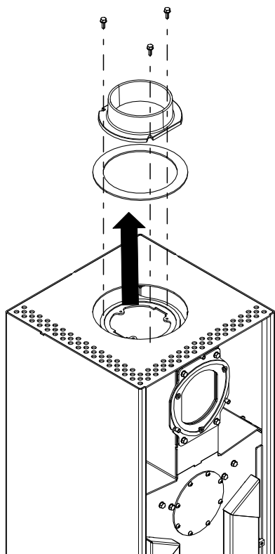
Fig. 12: Démontez la tubulure avec le joint
