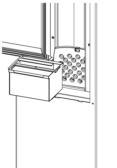
Fig. 49: Enlever et vider le bac à cendres
