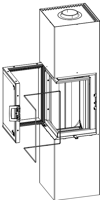
Fig. 41: Remplacer le joint
