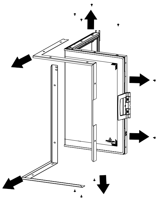
Fig. 42: Déposer les vis et les parcloles
