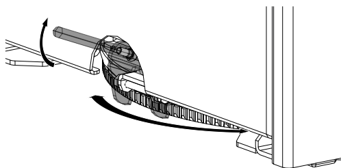
Fig. 42: Drehteller einstellen
