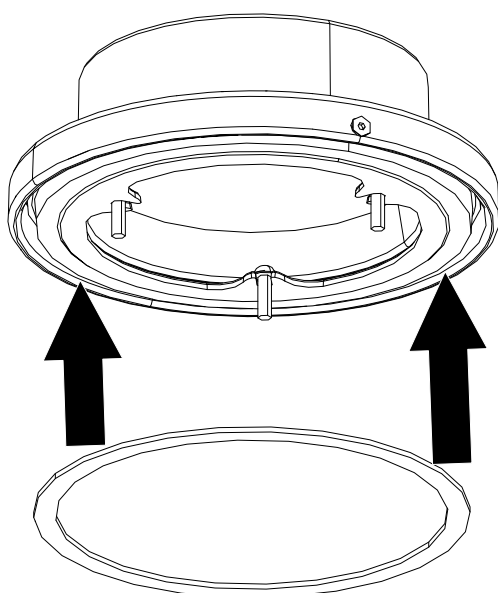
Fig. 30: Poser le joint sur la tubulure tournante
