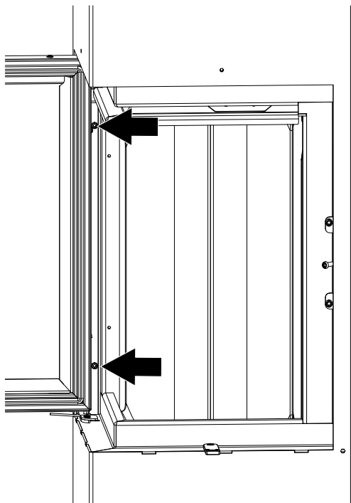
Fig. 56: Dévisser les vis de la paroi arrière
