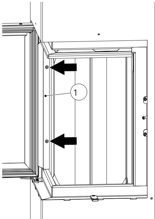
Fig. 55: Ouvrir la porte et dévisser les vis.
