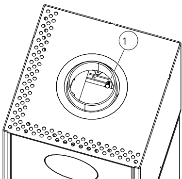
Fig. 9: Enlever la sécurité de transport
