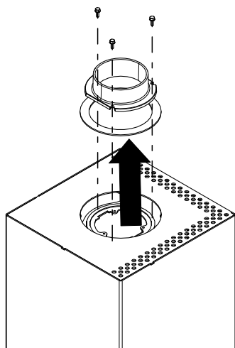
Fig. 34: Démonter la tubulure de fumées
