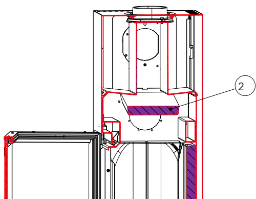
Fig. 63: Extraire le déflecteur en Keramott
