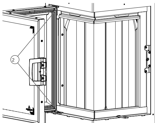
Fig. 41: Pos. 1 Régler la porte
