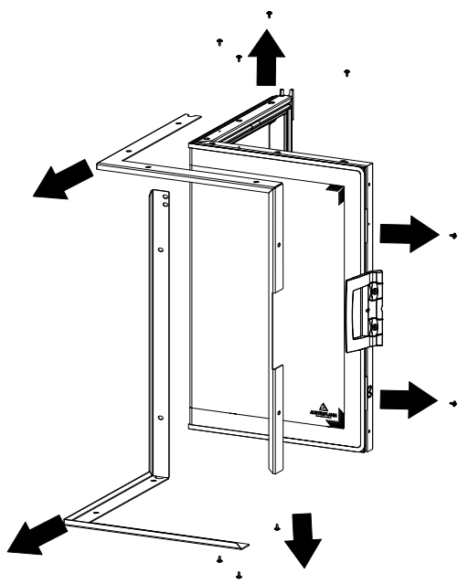
Fig. 47: Déposer les vis et les parcloles
