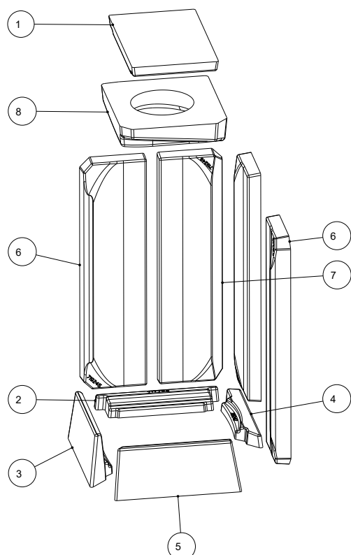
Fig. 22: Installation de la Keramott - gauche
