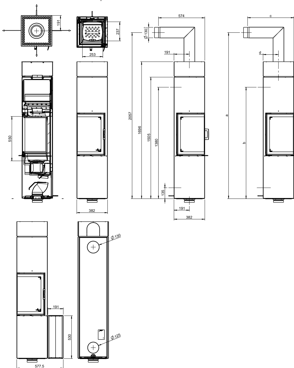
Fig. 1: Dimensioni Slim 2.0
