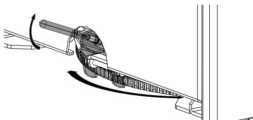
Fig. 40: Regolazione del piatto girevole
