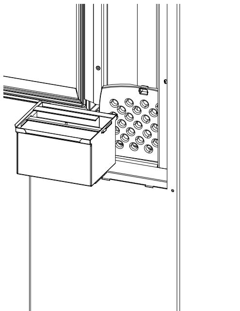
Fig. 52: Rimozione e svuotamento del box cenere
