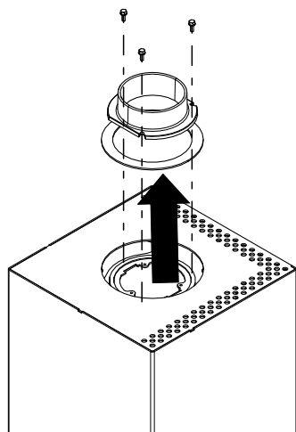
Fig. 27: Smontaggio della presa della canna fumaria.
