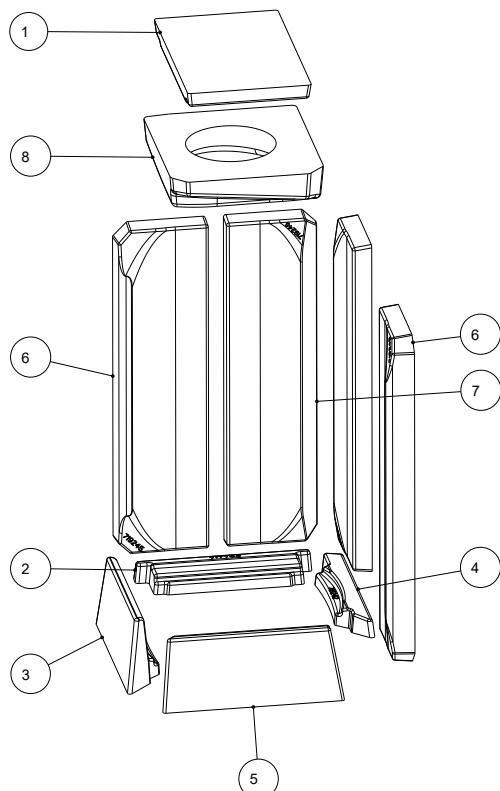
Fig. 20: Montaggio del Keramott - sinistra
