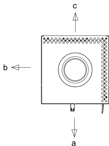
Fig. 8: Distanze di sicurezza (vista dall'alto ad angolo)
