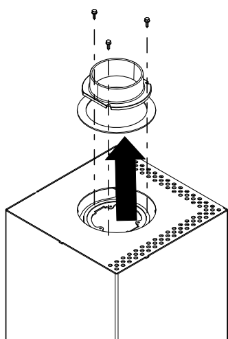
Fig. 32: Smontaggio della presa della canna fumaria.
