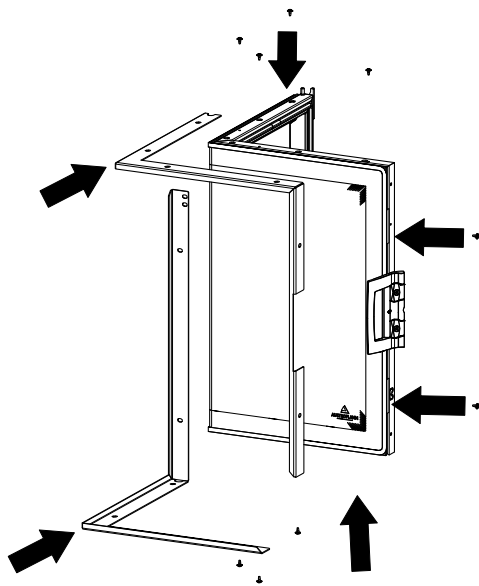
Fig. 48: Rimontaggio dei fermavetri
