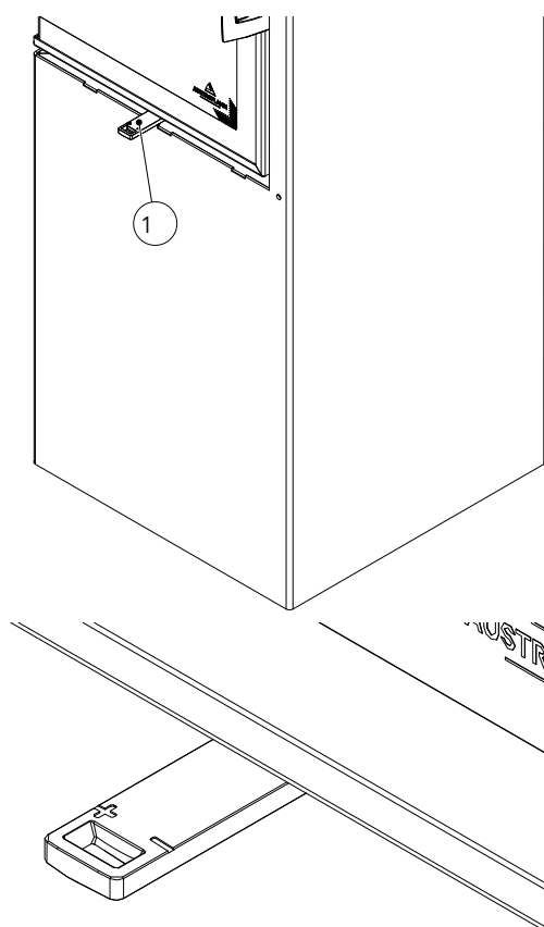
Fig. 2: Regolatore dell'aria
