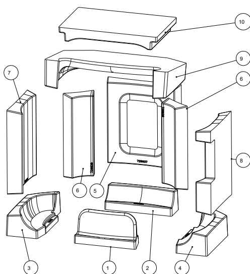
Fig. 36: Ordre d'installation de la Keramott
