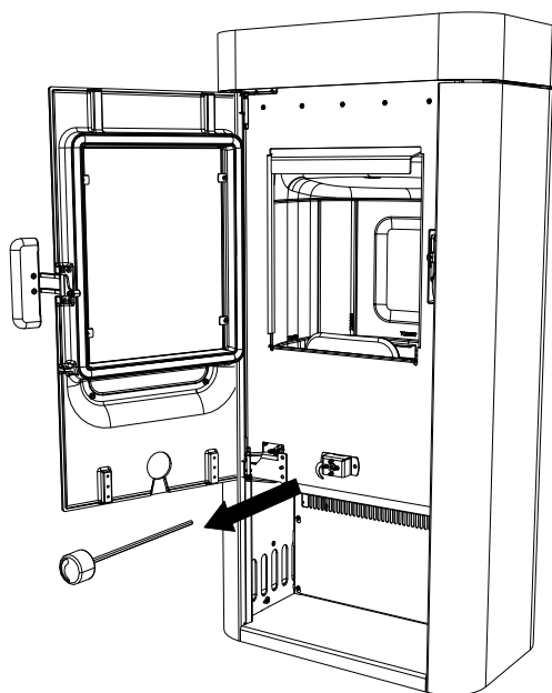
Fig. 19: Déposer la molette
