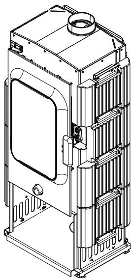
Fig. 28: Pierres de droite en place
