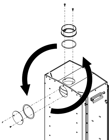
Fig. 10: Échanger le recouvrement et la tubulure
