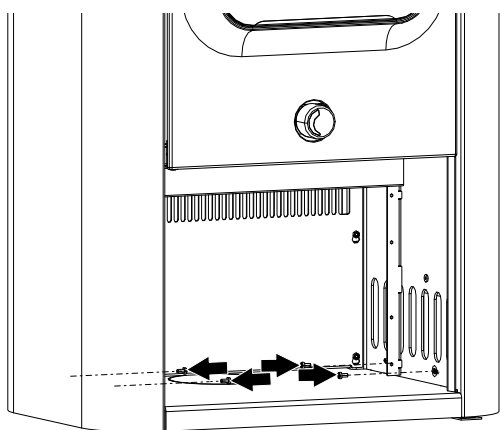
Fig. 6: Fixer l'habillage latéral en bas à l'intérieur
