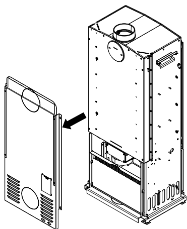
Fig. 8: Déposer le panneau arrière
