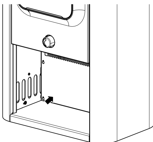
Fig. 35: Fixer l'obturateur de socle sur les fixations
