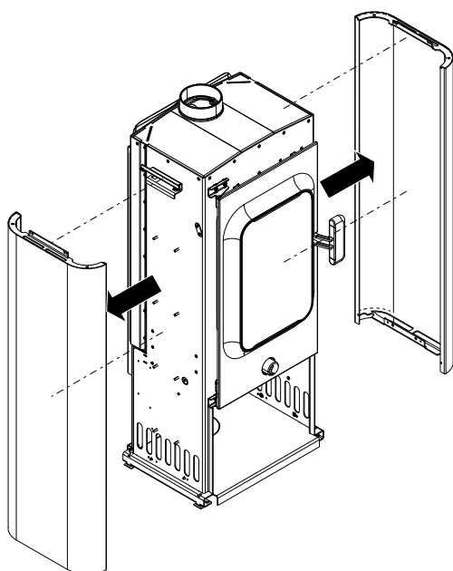
Fig. 52: Enlever l'habillage latéral
