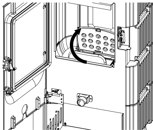
Fig. 44: Relever la grille
