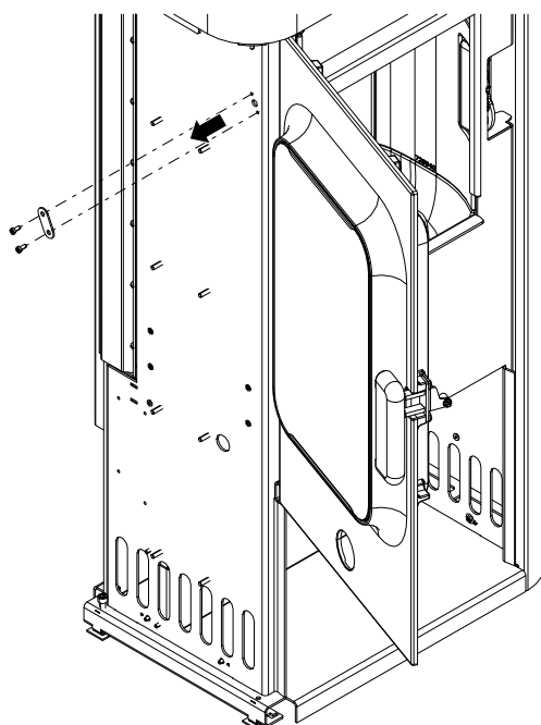
Fig. 20: Enlever la plaque de recouvrement
