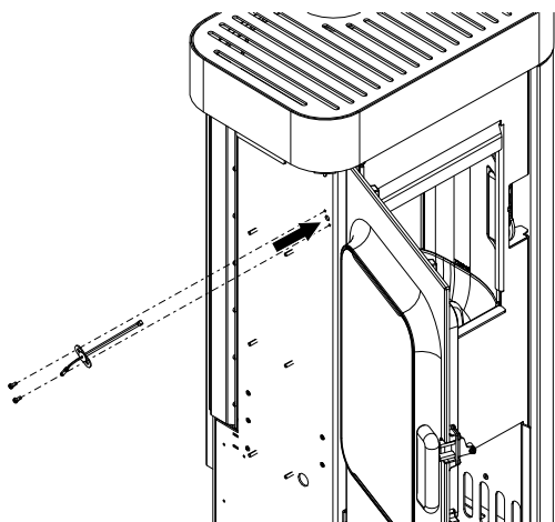
Fig. 22: Fixer le capteur de température de la chambre de combustion
