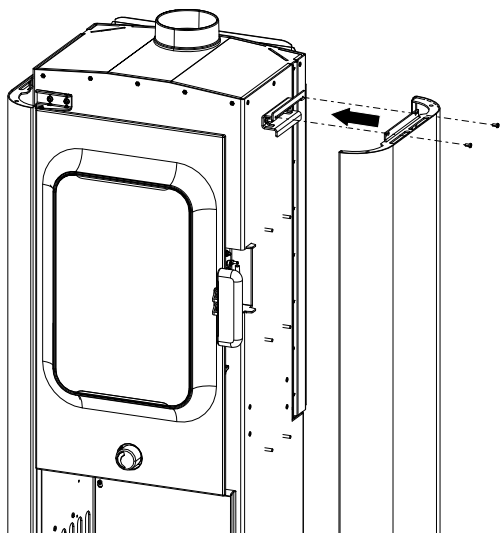
Fig. 5: Fixer l'habillage latéral à la fixation
