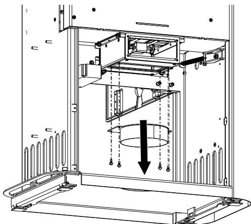
Fig. 16: Démontez le collet d'arrivée d'air en bas
