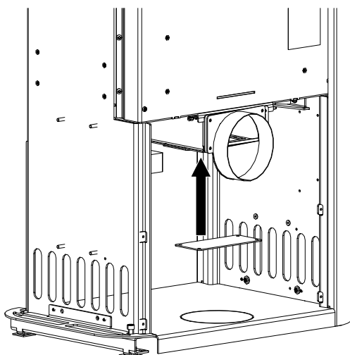
Fig. 18: Raccordement à l'air externe à l'arrière
