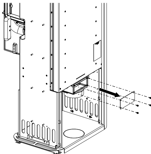
Fig. 15: Démontez le couvercle arrière
