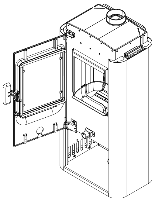
Fig. 39: Ouvrir la porte
