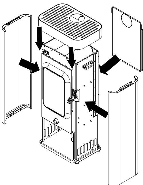
Fig. 12: Installer l'habillage latéral, le panneau arrière et le couvercle
