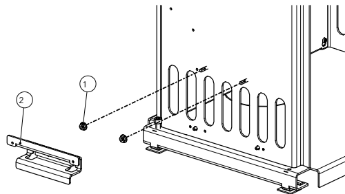
Fig. 25: Installer la fixation
