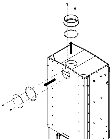
Fig. 9: Démonter le recouvrement et la tubulure
