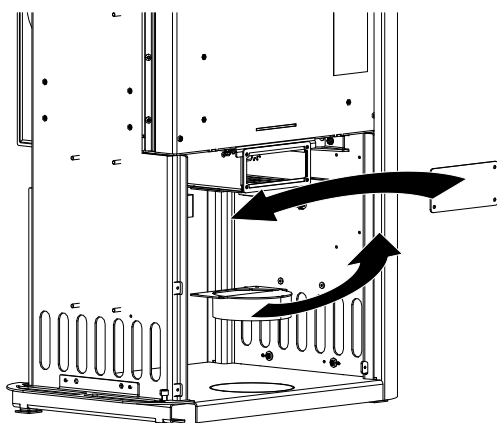
Fig. 17: Interchanger le collet d'arrivée d'air et le couvercle
