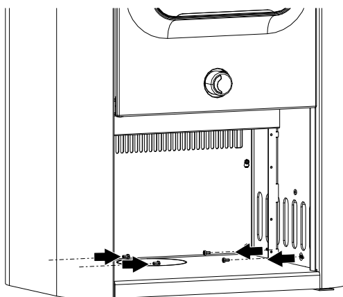
Fig. 51: Dévisser les vis en bas à l'intérieur
