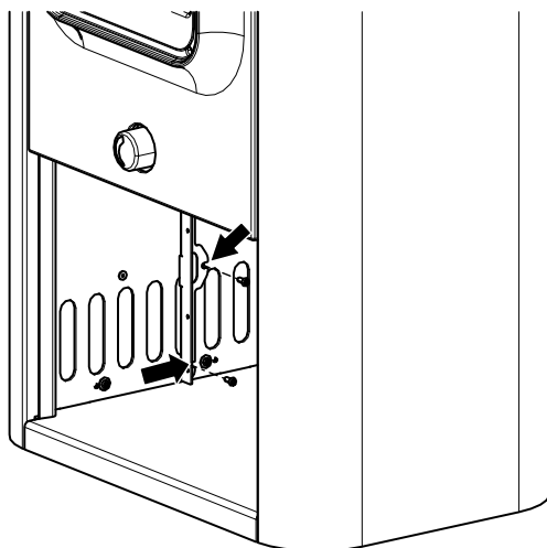
Fig. 34: Installer les fixations de l'obturateur de socle
