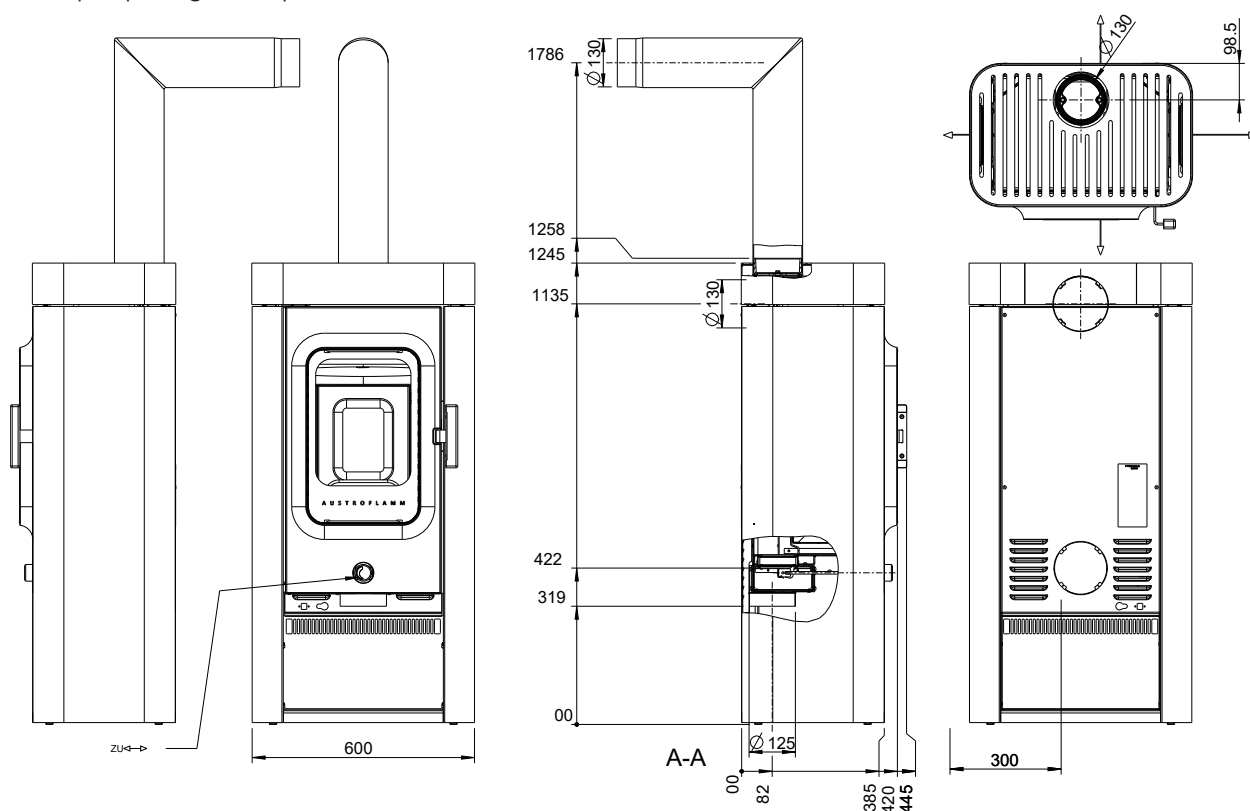
Fig. 1: Dimensions de l'appareil de base
