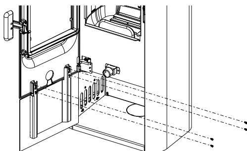
Fig. 32: Installer la porte pour socle
