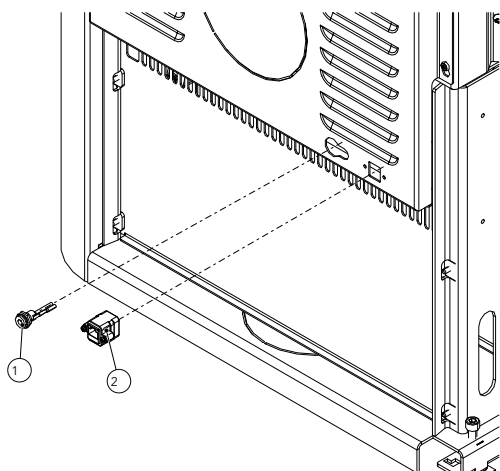
Fig. 23: Installer la prise CC et la prise réseau
