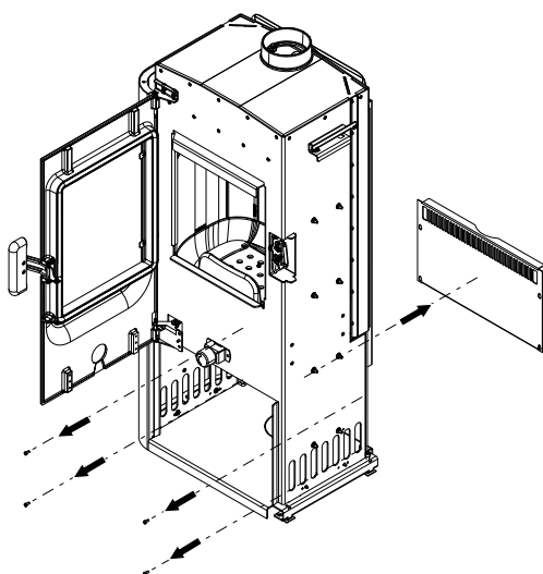
Fig. 13: Démontez le recouvrement arrière
