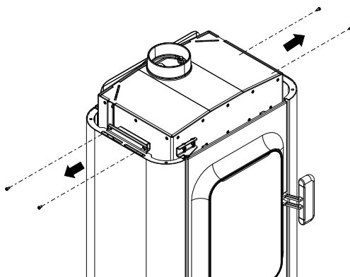
Fig. 50: Dévisser les vis ga + dr
