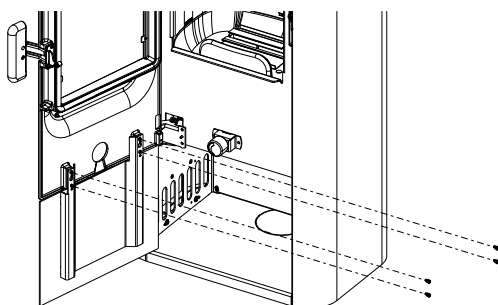
Fig. 32: Montaggio dello sportello dello zoccolo
