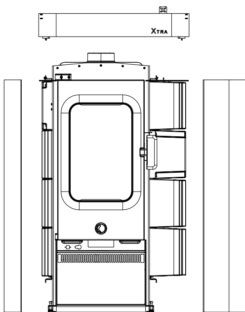
Fig. 30: Xtra montato
