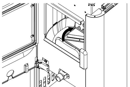
Fig. 45: Coperchio sul box cenere
