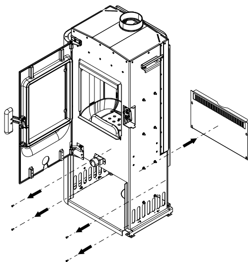
Fig. 13: Smontaggio del coperchio posteriore
