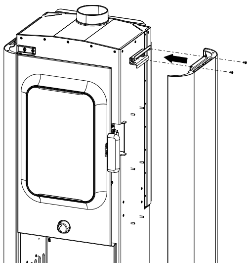
Fig. 5: Fissaggio del rivestimento laterale al supporto
