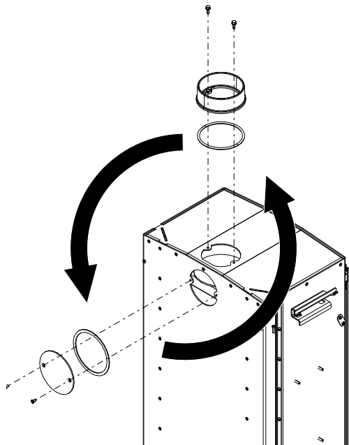
Fig. 10: Sostituzione del coperchio e del pezzo di collegamento
