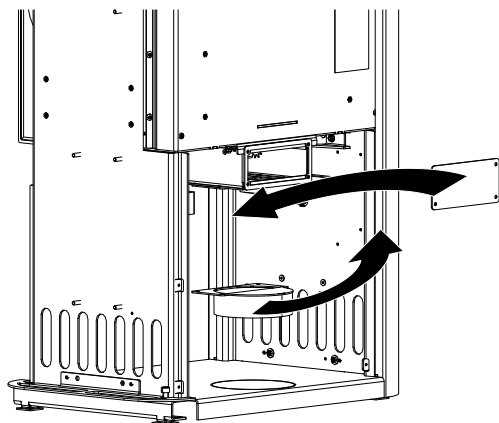
Fig. 17: Sostituzione della flangia e del coperchio
