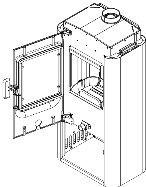
Fig. 53: Apertura dello sportello
