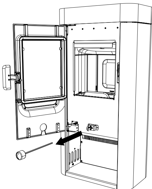
Fig. 19: Rimozione dell'unità del controllo rotativo
