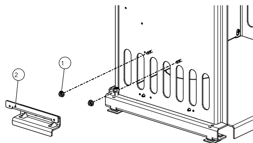
Fig. 25: Montaggio del supporto
