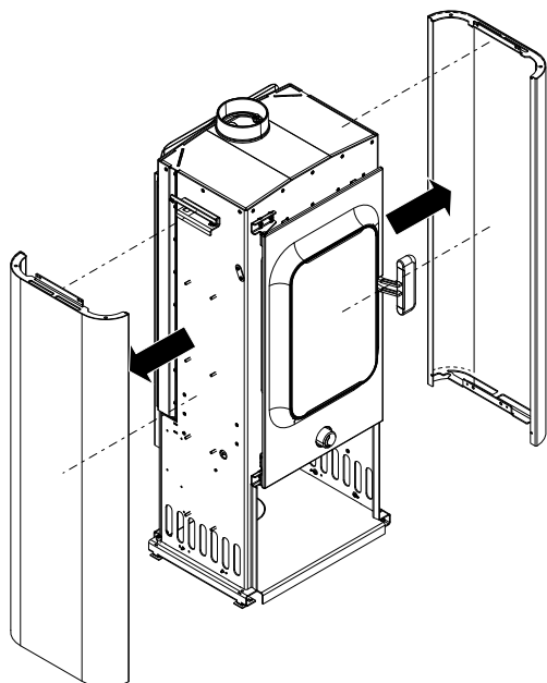
Fig. 52: Rimozione del rivestimento laterale
