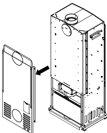
Fig. 8: Smontaggio della parete posteriore
