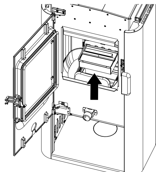
Fig. 47: Rimozione e svuotamento del box cenere
