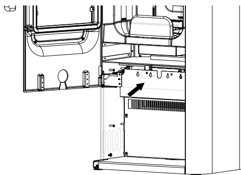
Fig. 24: Montaggio della copertura
