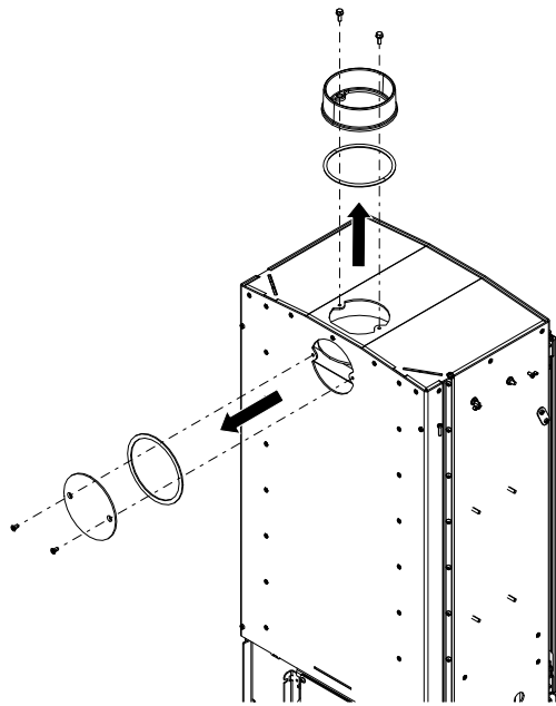
Fig. 9: Smontaggio del coperchio e del pezzo di collegamento
