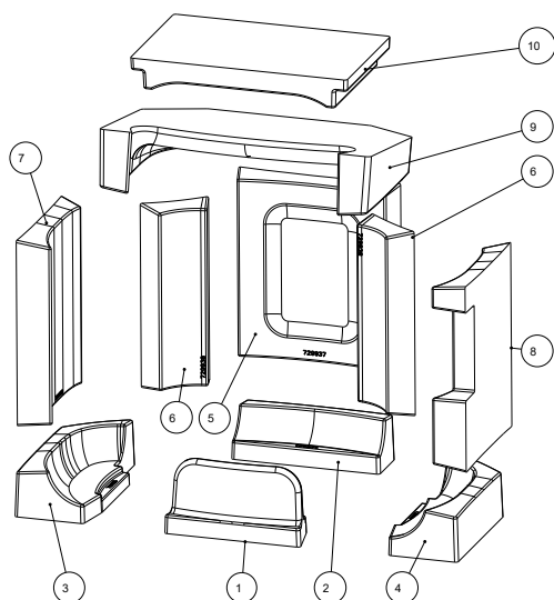
Fig. 36: Sequenza di installazione del Keramott
