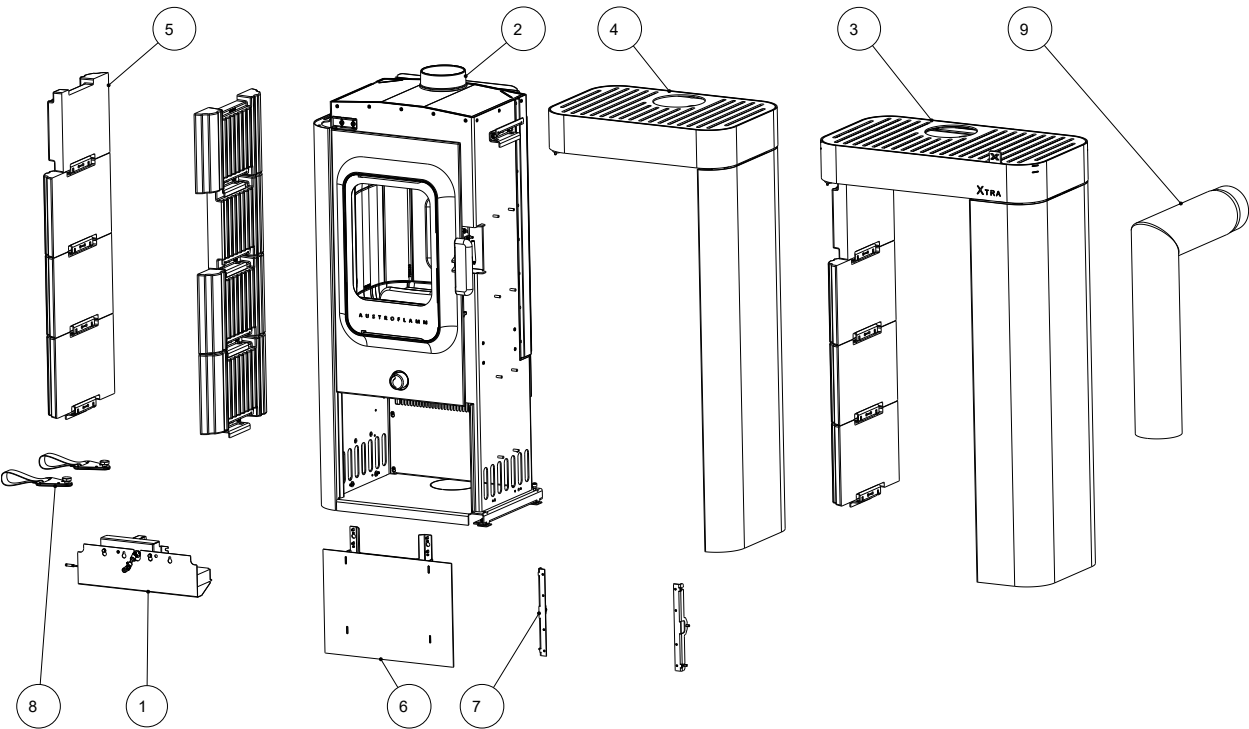
Fig. 48: Accessori
