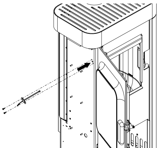
Fig. 22: Fissaggio del sensore di temperatura della camera di combustione
