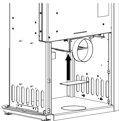
Fig. 18: Collegamento dell'aria posteriore
