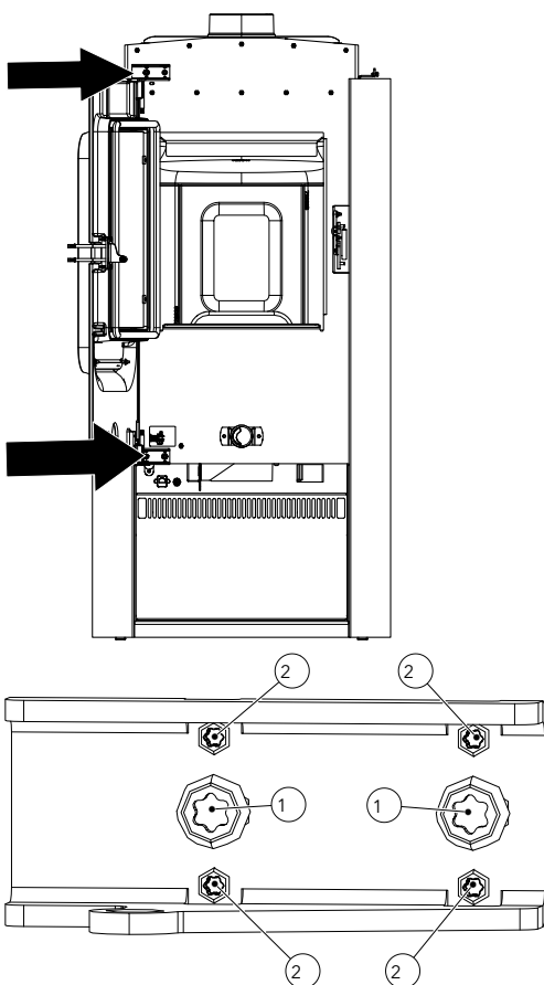
Fig. 38: Viti di registro dello sportello
