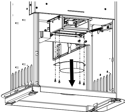
Fig. 16: Smontaggio della connessione dell'aria
