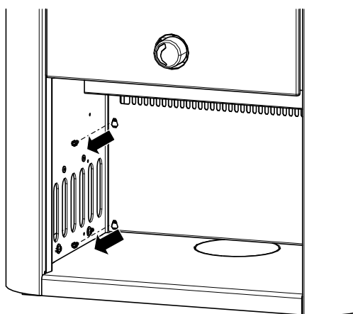
Fig. 33: Smontaggio della zoccolatura
