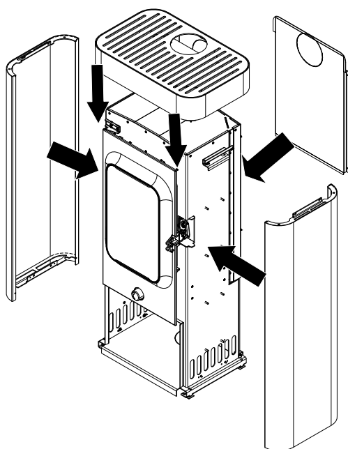
Fig. 12: Montaggio del rivestimento laterale, della parete posteriore e del coperchio
