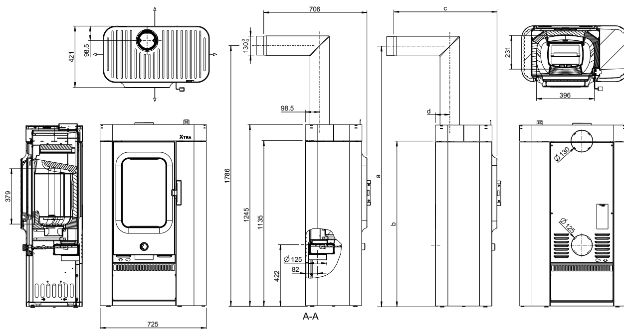
Fig. 2: Dimensioni incl. Xtra (opzione)
