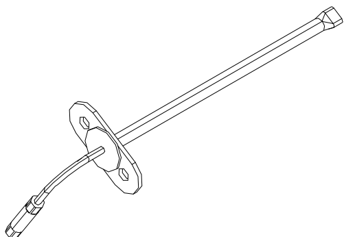
Fig. 21: Sensore temperatura camera di combustione
