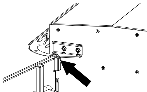
Fig. 54: Svitamento delle viti
