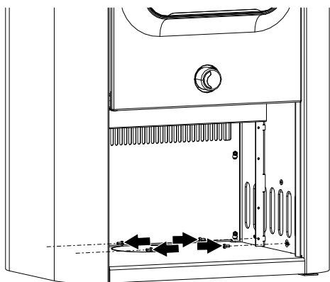
Fig. 6: Fissaggio del rivestimento laterale in basso dall'interno
