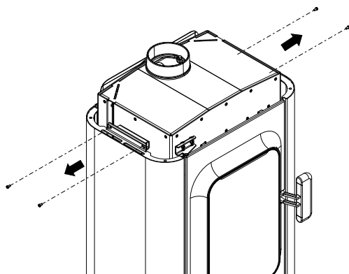
Fig. 50: Svitamento delle viti sx + dx
