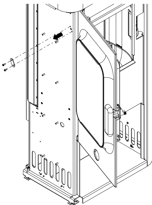
Fig. 20: Rimozione della piastra di copertura
