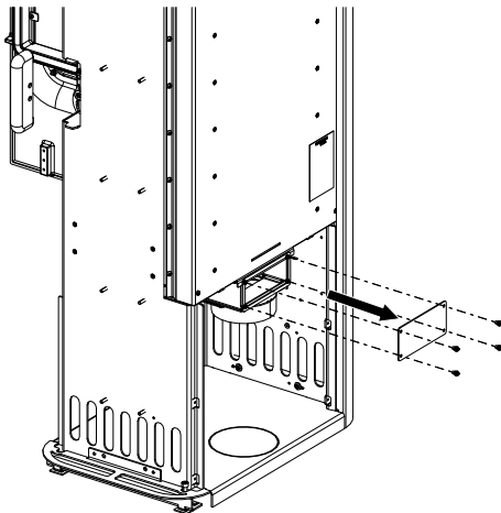
Fig. 15: Smontaggio del coperchio posteriore
