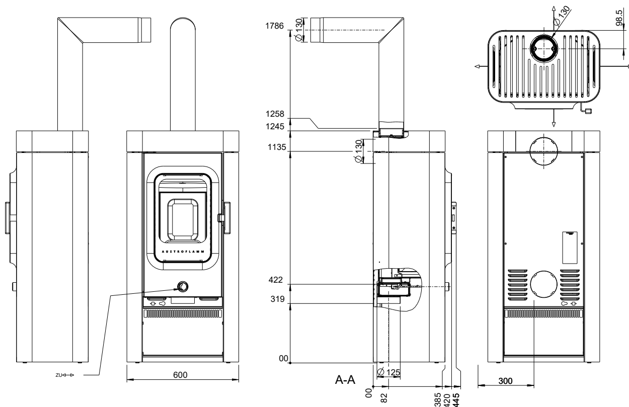
Fig. 1: Dimensioni dell'apparecchio di base
