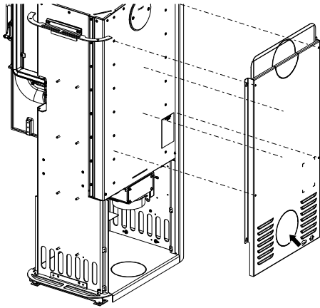
Fig. 14: Smontaggio della parete posteriore e rimozione della parte perforata
