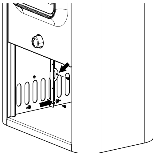
Fig. 34: Montaggio della zoccolatura
