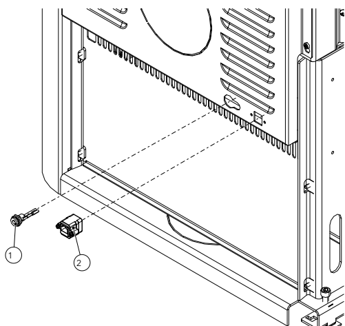
Fig. 23: Montaggio della presa DC e della presa di rete
