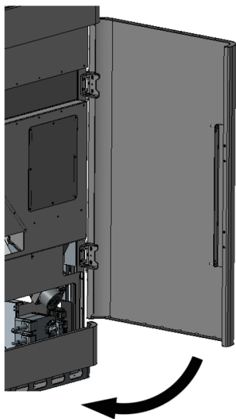
Fig. 22: Fermer l'habillage droit
