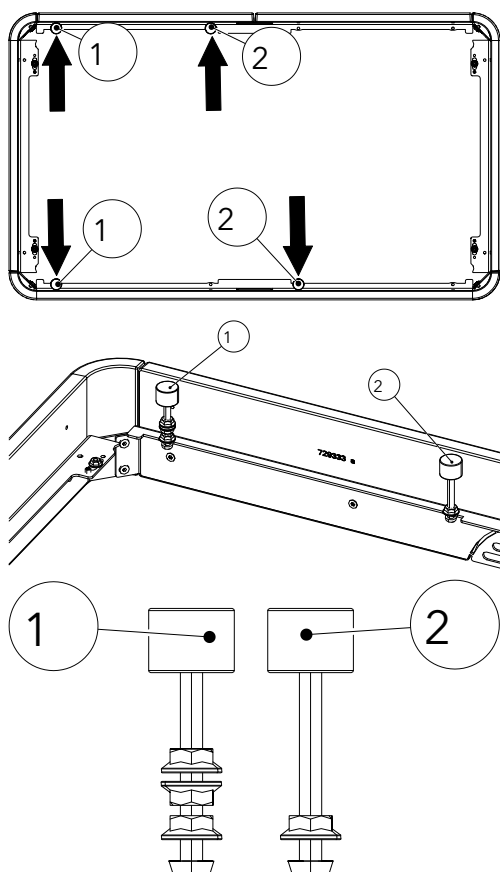
Fig. 47: Poser les vis, les écrous et les butoirs silicone/métal
