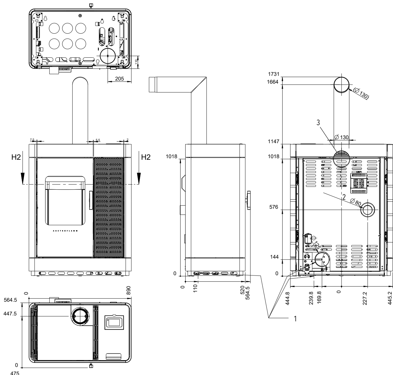
Fig. 3: Dimensions du Scotty Duo
