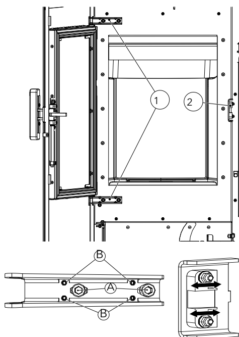
Fig. 116: Ajuster la porte du foyer
