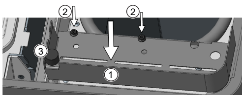
Fig. 31: Installer le réceptacle du réservoir
