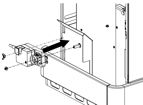
Fig. 43: Installer le moteur de la grille
