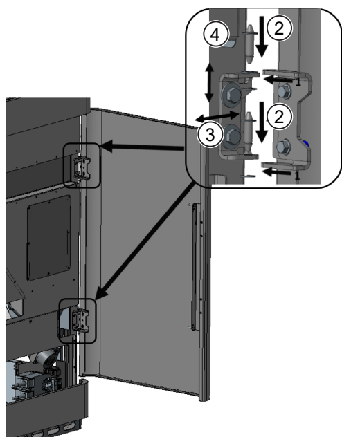
Fig. 20: Installer et ajuster l'habillage droit
