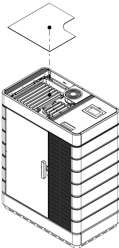
Fig. 72: Poser le couvercle en verre
