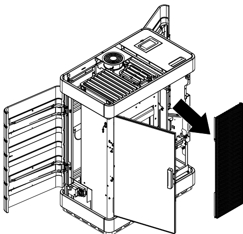
Fig. 59: Enlever l'habillage avant
