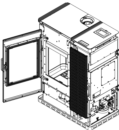
Fig. 115: Ouvrir la porte
