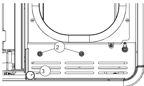
Fig. 68: Poser les écrous et les butoirs silicone/métal
