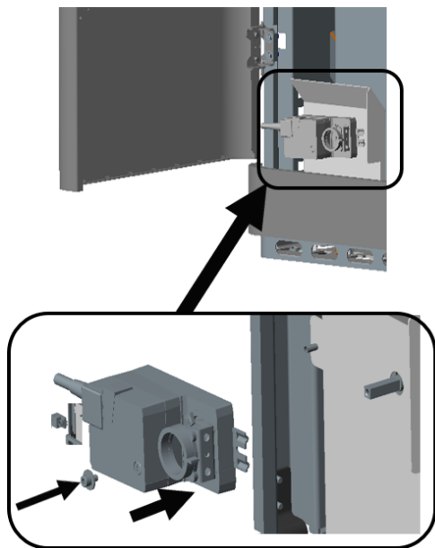
Fig. 16: Installer le moteur de la grille
