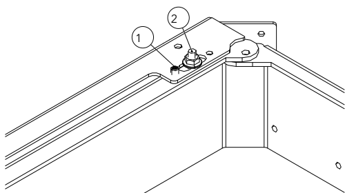
Fig. 51: Ajuster l'anneau supérieur
