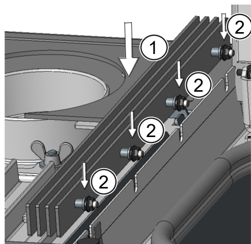
Fig. 32: Installer les lamelles de convection droites
