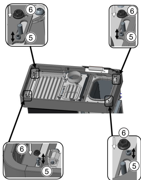
Fig. 18: Ajuster et visser à fond
