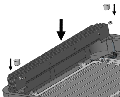
Fig. 33: Poser et ajuster les butoirs en silicone
