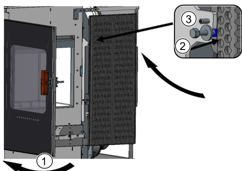
Fig. 25: Installer la plaque en acier de l'habillage avant
