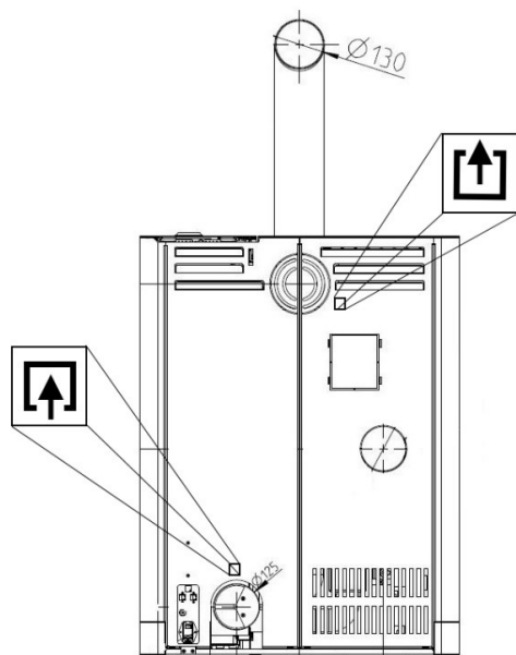
Fig. 89: Raccordement de l'alimentation en air de combustion
