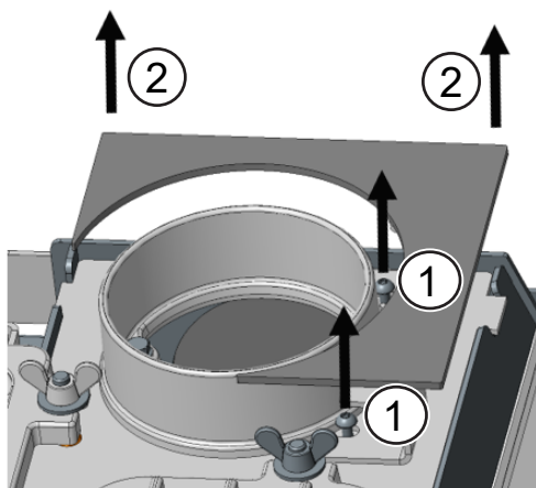
Fig. 15: Dévisser les vis et enlever le recouvrement
