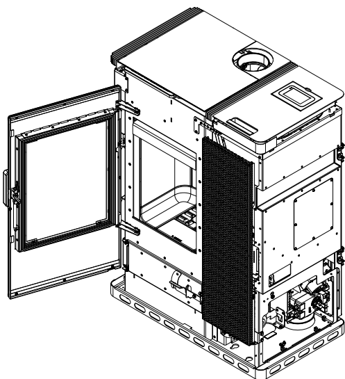
Fig. 111: Ouvrir la porte
