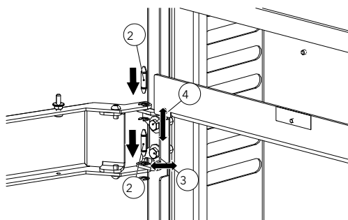
Fig. 54: Ajuster le cadre porteur
