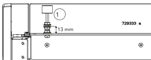
Fig. 49: Espacement de 13 mm
