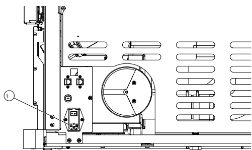
Fig. 74: Raccordement électrique
