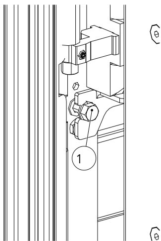
Fig. 65: Fixer la plaque céramique gauche
