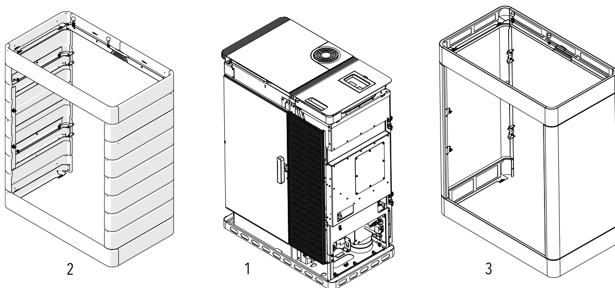
Fig. 2: Vue d'ensemble du Scotty Duo
