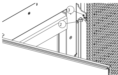
Fig. 64: Ajuster l'habillage
