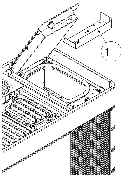
Fig. 67: Installer le réceptacle du réservoir
