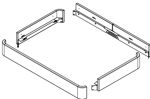
Fig. 45: Installer le cadre céramique supérieur
