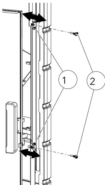
Fig. 60: Ajuster les plaques céramiques
