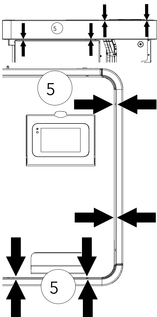
Fig. 52: Ajuster le cadre céramique supérieur
