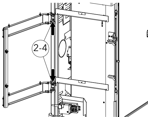
Fig. 53: Positionner le cadre porteur sur le poêle mixte
