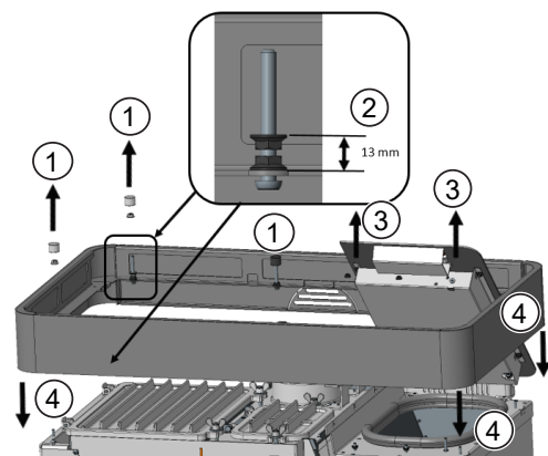
Fig. 17: Poser les butoirs silicone/métal
