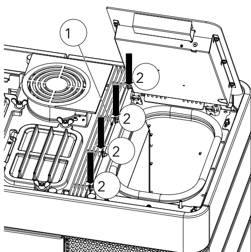
Fig. 69: Installer les lamelles de convection droites
