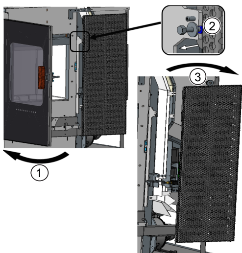
Fig. 21: Enlever l'habillage avant
