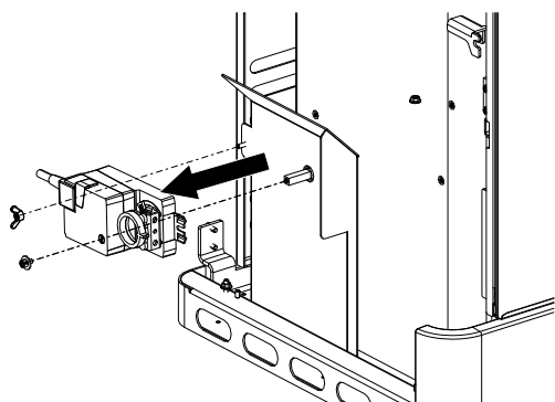
Fig. 38: Démontez le moteur de la grille
