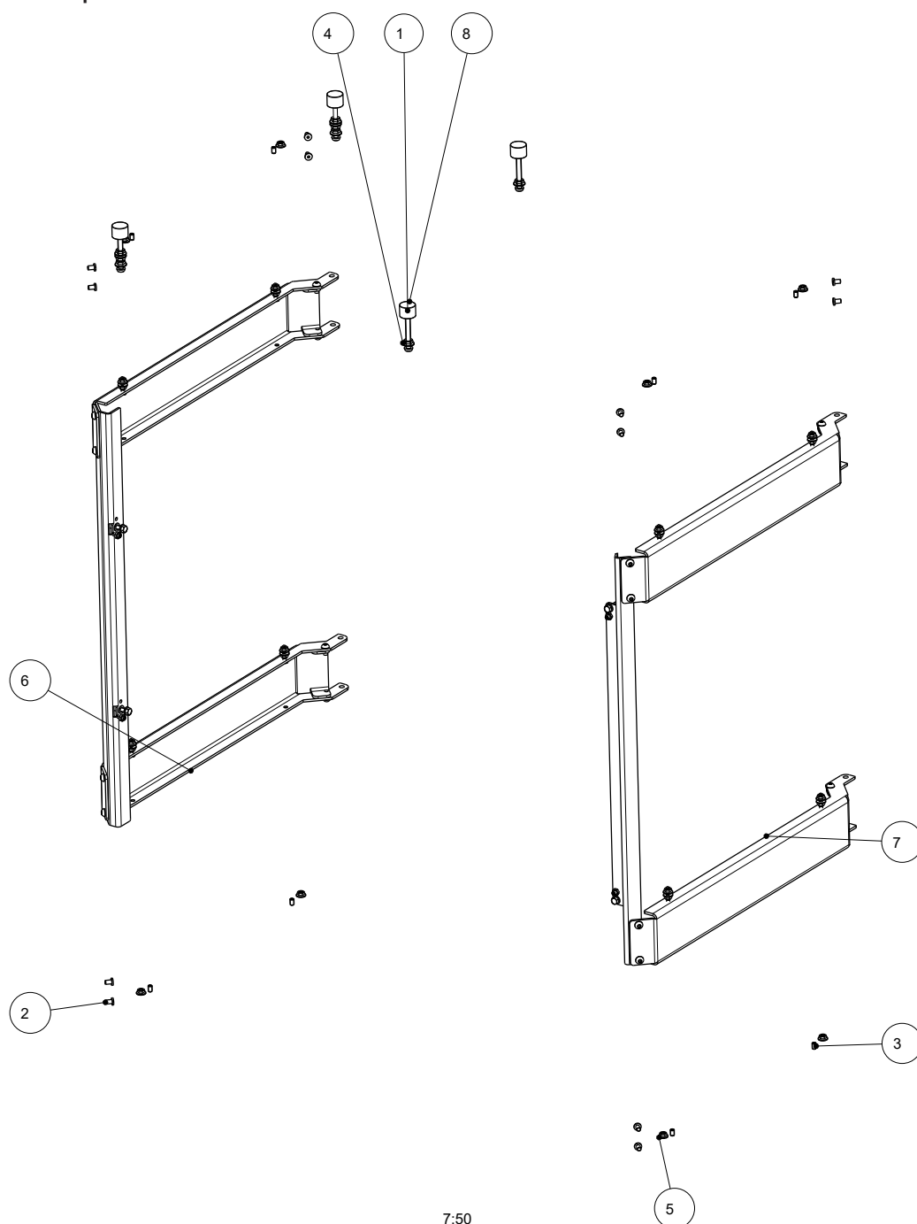
Fig. 36: Vue d'ensemble du cadre porteur
