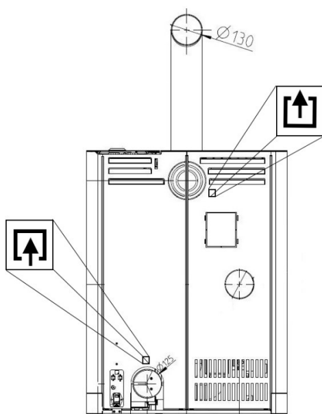
Fig. 73: Raccordement de l'alimentation en air de combustion
