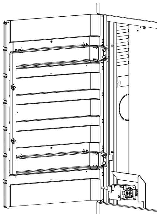
Fig. 56: Installer les plaques céramiques latérales
