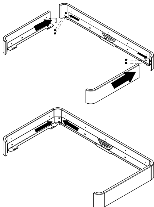
Fig. 39: Installer le cadre céramique bas
