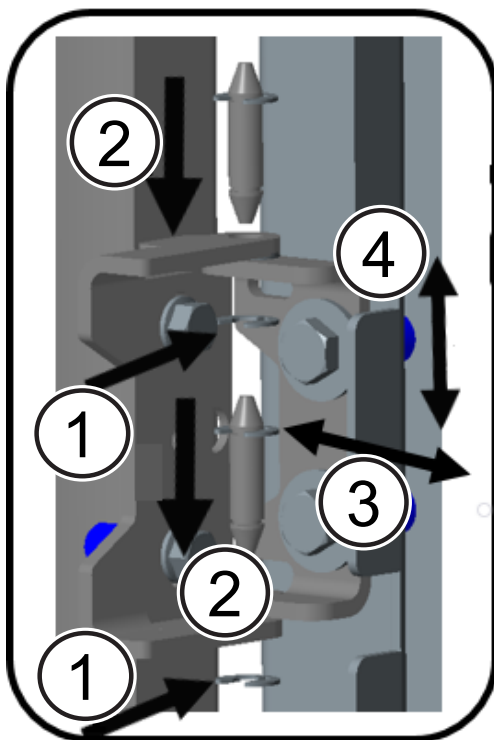
Fig. 26: Installer la plaque en acier gauche et l'ajuster
