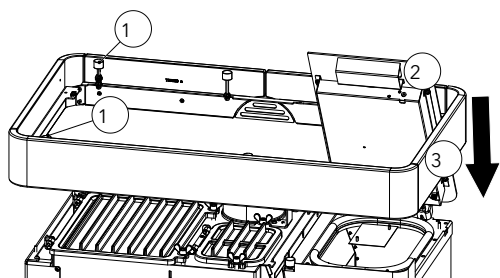
Fig. 50: Poser l'anneau supérieur
