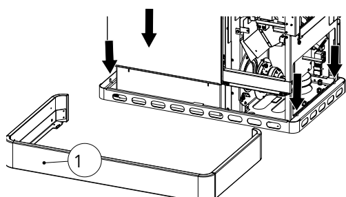
Fig. 40: Installer le socle
