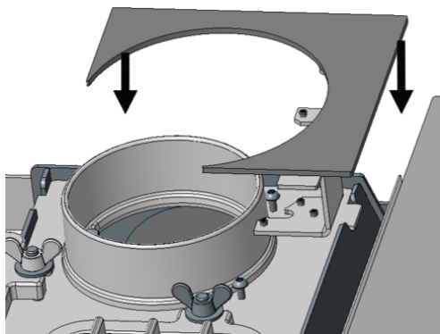
Fig. 29: Poser le recouvrement
