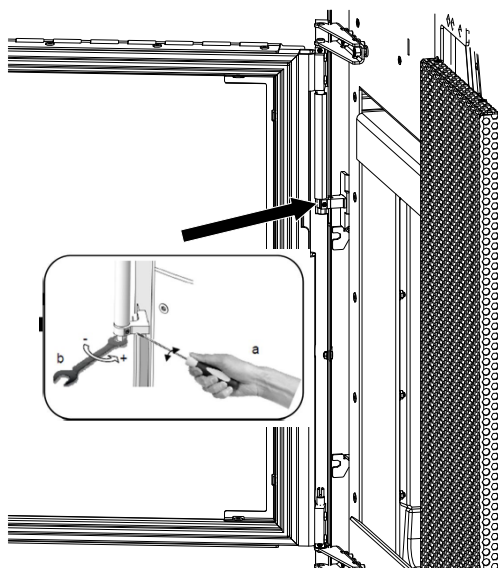
Fig. 112: Ajuster le ressort de tension
