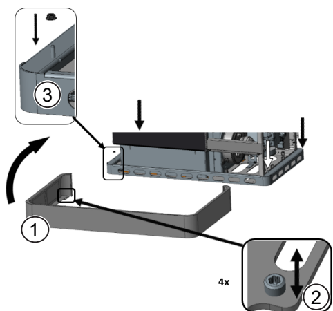
Fig. 13: Installer et ajuster le socle de l'habillage
