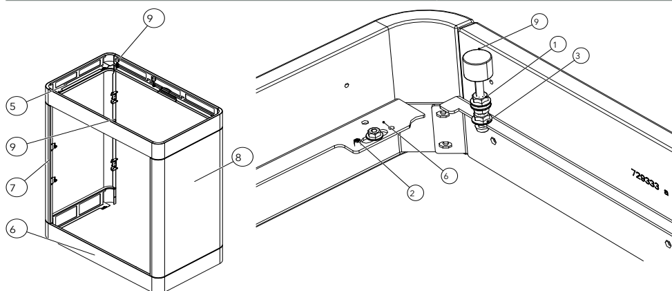
Fig. 10: Composants de l'habillage en acier
