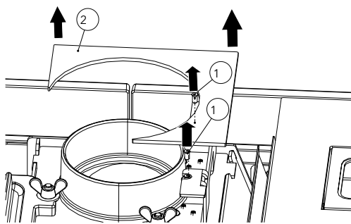
Fig. 44: Dévisser les vis et enlever le recouvrement
