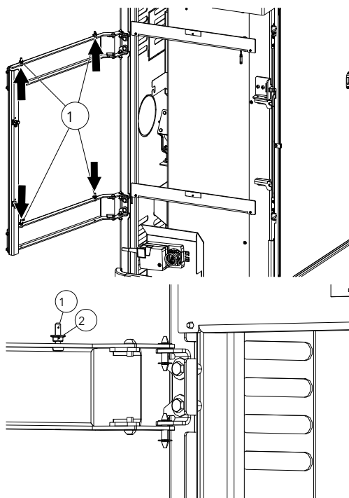
Fig. 55: Poser les vis et les écrous
