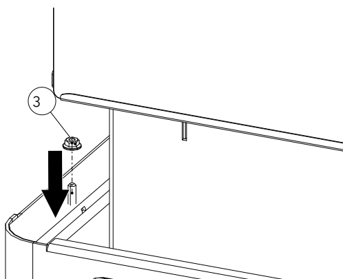
Fig. 42: Poser les quatre écrous et les visser à fond
