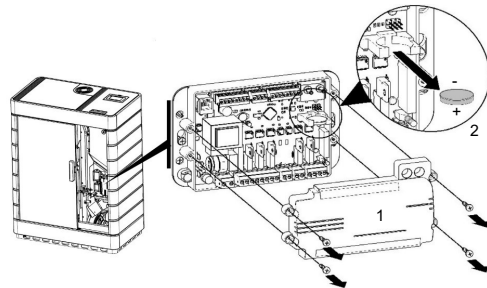
Fig. 119: Remplacer la pile mémoire
