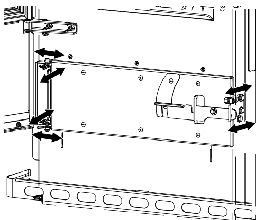
Fig. 114: Ajuster la porte du tiroir à cendres
