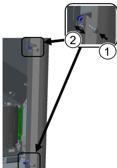
Fig. 23: Ajuster l'habillage droit
