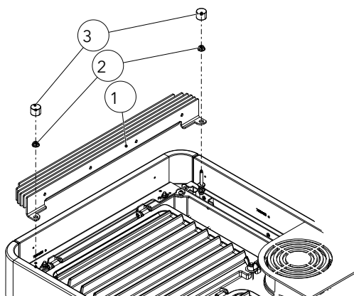
Fig. 71: Installer les lamelles de convection gauches
