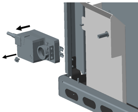
Fig. 12: Démontez le moteur de la grille
