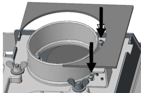
Fig. 30: Fixer les vis (TX25)
