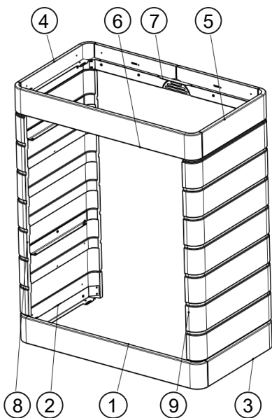
Fig. 35: Vue d'ensemble de l'habillage céramique
