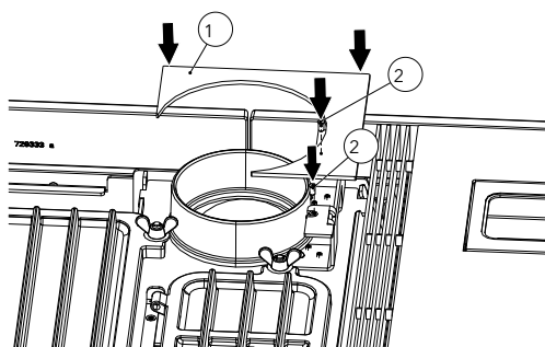
Fig. 70: Poser le recouvrement
