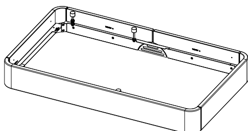
Fig. 48: Cadre céramique supérieur assemblé
