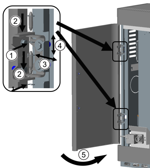
Fig. 25: Installer la plaque en acier de l'habillage avant
