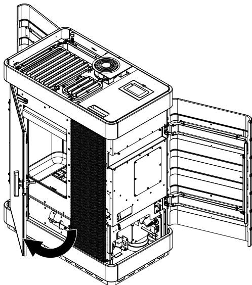
Fig. 57: Apertura dello sportello
