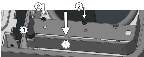
Fig. 31: Montaggio della nicchia del contenitore
