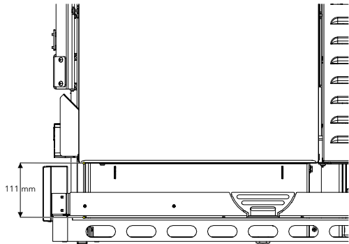
Fig. 37: Controllo della distanza
