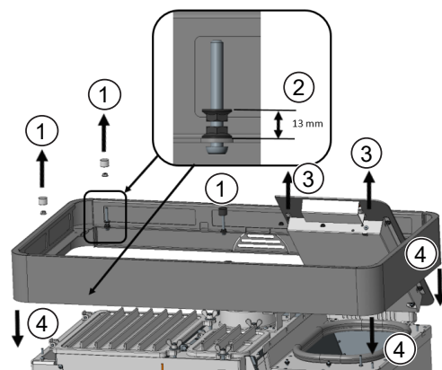
Fig. 17: Montaggio del tampone in silicone metallico
