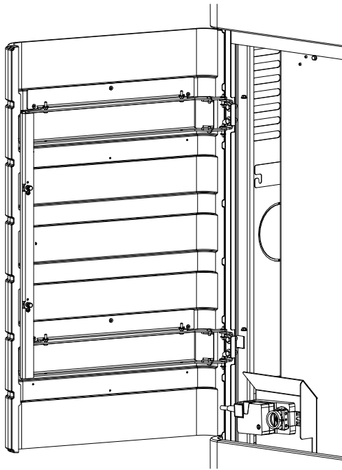
Fig. 56: Posizionamento dei piani in ceramica
