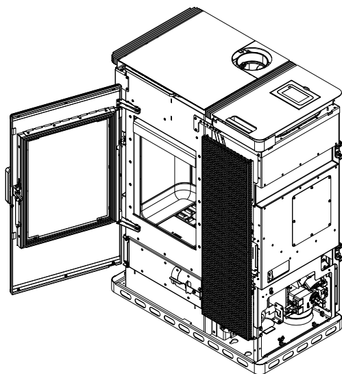
Fig. 113: Apertura dello sportello
