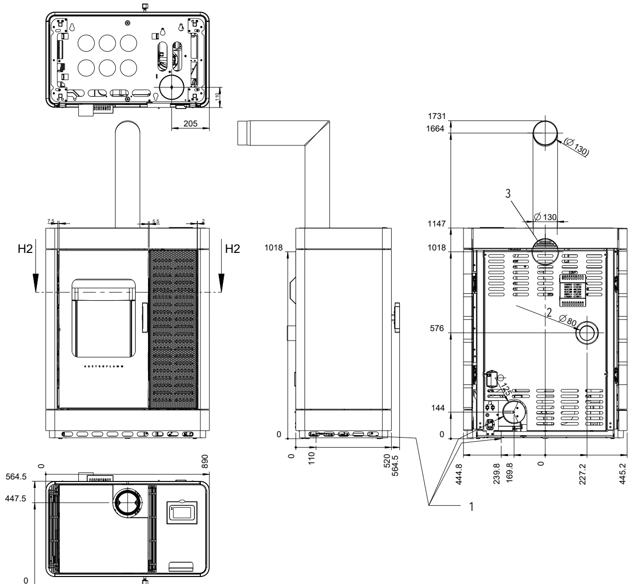
475 Fig. 3: Scotty Duo - Dimensioni
