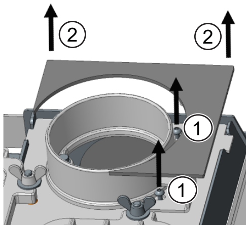
Fig. 15: Svitamento delle viti - Rimozione della copertura
