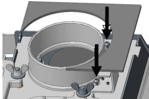
Fig. 30: Fissare le viti (TX25)
