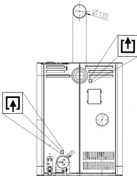
Fig. 73: Collegamento dell'alimentazione esterna di aria comburente
