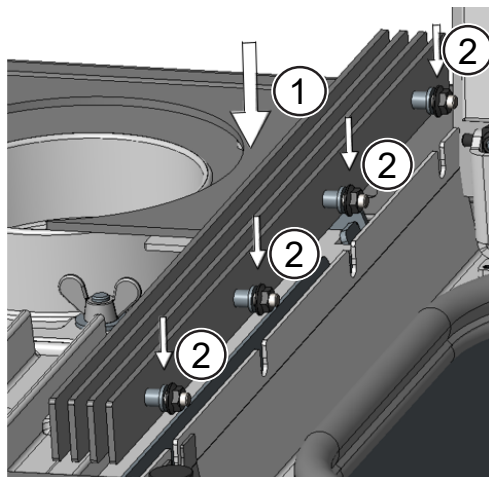
Fig. 32: Montaggio delle alette di convezione sulla destra
