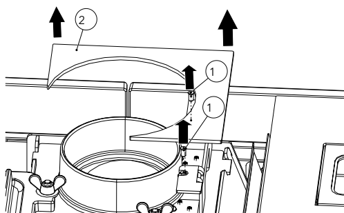
Fig. 44: Svitamento delle viti e rimozione della copertura
