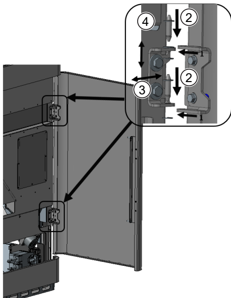
Fig. 20: Montaggio e allineamento del rivestimento di destra
