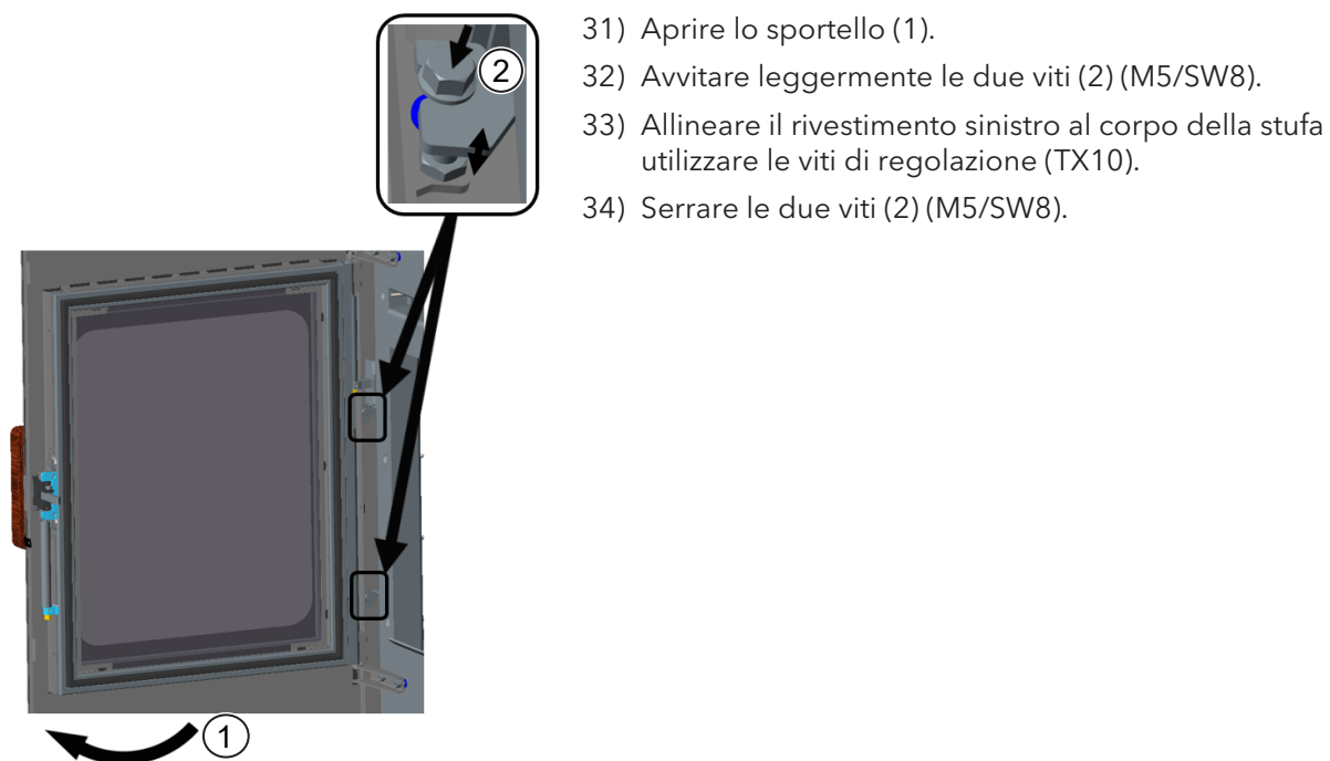
Fig. 27: Fissaggio del lato sinistro
