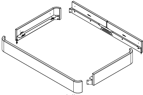
Fig. 45: Montaggio della struttura in ceramica superiore
