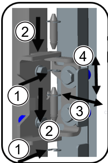
Fig. 26: Montaggio e allineamento della piastra d'acciaio di sinistra
