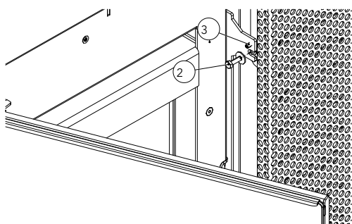
Fig. 64: Allineamento del rivestimento
