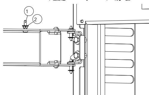
Fig. 55: Montaggio delle viti e dei dadi
