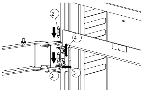
Fig. 54: Allineamento della struttura portante
