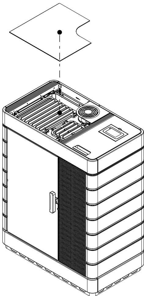
Fig. 72: Inserimento del coperchio dell'inserto in vetro
