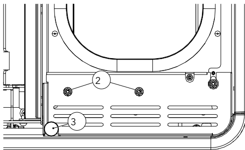
Fig. 68: Montaggio dei dadi e del tampone in silicone metallico
