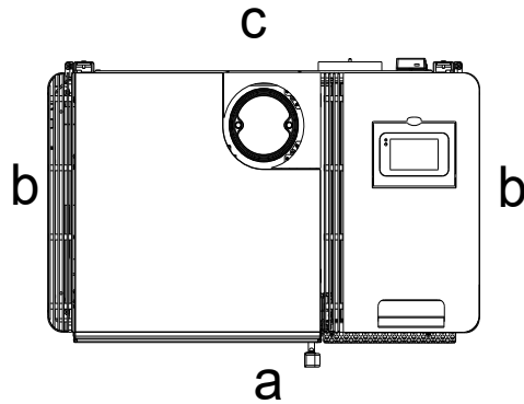
Fig. 1: Distanze di sicurezza (vista dall'alto)
