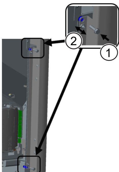
Fig. 23: Allineamento del rivestimento di destra
