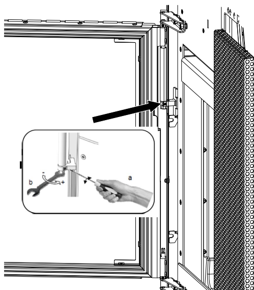
Fig. 112: Regolazione della molla di pressione
