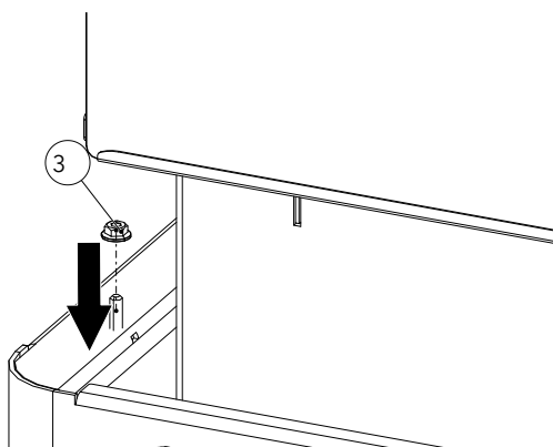
Fig. 42: Montaggio e serraggio dei dadi
