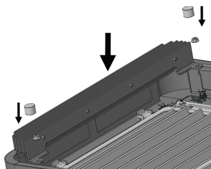
Fig. 33: Montare e allineare il tampone di silicone
