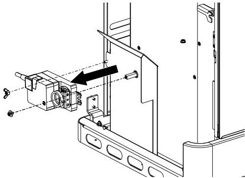
Fig. 38: Smontaggio del motore della griglia
