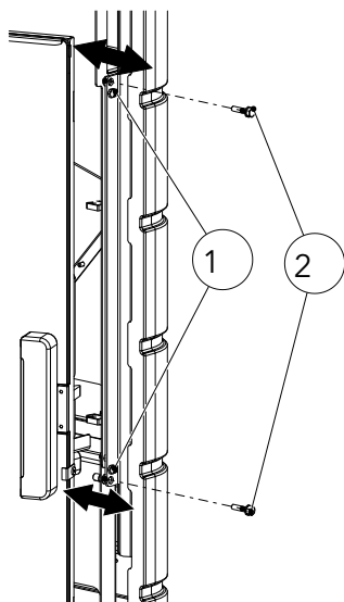
Fig. 60: Allineamento dei piani in ceramica
