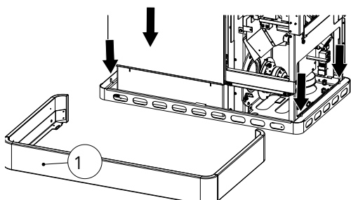
Fig. 40: Montaggio della base
