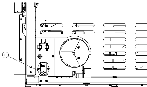
Fig. 74: Collegamento elettrico
