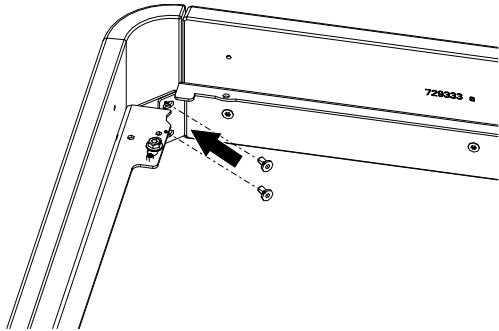
Fig. 46: Allineamento delle otto viti
