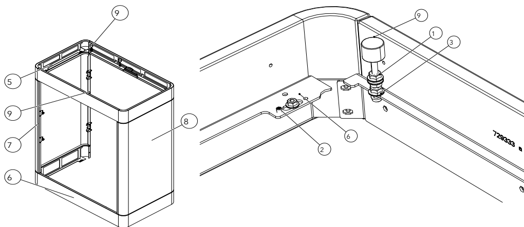
Fig. 10: Rivestimento pezzo singolo
