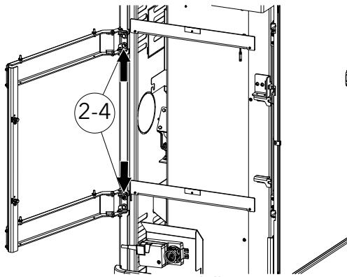
Fig. 53: Posizionamento della struttura portante sulla stufa combi
