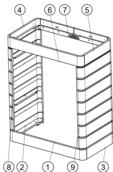
Fig. 35: Panoramica - Rivestimento in ceramica
