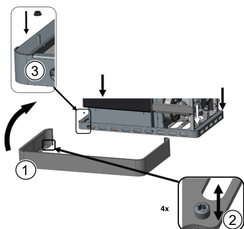
Fig. 13: Montaggio e allineamento del rivestimento della base
