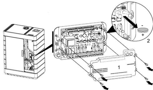
Fig. 119: Sostituzione della batteria tampone
