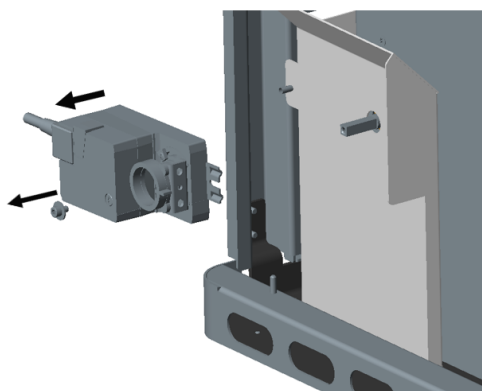
Fig. 12: Smontaggio del motore della griglia
