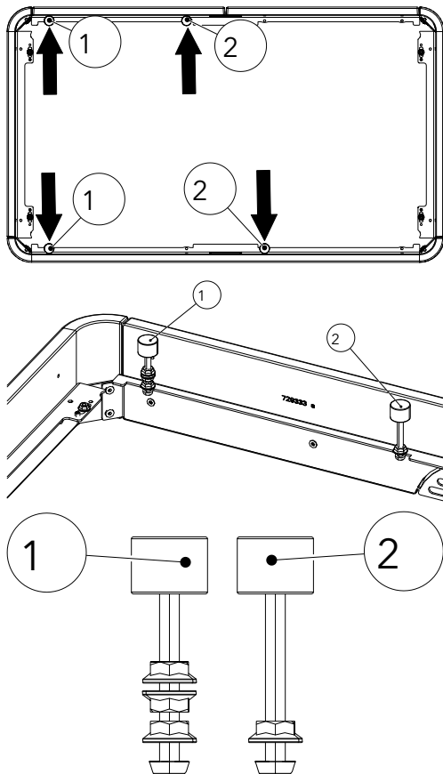
Fig. 47: Montaggio delle viti, dei dadi e del tampone in silicone metallico
