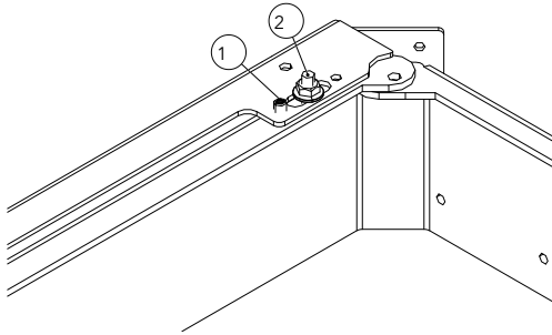
Fig. 51: Allineamento dell'anello superiore
