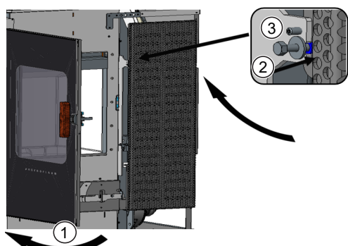
Fig. 25: Montaggio della piastra di rivestimento anteriore in acciaio
