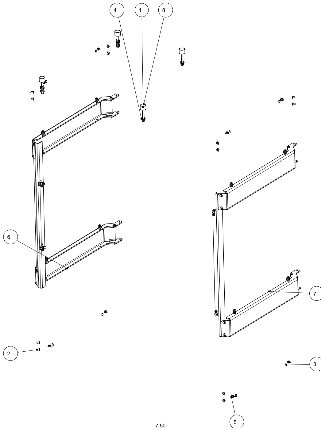
Fig. 36: Panoramica struttura portante
