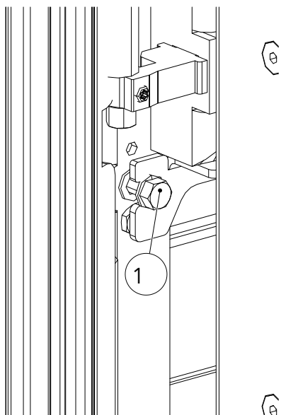
Fig. 65: Fissaggio del piano in ceramica sinistro
