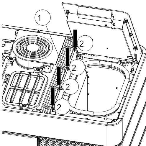
Fig. 69: Montaggio delle alette di convezione sulla destra
