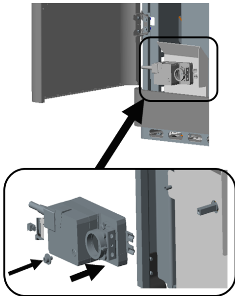
Fig. 16: Montaggio del motore della griglia
