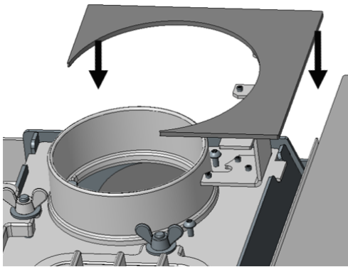
Fig. 29: Montaggio della copertura
