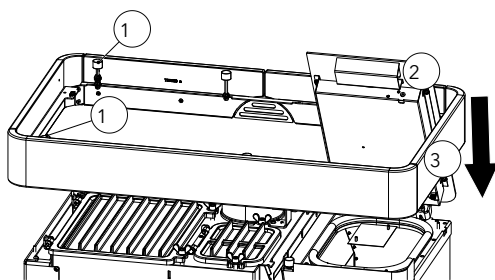
Fig. 50: Montaggio dell'anello superiore
