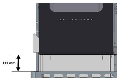
Fig. 11: Controllo della distanza
