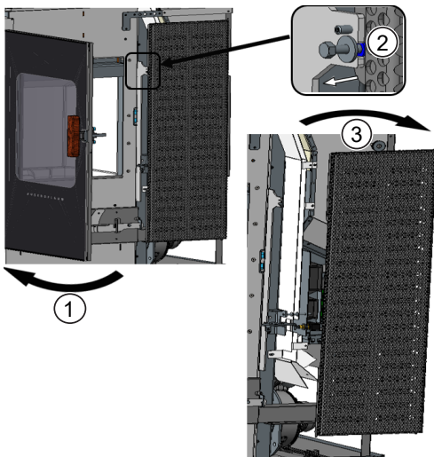
Fig. 21: Rimozione del rivestimento anteriore
