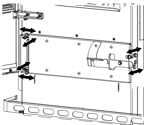
Fig. 114: Regolazione dello sportello del vassoio per la cenere
