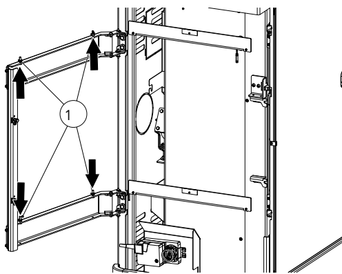
Fig. 54: Allineamento della struttura portante
