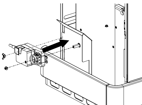
Fig. 43: Montaggio del motore della griglia
