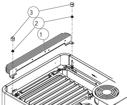
Fig. 71: Montaggio delle alette di convezione a sinistra.
