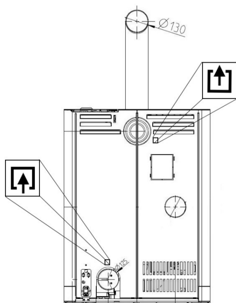
Fig. 89: Collegamento dell'alimentazione esterna di aria comburente
