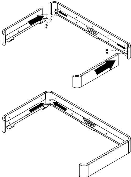
Fig. 39: Montaggio della struttura in ceramica inferiore
