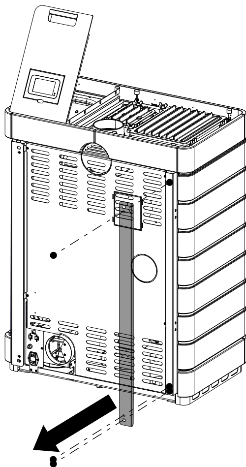
Abb. 25: Blende demontieren
