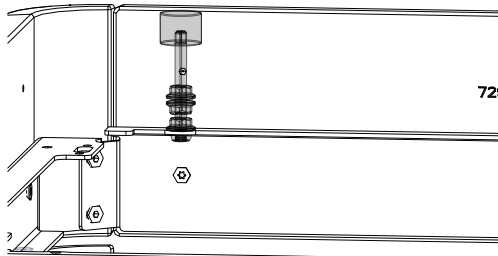
Abb. 19: Schrauben, Muttern und Silikon-Metall-Puffer montieren
