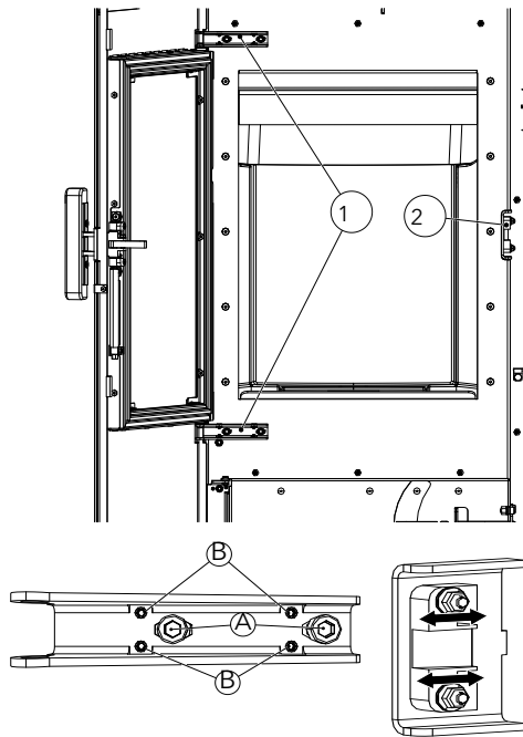
Abb. 86: Feuerraumtür einstellen
