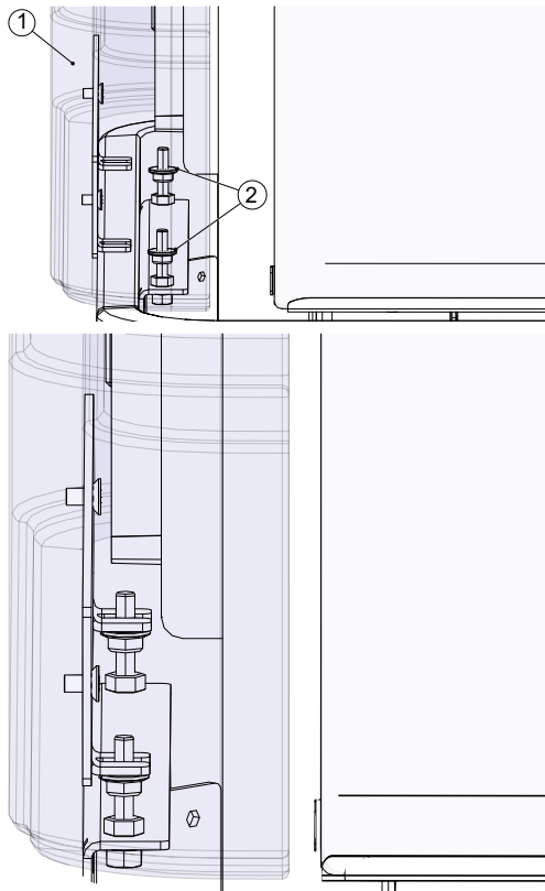
Abb. 26: Seitenverkleidung anbringen
