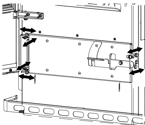
Abb. 84: Ascheladentür einstellen
