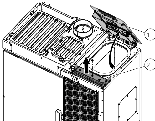
Abb. 21: Behälterdeckel öffnen
