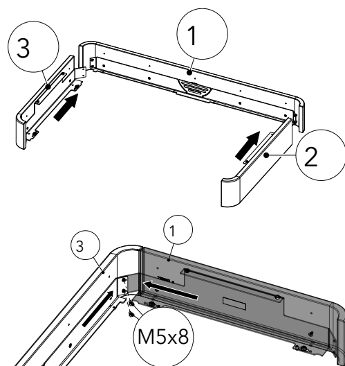
Fig. 11: Montaggio della struttura in ceramica inferiore
