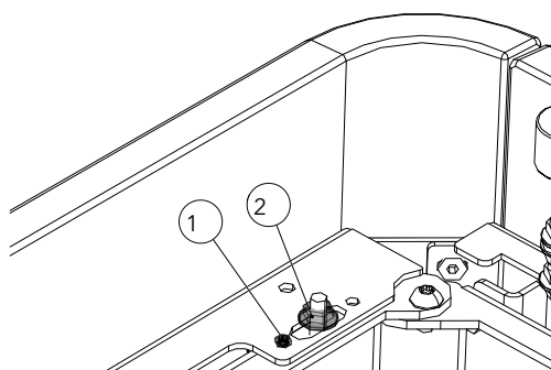
Fig. 23: Allineamento dell'anello superiore
