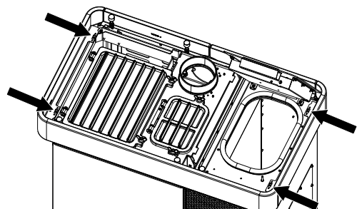
Fig. 22: Apertura del coperchio della coclea
