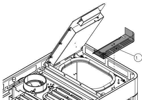
Fig. 64: Montaggio della nicchia del contenitore
