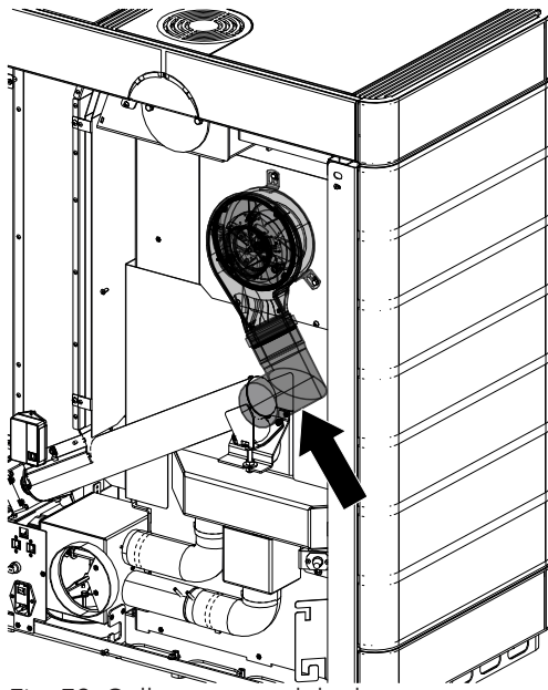
Fig. 79: Collegamento del tubo
