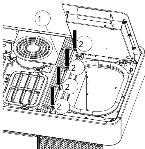
Fig. 66: Montaggio delle alette di convezione sulla destra
