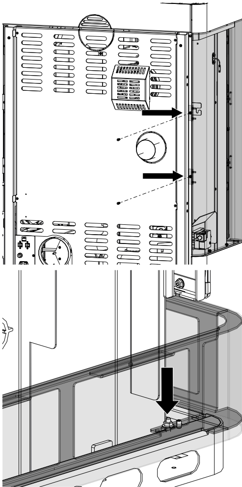
Fig. 55: Fissaggio del rivestimento in acciaio da dietro
