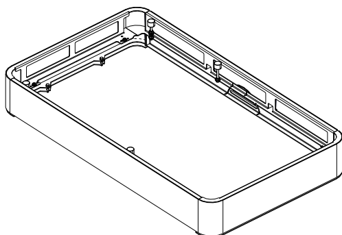
Fig. 47: Assemblaggio della base superiore
