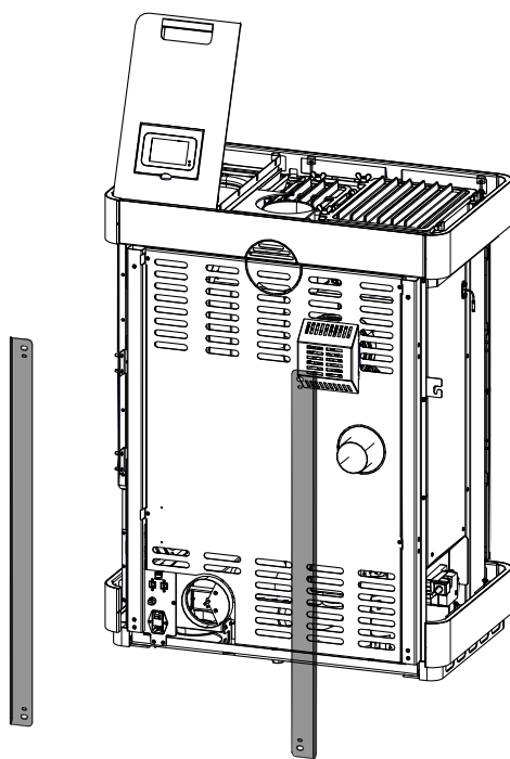
Fig. 54: Smontaggio dei diaframmi
