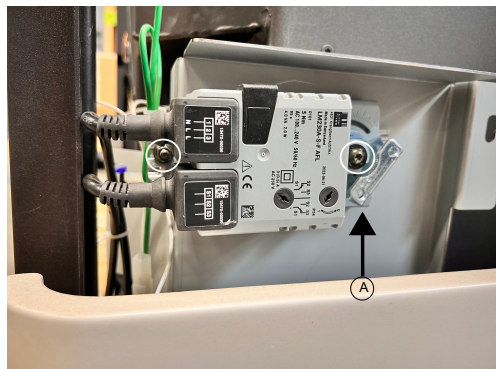
Fig. 16: Smontaggio del motore della griglia ribaltabile
