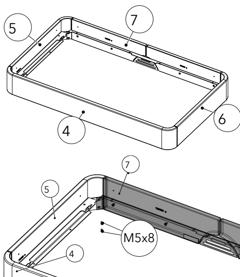
Fig. 17: Montaggio della struttura in ceramica superiore
