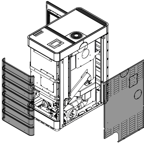
Fig. 72: Rimozione della parte posteriore e del rivestimento laterale
