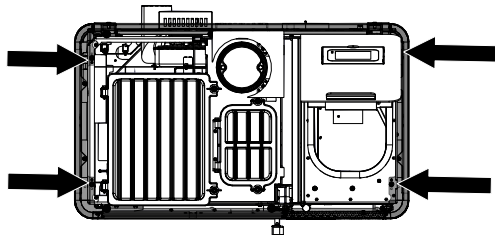
Fig. 51: Montaggio dell'anello superiore
