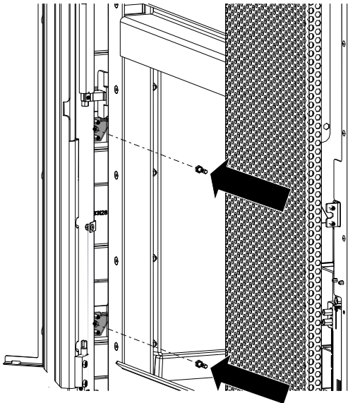
Fig. 56: Apertura dello sportello e fissaggio del rivestimento in acciaio
