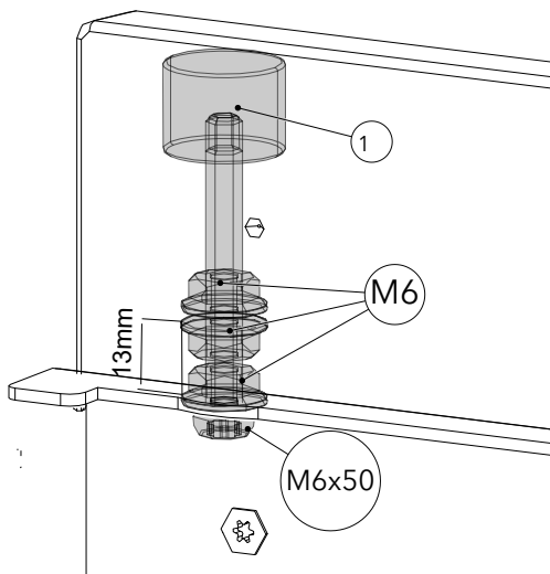
Fig. 48: Distanza a 13 mm
