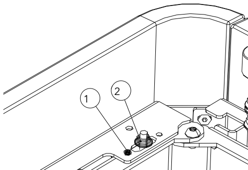
Fig. 52: Allineamento dell'anello superiore
