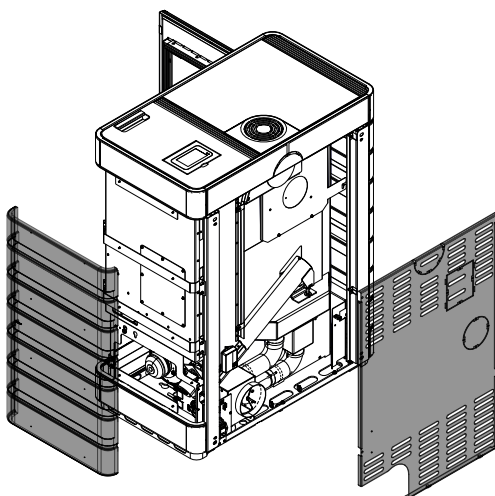
Fig. 81: Rimontaggio di tutte le parti
