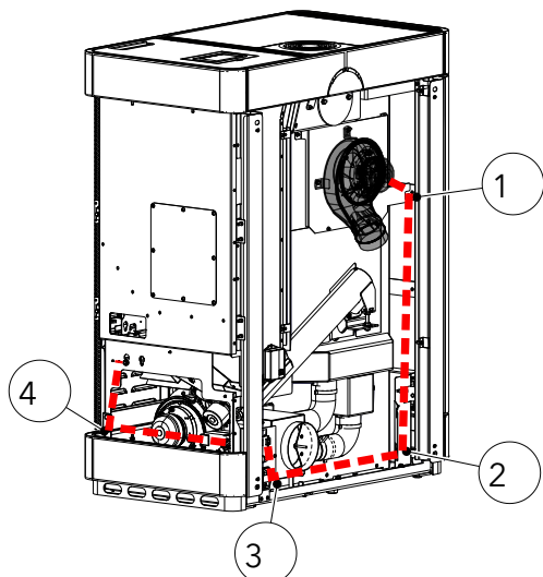
Fig. 75: Posa del cavo
