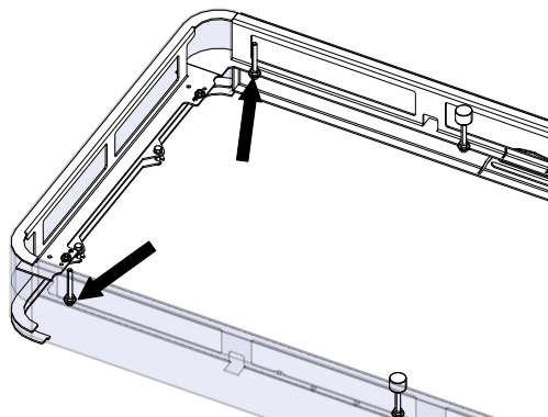
Fig. 67: Montaggio della copertura
