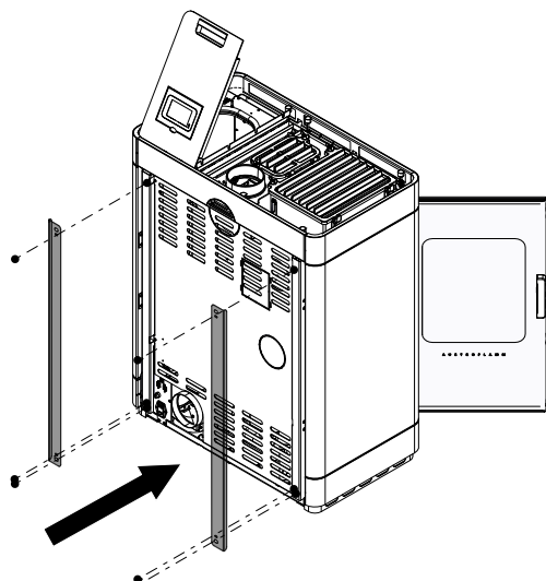
Fig. 63: Montaggio dei diaframmi
