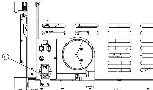
Fig. 141: Collegamento elettrico
