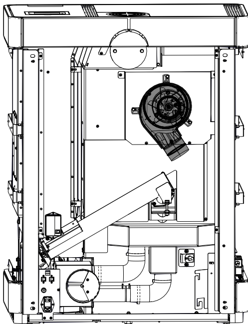
Fig. 72: Rimozione della parte posteriore e del rivestimento laterale
