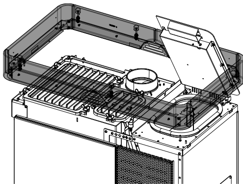
Fig. 51: Montaggio dell'anello superiore
