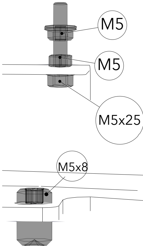
Fig. 12: Pre-assemblaggio delle viti
