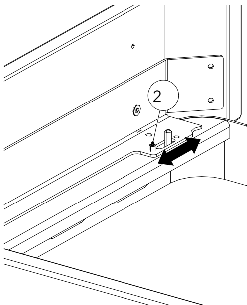
Fig. 14: Allineamento della base
