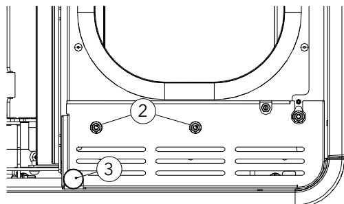
Fig. 65: Montaggio dei dadi e del tampone in silicone metallico
