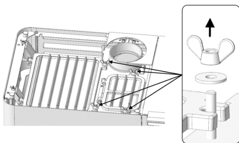
Fig. 132: Rimuovere la piastra
