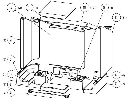
Fig. 10: Montaggio del Keramott
