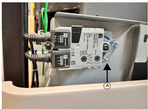
Fig. 44: Smontaggio del motore della griglia ribaltabile
