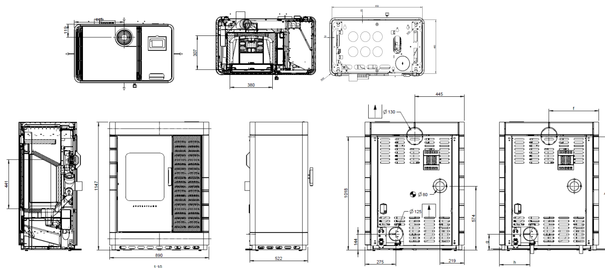
Fig. 2: Scotty Duo - Dimensioni
