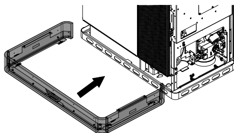
Fig. 13: Montaggio della base
