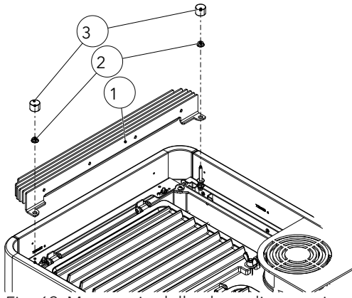
Fig. 69: Montaggio delle alette di convezione a sinistra.
