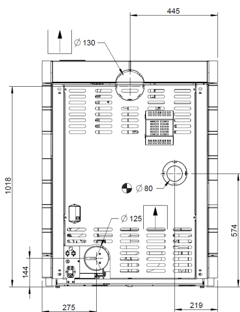
Fig. 83: Collegamento dell'alimentazione esterna di aria comburente
