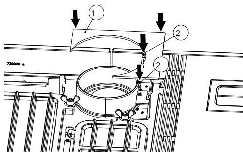
Fig. 67: Montaggio della copertura
