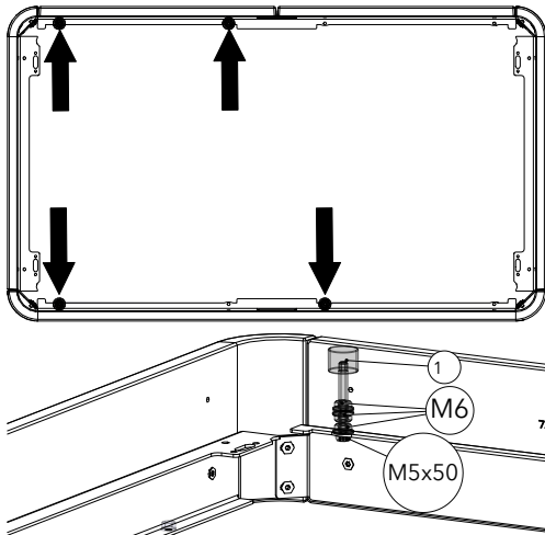
Fig. 18: Montaggio delle viti, dei dadi e del tampone in silicone metallico
