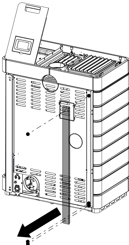
Fig. 25: Smontaggio del diaframma
