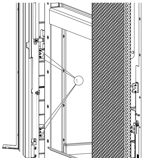
Fig. 57: Allineamento del rivestimento in acciaio
