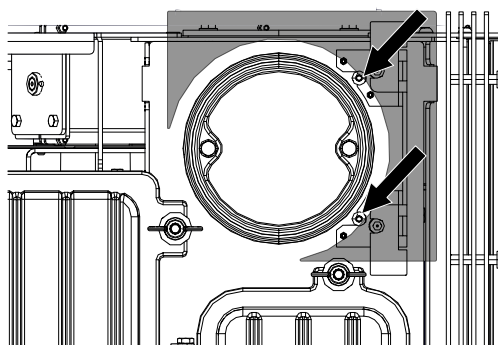
Fig. 49: Svitamento delle viti e rimozione della copertura
