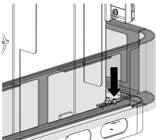
Fig. 45: Regolazione della base
