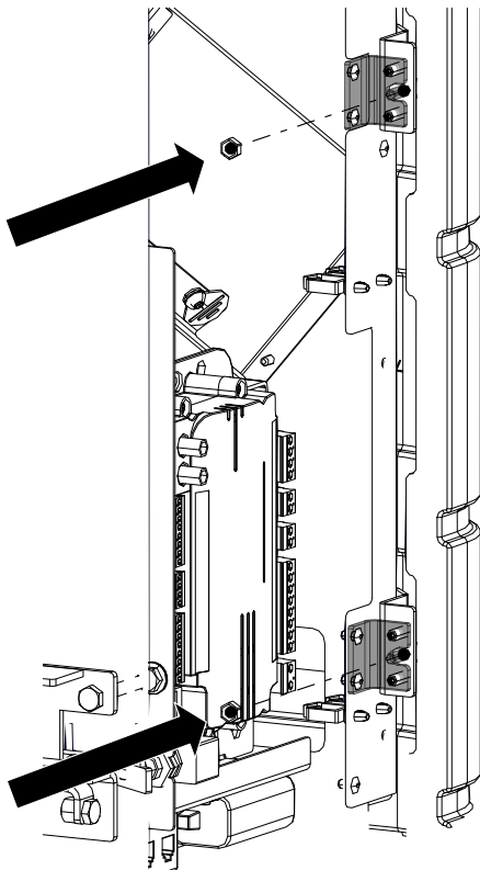
Fig. 60: Fissaggio e allineamento del rivestimento laterale
