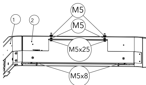
Fig. 11: Montaggio della struttura in ceramica inferiore
