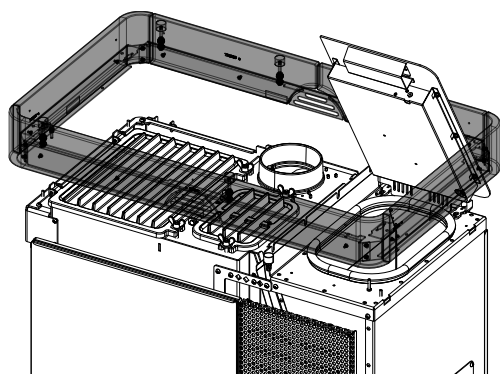
Fig. 22: Apertura del coperchio della coclea
