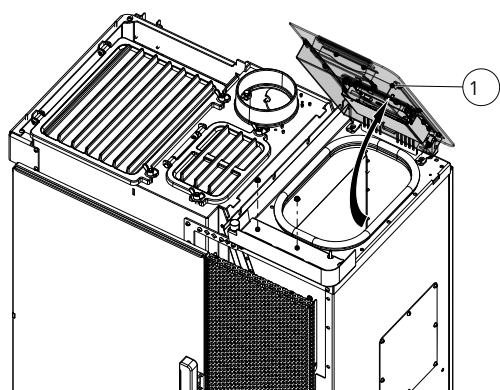
Fig. 21: Apertura del coperchio del contenitore
