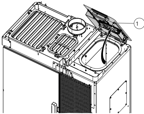
Fig. 50: Apertura del coperchio del contenitore
