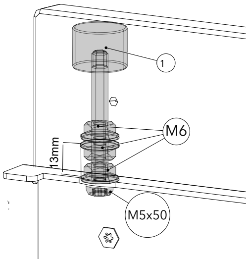
Fig. 19: Distanza a 13 mm
