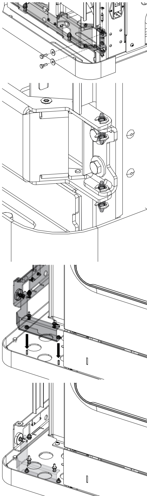
Abb. 32: Tragarme montieren
