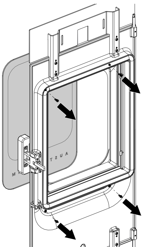
Abb. 103: Dekoglas abnehmen
