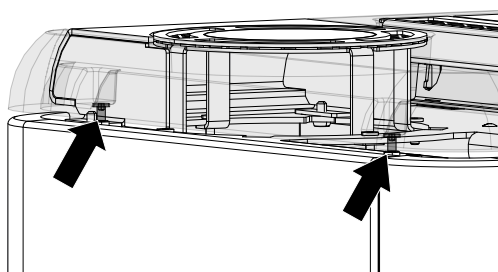
Abb. 40: Deckel einstellen
