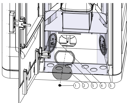
Abb. 93: Revisionsrönde herausnehmen
