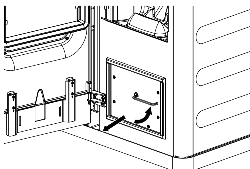
Abb. 92: Aschebox herausnehmen
