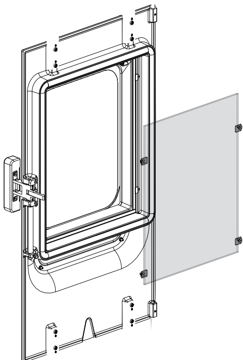
Abb. 102: Türglas abnehmen
