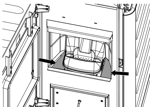
Abb. 91: Feuerraum reinigen
