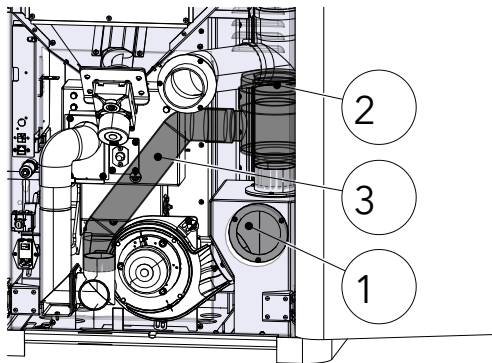
Abb. 14: Poujoulat montieren
