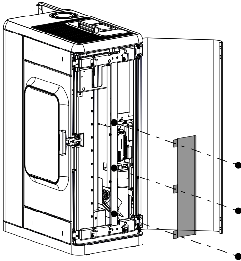
Abb. 19: Abdeckung abmontieren
