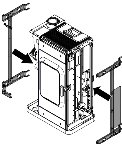
Abb. 31: Tragarme an Pelletofen anbringen
