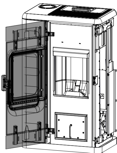
Abb. 81: Tür öffnen
