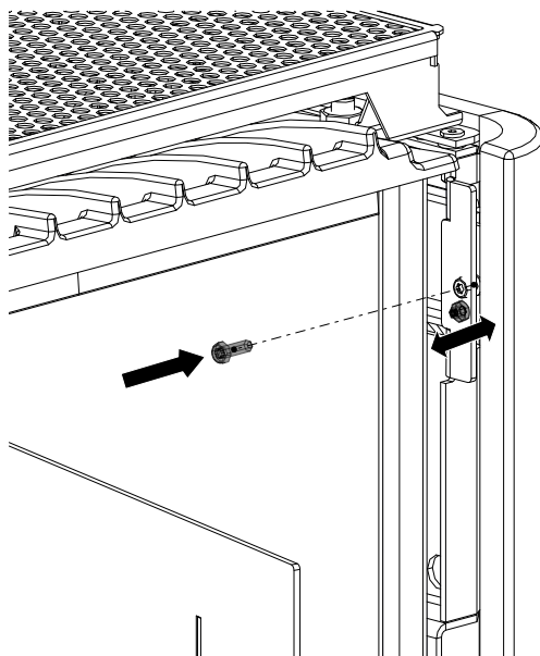
Abb. 37: Keramikverkleidung befestigen
