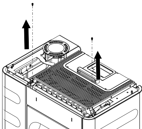
Abb. 87: Schrauben lösen
