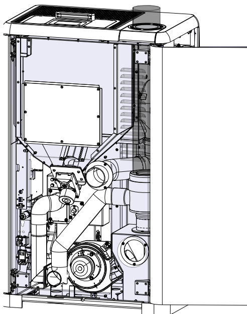
Abb. 15: Abgasrohr anschließen
