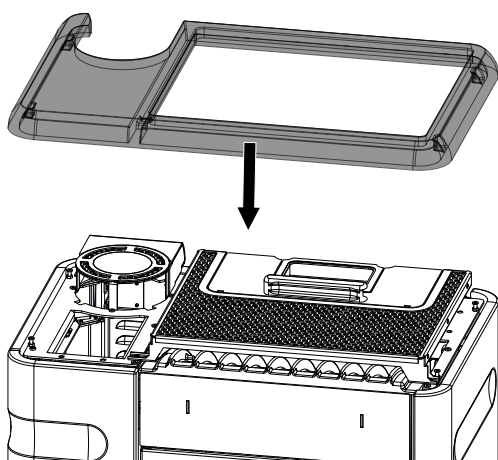
Abb. 39: Deckel anbringen
