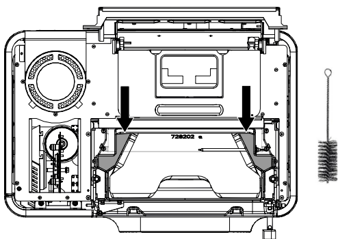
Abb. 90: Hohlraum reinigen
