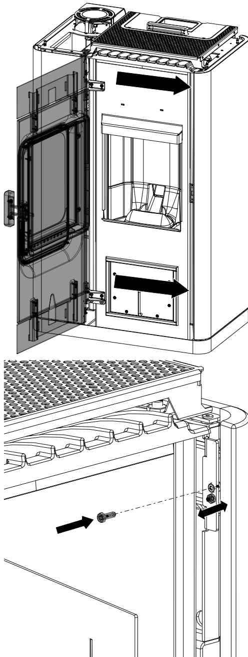
Abb. 42: Stahlverkleidung befestigen
