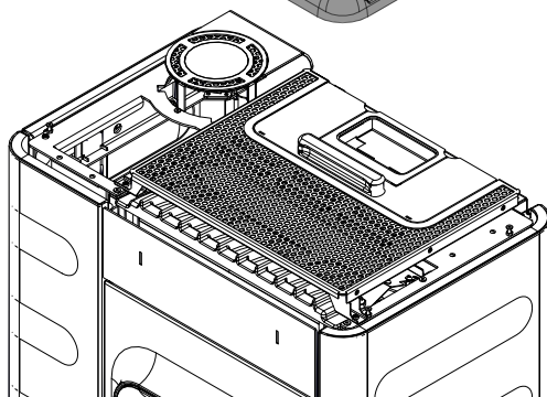
Abb. 10: Deckel abnehmen
