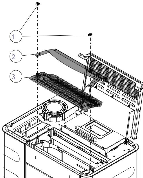
Abb. 89: Strahlungsblech und Gussdeckel abnehmen
