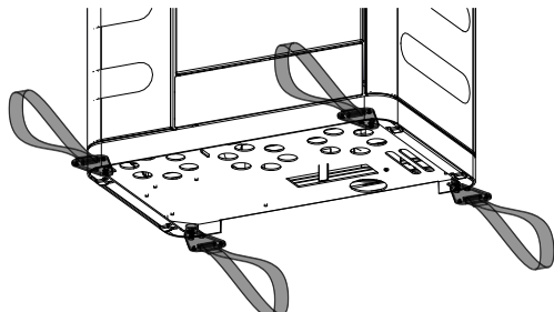
Abb. 6: Transporthilfe
