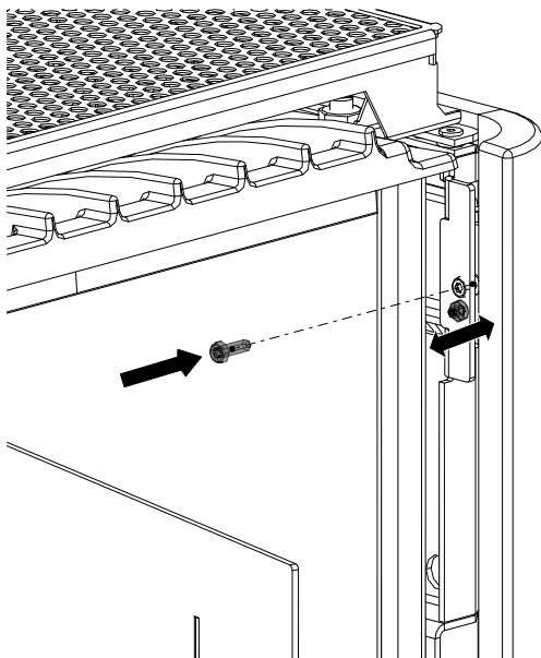
Abb. 12: Keramikverkleidung befestigen
