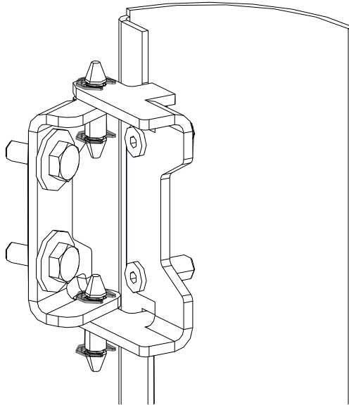
Abb. 41: Stahlverkleidung am Pelletofen montieren
