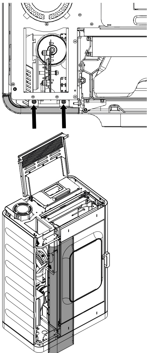
Abb. 94: Vordere Verkleidung abnehmen
