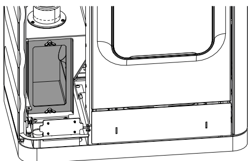
Abb. 95: Putzdeckel entfernen
