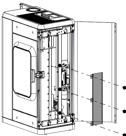
Abb. 83: Abdeckung abmontieren
