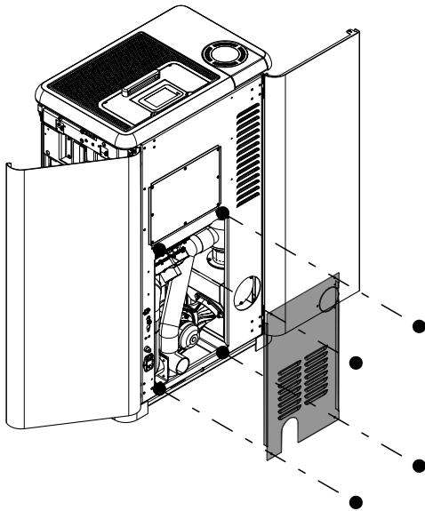
Abb. 13: Rückwand abmontieren
