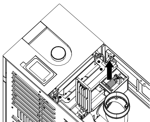
Fig. 97: Extraire la tôle de cloison
