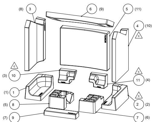
Fig. 23: Installer la Keramott
