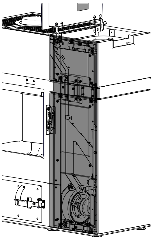
Fig. 12: Accrocher et fixer l'habillage avant
