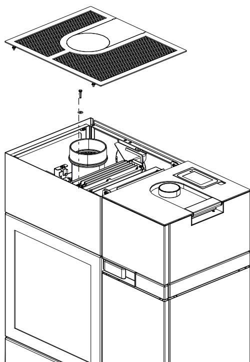
Fig. 25: Enlever le couvercle
