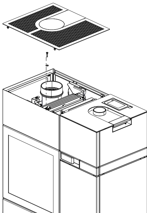
Fig. 99: Poser le couvercle
