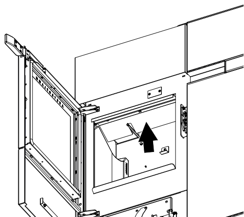
Fig. 96: Nettoyer la plaque déflectrice
