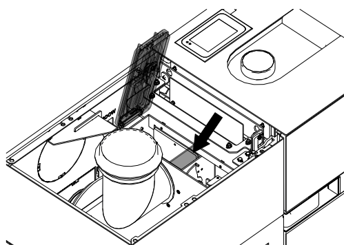
Fig. 89: Enlever l'extension de la trappe de visite
