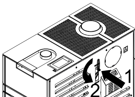
Fig. 41: Fermer le clapet de fumées
