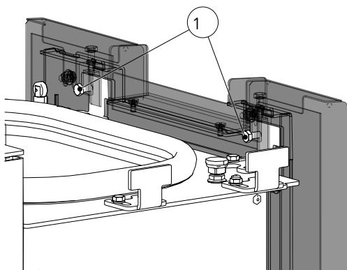
Fig. 106: Dévisser les vis et décrocher l'habillage latéral en haut
