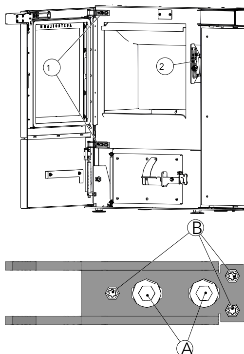
Fig. 80: Ajuster la porte du foyer
