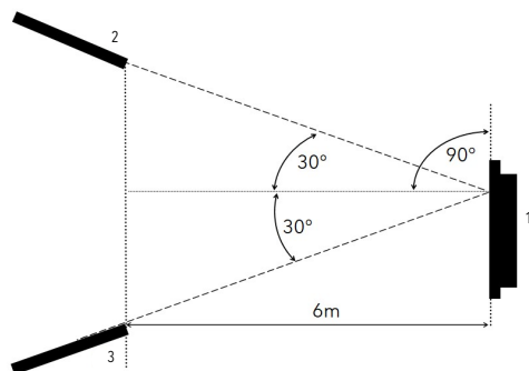
Fig. 49: Angle de fonctionnement
