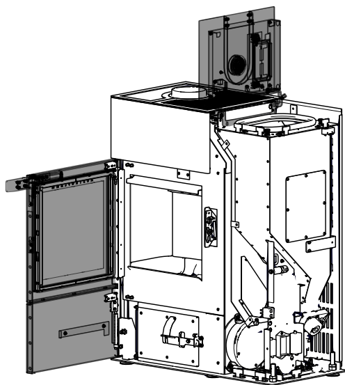
Fig. 9: Ouvrir le couvercle du réservoir et la porte du foyer
