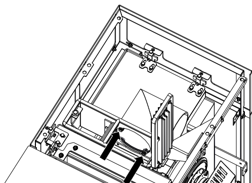
Fig. 29: Visser le conduit de fumée
