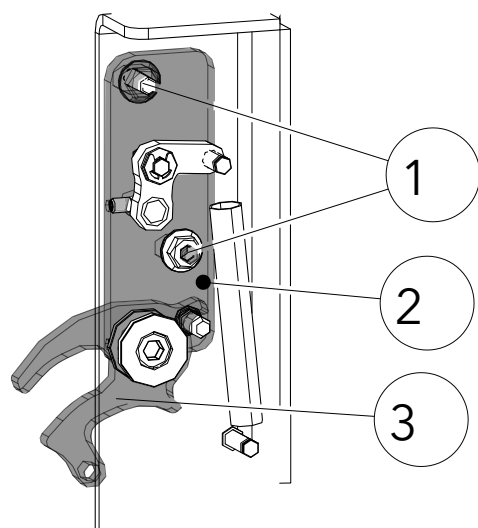
Fig. 81: Régler la force de fermeture de la porte
