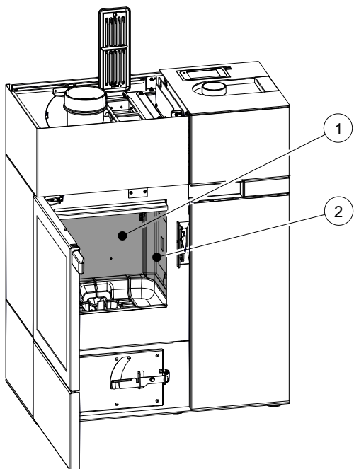
Fig. 92: Enlever la Keramott
