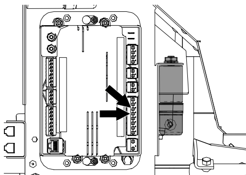
Fig. 18: Brancher le kit canalisation
