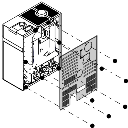
Fig. 104: Déposer le panneau arrière
