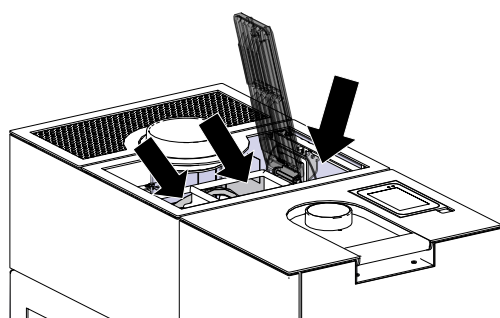
Fig. 26: Ouvrir la trappe de visite et nettoyer
