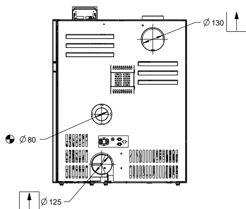
Fig. 33: Raccordement de l'alimentation en air de combustion
