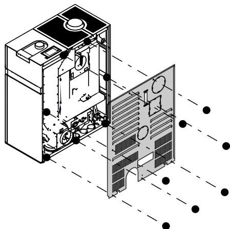
Fig. 24: Déposer le panneau arrière
