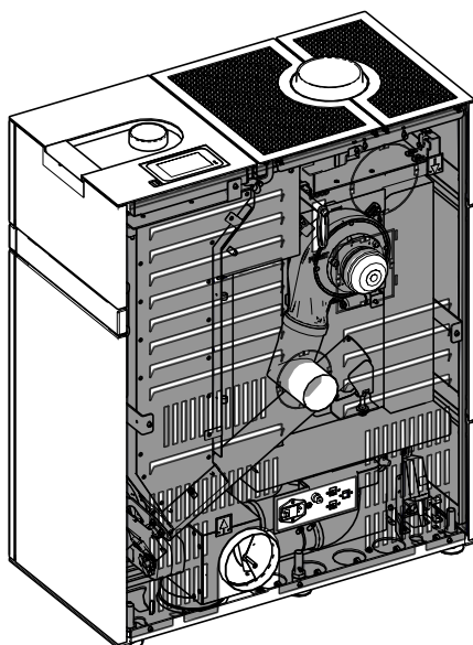
Fig. 21: Fixer le panneau arrière et l'habillage
