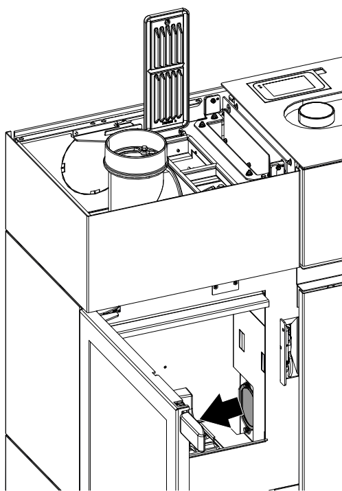
Fig. 95: Ouvrir la trappe de visite du bas
