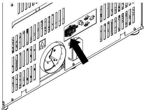
Fig. 103: Cartouche fusible avec fusibles à tube de verre T2,5 A
