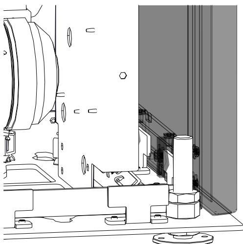
Fig. 107: Décrocher l'habillage latéral en bas
