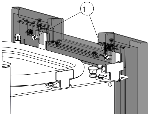
Fig. 11: Accrocher et fixer l'habillage latéral en haut
