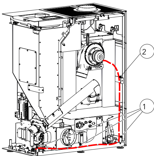
Fig. 16: Poser le câble et fixer le condensateur
