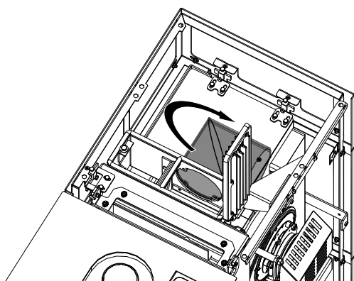
Fig. 28: Tourner le conduit de fumée
