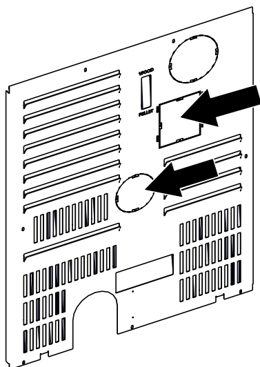
Fig. 20: Enlever les découpes perforées
