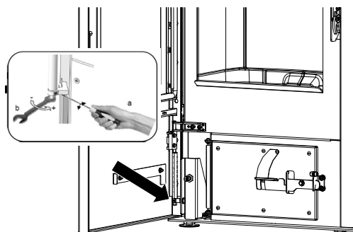
Fig. 76: Ajuster le ressort de tension
