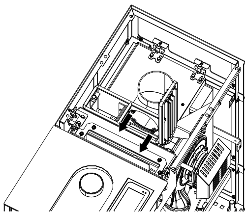
Fig. 27: Dévisser les vis du conduit de fumées
