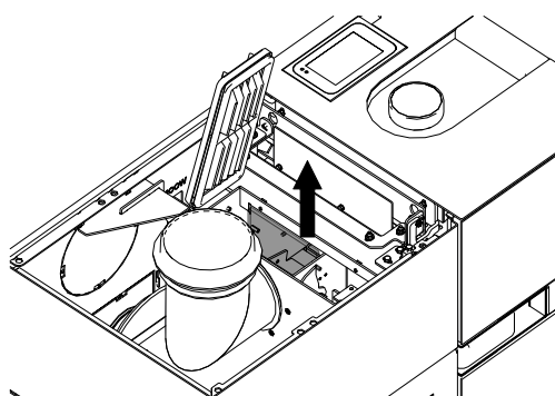
Fig. 90: Enlever la tôle de cloison
