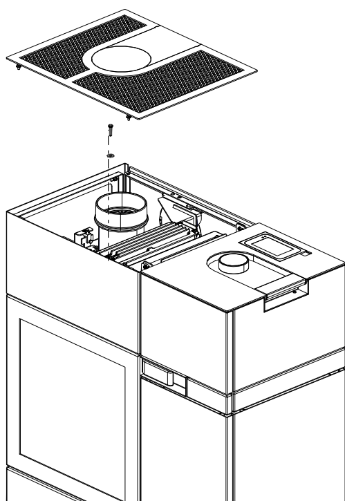
Fig. 88: Enlever le couvercle
