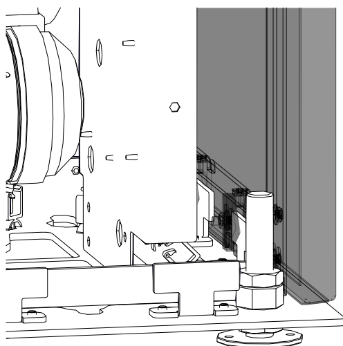
Fig. 10: Accrocher l'habillage latéral en bas
