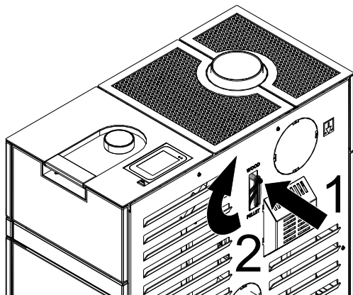
Fig. 45: Ouvrir le clapet de fumées
