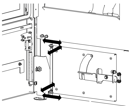
Fig. 78: Ajuster la porte du tiroir à cendres
