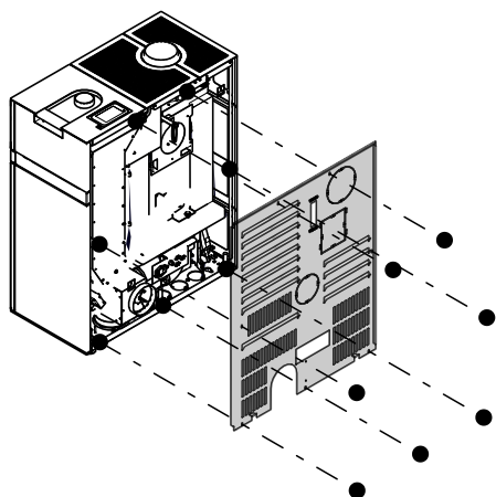
Fig. 32: Installer le panneau arrière
