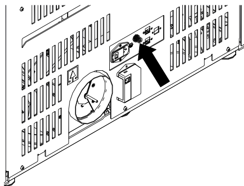
Fig. 102: Limiteur de température de sécurité
