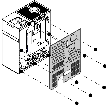
Abb. 105: Rückwand demontieren
