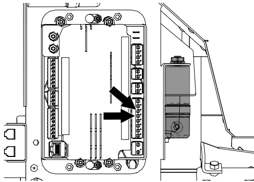
Abb. 19: Luftverteilermodul anstecken
