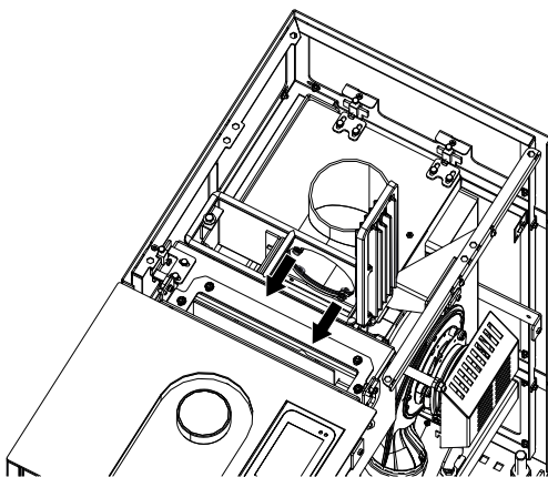
Abb. 28: Schrauben Rauchrohr lösen
