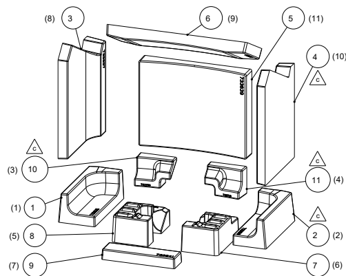
Abb. 24: Keramott montieren
