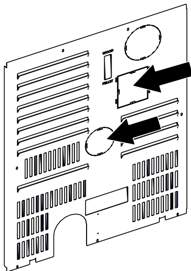
Abb. 21: Perforierte Ausschnitte entfernen
