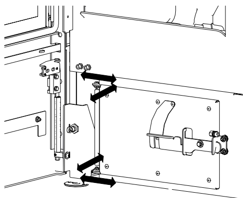
Abb. 79: Ascheladentür einstellen
