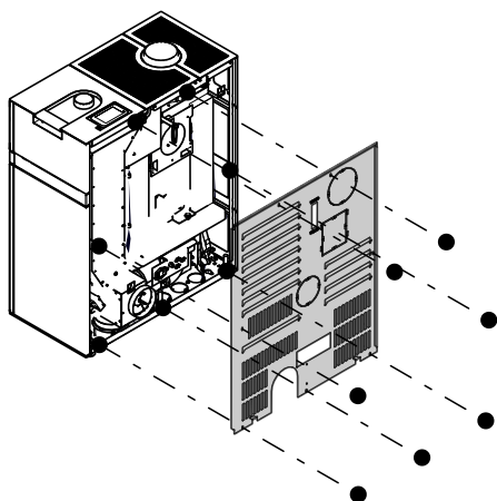
Abb. 33: Rückwand montieren
