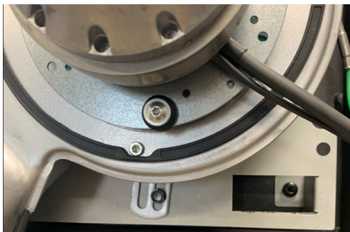
Abb. 15: LVM montieren
