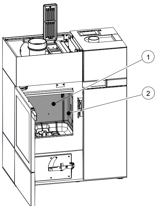
Abb. 93: Keramik entfernen
