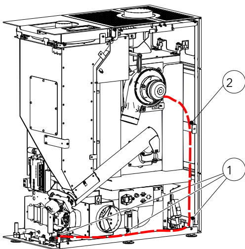
Abb. 17: Kabel verlegen und Kondensator befestigen
