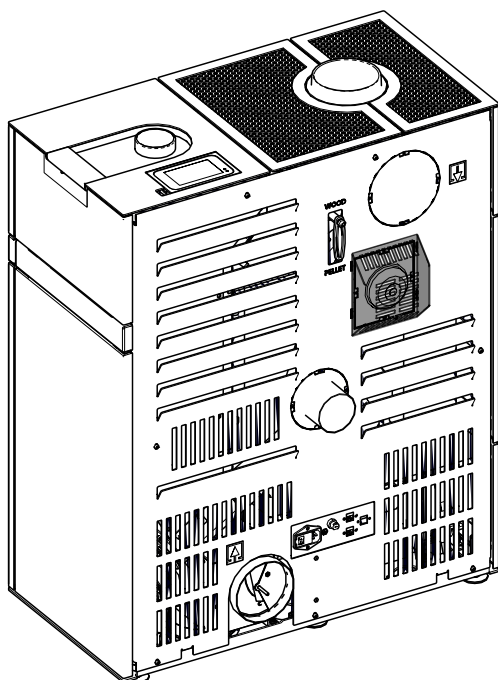
Abb. 23: Abdeckungen anbringen
