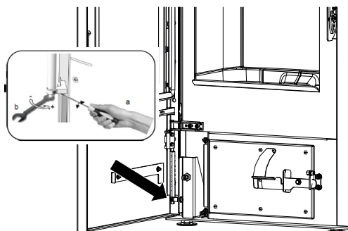
Abb. 77: Spannfeder einstellen
