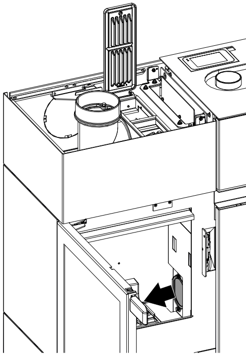
Abb. 96: Putzdeckel unten öffnen
