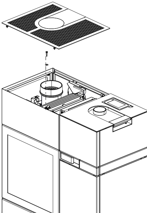
Abb. 89: Deckel abnehmen
