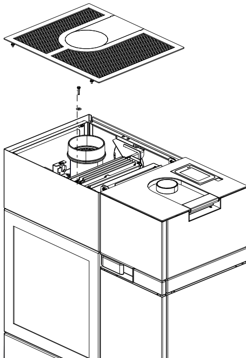
Abb. 31: Deckel anbringen
