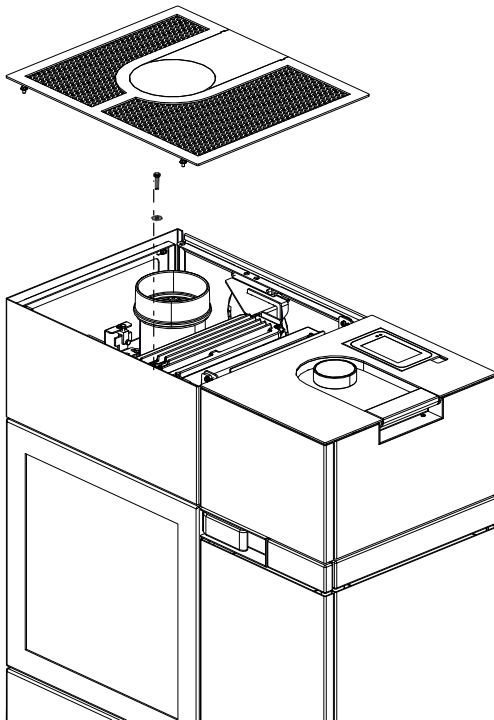
Abb. 26: Deckel abnehmen
