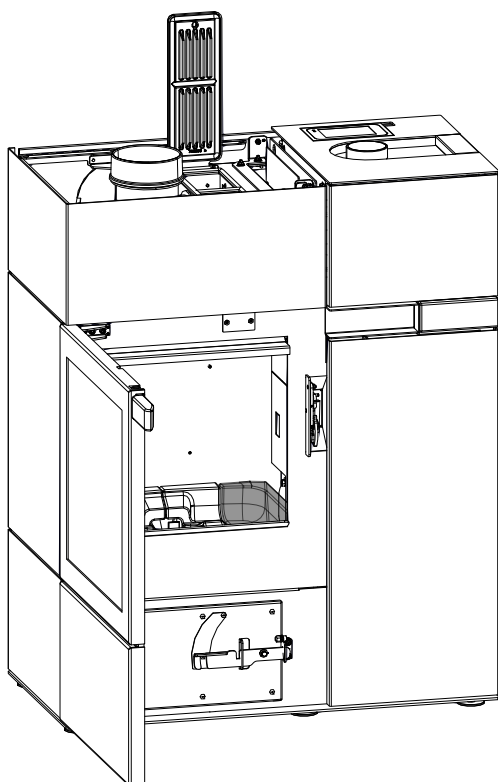
Abb. 95: Keramott entfernen
