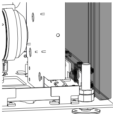
Abb. 11: Seitliche Verkleidung unten einhängen
