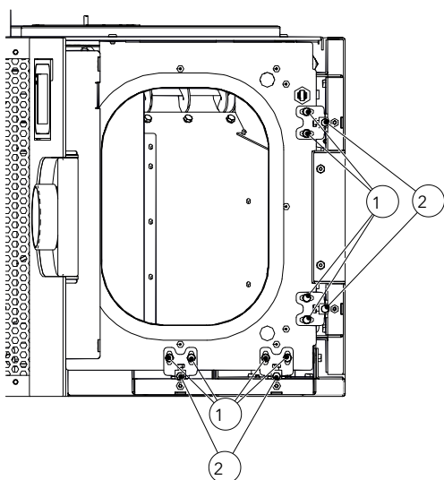
Abb. 14: Verkleidung einstellen
