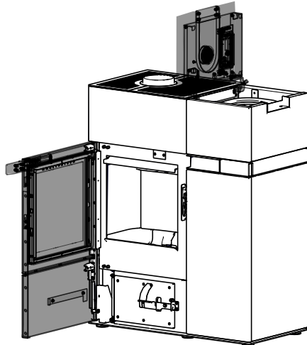
Abb. 106: Tankdeckel und Feuerraumtür öffnen
