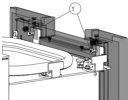
Abb. 12: Seitliche Verkleidung oben einhängen und befestigen
