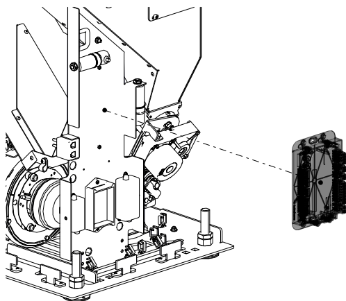
Abb. 83: Speicherbatterie tauschen
