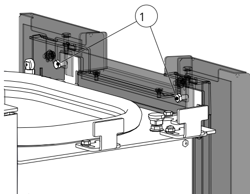
Abb. 107: Seitliche Verkleidung oben, Schrauben lösen und aushängen
