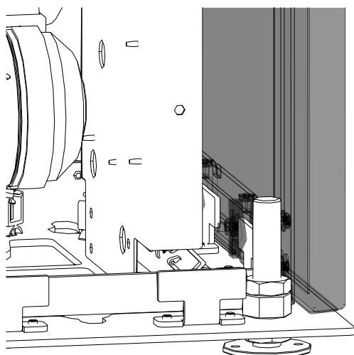
Abb. 108: Seitliche Verkleidung unten aushängen
