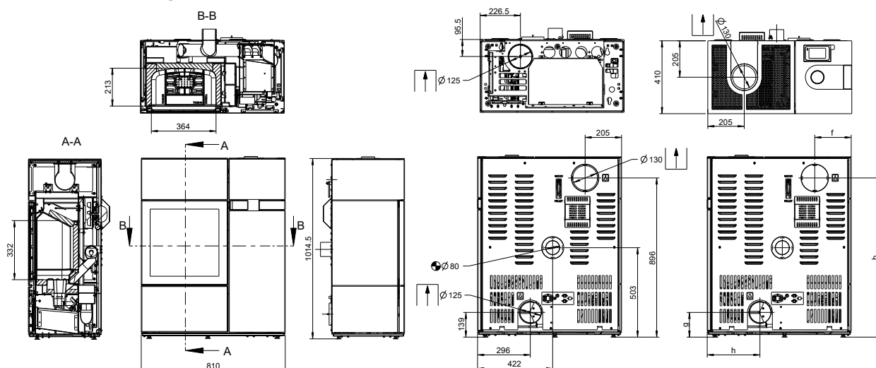
Abb. 2: Abmessungen
