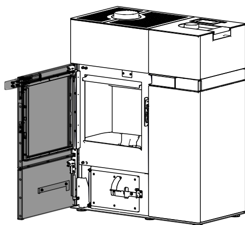
Abb. 80: Feuerraumtür öffnen
