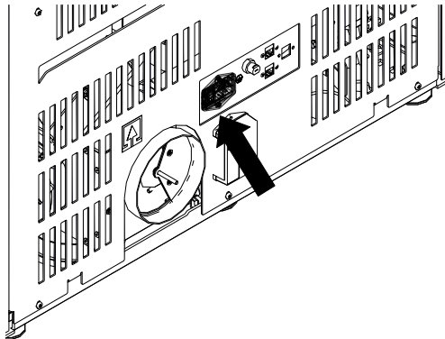
Abb. 104: Sicherungseinschub mit T2,5A-Glasrohrsicherungen
