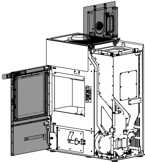
Abb. 10: Tankdeckel und Feuerraumtür öffnen
