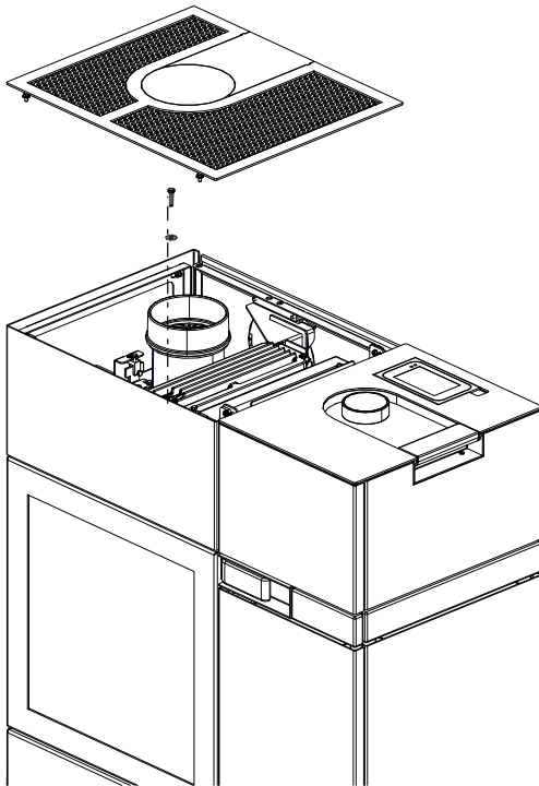
Abb. 100: Deckel anbringen
