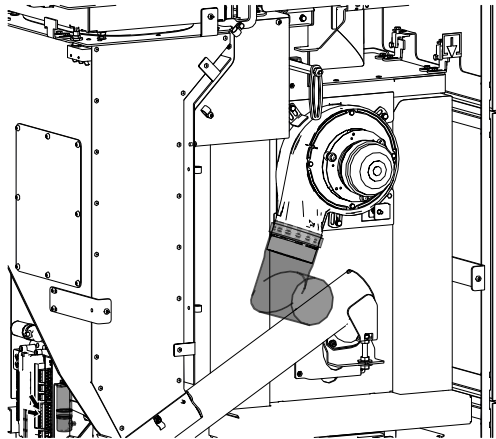
Abb. 20: Rohr aufstecken
