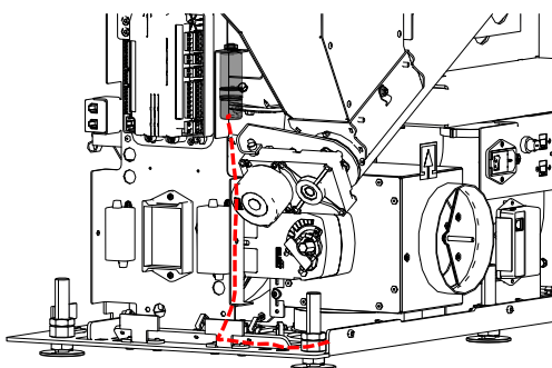
Abb. 18: Kondensator befestigen
