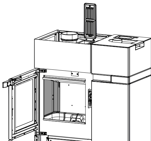
Abb. 94: Keramott entfernen
