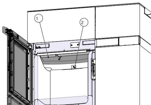
Abb. 92: Zugplatte anheben
