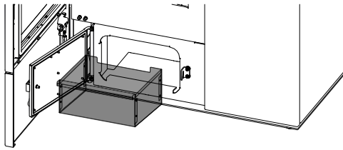
Abb. 86: Aschelade entnehmen
