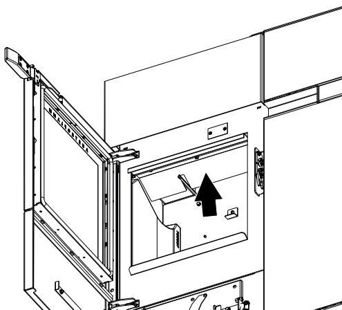
Abb. 97: Umlenblech reinigen
