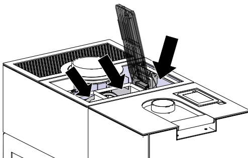
Abb. 27: Putzdeckel öffnen und reinigen
