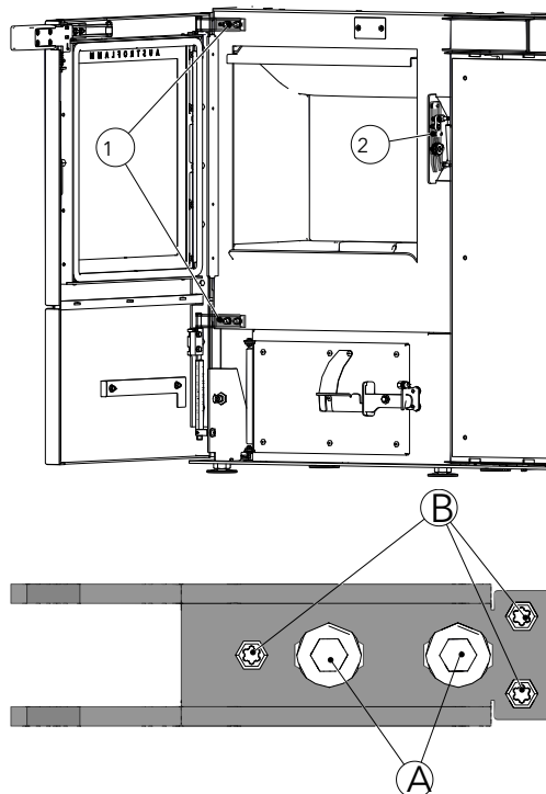
Abb. 81: Feuerraumtür einstellen
