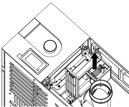
Abb. 98: Schottblech rausziehen
