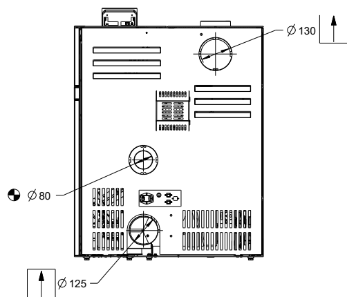
Abb. 34: Anschluss Verbrennungsluftzufuhr
