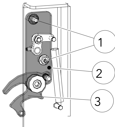
Abb. 82: Türschließkraft einstellen
