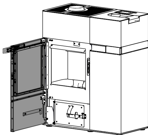
Abb. 78: Feuerraumtür öffnen
