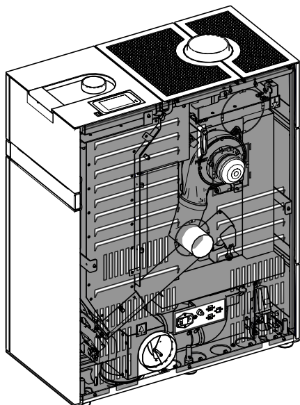
Abb. 22: Rückwand und Verkleidung befestigen
