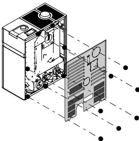
Abb. 25: Rückwand demontieren
