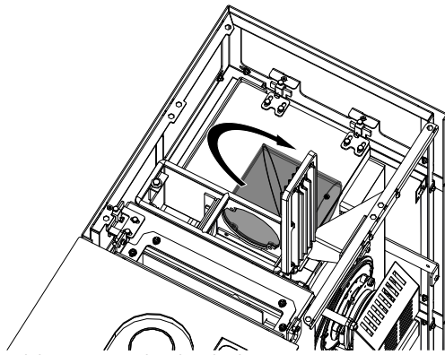
Abb. 29: Rauchrohr drehen
