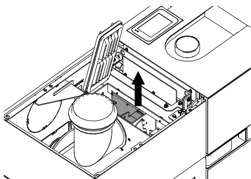
Abb. 91: Schottwand-Blech entfernen
