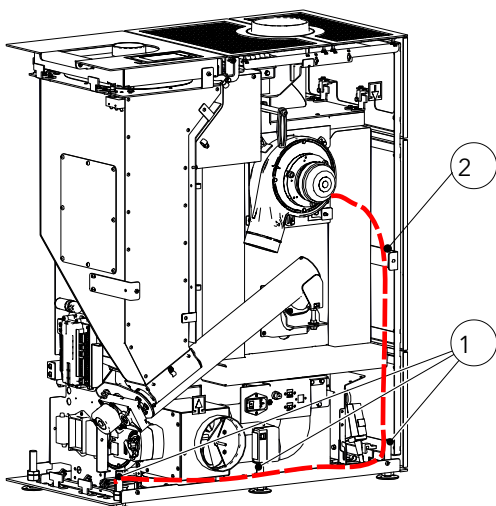
Abb. 18: Kabel verlegen und Kondensator befestigen
