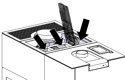
Abb. 28: Putzdeckel öffnen und reinigen
