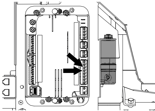
Abb. 20: Luftverteilermodul anstecken
