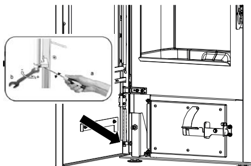
Abb. 78: Spannfeder einstellen
