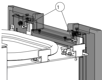
Abb. 13: Seitliche Verkleidung oben einhängen und befestigen
