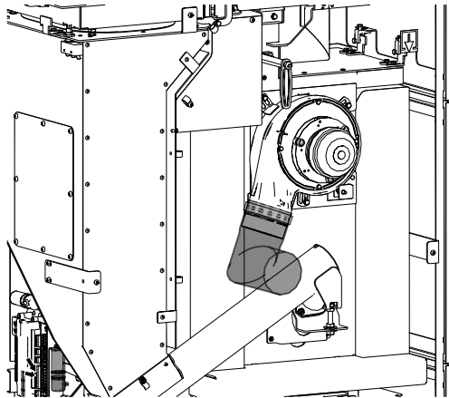
Abb. 21: Rohr aufstecken
