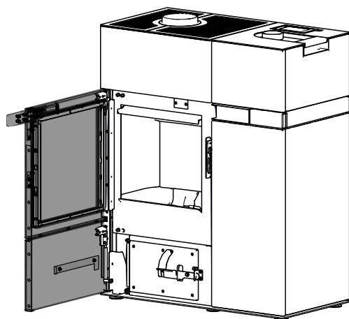
Abb. 79: Feuerraumtür öffnen
