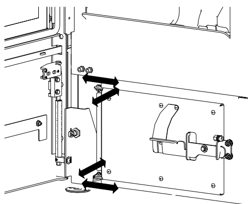
Abb. 80: Ascheladentür einstellen
