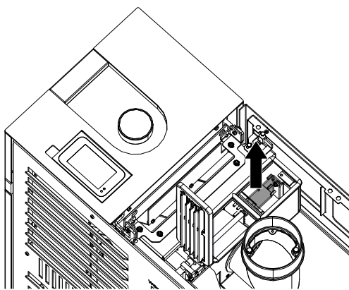
Abb. 99: Schottblech rausziehen
