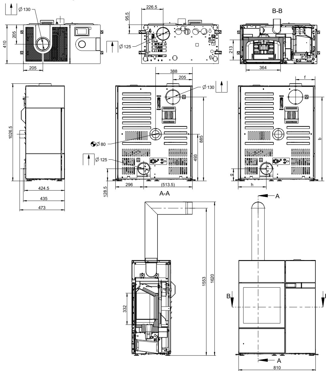
Abb. 2: Abmessungen
