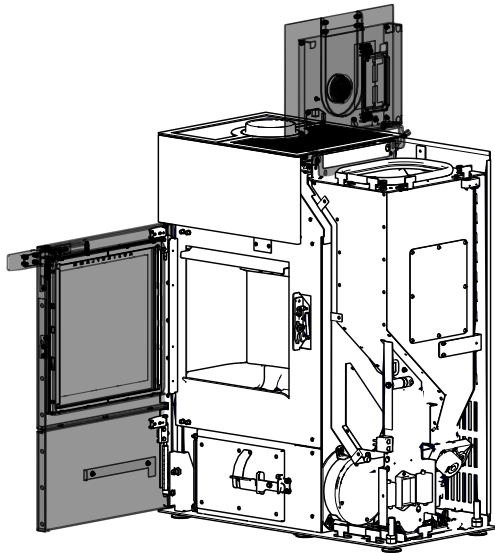
Abb. 11: Tankdeckel und Feuerraumtür öffnen
