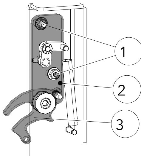
Abb. 83: Türschließkraft einstellen
