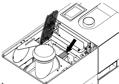
Abb. 91: Putzdeckelerweiterung weg
