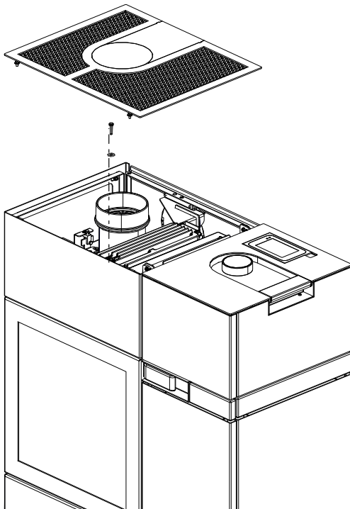
Abb. 90: Deckel abnehmen
