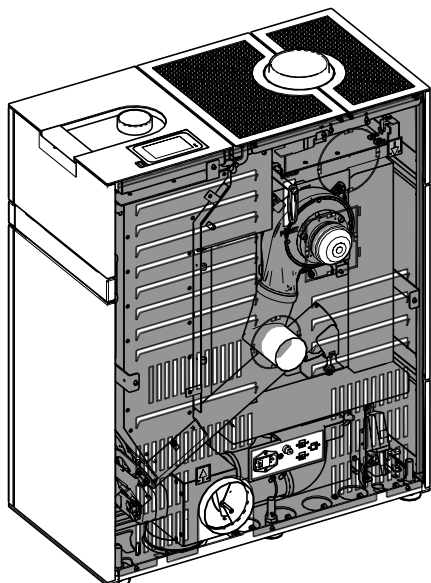
Abb. 23: Rückwand und Verkleidung befestigen
