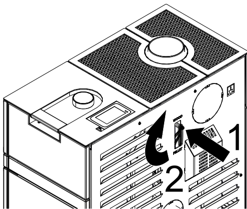
Abb. 47: Rauchgasklappe öffnen
