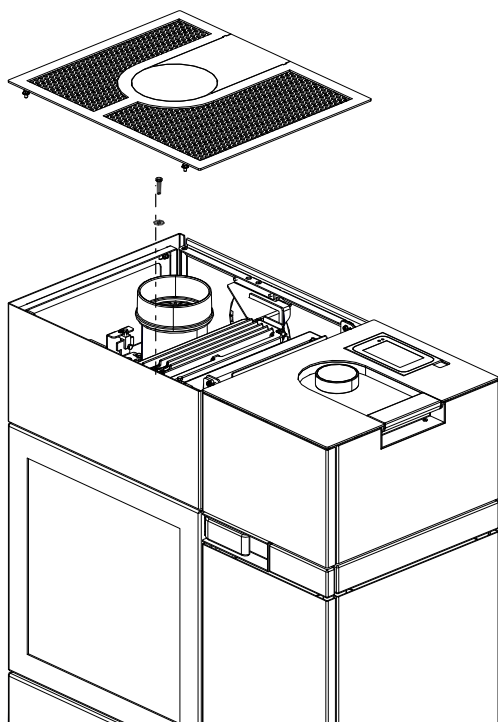
Abb. 101: Deckel anbringen
