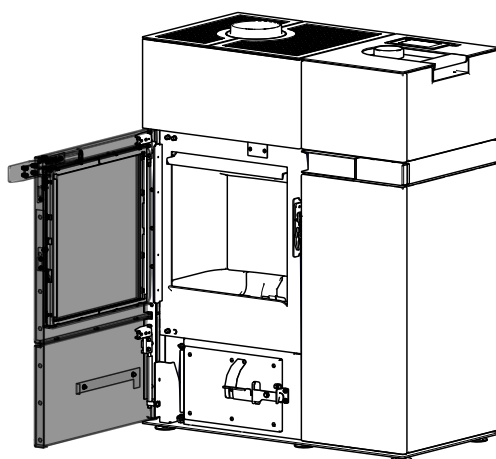
Abb. 85: Feuerraumtür öffnen
