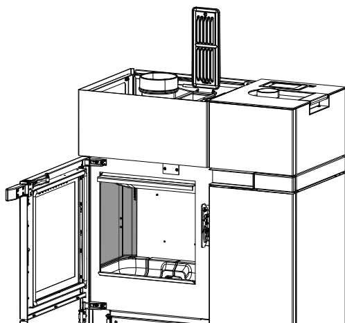
Abb. 95: Keramott entfernen
