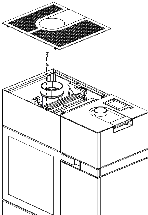
Abb. 32: Deckel anbringen
