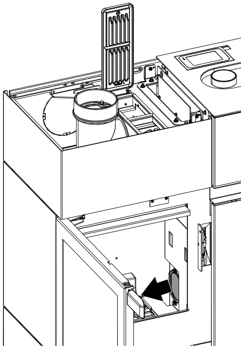
Abb. 97: Putzdeckel unten öffnen
