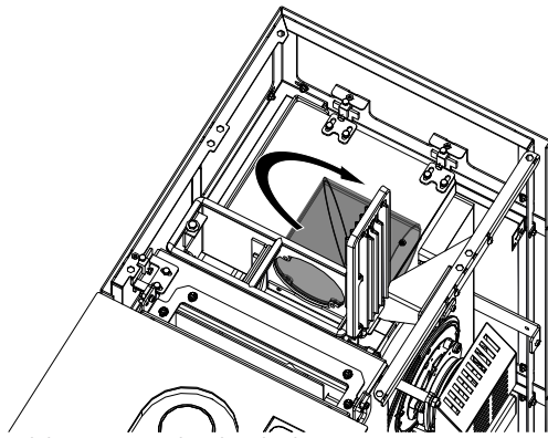
Abb. 30: Rauchrohr drehen
