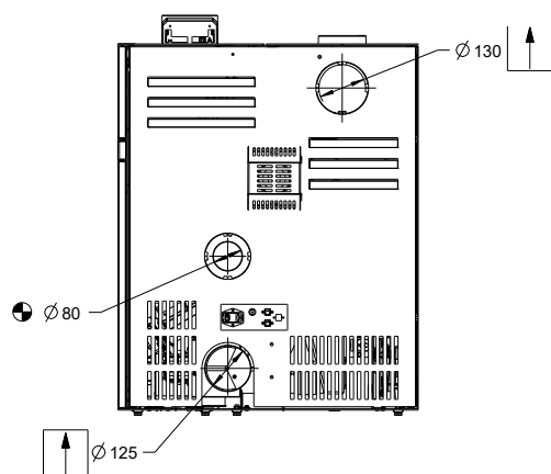
Abb. 35: Anschluss Verbrennungsluftzufuhr
