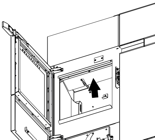
Abb. 98: Umlenblech reinigen
