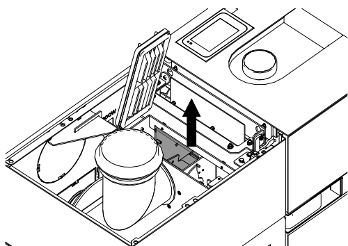
Abb. 92: Schottwand-Blech entfernen
