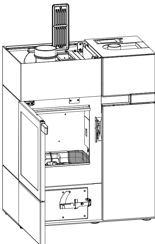
Abb. 96: Keramott entfernen
