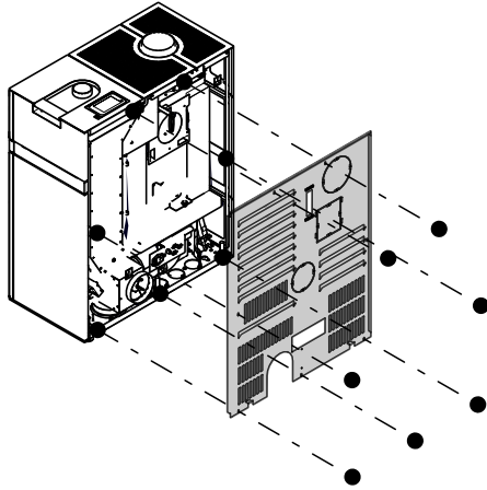
Abb. 106: Rückwand demontieren
