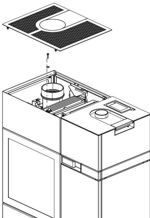
Abb. 27: Deckel abnehmen
