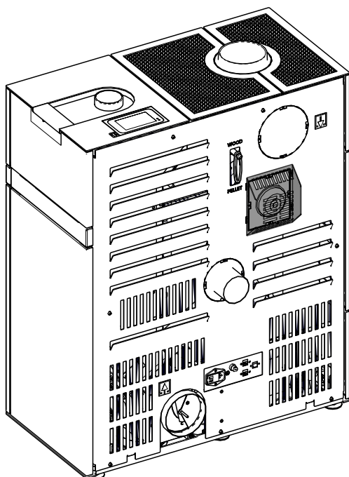
Abb. 24: Abdeckungen anbringen
