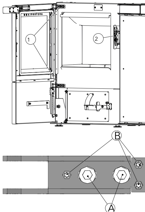
Abb. 82: Feuerraumtür einstellen
