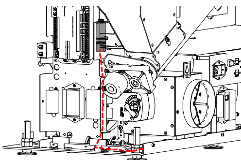
Abb. 19: Kondensator befestigen
