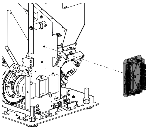
Abb. 84: Speicherbatterie tauschen
