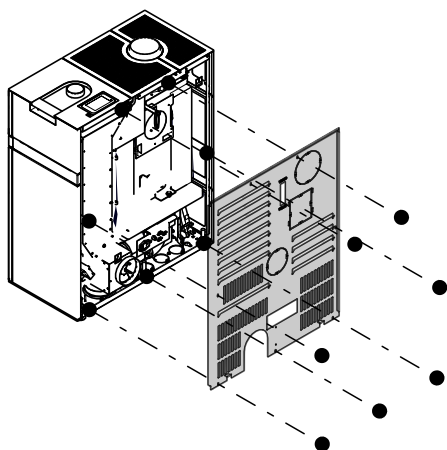
Abb. 34: Rückwand montieren
