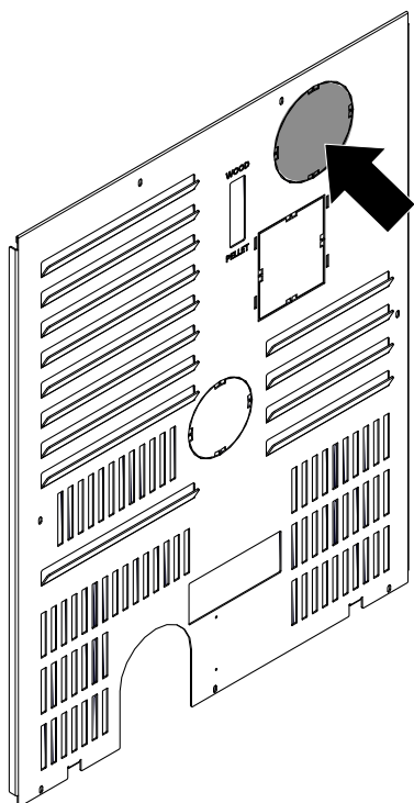
Abb. 33: Perforierten Ausschnitt entfernen
