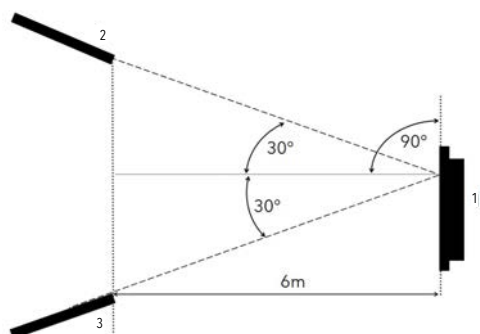
Abb. 51: Betriebswinkel
