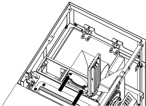
Abb. 31: Rauchrohr anschrauben
