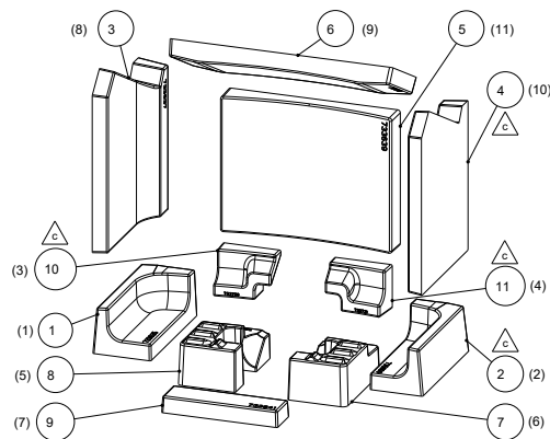
Abb. 25: Keramott montieren
