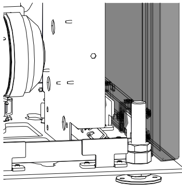
Abb. 12: Seitliche Verkleidung unten einhängen
