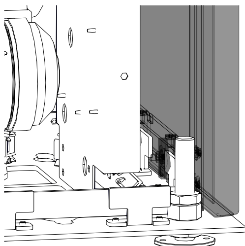
Abb. 109: Seitliche Verkleidung unten aushängen
