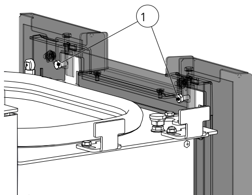
Abb. 108: Seitliche Verkleidung oben, Schrauben lösen und aushängen
