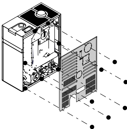
Abb. 26: Rückwand demontieren
