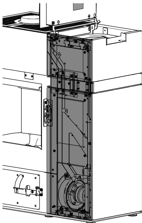
Abb. 14: Vordere Verkleidung einhängen und befestigen
