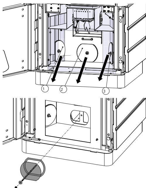
Fig. 72: Enlever les couvercles de révision
