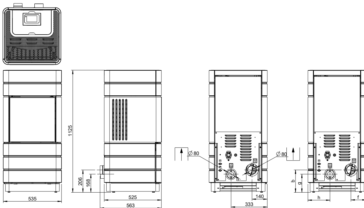
Fig. 1: Dimensions
