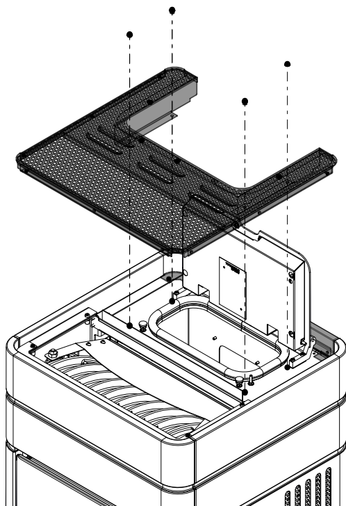
Fig. 16: Remettre le couvercle en place
