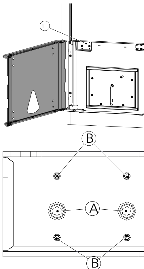
Fig. 61: Vis de réglage pour la porte
