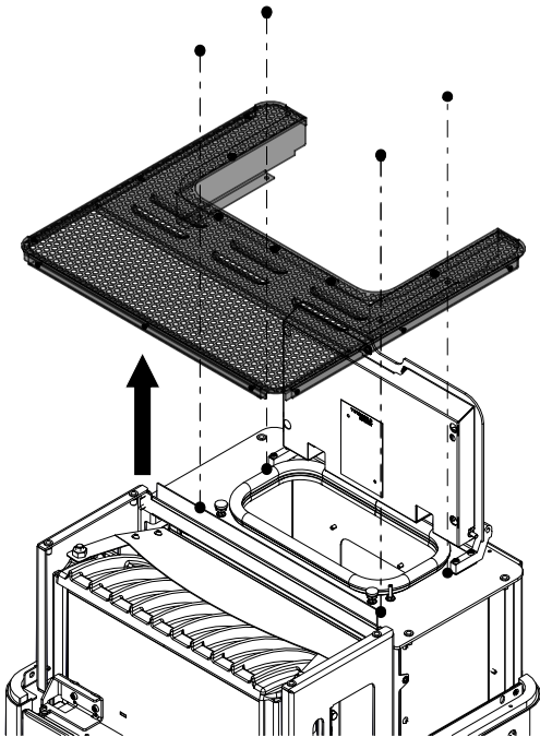
Fig. 21: Enlever le couvercle
