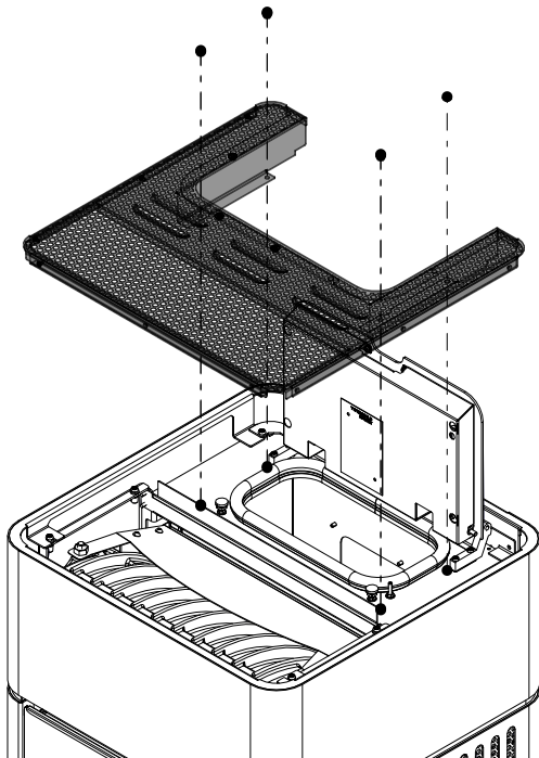
Fig. 26: Remettre le couvercle en place
