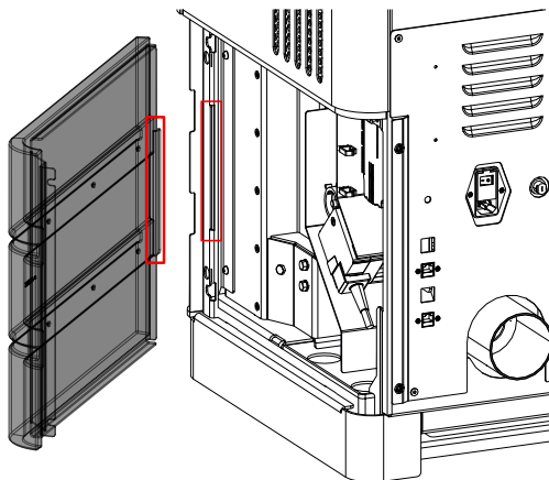
Fig. 11: Accrocher les parties latérales basses
