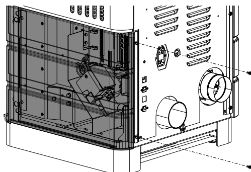
Fig. 12: Fixer les parties latérales
