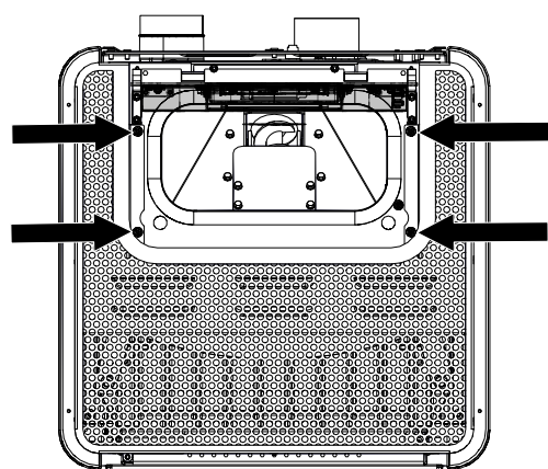
Fig. 9: Dévisser les vis
