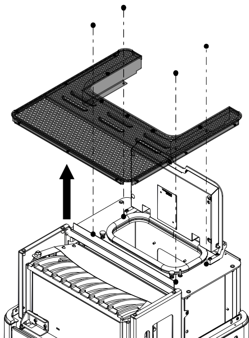
Fig. 10: Enlever le couvercle
