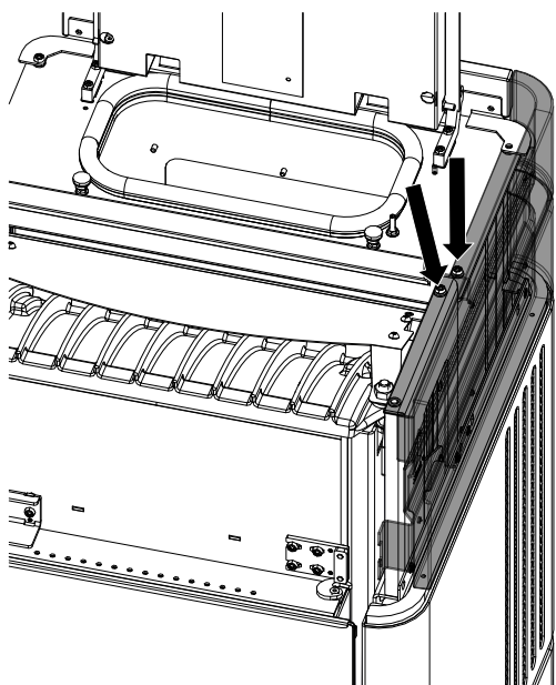
Fig. 15: Fixer les parties latérales supérieures
