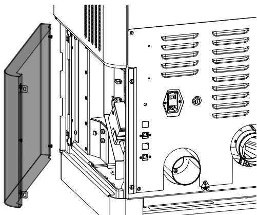
Fig. 22: Fixer les parties latérales inférieures
