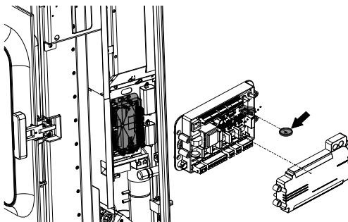
Fig. 72: Remplacer la pile mémoire
