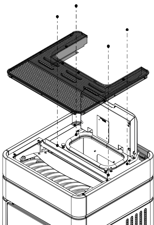
Fig. 18: Remettre le couvercle en place
