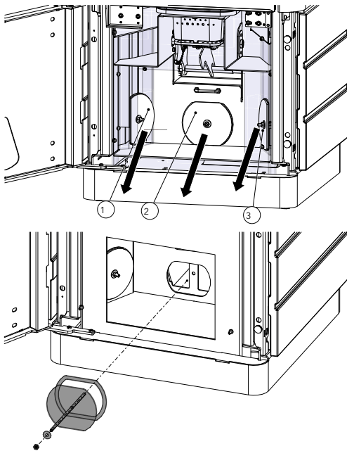
Fig. 70: Enlever les couvercles de révision
