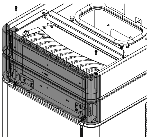
Fig. 16: Poser l'habillage en céramique supérieur avant
