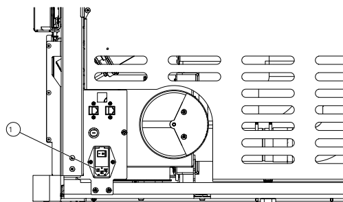
Fig. 29: Raccordement électrique
