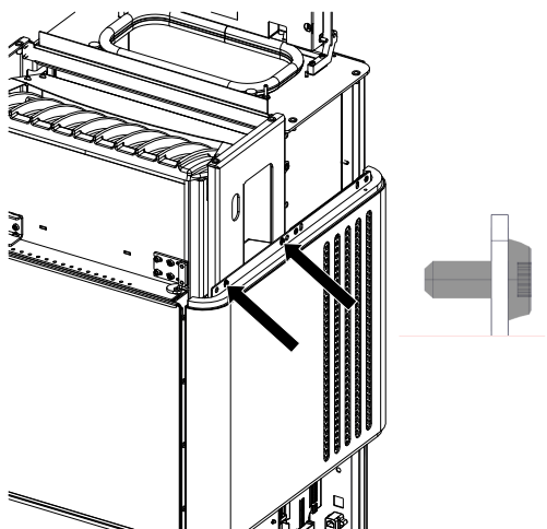
Fig. 14: Visser les vis latérales
