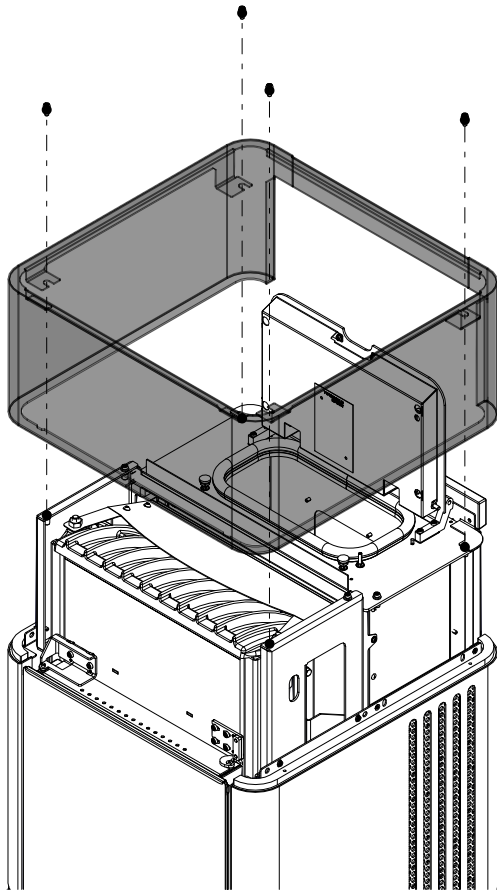
Fig. 25: Installer l'habillage en acier supérieur
