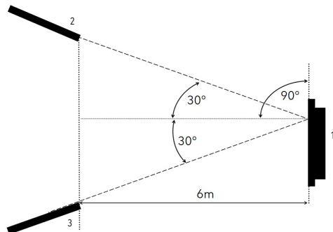
Fig. 35: Angle de fonctionnement
