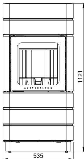
Fig. 2: Dimensions
