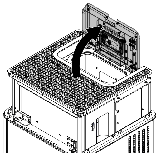
Fig. 8: Ouvrir le réservoir
