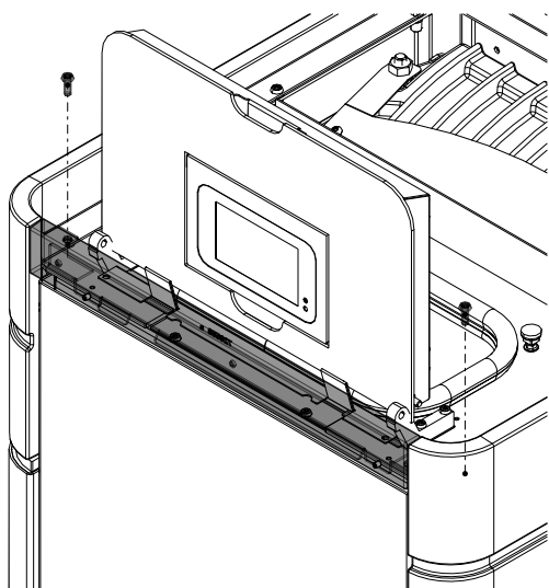
Fig. 17: Poser l'habillage en céramique supérieur arrière
