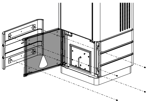
Fig. 13: Installer l'habillage en céramique avant
