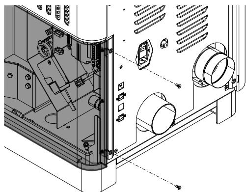
Fig. 23: Fixer les parties latérales
