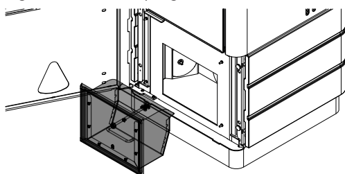
Fig. 69: Extraire le bac à cendres
