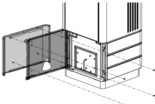
Fig. 24: Installer l'habillage en acier avant
