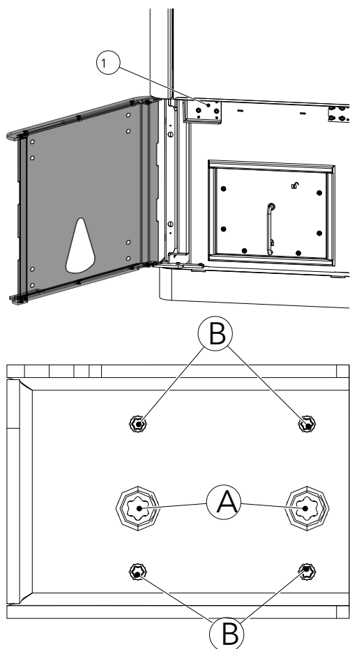
Fig. 60: Vis de réglage pour la porte
