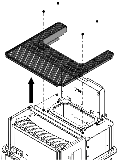
Fig. 67: Rimozione del coperchio
