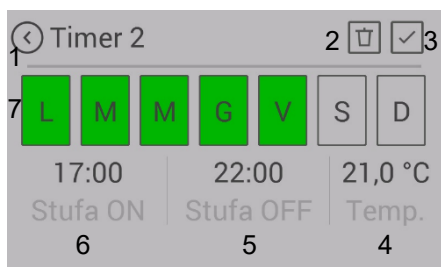
Fig. 42: Predisposizione degli orari di riscaldamento
