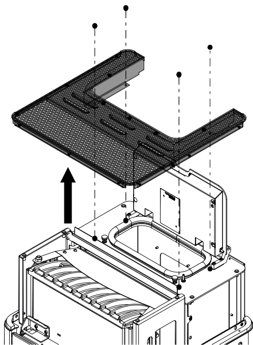
Fig. 9: Rimozione del coperchio
