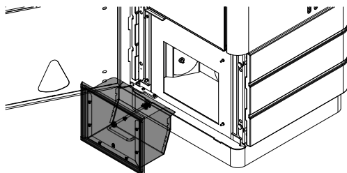
Fig. 72: Rimozione del box cenere
