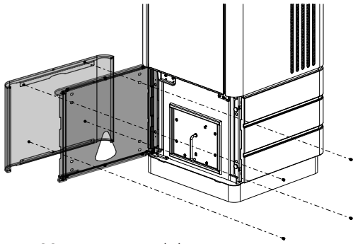
Fig. 23: Montaggio del cappotto in acciaio anteriore
