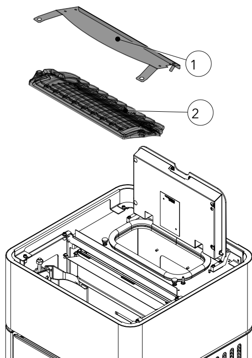
Fig. 68: Rimozione della lamiera anti-irradiazione e del coperchio in fusione
