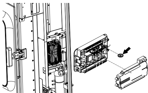
Fig. 63: Sostituzione della batteria tampone
