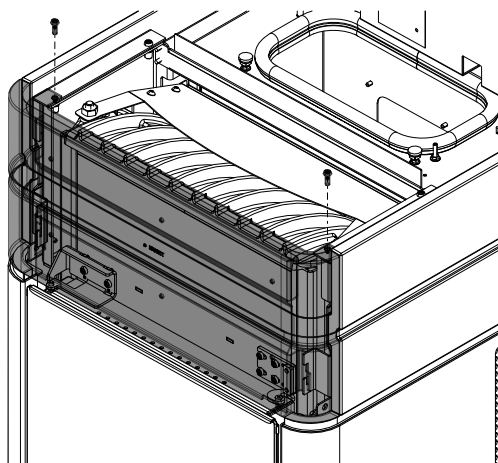
Fig. 15: Montaggio del rivestimento in ceramica superiore anteriore
