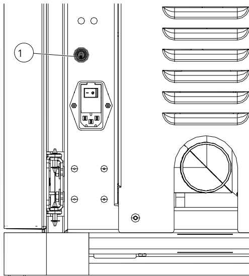
Fig. 77: Limitatore di temperatura di sicurezza
