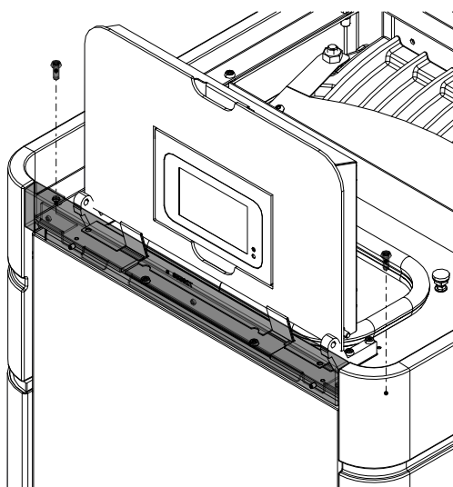
Fig. 16: Montaggio del rivestimento in ceramica superiore posteriore
