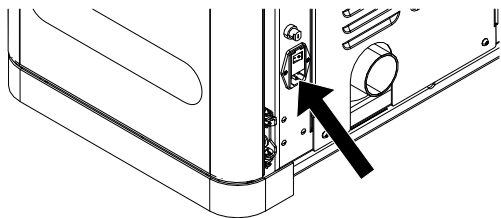
Fig. 78: Cassetto con fusibili in vetro T2,5A
