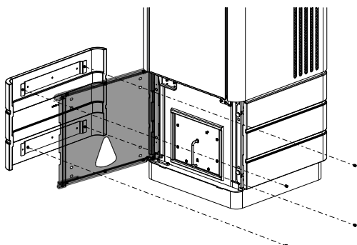
Fig. 12: Montaggio del rivestimento in ceramica anteriore
