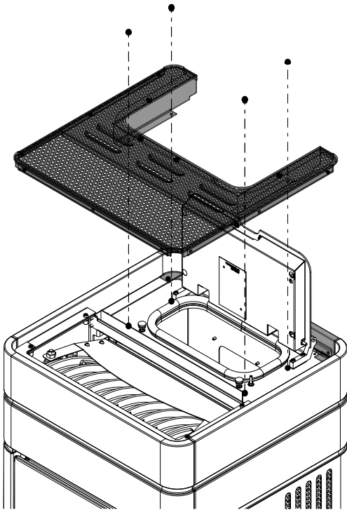
Fig. 17: Rimontaggio del coperchio
