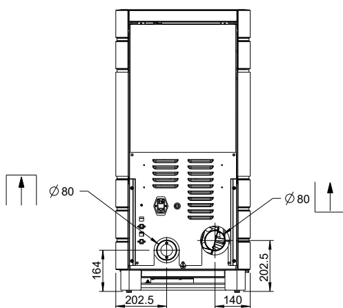
Fig. 27: Dimensioni
