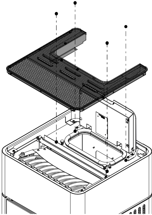
Fig. 25: Rimontaggio del coperchio
