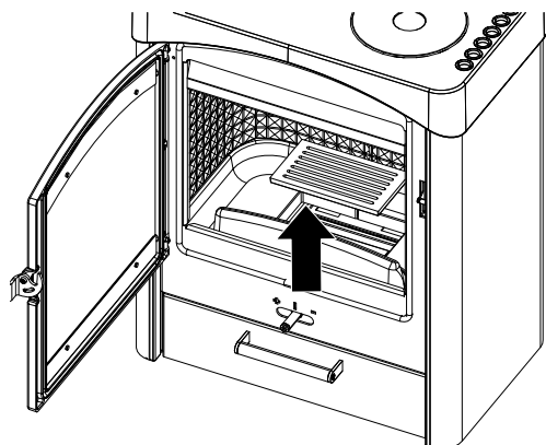
Fig. 34: Extraire la grille
