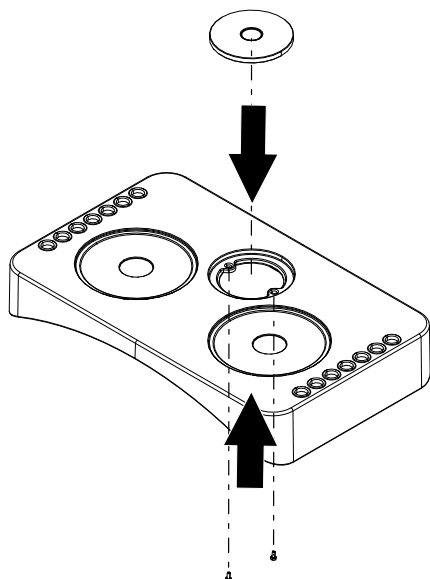
Fig. 26: Installer le recouvrement sur le couvercle
