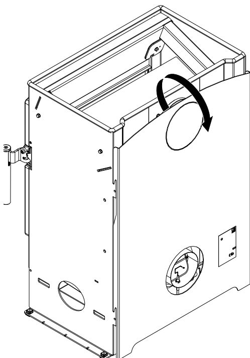
Fig. 8: Soulever la paroi arrière et l'enlever
