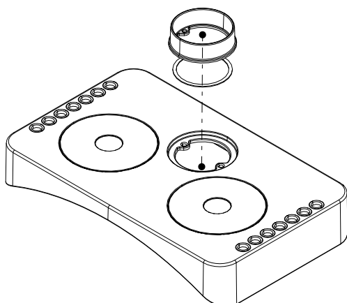
Fig. 22: Démonter tubulure et le joint du couvercle
