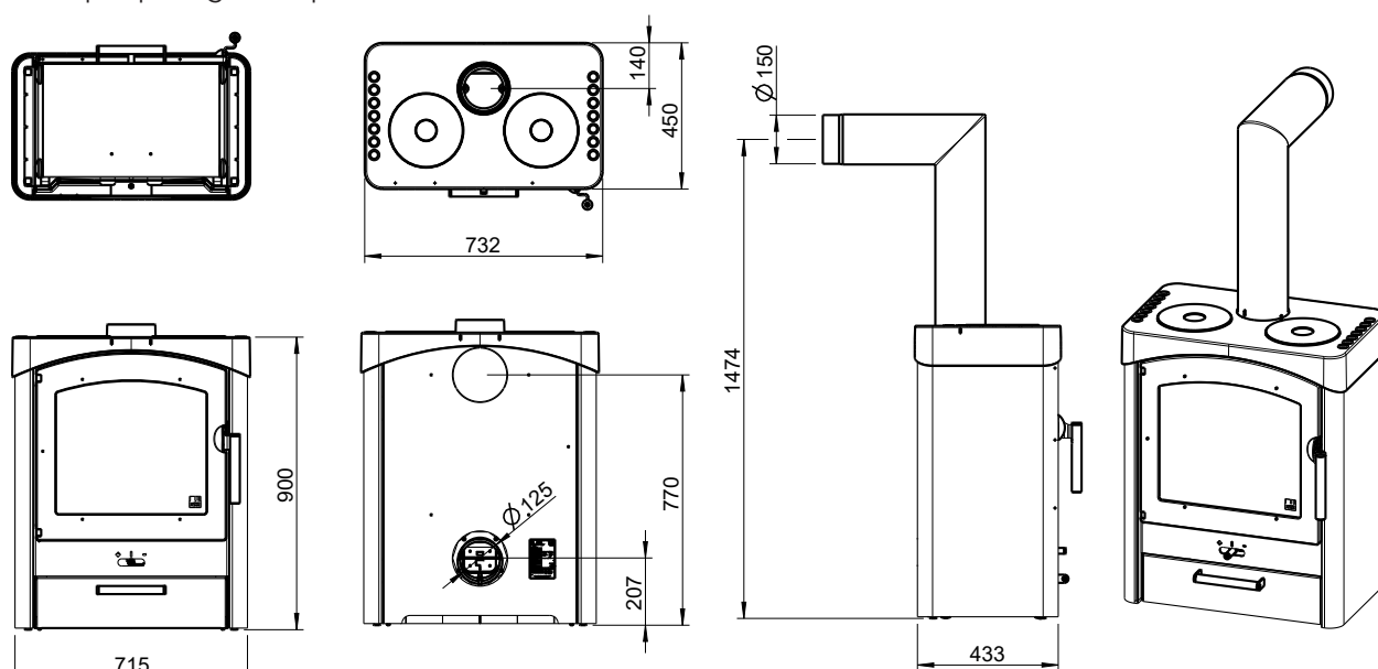
Fig. 1: Dimensions
