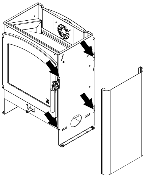
Fig. 10: Installer l'habillage latéral
