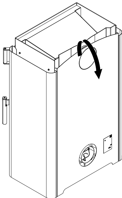
Fig. 39: Soulever la paroi arrière et l'enlever
