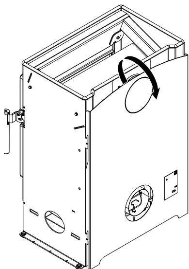
Fig. 8: Soulever la paroi arrière et l'enlever
