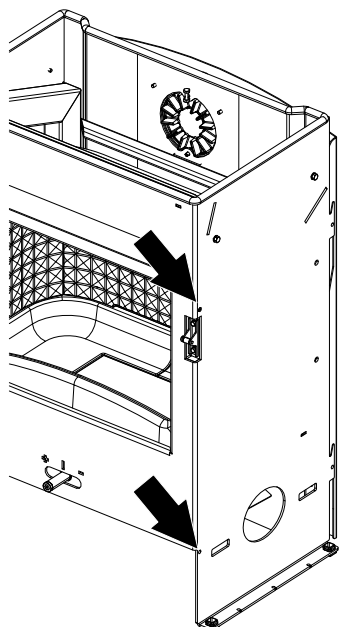
Fig. 9: Enlever les vis préinstallées
