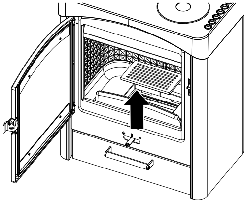
Fig. 34: Extraction de la grille
