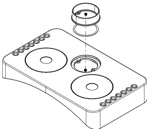
Fig. 21: Démontez tubulure et le joint du couvercle
