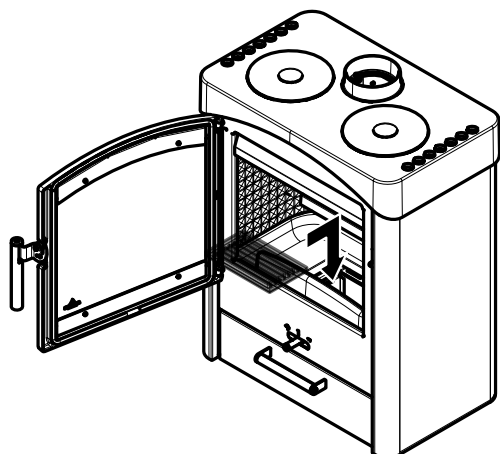
Fig. 30: Mettre la grille du bac à cendre en place
