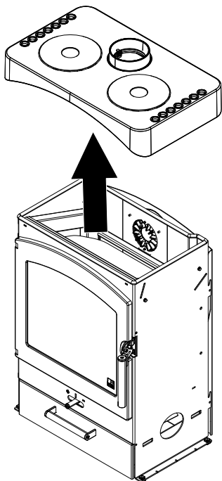
Fig. 6: Enlever le couvercle.
