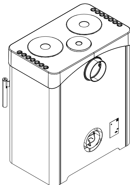
Fig. 26: Poser le couvercle
