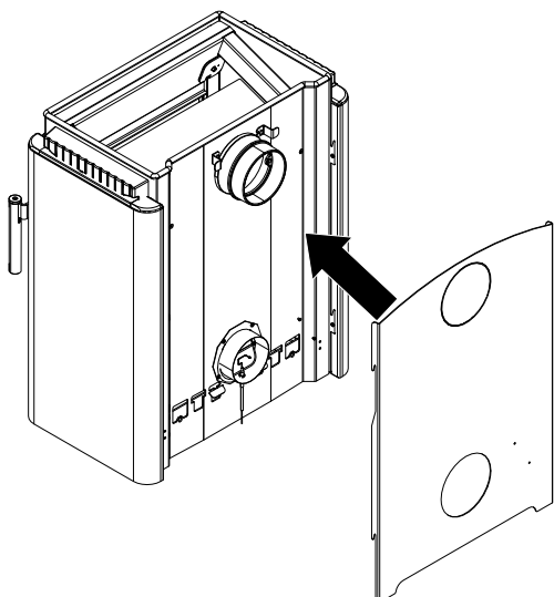
Fig. 24: Accrocher la paroi arrière
