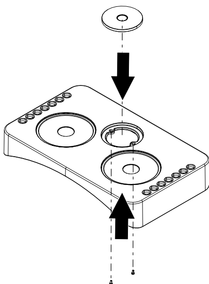
Fig. 25: Installer le recouvrement sur le couvercle
