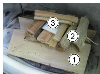
Fig. 33: Avant l'allumage
