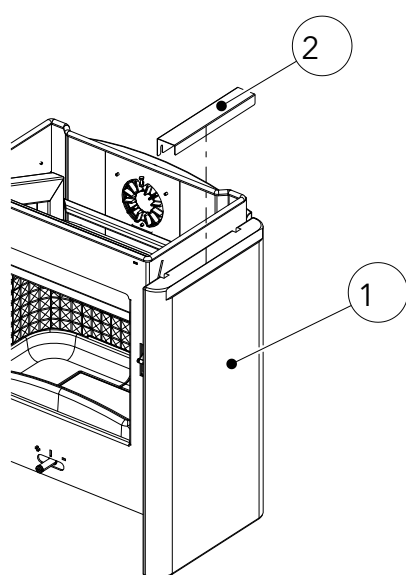
Fig. 13: Accrocher l'habillage latéral en pierre ollaire
