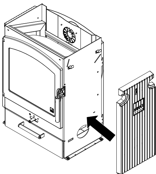
Fig. 15: Poser la pierre HMS
