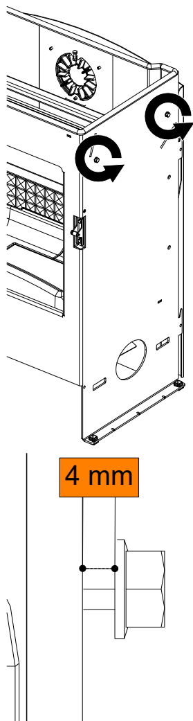
Fig. 10: Dévisser les vis
