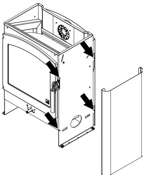
Fig. 9: Installer l'habillage latéral
