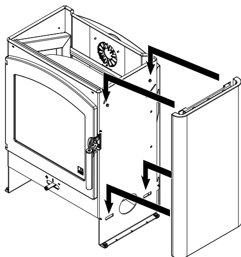
Fig. 11: Accrocher l'habillage latéral en céramique
