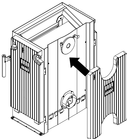
Fig. 17: Poser la pierre HMS à l'arrière
