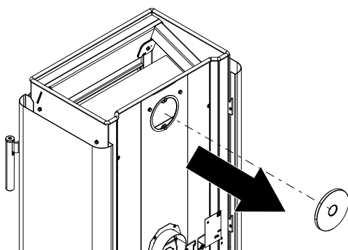
Fig. 22: Démontez le recouvrement
