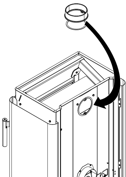
Fig. 23: Installer la tubulure à l'arrière
