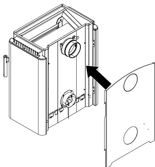
Fig. 24: Aggancio della parete posteriore
