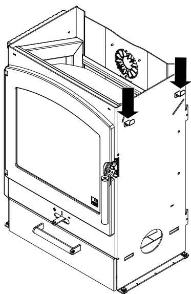
Fig. 14: Aggancio dei supporti dell'HMS
