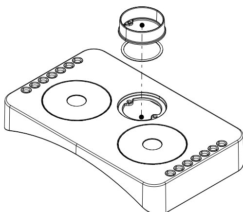
Fig. 21: Smontaggio del pezzo di collegamento e della guarnizione dal coperchio
