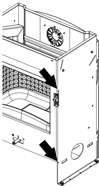
Fig. 8: Rimozione delle viti pre-assemblate
