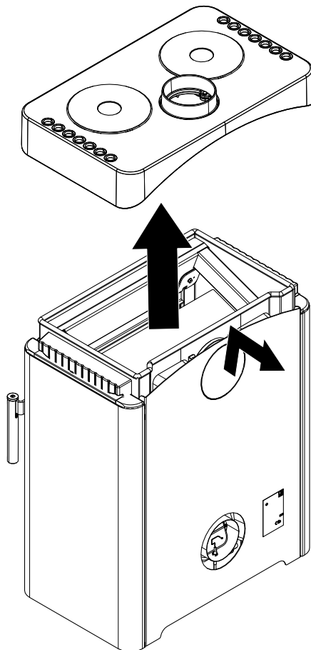
Fig. 19: Rimozione del coperchio e della parete posteriore
