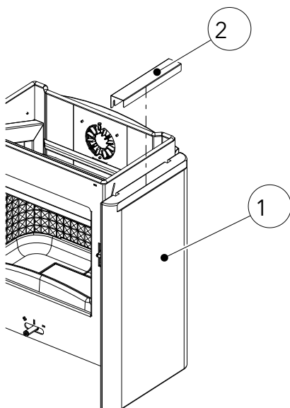
Fig. 13: Aggancio del rivestimento laterale in steatite
