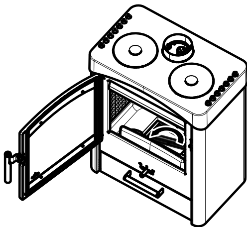
Fig. 29: Sbloccaggio e rimozione del box cenere
