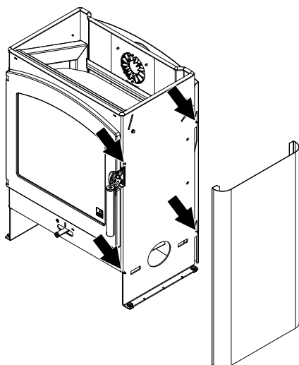
Fig. 9: Montaggio del rivestimento laterale
