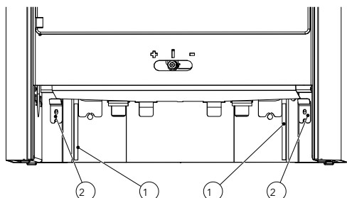
Fig. 27: Montaggio del cassetto in legno
