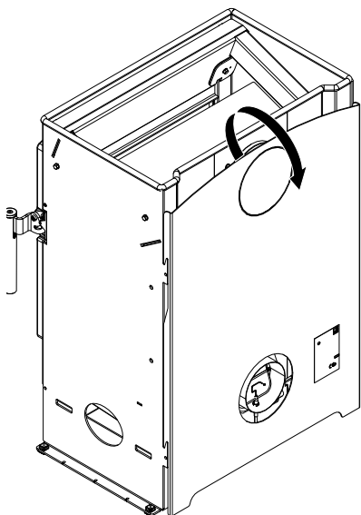
Fig. 7: Sollevamento e rimozione della parete posteriore
