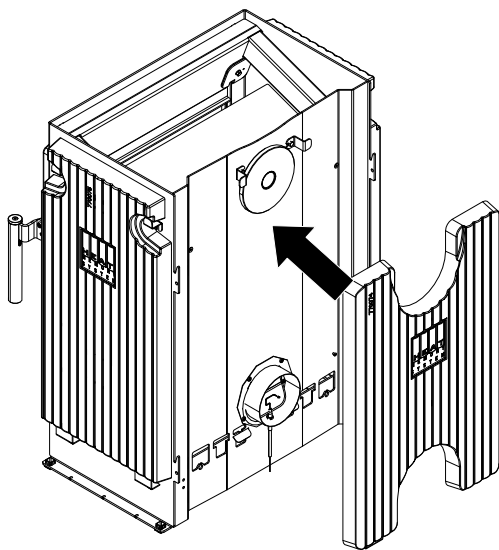
Fig. 17: Attaccare le pietre HMS in alto.
