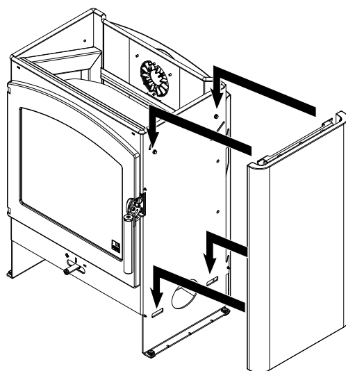
Fig. 11: Aggancio del rivestimento laterale in ceramica
