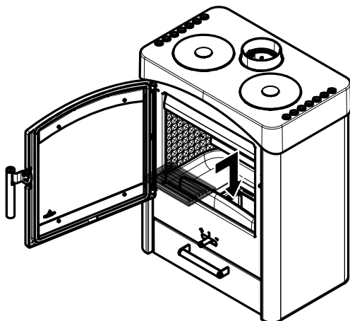
Fig. 30: Inserimento della griglia del box cenere
