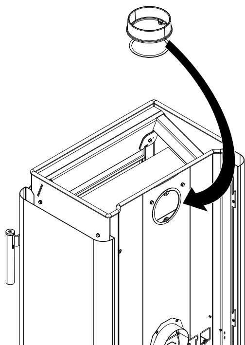
Fig. 23: Montaggio posteriore del pezzo di collegamento
