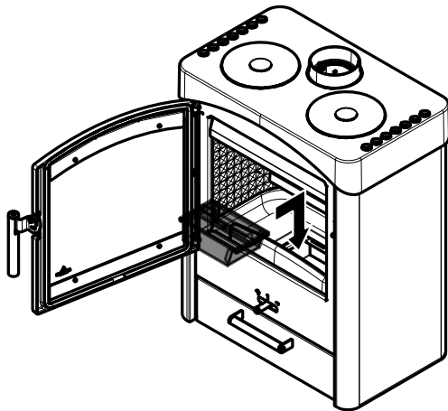
Fig. 28: Inserimento del box cenere nella stufa a caminetto
