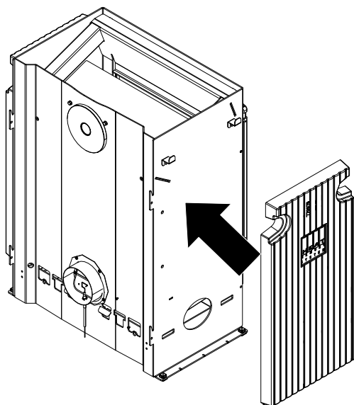
Fig. 16: Collocamento della pietra HMS
