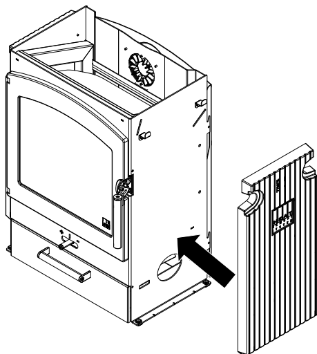
Fig. 15: Collocamento della pietra HMS
