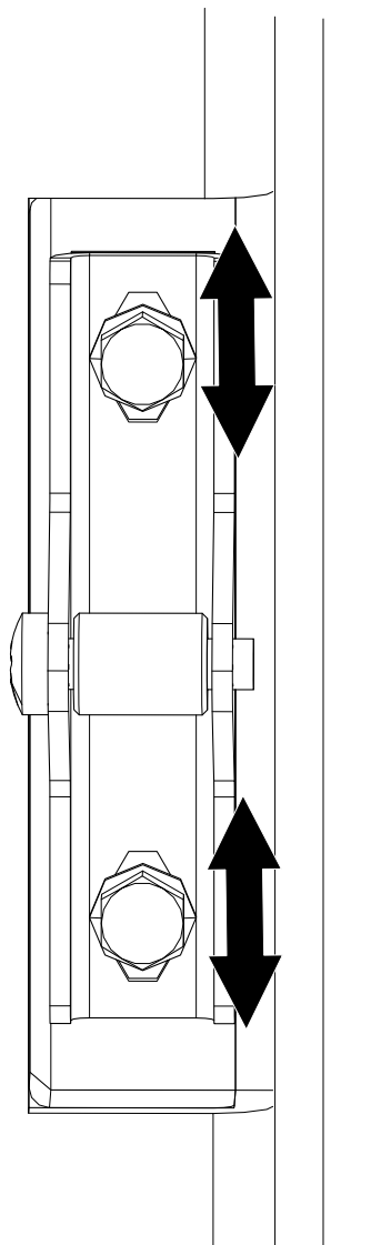
Abb. 29: Türverschluss einstellen
