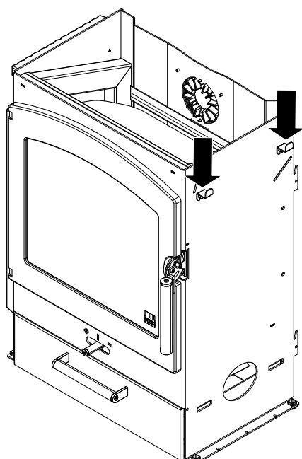
Abb. 15: HMS Halter einhängen
