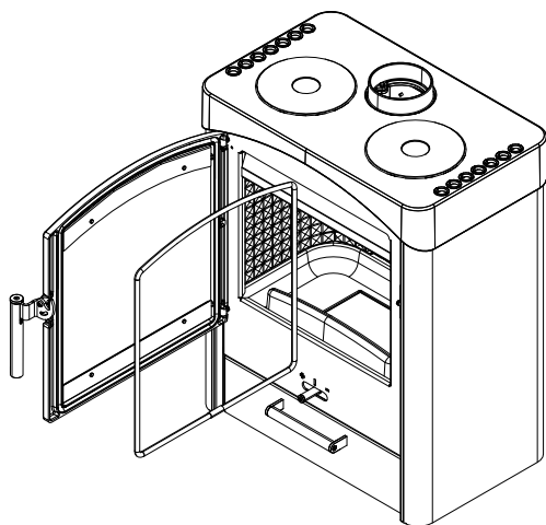
Abb. 33: Dichtung tauschen
