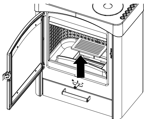
Abb. 34: Rost herausnehmen
