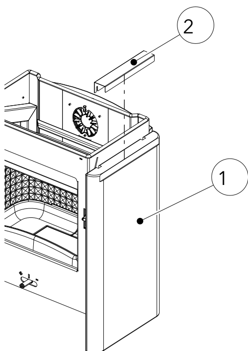
Abb. 14: Specksteinseitenverkleidung einhängen
