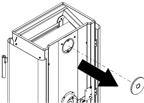
Abb. 23: Abdeckung demontieren
