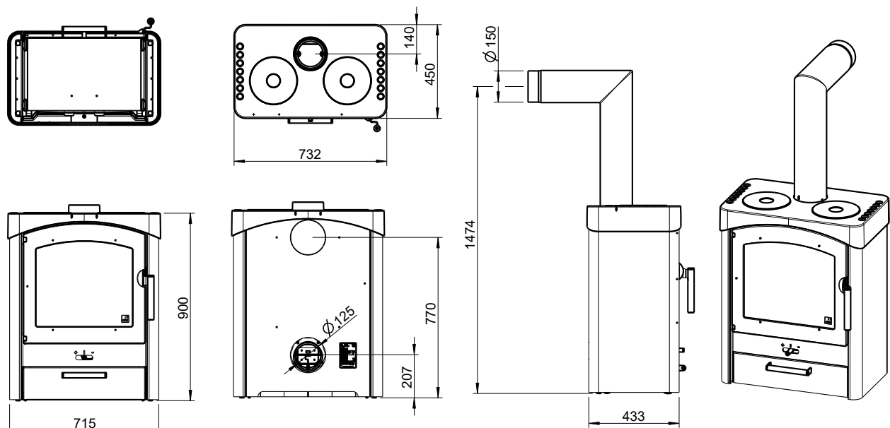
Abb. 1: Abmessungen
