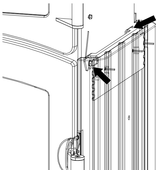
Fig. 11: Accrocher la partie inférieure de l'habillage latéral en céramique
