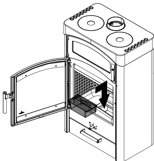
Fig. 30: Insérer le bac à cendres dans le poêle à bois
