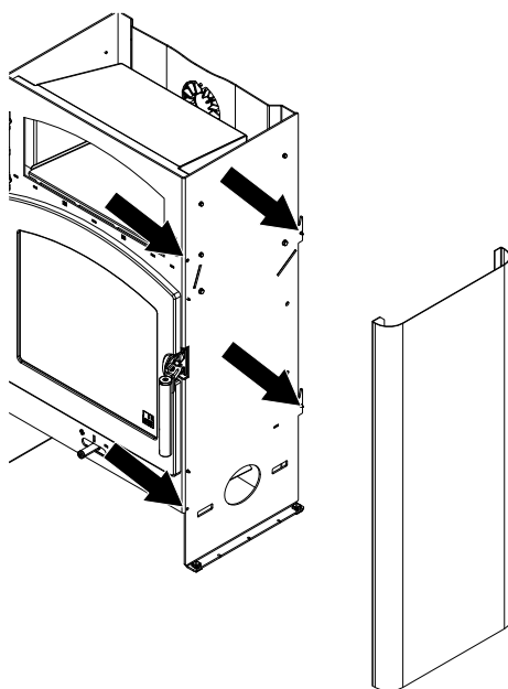
Fig. 9: Installer l'habillage latéral
