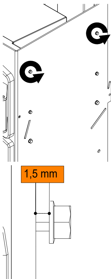
Fig. 13: Dévisser les vis
