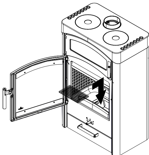
Fig. 32: Mettre la grille du bac à cendre en place
