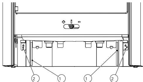
Fig. 29: Installer le tiroir en bois
