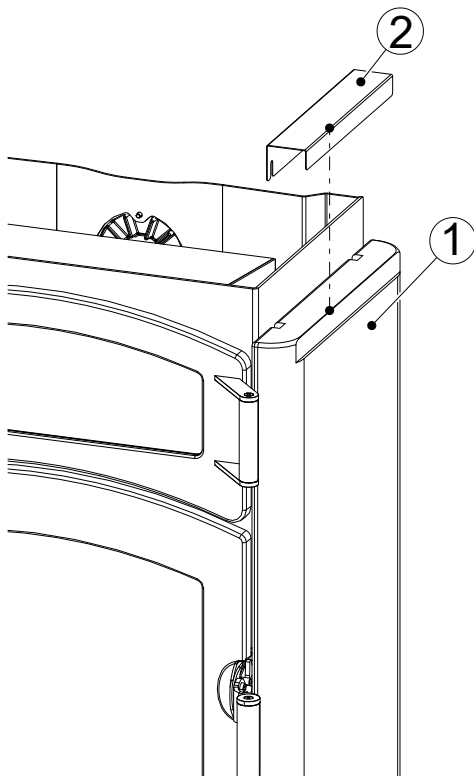
Fig. 14: Accrocher l'habillage latéral en pierre ollaire
