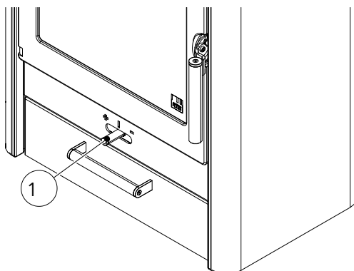
Fig. 35: Manette de régulation de l'air primaire / secondaire
