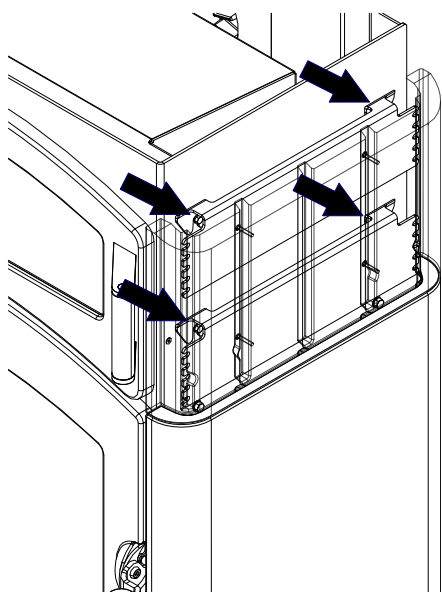
Fig. 12: Accrocher la partie supérieure de l'habillage latéral en céramique
