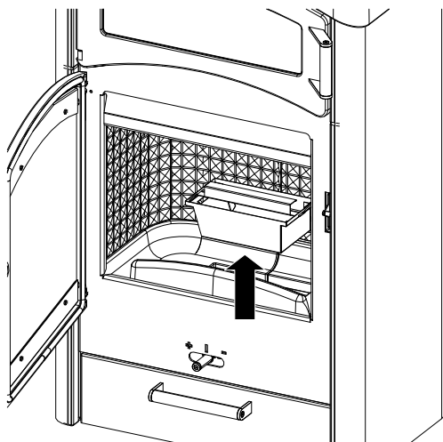
Fig. 41: Vider le bac à cendres
