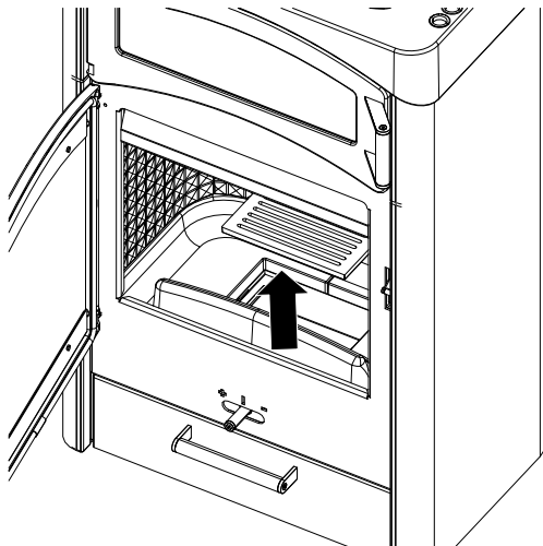
Fig. 38: Extraction de la grille
