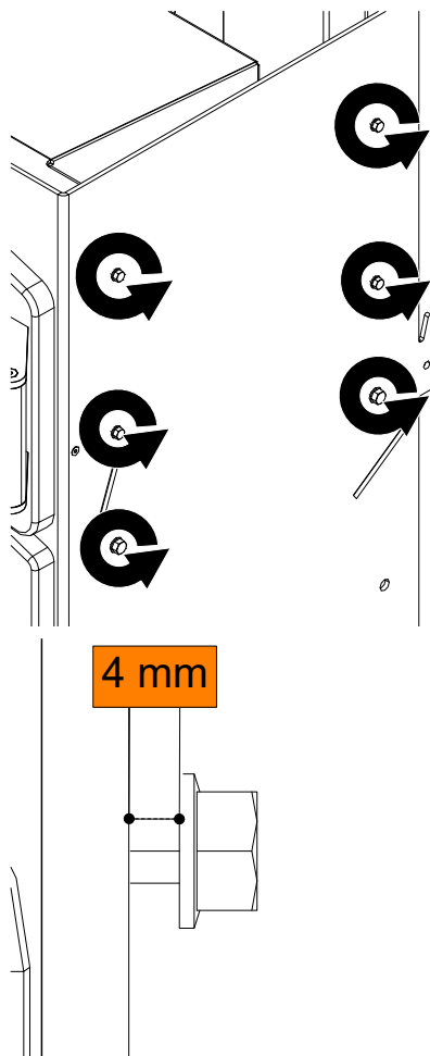
Fig. 10: Dévisser les vis
