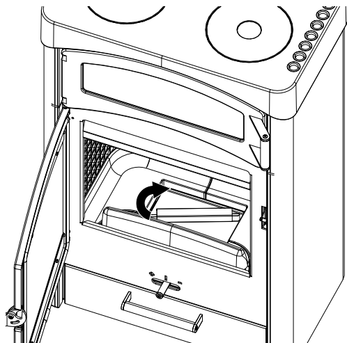
Fig. 39: Mettre le couvercle sur le bac à cendres
