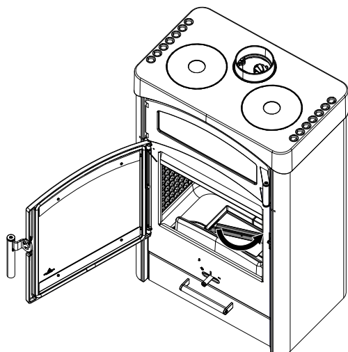
Fig. 31: Déverrouiller le couvercle du bac à cendres
