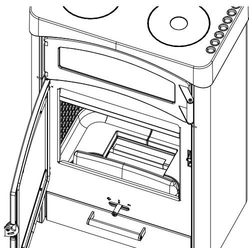
Fig. 40: Fermer le couvercle
