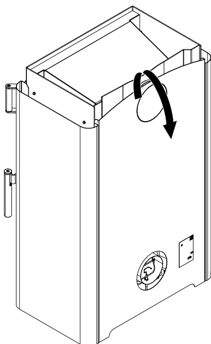
Fig. 43: Soulever la paroi arrière et l'enlever
