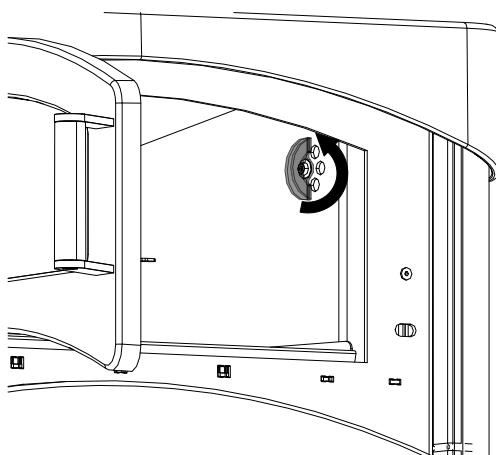
Fig. 34: Manette de régulation de l'air
