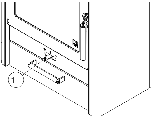
Fig. 31: Manette de régulation de l'air primaire / secondaire
