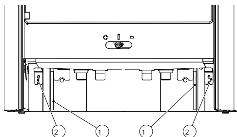
Fig. 20: Installer le tiroir en bois
