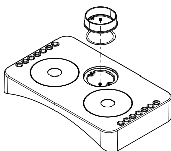
Fig. 8: Démonter tubulure et le joint du couvercle
