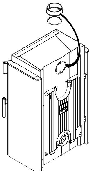
Fig. 10: Installer la tubulure à l'arrière
