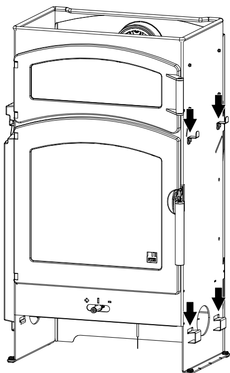
Fig. 15: Accrocher les fixations HMS
