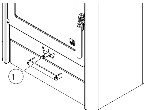
Fig. 26: Manette de régulation de l'air primaire / secondaire
