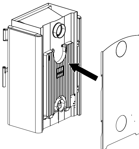
Fig. 11: Accrocher la paroi arrière
