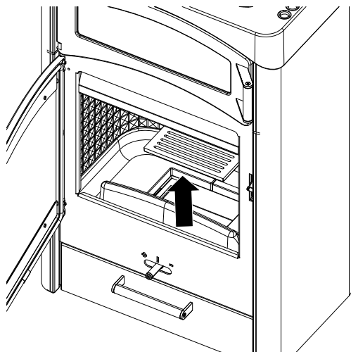
Fig. 29: Extraction de la grille
