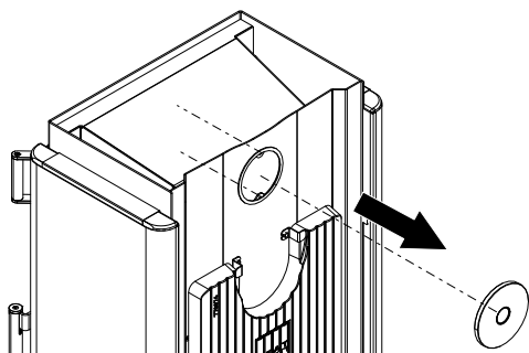
Fig. 9: Démonter le recouvrement
