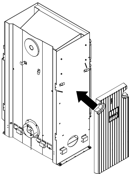
Fig. 17: Poser la pierre HMS
