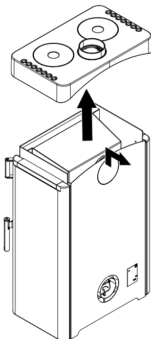
Fig. 6: Enlever le couvercle et la paroi arrière
