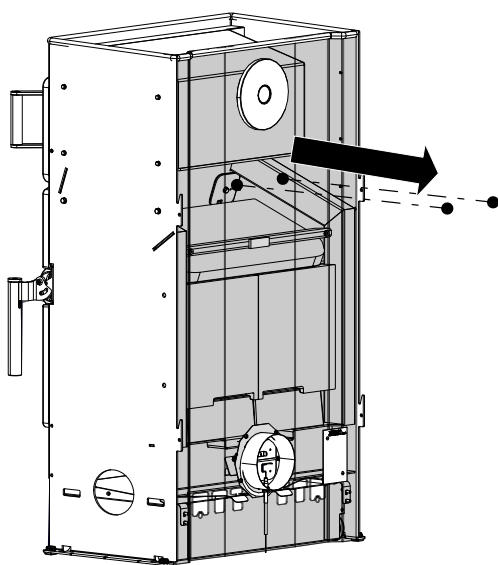
Fig. 14: Retirez le garde-boue
