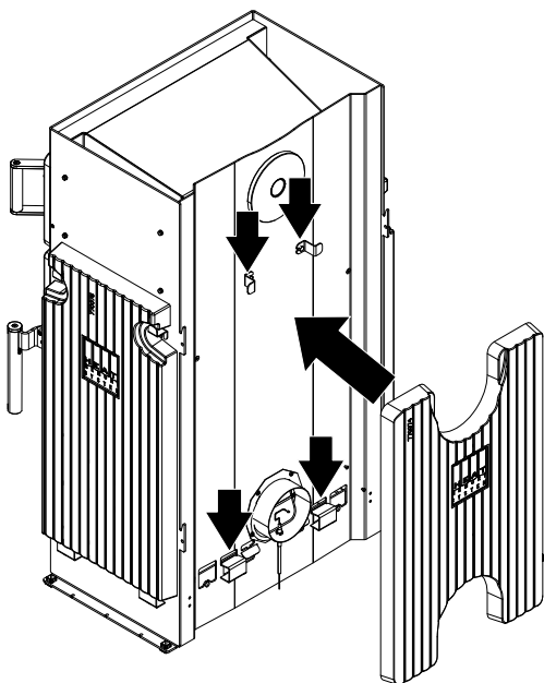
Fig. 18: Poser la pierre HMS à l'arrière
