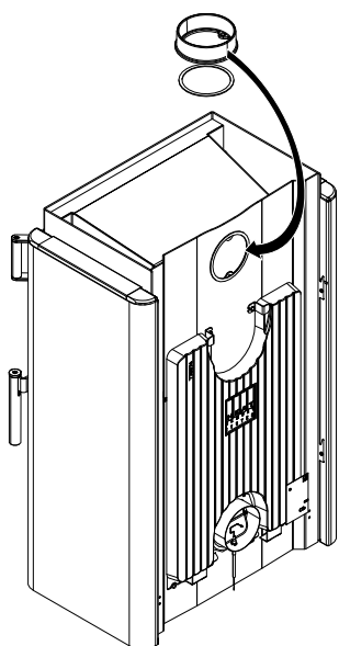
Fig. 25: Installez la tubulure à l'arrière
