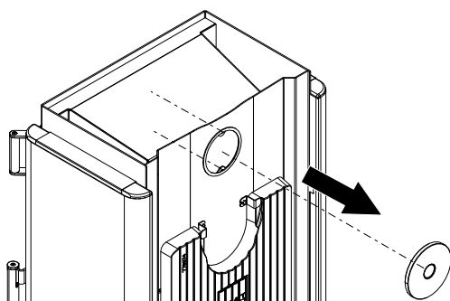
Fig. 9: Smontaggio della copertura
