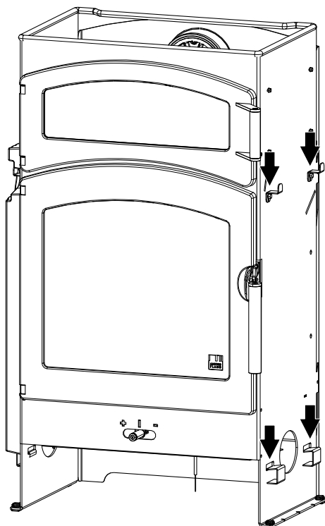
Fig. 15: Appendere il supporto HMS
