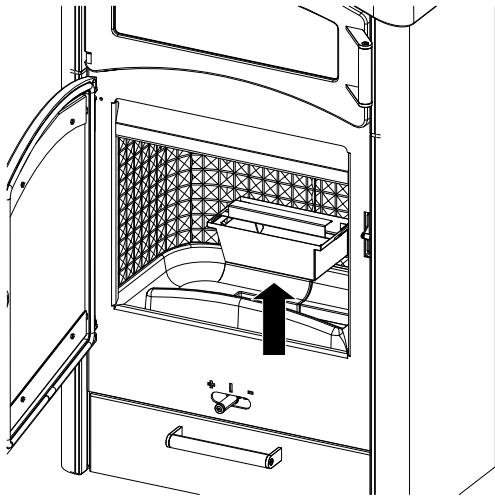
Fig. 32: Svuotamento del box cenere
