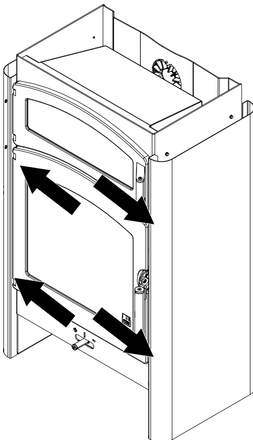
Fig. 36: Rimozione delle quattro viti anteriori
