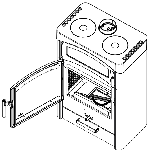
Fig. 22: Sbloccaggio e rimozione del box cenere
