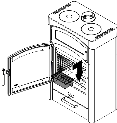
Fig. 21: Inserimento del box cenere nella stufa
