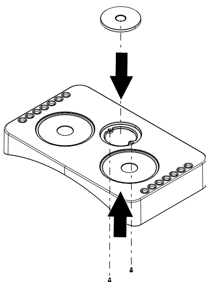
Fig. 12: Montaggio della copertura sul coperchio.
