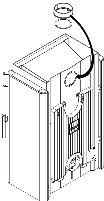
Fig. 10: Montaggio del pezzo di collegamento posteriormente
