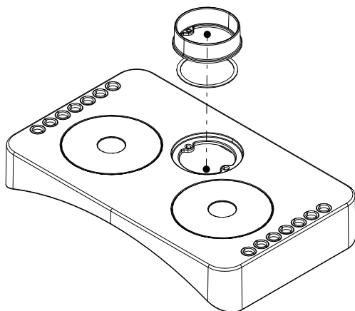
Fig. 8: Smontaggio del pezzo di collegamento e della guarnizione dal coperchio
