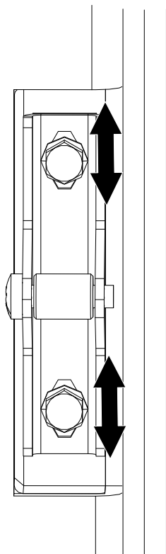
Fig. 24: Regolazione della serratura dello sportello
