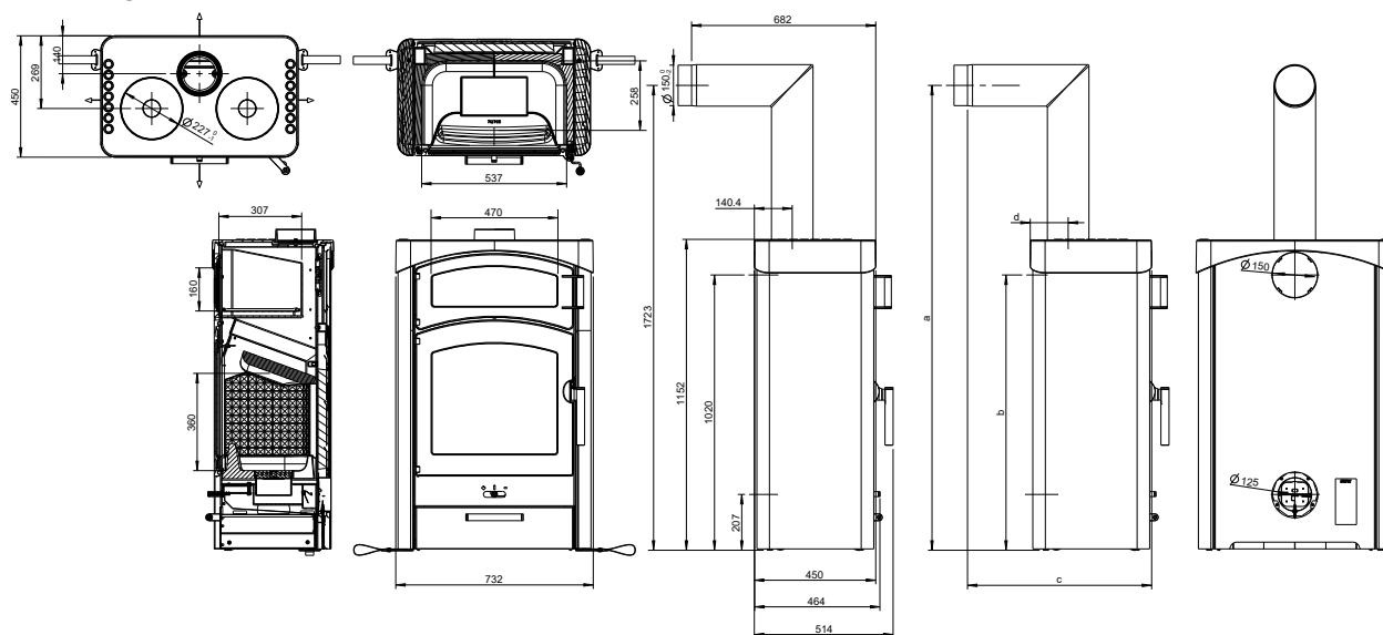
Fig. 1: Dimensioni
