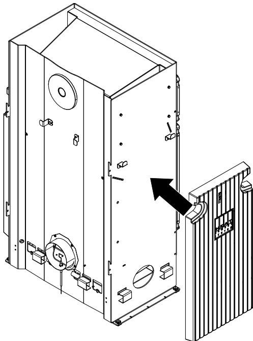
Fig. 17: Collocazione della pietra HMS
