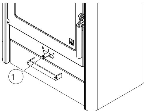
Fig. 26: Regolatore dell'aria primaria/secondaria
