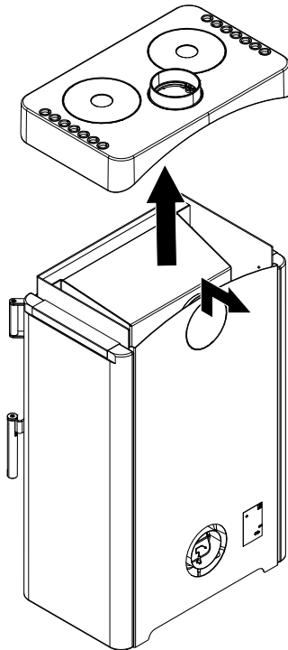
Fig. 6: Rimozione del coperchio e della parete posteriore
