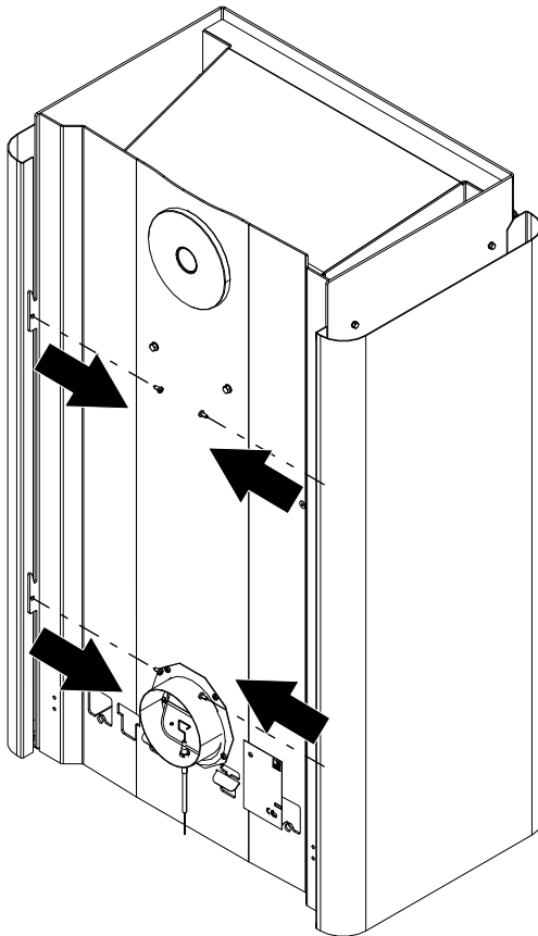
Fig. 35: Rimozione delle viti sul retro
