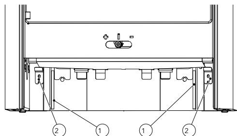
Fig. 20: Montaggio del cassetto in legno
