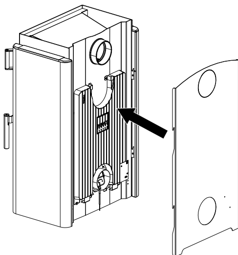
Fig. 11: Aggancio della parete posteriore
