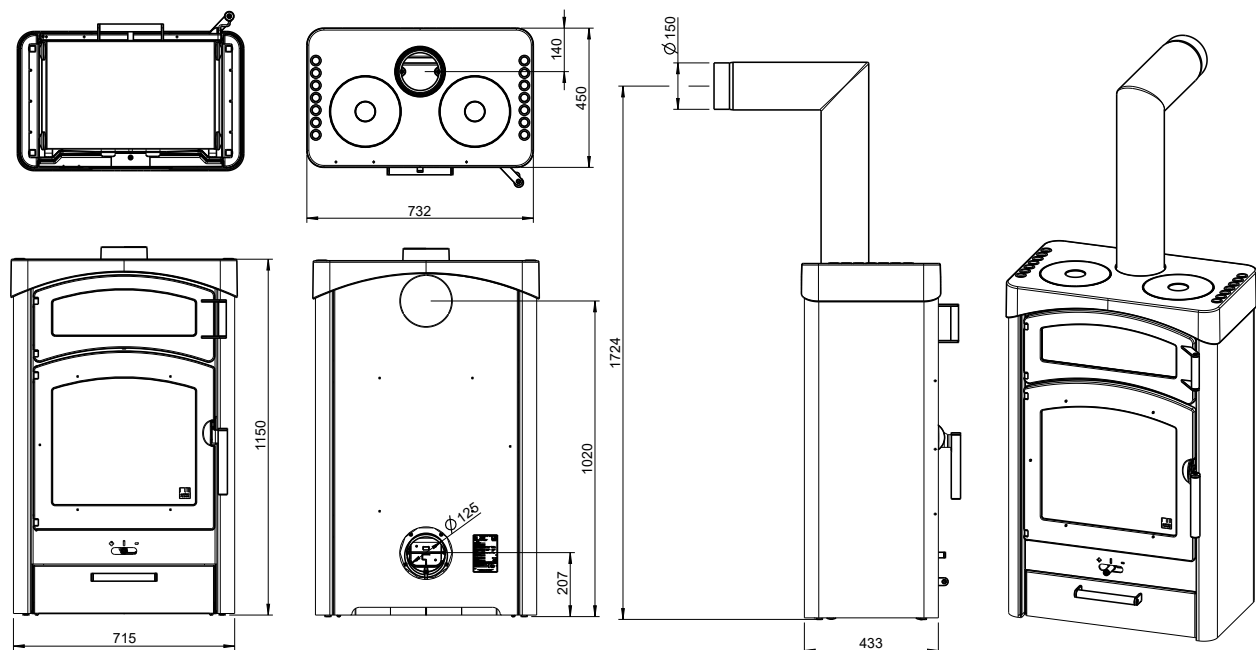
Abb. 1: Abmessungen
