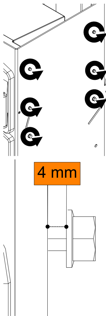
Abb. 11: Schrauben aufdrehen
