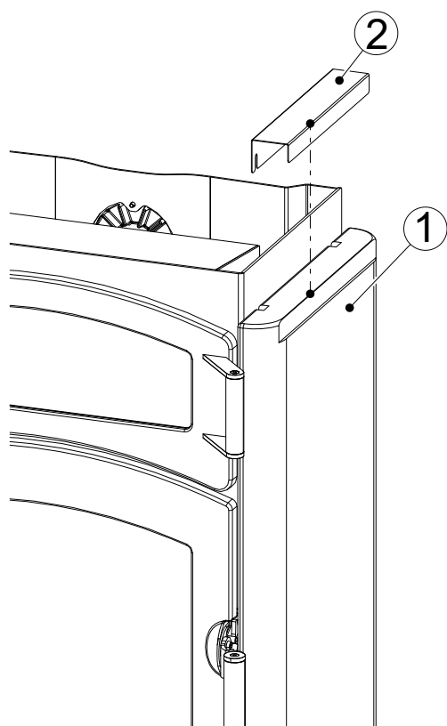
Abb. 15: Specksteinseitenverkleidung einhängen
