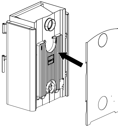
Abb. 26: Rückwand einhängen
