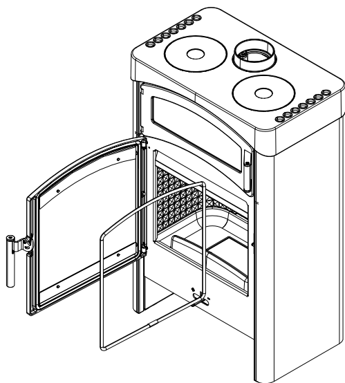
Abb. 34: Dichtung tauschen
