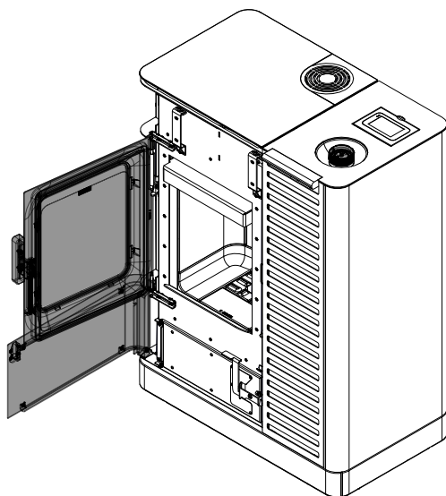
Fig. 79: Ouvrir les portes.
