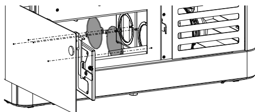
Fig. 97: Déposer les recouvrements
