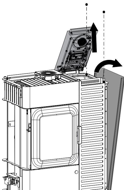
Fig. 104: Déposer l'habillage latéral droit
