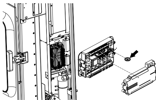
Fig. 85: Remplacer la pile mémoire
