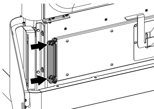
Fig. 80: Ajuster la porte du tiroir à cendres
