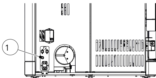
Fig. 100: Limiteur de température de sécurité
