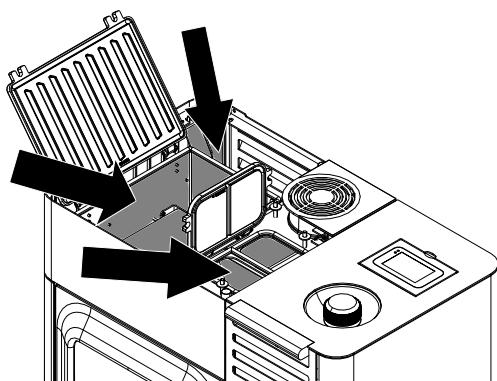
Fig. 93: Nettoyer le circuit de fumées en haut
