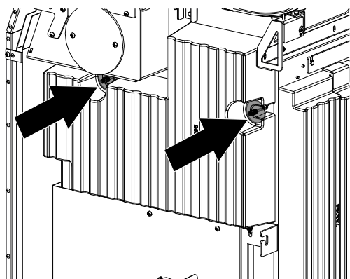
Fig. 12: Installer la pierre HMS arrière
