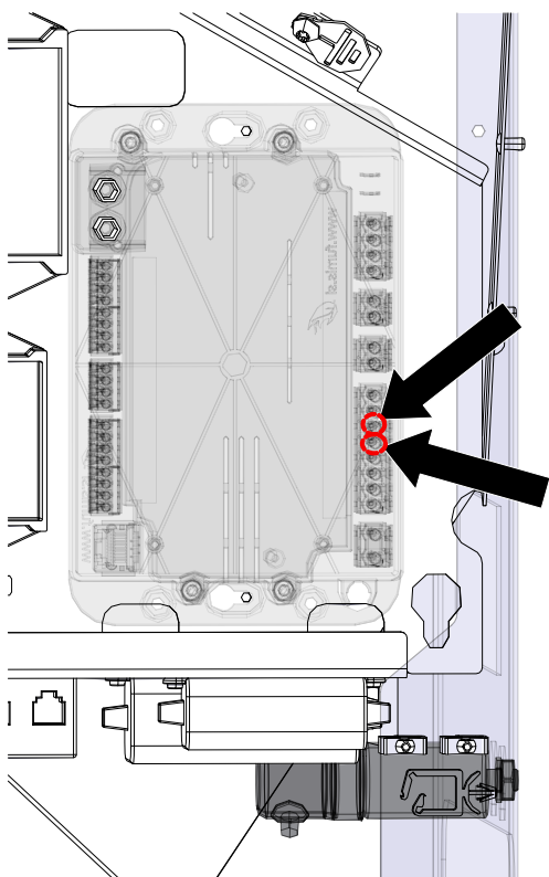
Fig. 25: Brancher le kit canalisation
