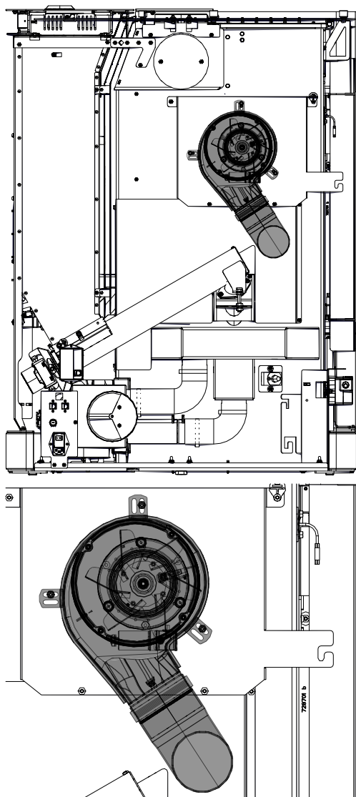
Fig. 21: Installer le kit canalisation
