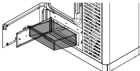
Fig. 96: Retirer le tiroir à cendres
