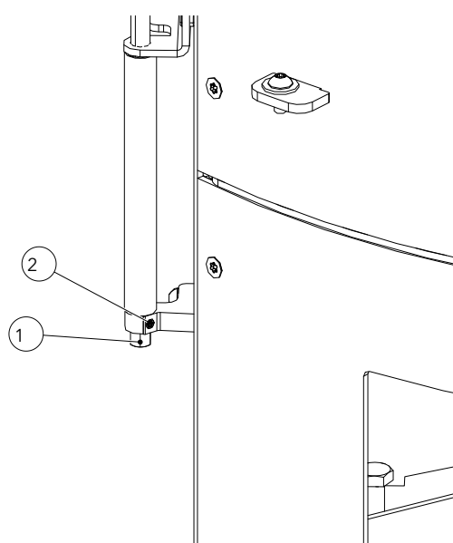
Fig. 78: Régler la force de fermeture de la porte
