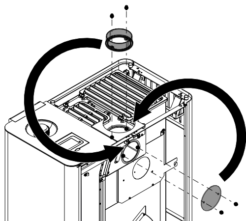
Fig. 17: Enlever le raccordement du conduit de fumée et le couvercle
