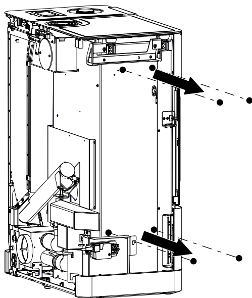
Fig. 9: Dévisser les vis en place
