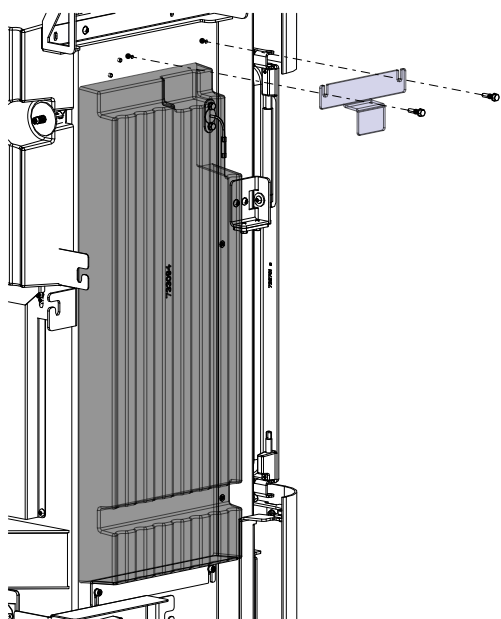
Fig. 14: Poser la pierre HMS
