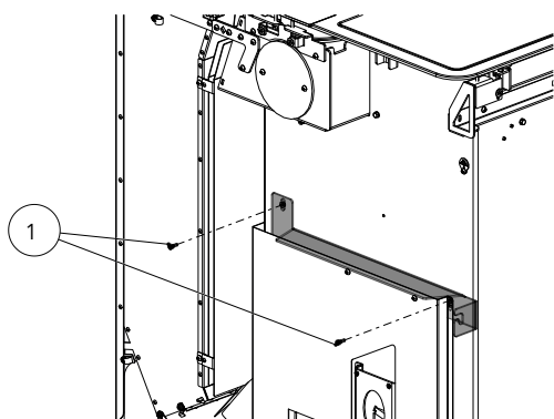
Fig. 11: Installer la fixation HMS arrière
