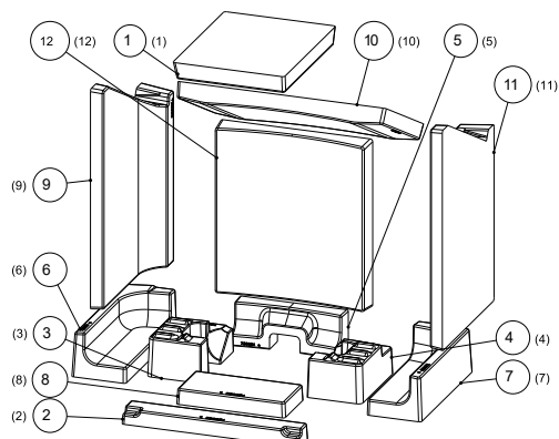
Fig. 8: Installer la Keramott
