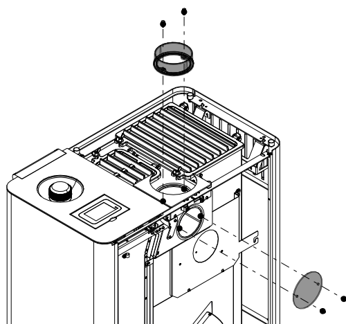
Fig. 17: Enlever le raccordement du conduit de fumée et le couvercle
