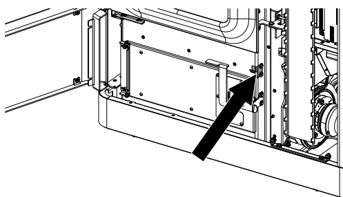
Fig. 84: Régler la porte du bas au niveau de la serrure
