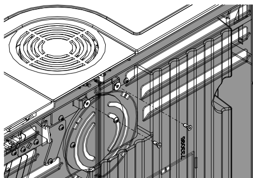
Fig. 108: Enlever le panneau arrière
