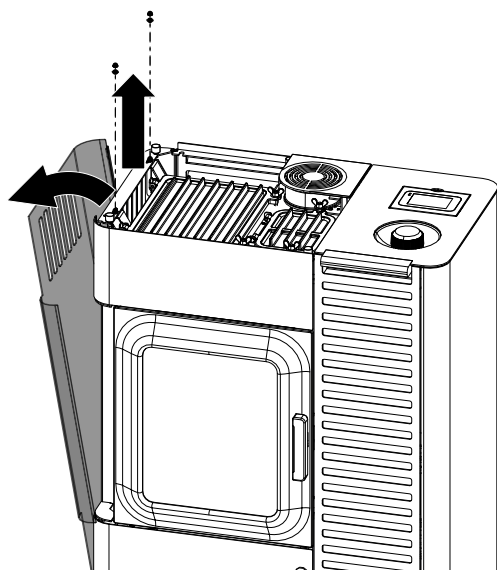
Fig. 103: Déposer l'habillage latéral gauche
