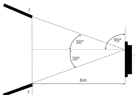
Fig. 45: Angle de fonctionnement
