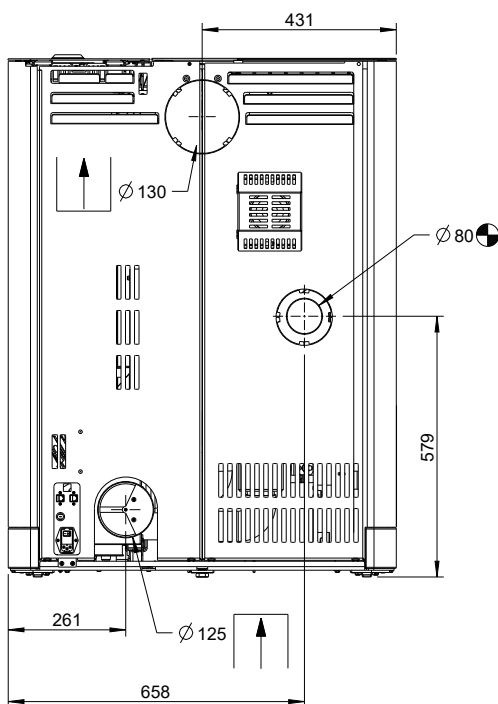
Fig. 31: Raccordement de l'alimentation en air de combustion
