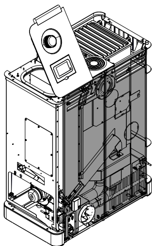
Fig. 106: Enlever le panneau arrière
