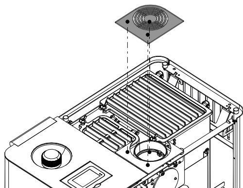
Fig. 16: Enlever le couvercle emboîtable
