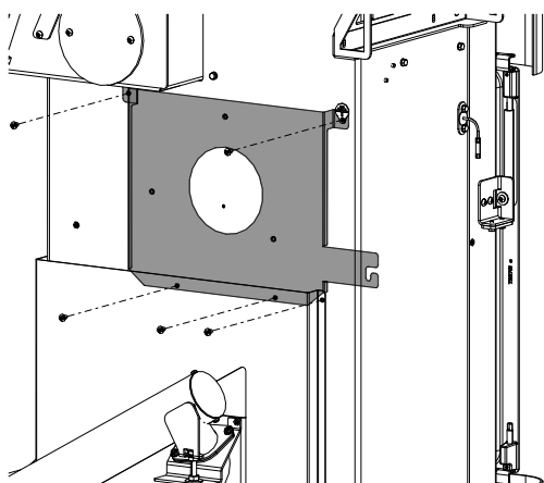
Fig. 10: Enlever la tôle
