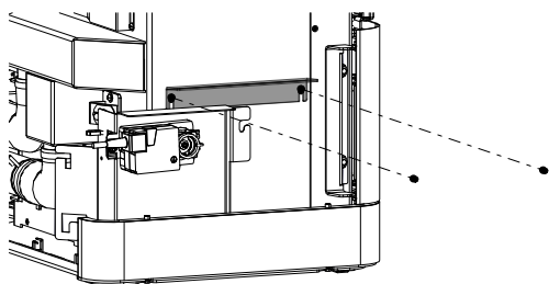
Fig. 13: Installer la fixation HMS latérale
