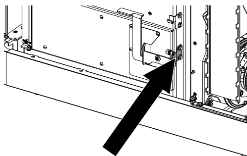
Fig. 81: Réglage de la porte du tiroir à cendres au niveau de la serrure
