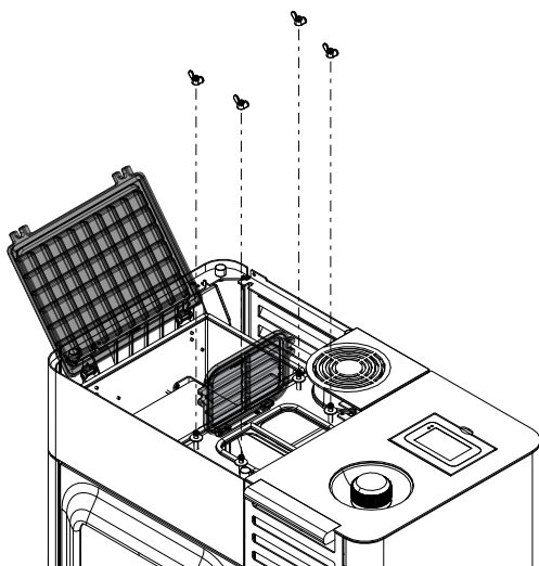
Fig. 92: Trappe de visite
