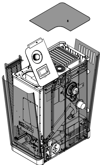
Fig. 29: Remettre tout en place
