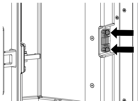
Fig. 76: Réglage au niveau de la serrure
