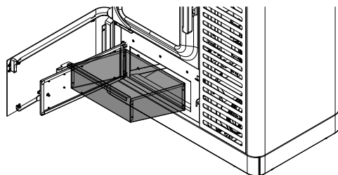
Fig. 90: Retirer le tiroir à cendres
