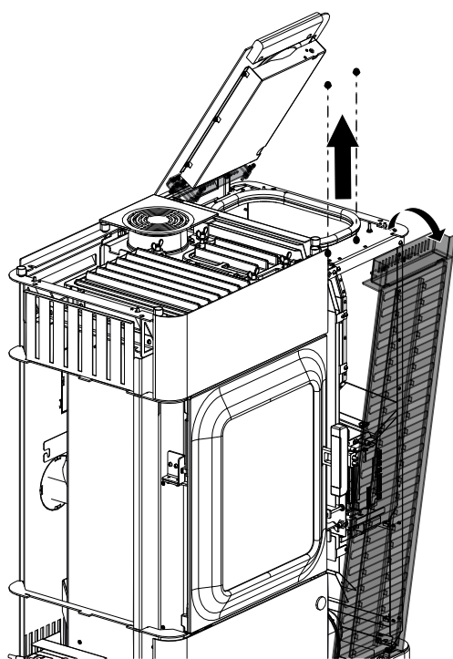
Fig. 105: Déposer l'habillage latéral avant
