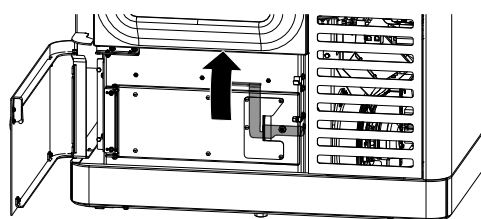
Fig. 89: Ouvrir la porte du tiroir à cendres.
