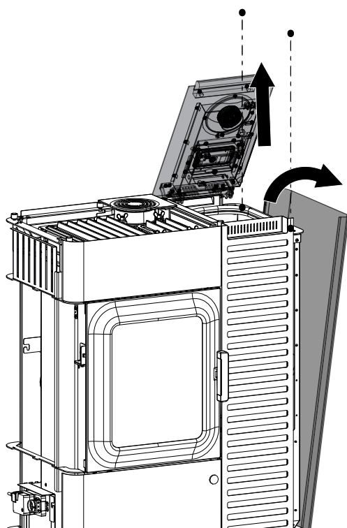
Fig. 105: Déposer l'habillage latéral droit
