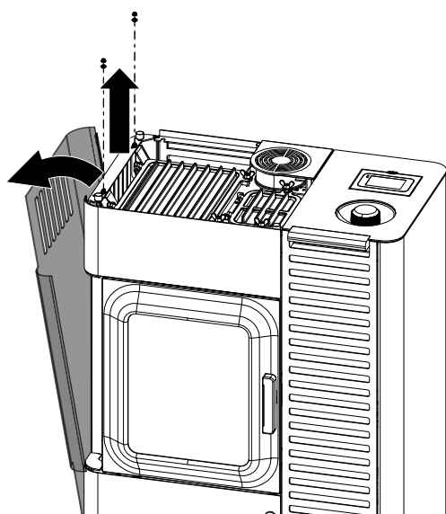
Fig. 104: Déposer l'habillage latéral gauche
