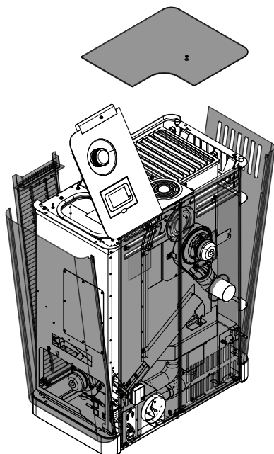
Fig. 30: Remettre tout en place
