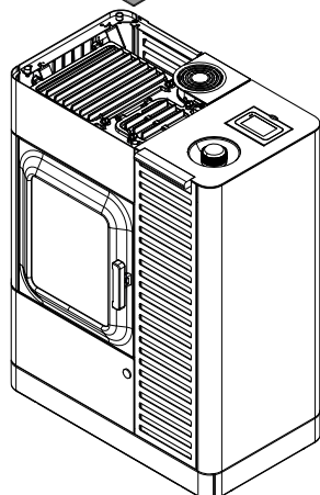
Fig. 92: Enlever la plaque en verre
