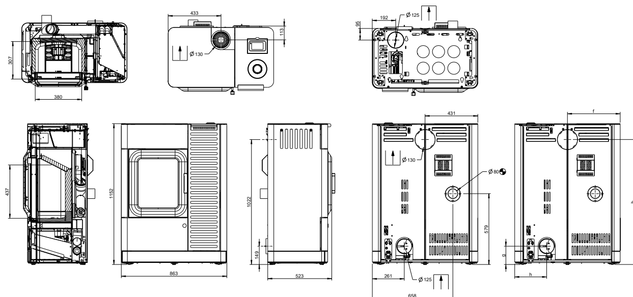
Fig. 1: Dimensions du Mo Duo
