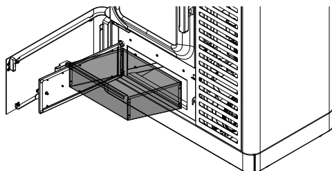
Fig. 97: Retirer le tiroir à cendres
