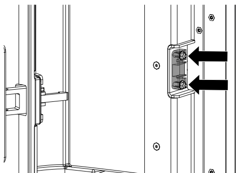
Fig. 77: Réglage au niveau de la serrure
