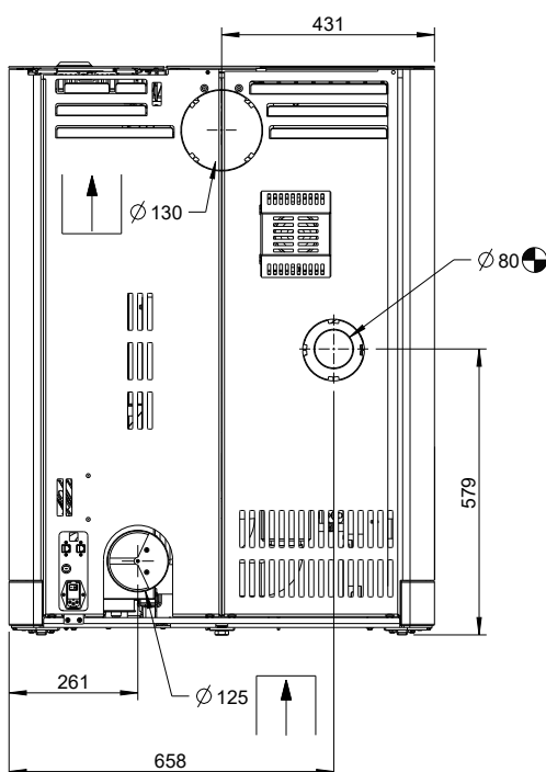
Fig. 32: Collegamento dell'alimentazione esterna di aria comburente
