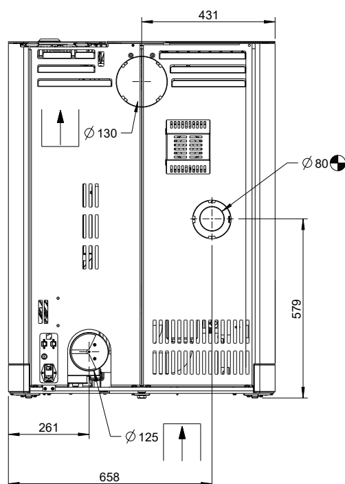
Fig. 32: Collegamento dell'alimentazione esterna di aria comburente
