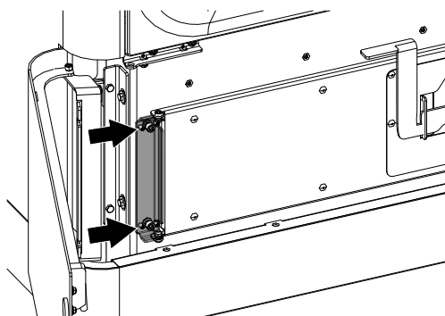
Fig. 81: Regolazione dello sportello del vassoio per la cenere
