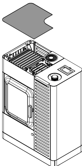
Fig. 92: Rimozione della lastra di vetro
