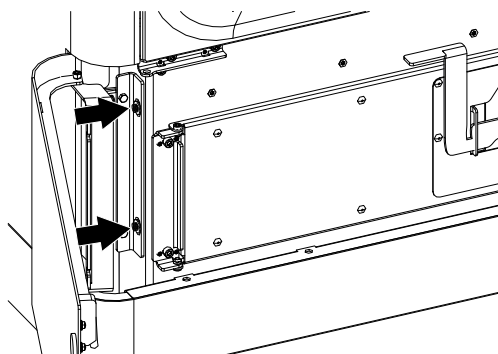
Fig. 84: Regolazione dello sportello inferiore
