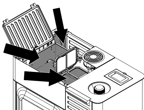
Fig. 94: Pulizia delle canne fumarie in alto
