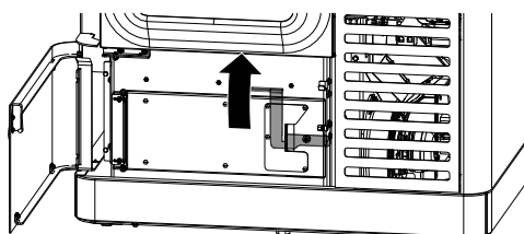
Fig. 96: Apertura dello sportello del cassetto della cenere
