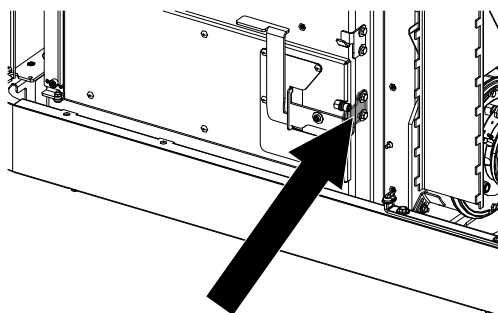
Fig. 82: Regolazione dello sportello del cassetto della cenere sul lato di chiusura
