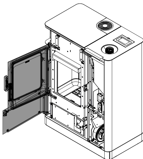
Fig. 74: Apertura di entrambi gli sportelli
