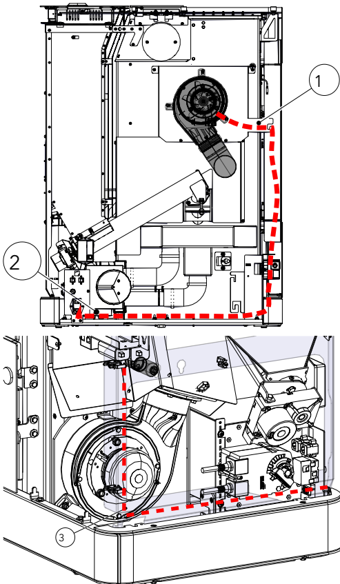
Fig. 24: Posa del cavo
