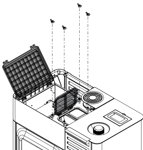
Fig. 93: Coperchio per la pulizia
