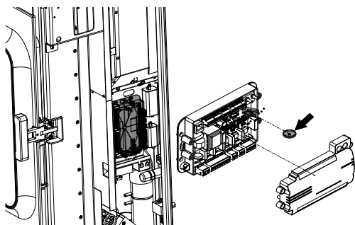
Fig. 86: Sostituzione della batteria tampone
