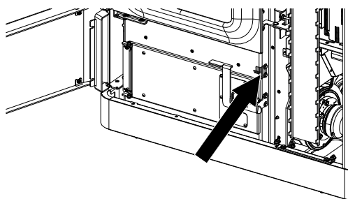
Fig. 85: Regolazione in basso dello sportello sul lato di chiusura
