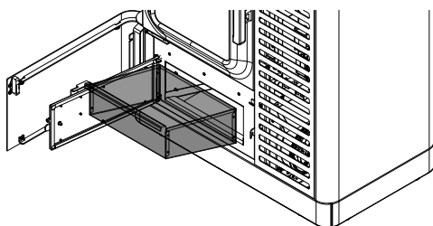
Fig. 97: Rimozione del cassetto della cenere
