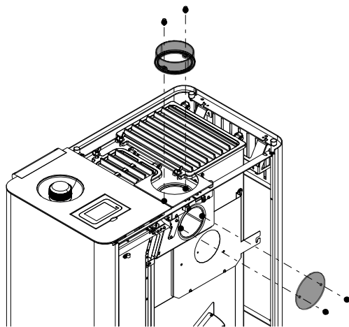
Fig. 18: Rimozione del raccordo del tubo dei fumi e del coperchio
