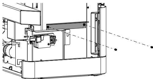
Fig. 14: Montaggio del supporto laterale dell'HMS
