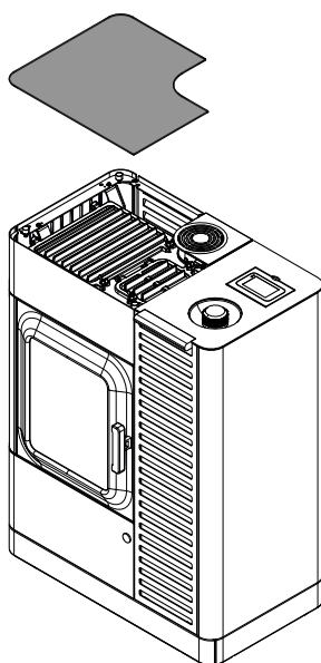
Fig. 16: Rimozione della lastra di vetro
