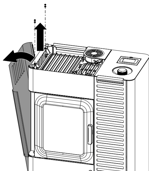
Fig. 104: Smontaggio del rivestimento laterale sinistro
