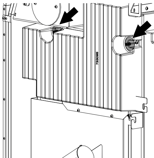
Fig. 13: Montaggio della pietra posteriore dell'HMS
