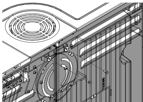
Fig. 109: Rimozione della parete posteriore
