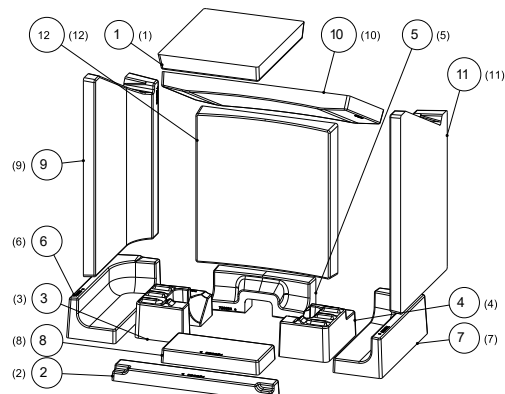
Fig. 9: Montaggio del Keramott
