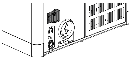
Fig. 108: Rimozione del box WLAN
