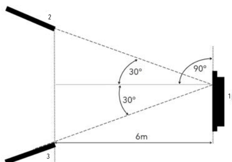
Fig. 46: Angolo di lavoro
