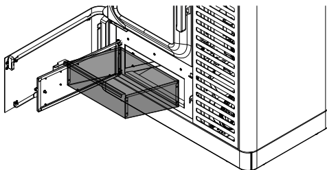
Fig. 91: Rimozione del cassetto della cenere
