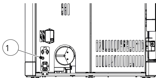
Fig. 101: Limitatore di temperatura di sicurezza
