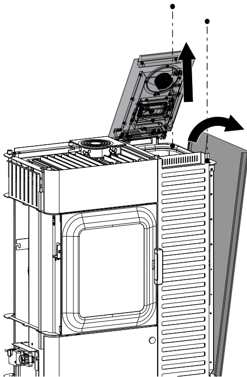
Fig. 105: Smontaggio del rivestimento laterale destro
