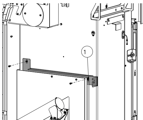
Fig. 12: Montaggio del supporto posteriore dell'HMS
