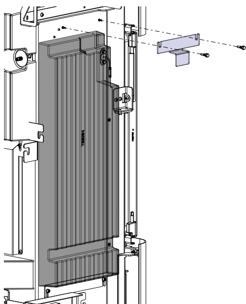
Fig. 15: Collocazione della pietra HMS
