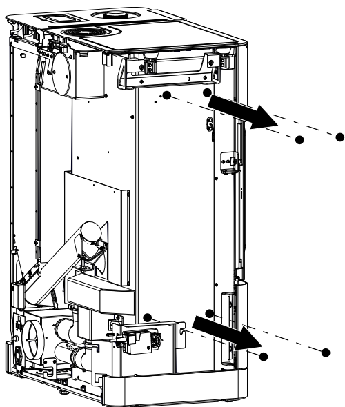
Fig. 10: Svitamento delle viti pre-esistenti
