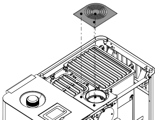
Fig. 17: Rimozione del coperchio interno
