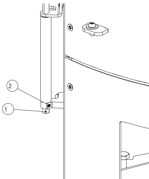
Fig. 79: Regolazione della forza di chiusura dello sportello
