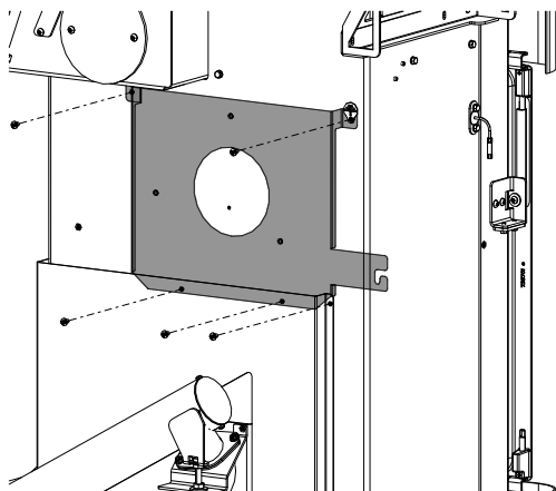
Fig. 11: Rimozione della lamiera
