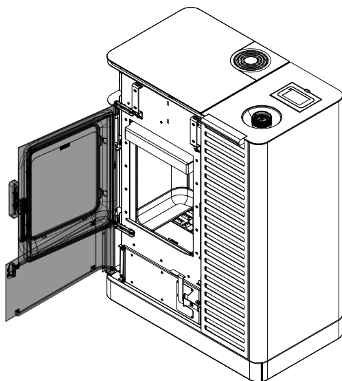
Fig. 80: Apertura degli sportelli
