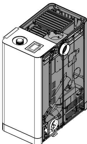
Fig. 21: Rimontaggio di tutte le parti
