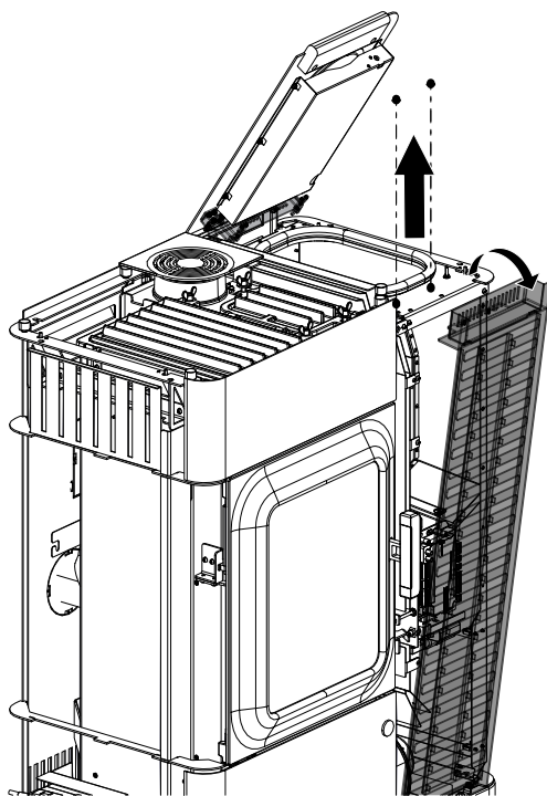
Fig. 106: Smontaggio del rivestimento laterale anteriore
