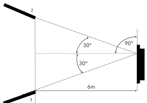
Abb. 46: Betriebswinkel
