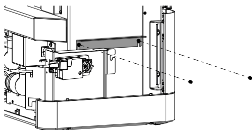
Abb. 14: Seitlichen HMS-Halter montieren
