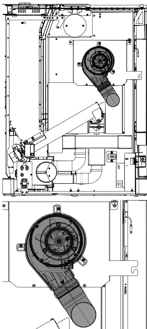
Abb. 22: Luftmodul anbringen
