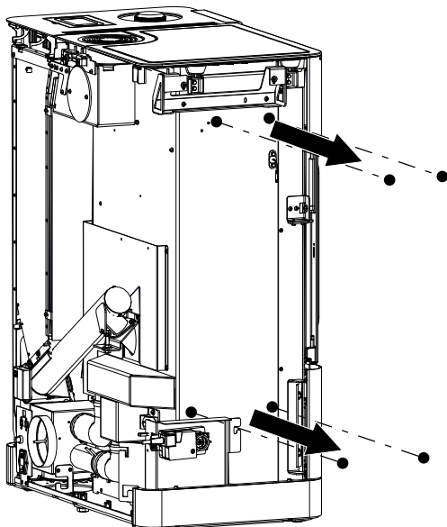
Abb. 10: Bestehende Schrauben lösen
