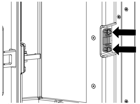
Abb. 77: Verschlussseitig einstellen
