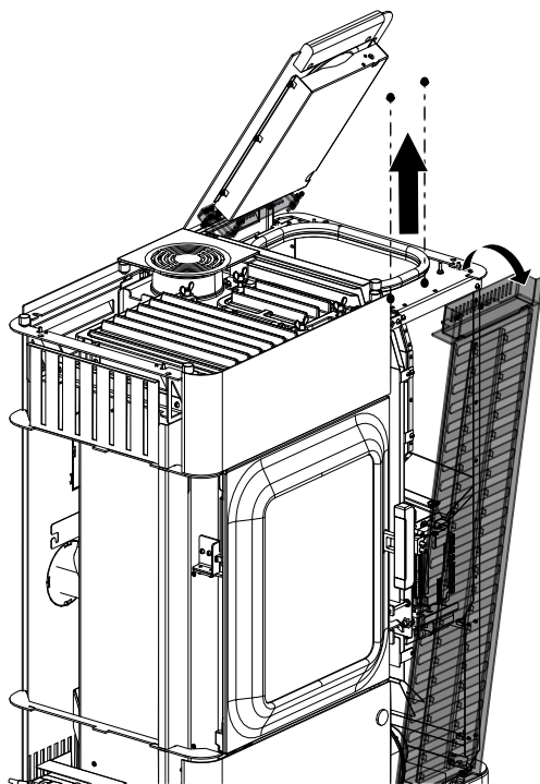
Abb. 106: Vordere Seitenverkleidung abmontieren
