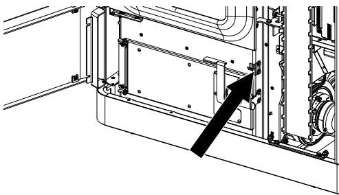
Abb. 85: verschlusseitig Tür unten einstellen
