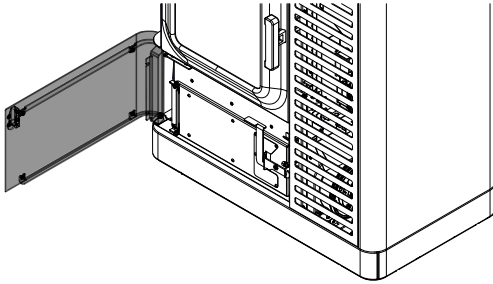
Abb. 83: Untere Tür öffnen
