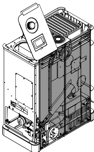
Abb. 107: Rückwand abnehmen
