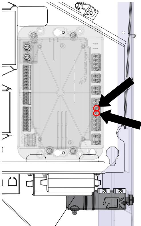
Abb. 26: Luftverteilermodul anstecken
