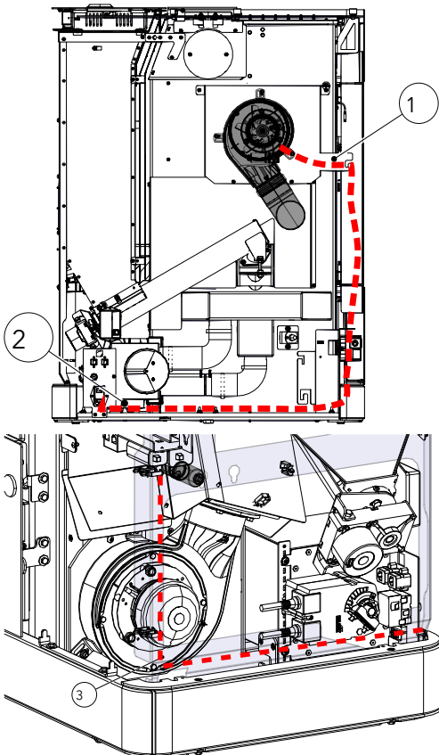
Abb. 24: Kabel verlegen
