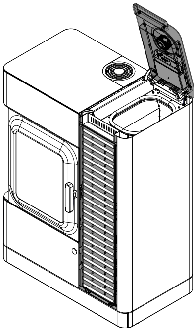
Abb. 73: Fronträger demontieren
