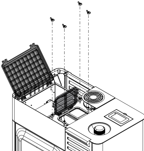
Abb. 93: Putzdeckel
