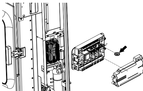
Abb. 86: Speicherbatterie tauschen
