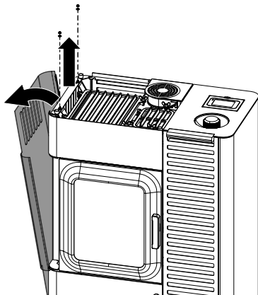
Abb. 104: Linke Seitenverkleidung abmontieren
