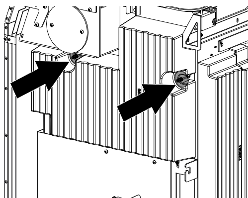
Abb. 13: Hinteren HMS-Stein montieren
