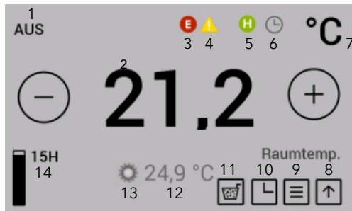
Abb. 47: Raumtemperaturanzeige, div. Funktionen
