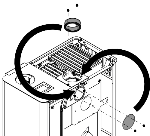
Abb. 18: Rauchrohranschluss und Deckel abnehmen
