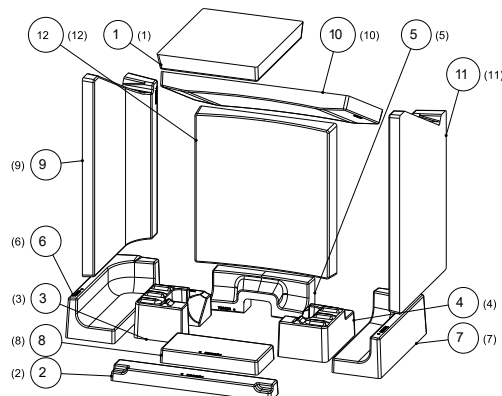
Abb. 9: Keramott montieren
