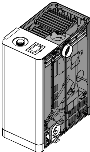
Abb. 21: Alles wieder montieren
