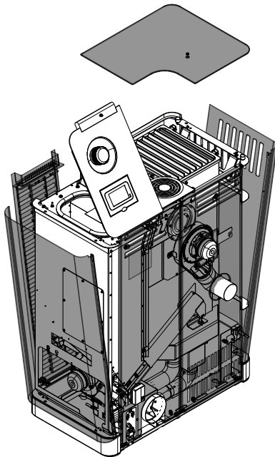
Abb. 30: Alles wieder montieren
