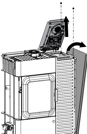
Abb. 105: Rechte Seitenverkleidung abmontieren
