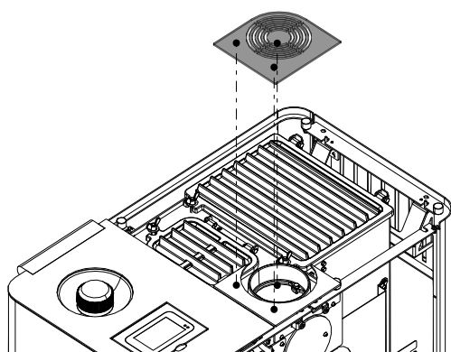
Abb. 17: Einlagedeckel abnehmen
