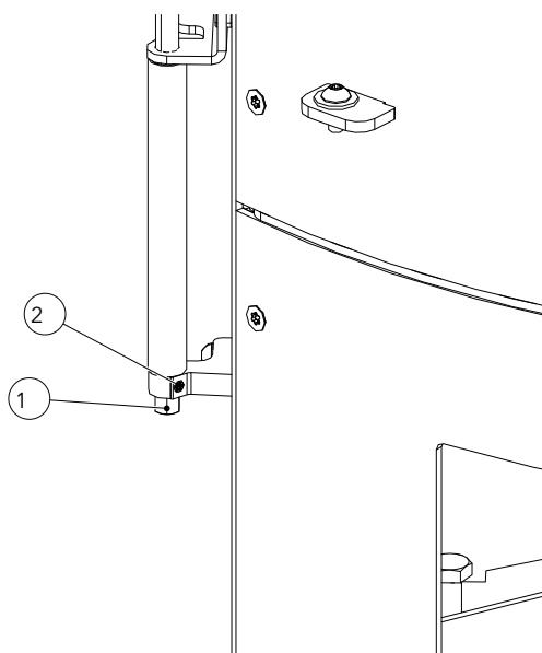
Abb. 79: Türschließkraft einstellen
