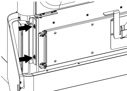
Abb. 84: Untere Tür einstellen
