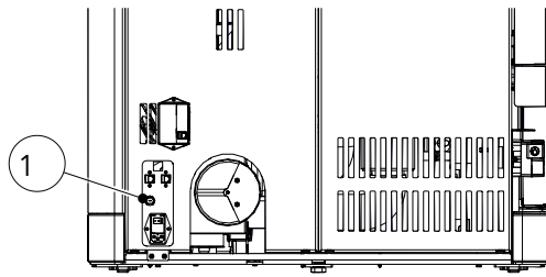
Abb. 101: Sicherheitstemperaturbegrenzer
