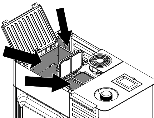
Abb. 94: Rauchgaszüge oben reinigen
