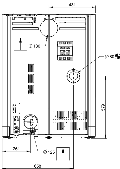
Abb. 32: Anschluss Verbrennungsluftzufuhr
