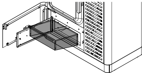
Abb. 91: Aschelade entnehmen
