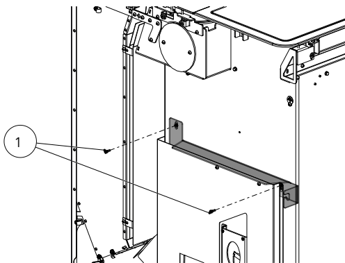
Abb. 13: Hinteren HMS-Halter montieren
