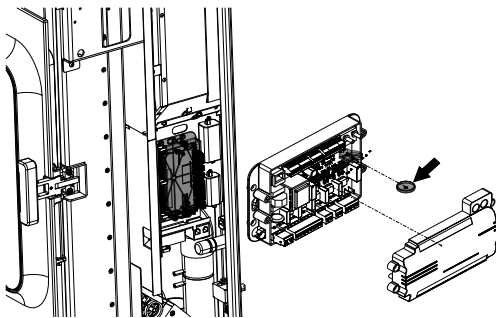
Abb. 87: Speicherbatterie tauschen
