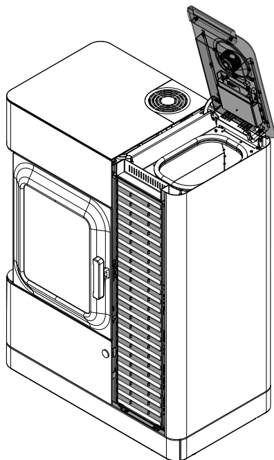
Abb. 41: Pellets füllen
