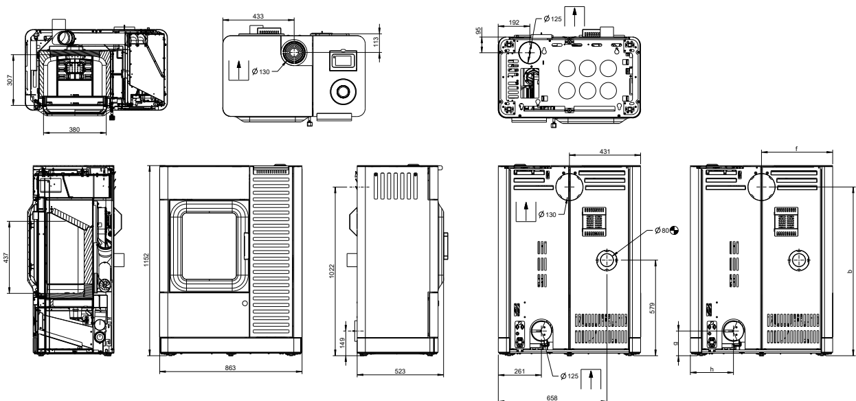
Abb. 2: Mo Duo Abmessungen
