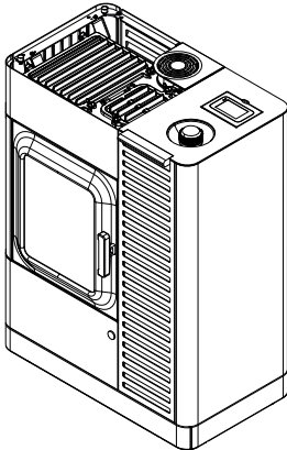
Abb. 104: Glasplatte abnehmen
