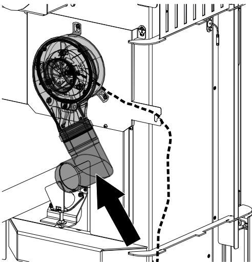
Abb. 29: Rohr raufstecken
