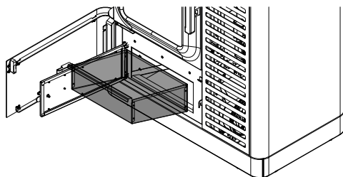
Abb. 92: Aschenlade entnehmen
