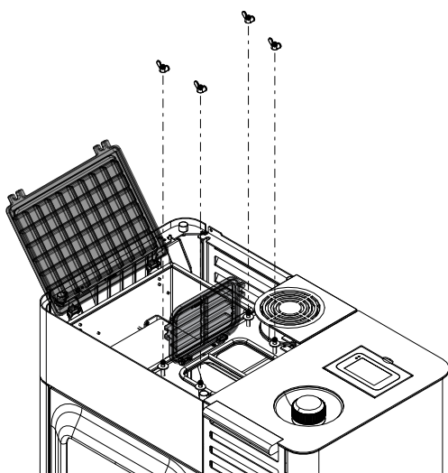
Abb. 94: Putzdeckel
