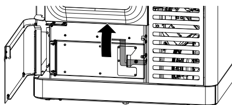
Abb. 91: Aschenladetür öffnen
