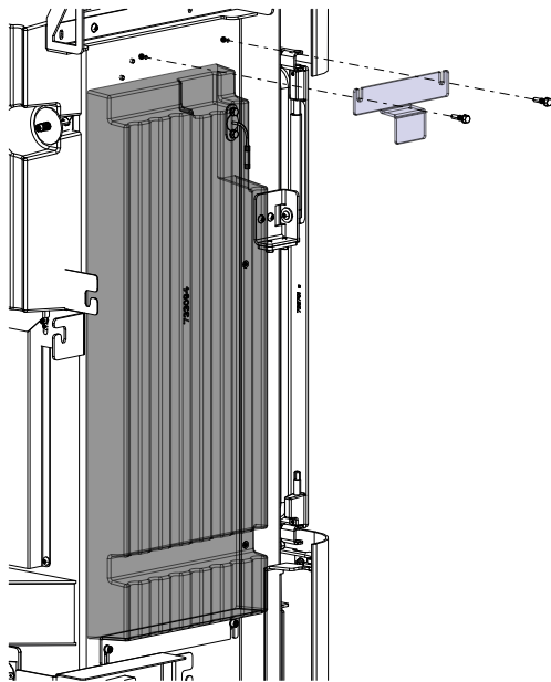
Abb. 16: HMS-Stein anbringen
