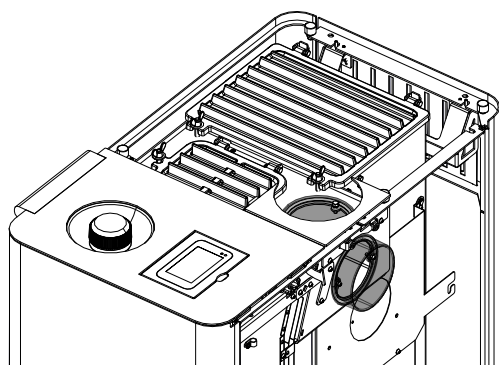
Abb. 20: Teile vertauscht
