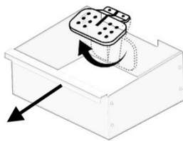
Abb. 49: Aschelade entnehmen
