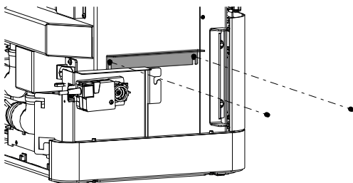
Abb. 15: Seitlichen HMS-Halter montieren
