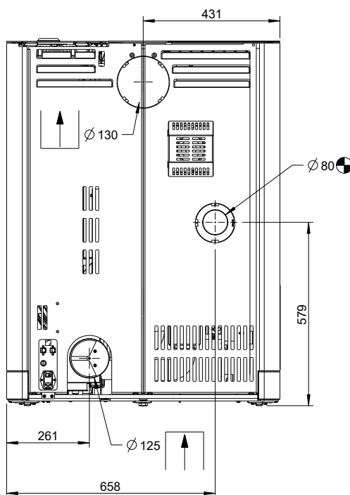
Abb. 33: Anschluss Verbrennungsluftzufuhr
