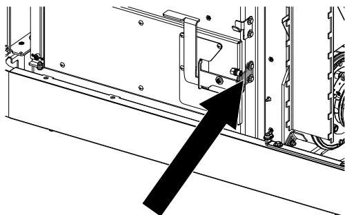
Fig. 101: Réglage de la porte du tiroir à cendres au niveau de la serrure
