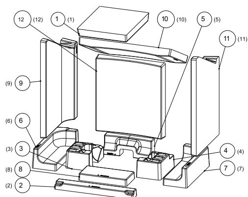
Fig. 22: Installer la Keramott
