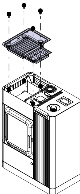
Fig. 113: Enlever la plaque de cuisson
