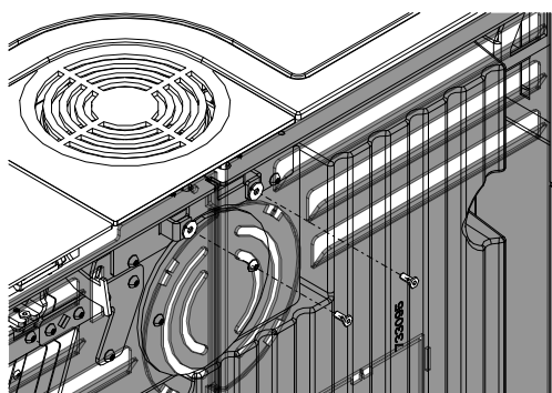
Fig. 128: Enlever le panneau arrière
