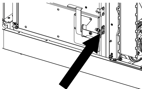
Fig. 102: Réglage de la porte du tiroir à cendres au niveau de la serrure
