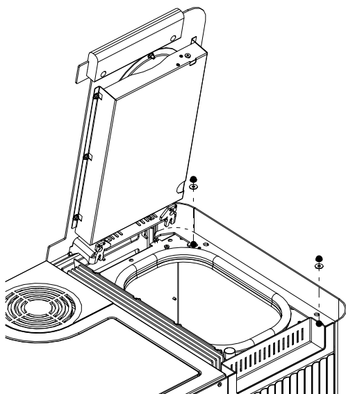
Fig. 126: Retirez le panneau latéral droit
