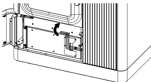
Fig. 108: Ouvrir la porte du tiroir à cendres
