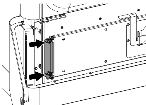
Fig. 101: Ajuster la porte du tiroir à cendres
