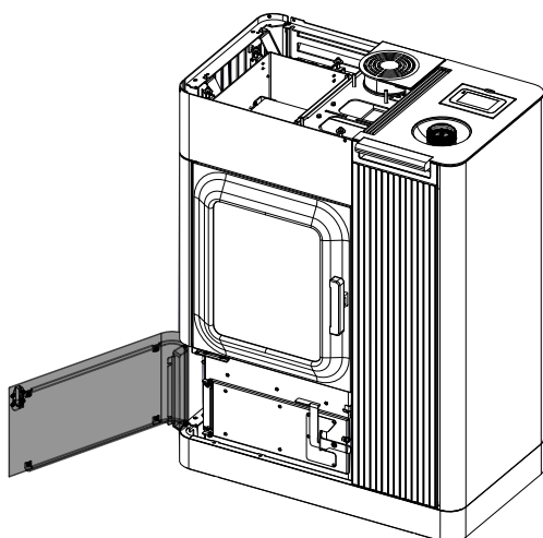
Fig. 115: Ouvrir la porte
