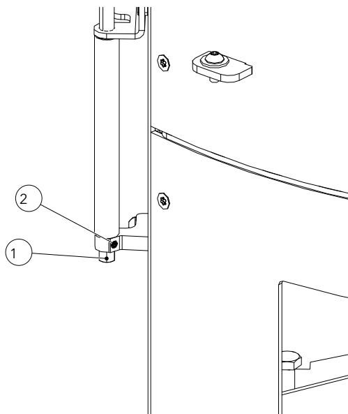
Fig. 96: Régler la force de fermeture de la porte
