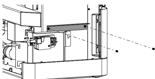
Fig. 47: Installer la fixation HMS latérale
