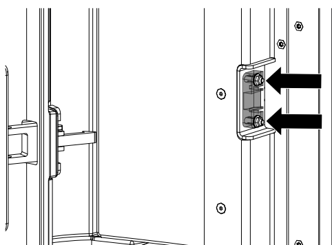
Fig. 94: Réglage au niveau de la serrure
