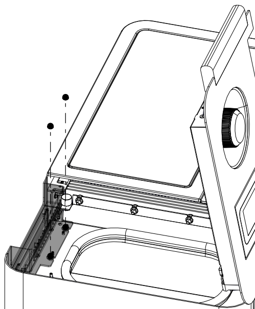
Fig. 123: Installer la façade en acier
