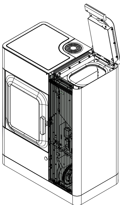
Fig. 90: Mettre le support pour habillage en place
