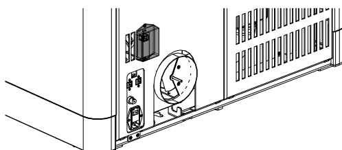
Fig. 127: Enlever le recouvrement de la box WiFi
