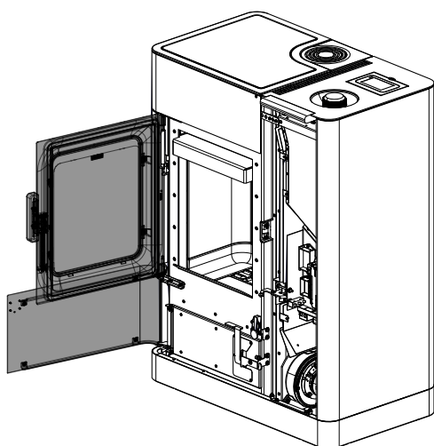
Fig. 91: Ouvrir les deux portes
