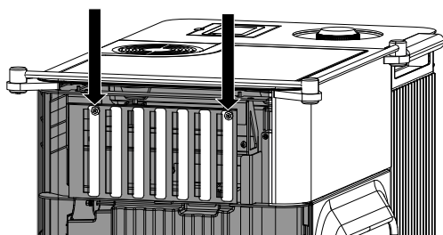
Fig. 125: Enlever l'habillage latéral gauche
