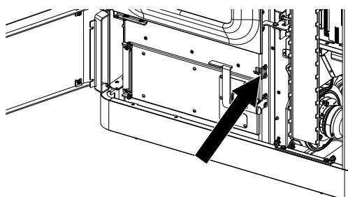
Fig. 99: Régler la porte du bas au niveau de la serrure
