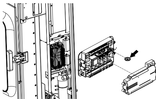
Fig. 106: Remplacer la pile mémoire
