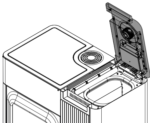
Fig. 122: Ouvrir le couvercle du réservoir
