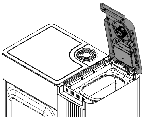
Fig. 124: Ouvrir le couvercle du réservoir
