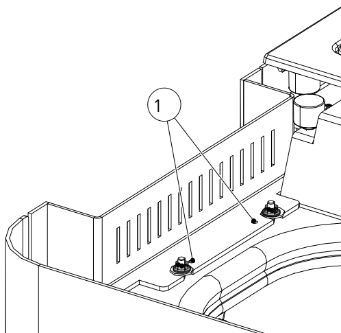
Fig. 104: Ajuster le support pour habillage en haut
