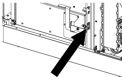
Fig. 101: Regolazione dello sportello del cassetto della cenere sul lato di chiusura
