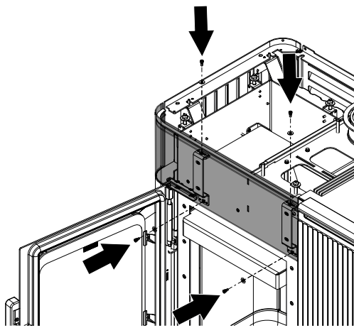
Fig. 12: Montaggio del pannello anteriore nuovo
