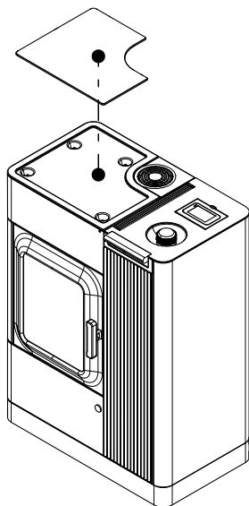
Fig. 111: Rimozione del coperchio dell'area di cottura
