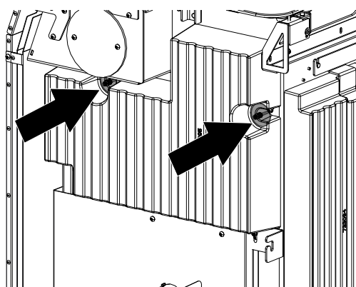
Fig. 45: Montaggio della pietra posteriore dell'HMS
