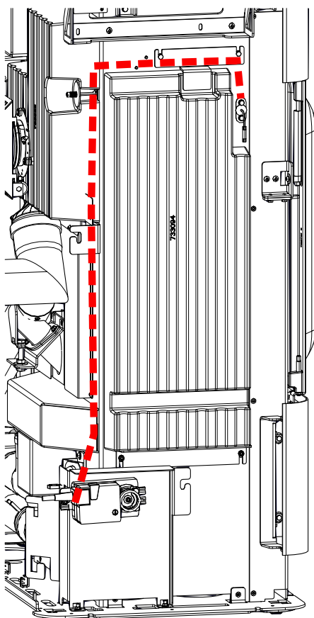
Fig. 48: Posare il cavo FTF
