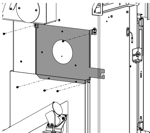
Fig. 43: Rimozione della lamiera
