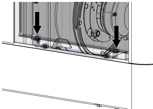
Fig. 24: Inserimento del supporto frontale nell'angolare
