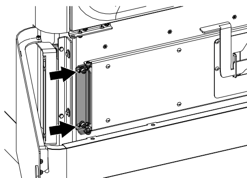
Fig. 100: Regolazione dello sportello del vassoio per la cenere
