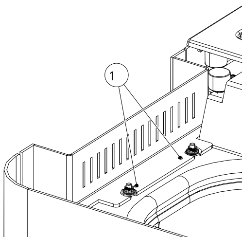
Fig. 103: Regolazione del supporto frontale in alto
