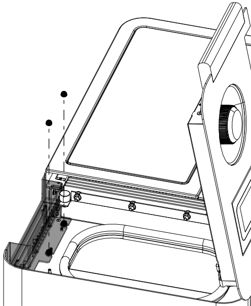
Fig. 122: Montaggio del frontale in acciaio
