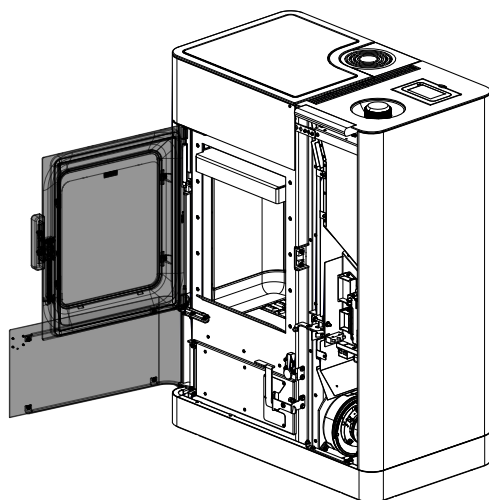
Fig. 99: Apertura degli sportelli
