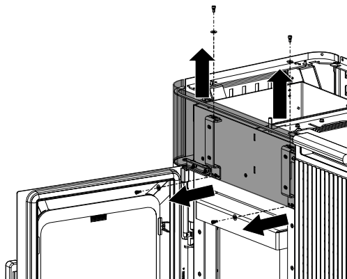
Fig. 10: Smontaggio del pannello anteriore
