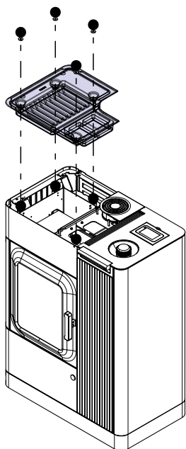
Fig. 112: Rimozione della piastra di cottura
