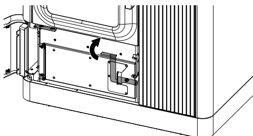
Fig. 107: Apertura dello sportello del cassetto della cenere
