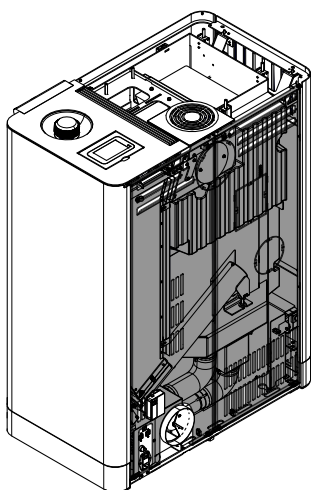
Fig. 18: Rimontaggio della parete posteriore
