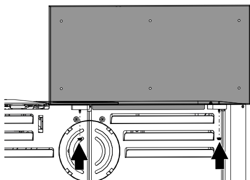
Fig. 19: Montaggio del supporto del pannello a parete
