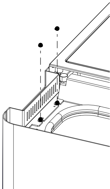
Fig. 25: Fissaggio del supporto frontale in alto
