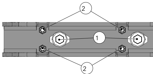
Fig. 92: Viti di regolazione
