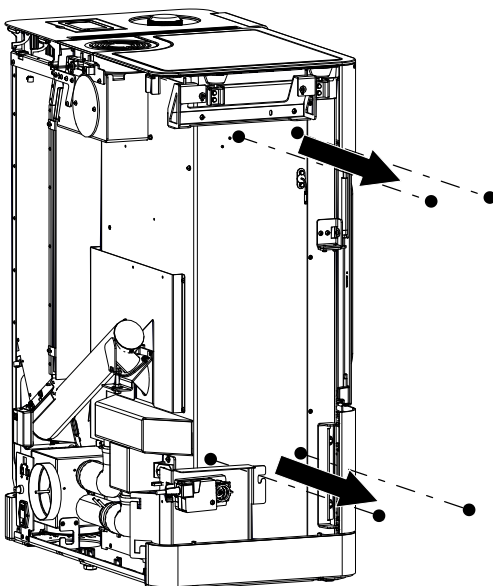
Fig. 42: Svitamento delle viti pre-esistenti
