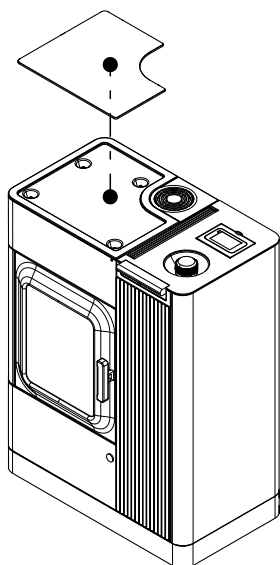
Fig. 8: Rimozione del coperchio dell'area di cottura
