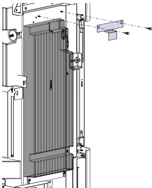
Fig. 47: Collocazione della pietra HMS
