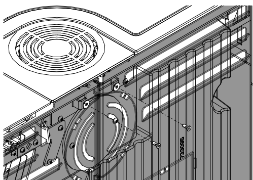
Fig. 127: Rimozione della parete posteriore
