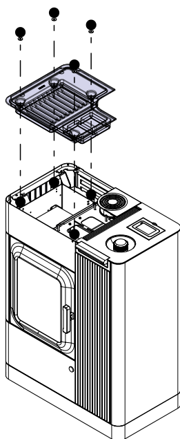
Fig. 9: Rimozione della piastra di cottura
