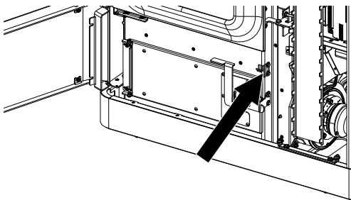
Fig. 98: Regolazione in basso dello sportello sul lato di chiusura
