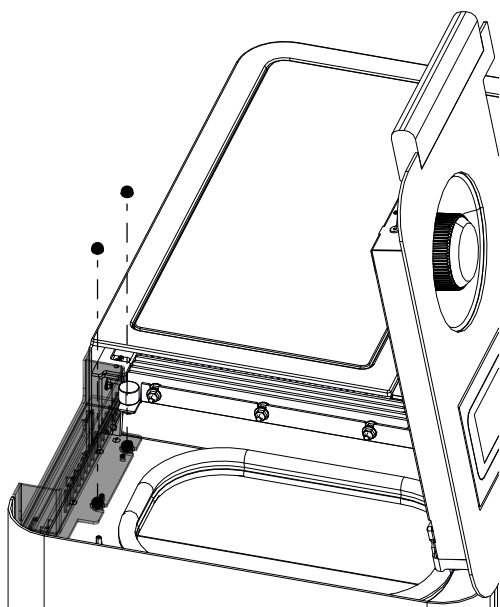
Fig. 27: Montaggio del frontale in acciaio
