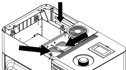
Fig. 113: Pulizia delle canne fumarie in alto
