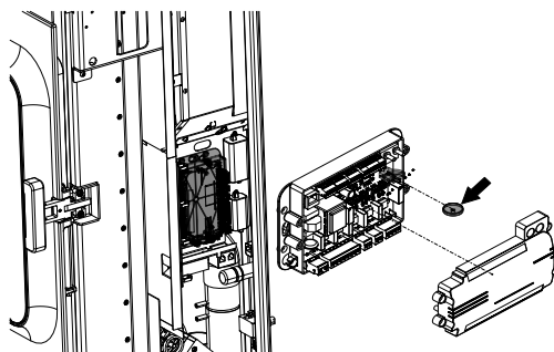
Fig. 105: Sostituzione della batteria tampone
