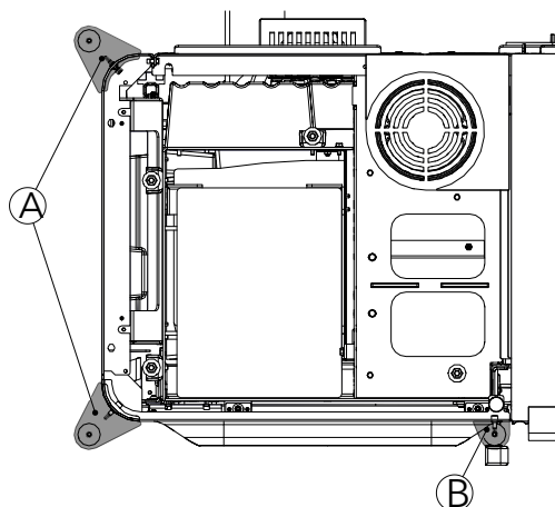
Fig. 13: Montaggio della bordatura di protezione
