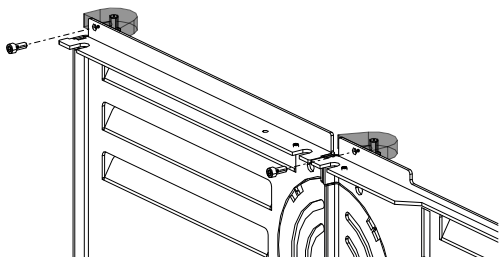
Fig. 17: Avvitamento dei supporti a parete sulla parete posteriore
