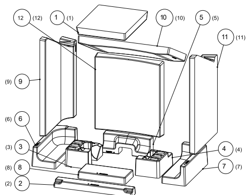
Fig. 21: Montaggio del Keramott
