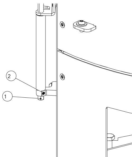
Fig. 95: Regolazione della forza di chiusura dello sportello
