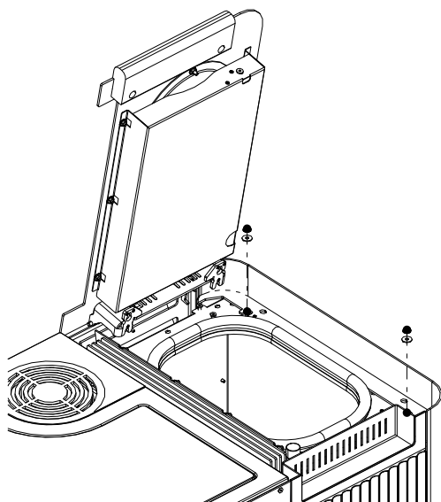
Fig. 125: Rimuovere il rivestimento laterale destro.
