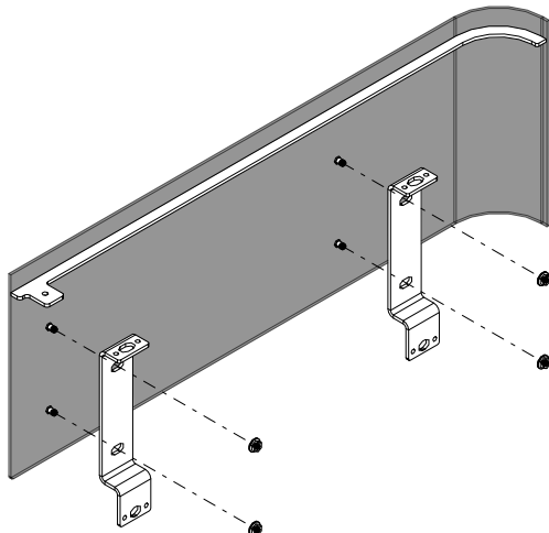
Fig. 11: Rimozione del pannello anteriore
