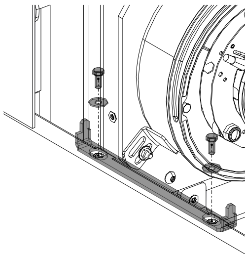
Fig. 23: Fissaggio dell'elemento angolare
