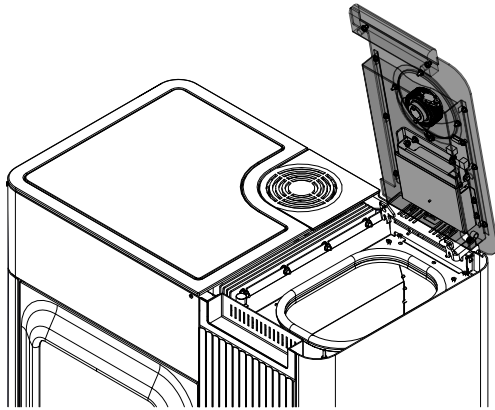
Fig. 121: Aprire il coperchio del contenitore dei pellet.
