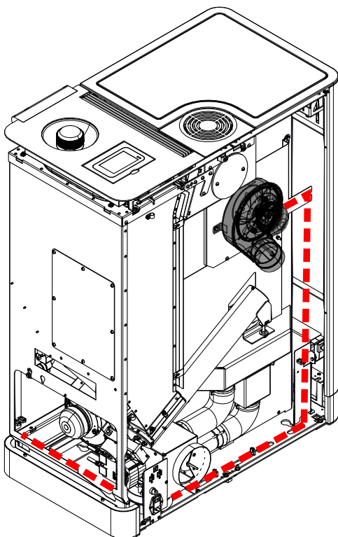
Fig. 34: Posa del cavo
