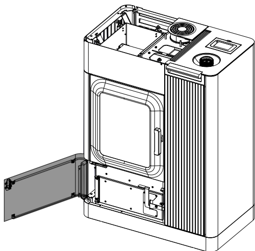
Fig. 114: Apertura dello sportello
