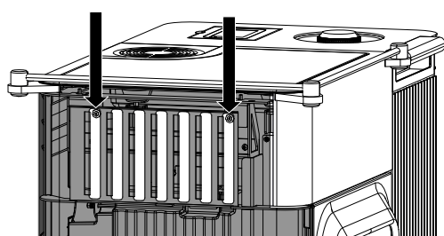
Fig. 124: Rimozione del rivestimento laterale sinistro
