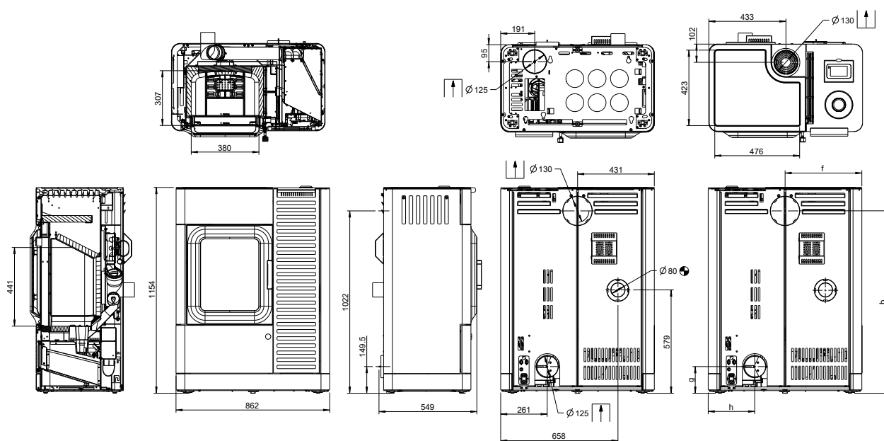
Fig. 1: Dimensioni di Mo Dou Cook
