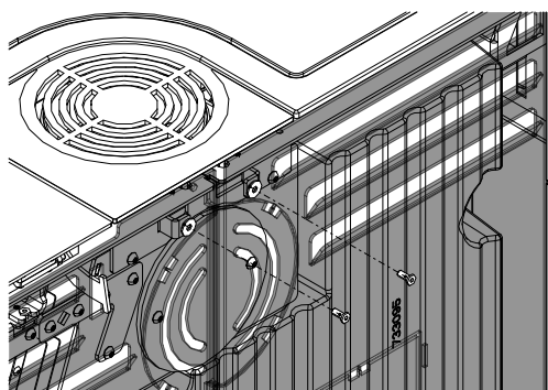
Fig. 103: Rimozione della parete posteriore
