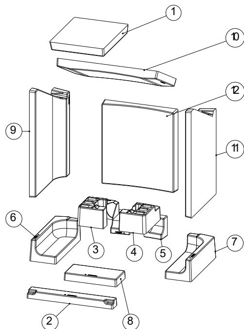
Fig. 9: Montaggio del Keramott
