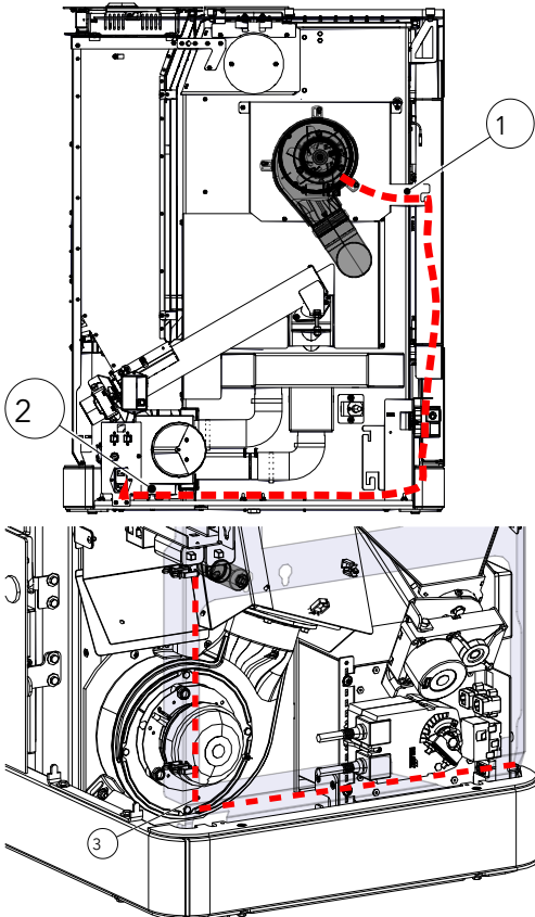
Fig. 18: Posa del cavo
