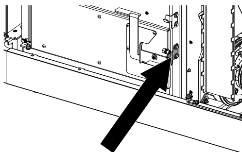
Fig. 77: Regolazione dello sportello del cassetto della cenere sul lato di chiusura
