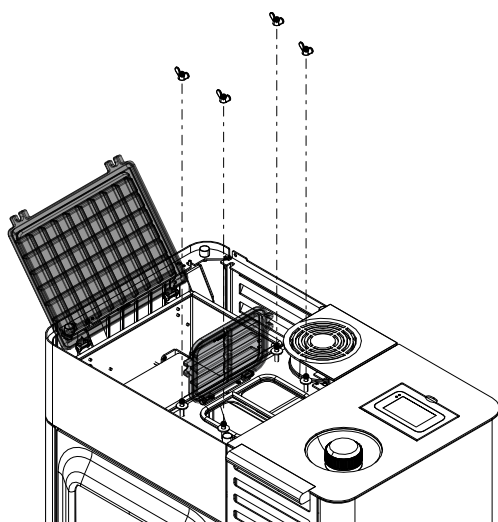
Fig. 88: Coperchio per la pulizia
