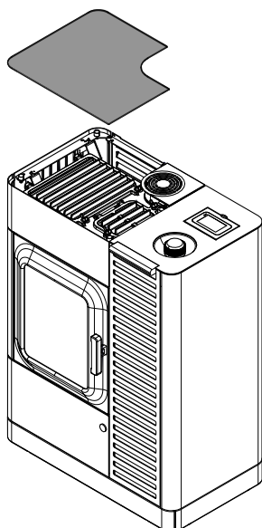
Fig. 87: Rimozione della piastra riscaldante
