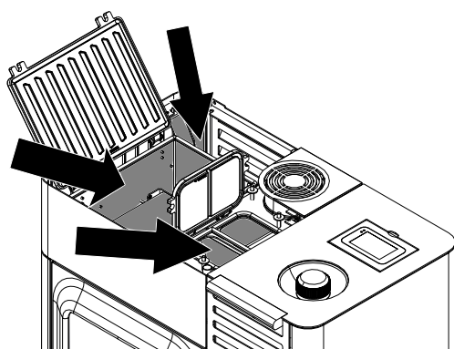
Fig. 89: Pulizia delle canne fumarie in alto
