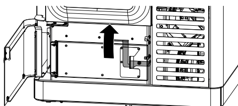
Fig. 91: Apertura dello sportello del cassetto della cenere
