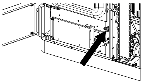
Fig. 80: Regolazione in basso dello sportello sul lato di chiusura
