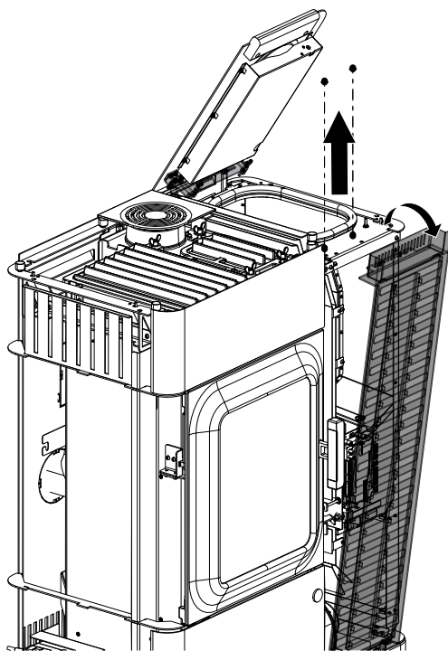
Fig. 100: Smontaggio del rivestimento laterale anteriore
