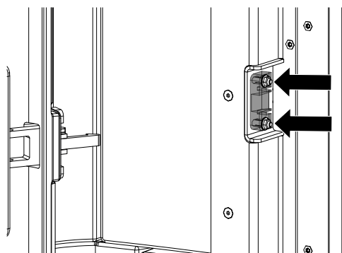
Fig. 72: Regolazione dal lato di chiusura
