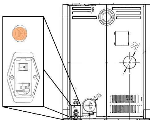
Fig. 96: Limitatore di temperatura di sicurezza
