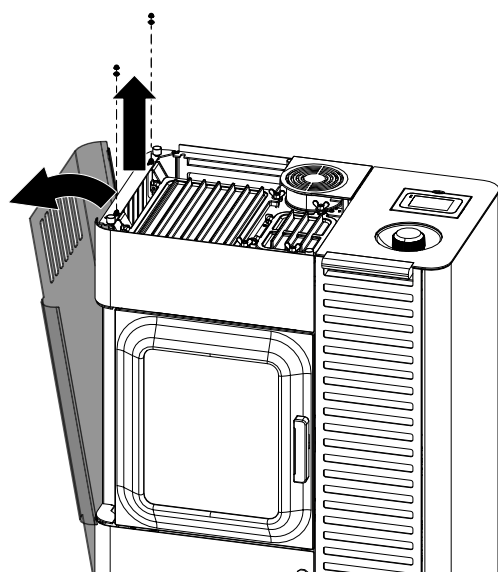
Fig. 98: Smontaggio del rivestimento laterale sinistro
