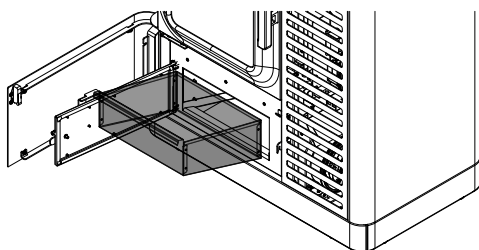
Fig. 92: Rimozione del cassetto della cenere
