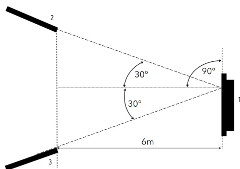
Fig. 41: Angolo di lavoro
