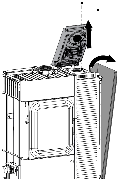
Fig. 99: Smontaggio del rivestimento laterale destro
