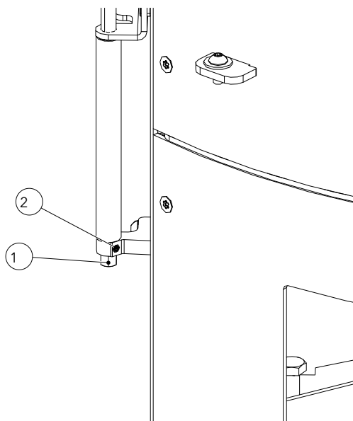
Fig. 74: Regolazione della forza di chiusura dello sportello
