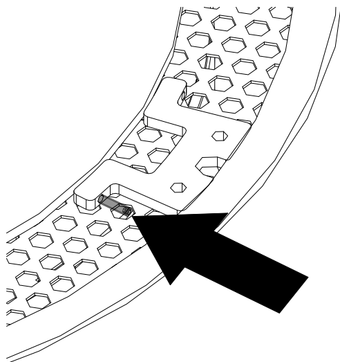
Fig. 19: Fixer l'anneau de centrage
