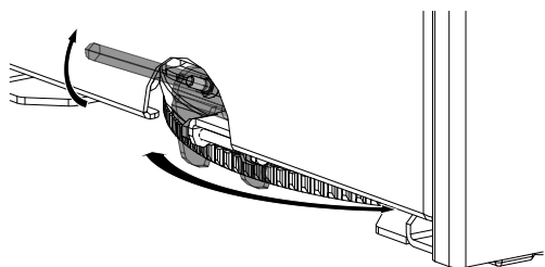
Fig. 46: Régler le plateau tournant
