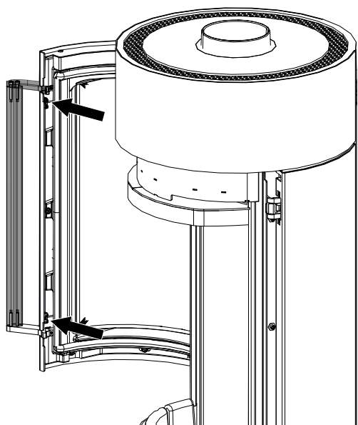
Fig. 45: Régler la force de fermeture de la poignée
