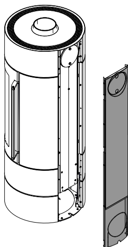
Fig. 27: Enlever la plaque arrière
