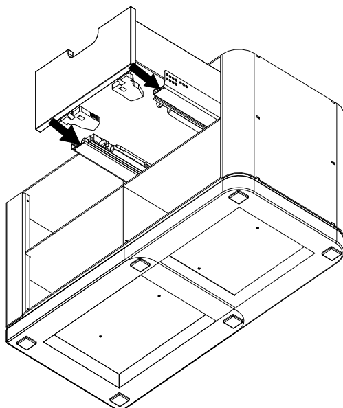
Fig. 25: Introduire le tiroir à bois dans les glissières
