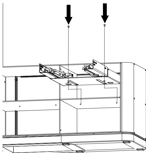
Fig. 24: Installer le support à glissières
