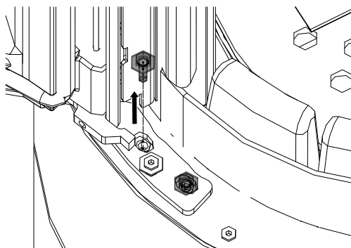
Fig. 56: Vis en bas
