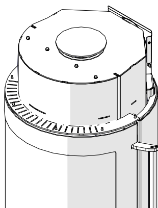
Fig. 40: Démonter la tubulure de fumées
