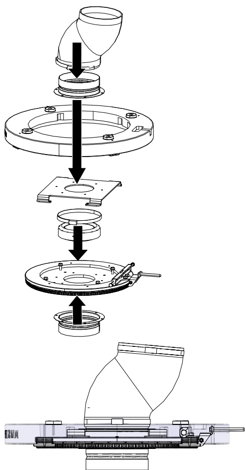
Fig. 35: Assembler le socle et le plateau tournant
