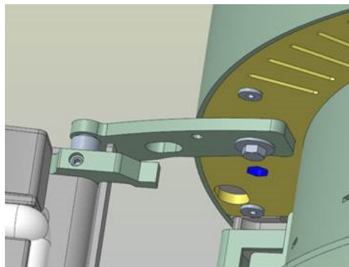
Fig. 57: Faire pivoter la porte vers l'extérieur
