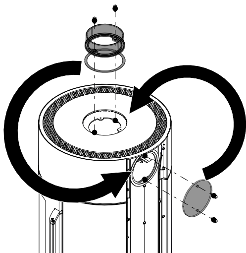
Fig. 11: Échanger le recouvrement et la tubulure
