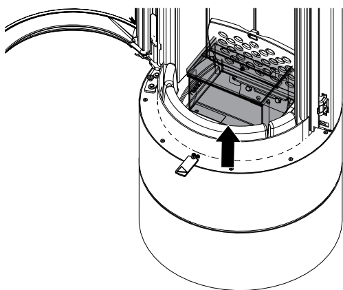
Fig. 53: Enlever et vider le bac à cendres
