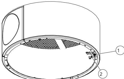
Fig. 16: Mettre en place l'anneau de centrage
