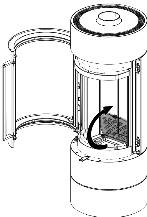
Fig. 50: Relever la grille
