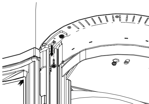
Fig. 55: Vis en haut
