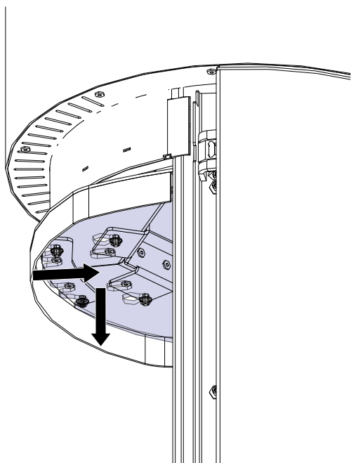
Fig. 59: Enlever la plaque
