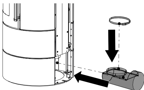
Fig. 28: Enlever la découpe perforée
