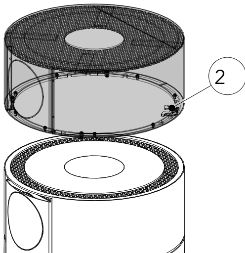
Fig. 17: Poser le module supérieur
