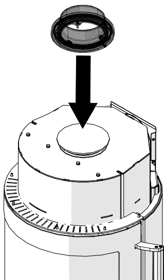
Fig. 41: Installer la tubulure de fumées orientable
