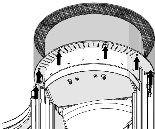
Fig. 31: Enlever le couvercle
