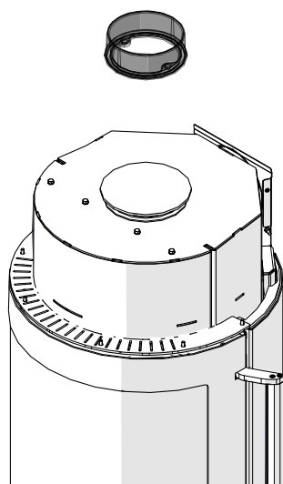
Fig. 33: Démonter la tubulure de fumées
