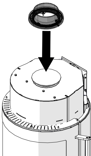
Fig. 42: Installer la tubulure de fumées orientable
