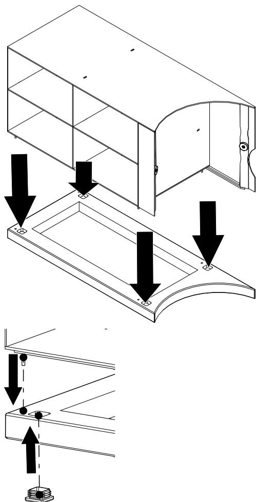
Fig. 22: Assembler le module latéral
