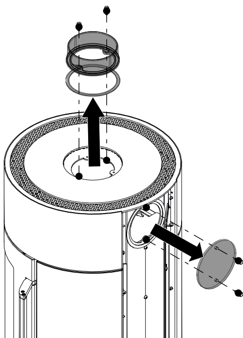
Fig. 11: Démonter le recouvrement et la tubulure de fumées
