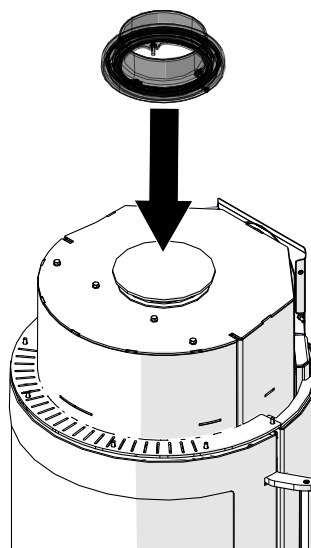
Fig. 35: Installer la tubulure de fumées orientable
