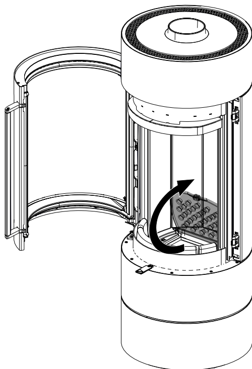
Fig. 47: Relever la grille
