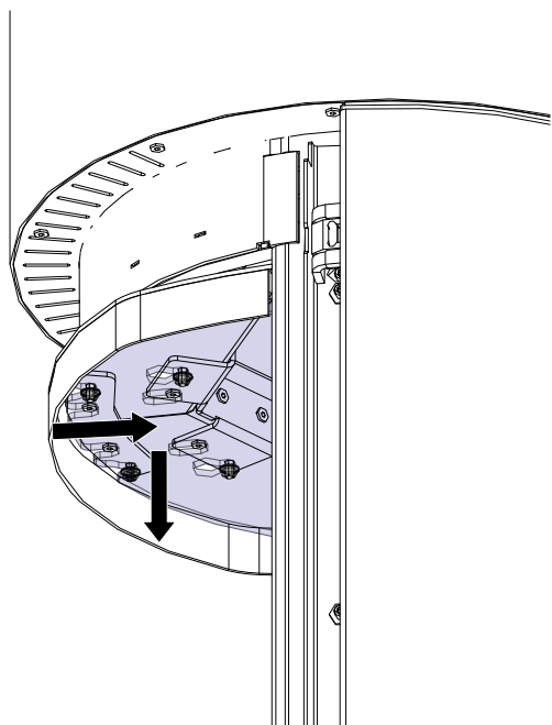
Fig. 56: Enlever la plaque
