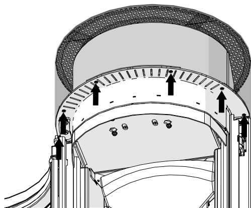
Fig. 28: Enlever le couvercle
