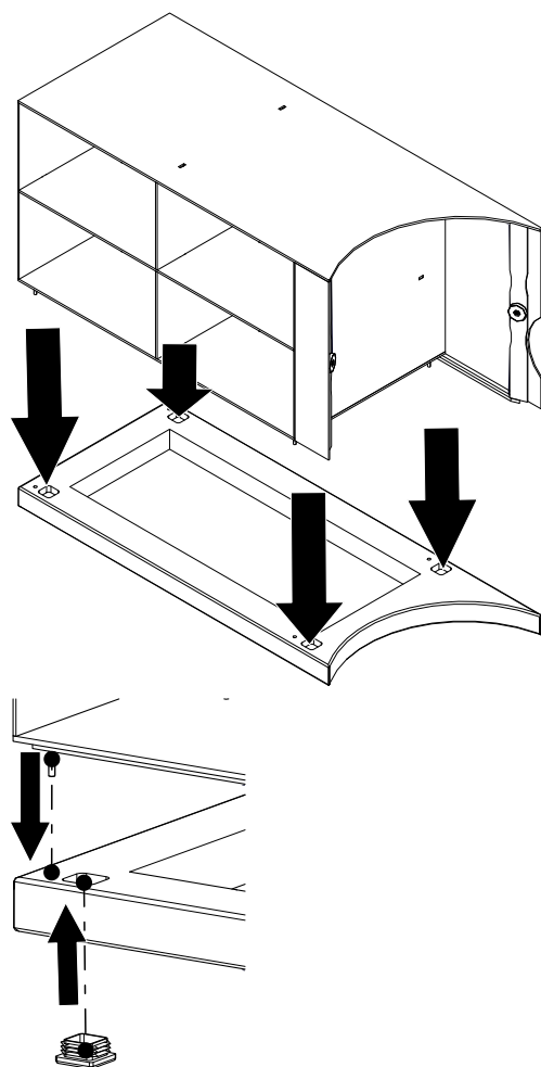
Fig. 18: Assembler le module latéral
