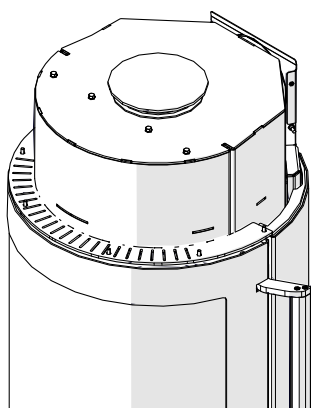
Fig. 37: Démonter la tubulure de fumées
