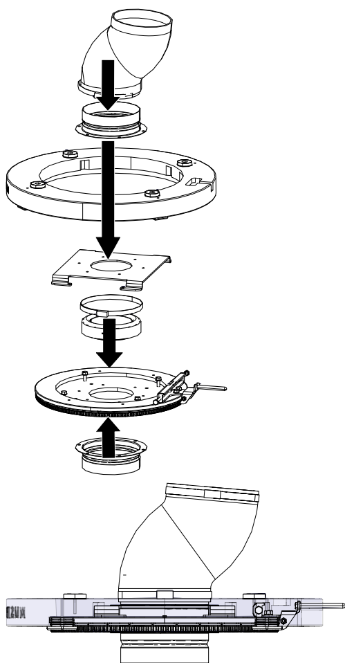
Fig. 32: Assembler le socle et le plateau tournant
