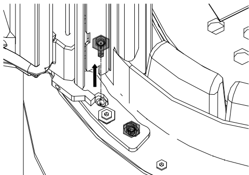
Fig. 53: Vis en bas
