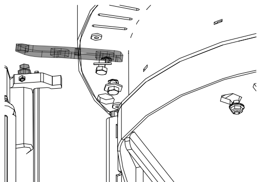
Fig. 55: Extraire la porte des charnières
