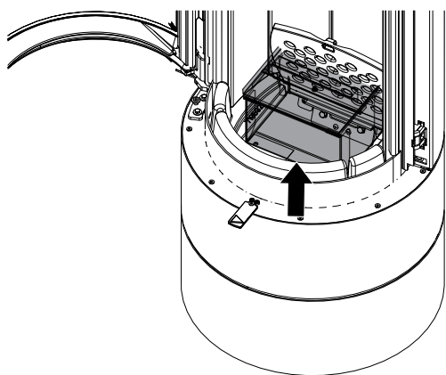
Fig. 50: Enlever et vider le bac à cendres
