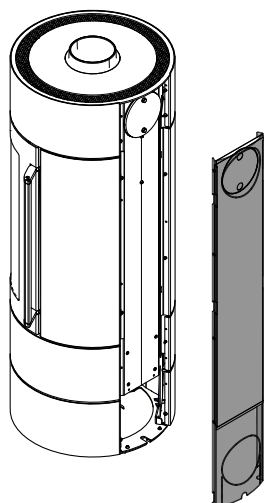
Fig. 24: Enlever la plaque arrière
