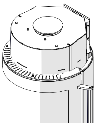
Fig. 30: Démonter la tubulure de fumées
