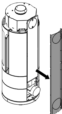
Fig. 29: Enlever la paroi arrière
