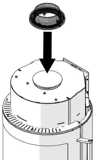
Fig. 31: Installer la tubulure de fumées orientable
