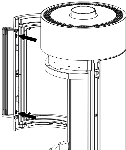
Fig. 42: Régler la force de fermeture de la poignée
