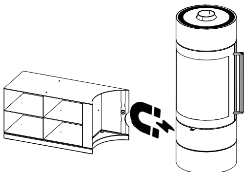
Fig. 19: Poser le module latéral contre le poêle à bois
