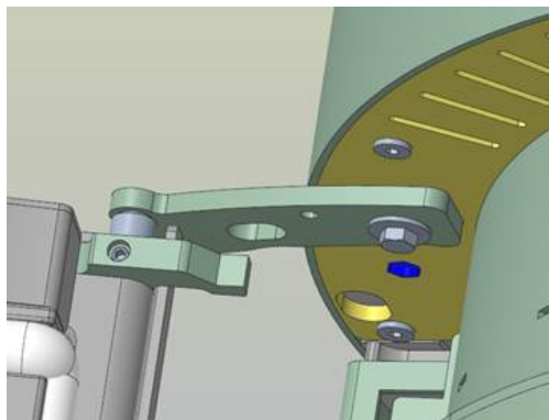
Fig. 54: Faire pivoter la porte vers l'extérieur
