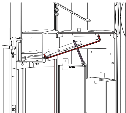
Fig. 59: Extraire la plaque par le bas
