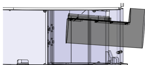
Fig. 26: Installer l'adaptateur d'arrivée d'air
