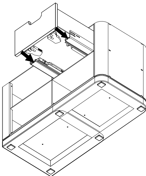
Fig. 22: Introduire le tiroir à bois dans les glissières
