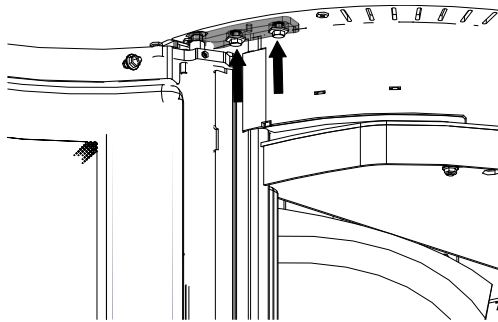
Fig. 41: Régler les charnières de porte
