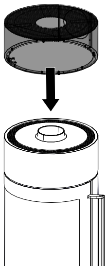
Fig. 19: Fissaggio dell'anello di centraggio
