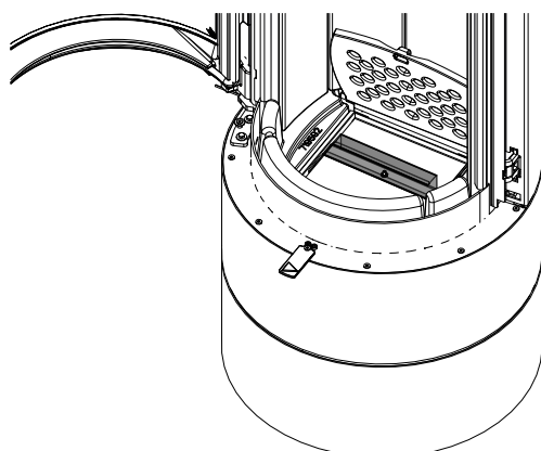
Fig. 52: Chiusura del coperchio
