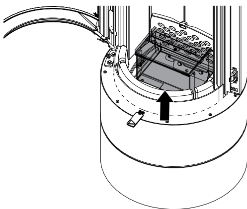
Fig. 53: Rimozione e svuotamento del box cenere
