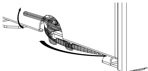
Fig. 46: Regolazione del piatto girevole
