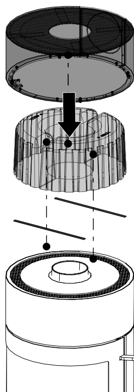
Fig. 15: Montaggio delle pietre HMS
