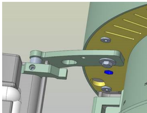
Fig. 57: Rotazione dello sportello verso l'esterno
