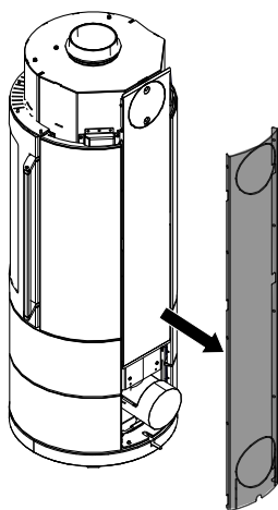
Fig. 39: Rimozione della parete posteriore
