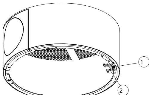
Fig. 16: Applicazione dell'anello di centraggio
