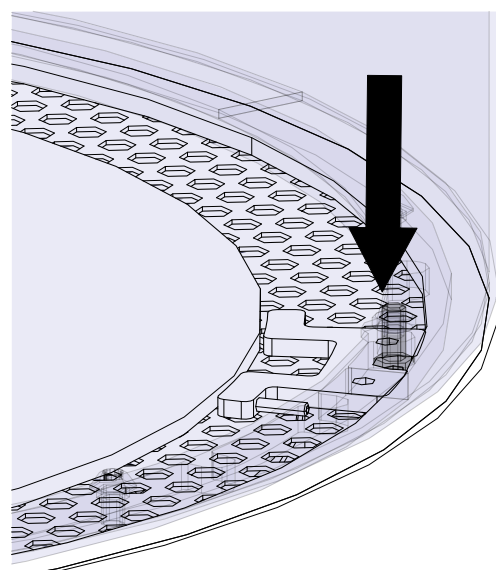
Fig. 20: Montaggio del box portautensili
