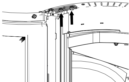
Fig. 44: Regolazione delle cerniere dello sportello
