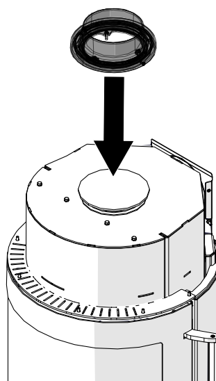
Fig. 34: Montaggio della presa della canna fumaria rotante
