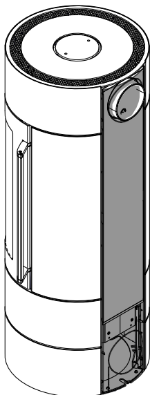
Fig. 13: Montaggio della parte posteriore
