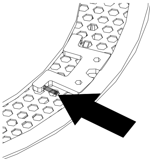
Fig. 19: Fissaggio dell'anello di centraggio
