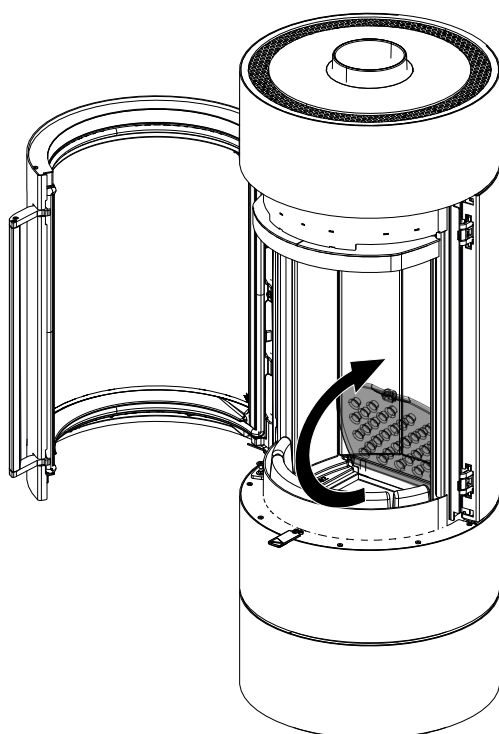
Fig. 50: Sollevamento della griglia
