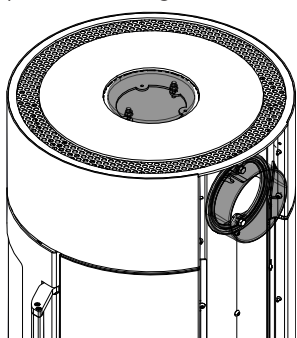
Fig. 12: Copertura e pezzo di collegamento sostituiti
