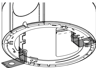
Fig. 6: Sicurezze per il trasporto
