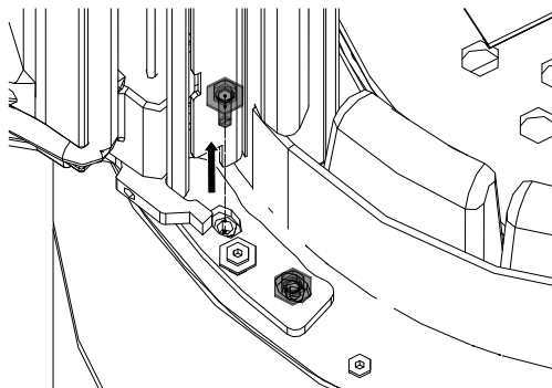
Fig. 56: Viti inferiori
