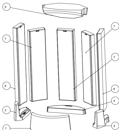
Fig. 14: Installazione del Keramott
