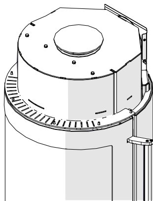
Fig. 40: Smontaggio della presa della canna fumaria
