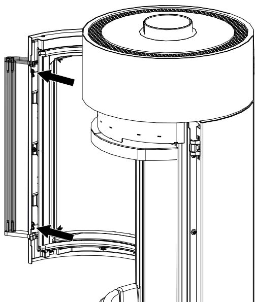
Fig. 45: Regolazione della forza di chiusura della maniglia
