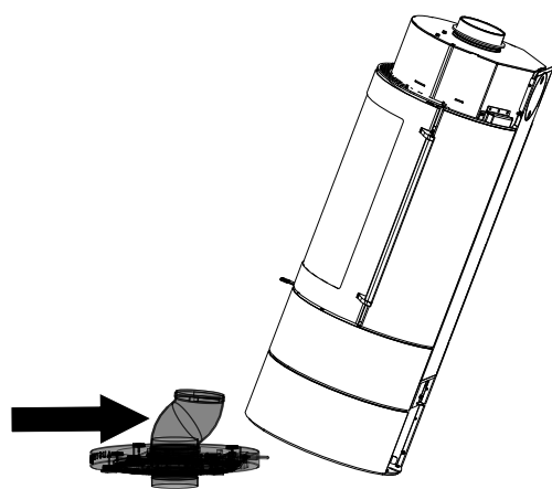
Fig. 36: Inclinamento della stufa
