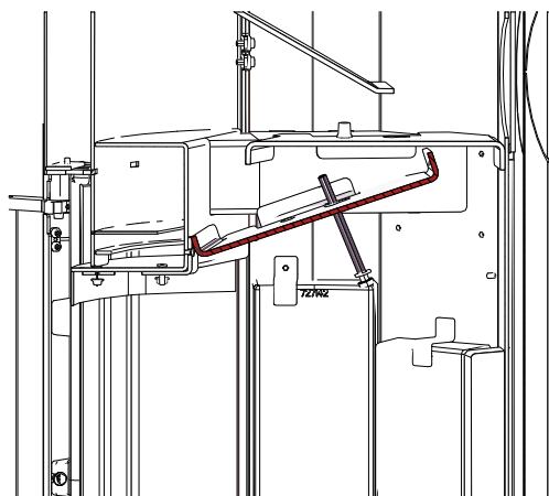
Fig. 62: Rimozione della piastra verso il basso
