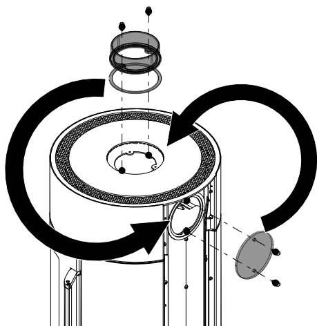
Fig. 11: Sostituzione del coperchio e del pezzo di collegamento
