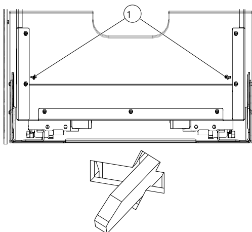
Fig. 26: Perni di fissaggio
