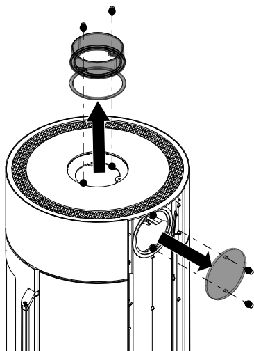
Fig. 10: Smontaggio del coperchio e della presa della canna fumaria
