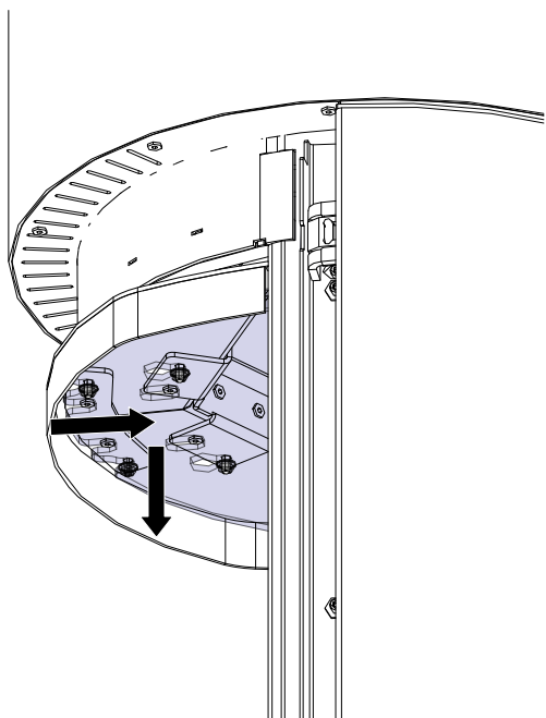
Fig. 59: Rimozione della piastra
