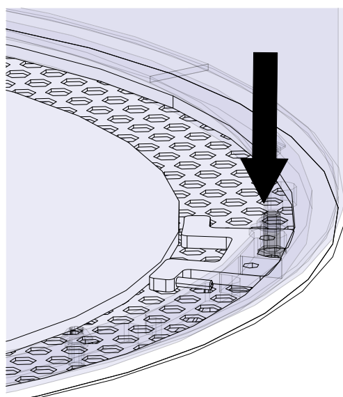
Fig. 21: Montaggio del box portautensili
