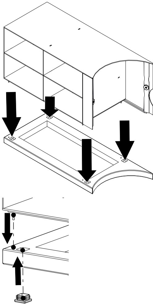
Fig. 22: Montaggio del box laterale
