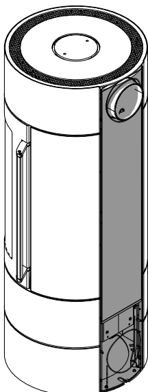
Abb. 14: Rückseite montieren
