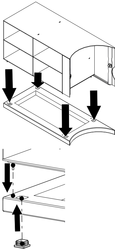
Abb. 22: Beistellbox zusammenbauen
