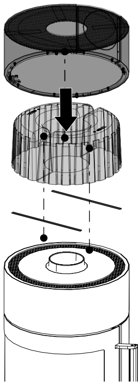
Abb. 16: HSM-Steine montieren
