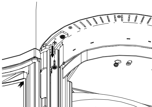
Abb. 56: Schrauben oben
