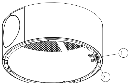
Abb. 17: Zentrierring anbringen
