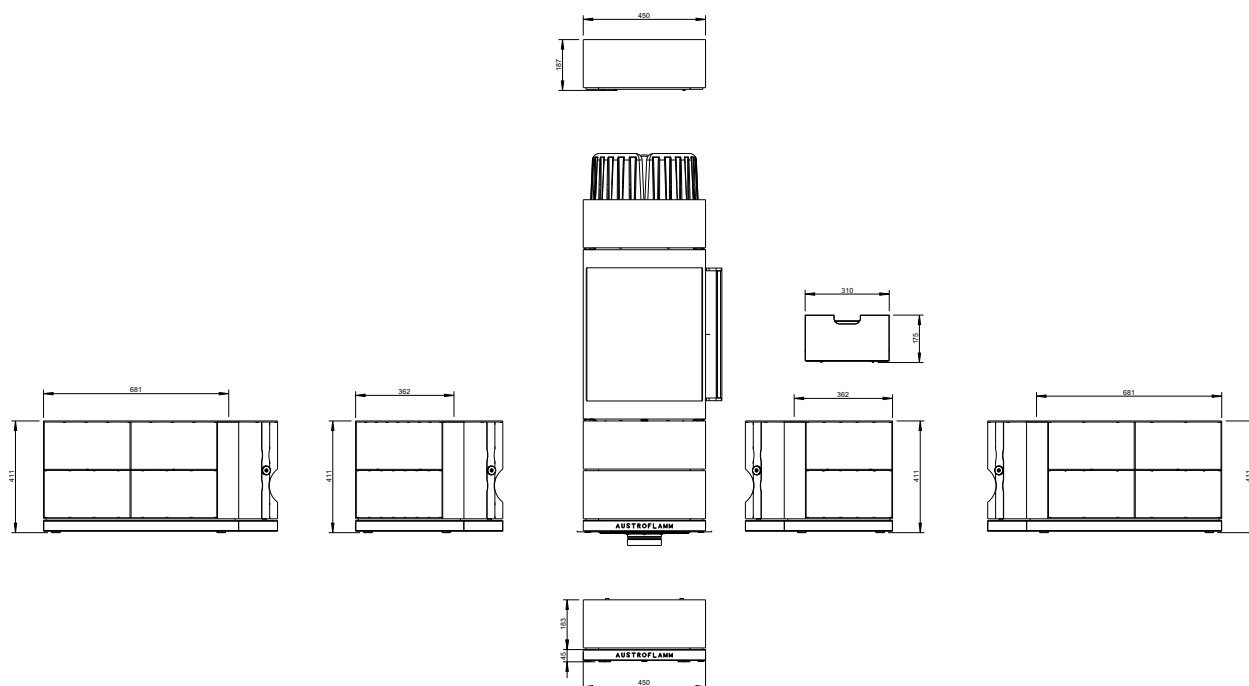
Abb. 3: Abmessungen Beistellboxen
