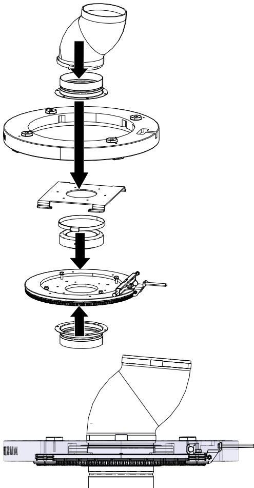
Abb. 36: Sockel mit Drehteller zusammensetzen
