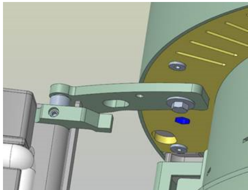
Abb. 58: Tür nach außen schwenken
