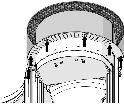
Abb. 32: Deckel abnehmen
