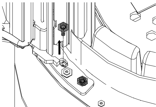
Abb. 57: Schrauben unten
