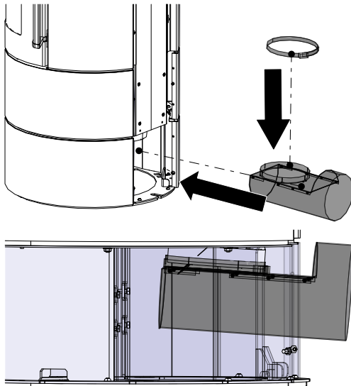
Abb. 30: Zuluftadapter montieren
