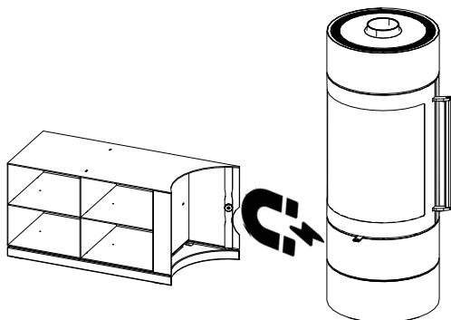
Abb. 23: Beistellbox an den Kaminofen stellen
