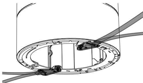
Abb. 8: Transporthilfe
