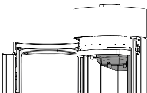
Abb. 61: Keramott-Stein entfernen
