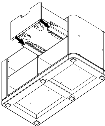
Abb. 26: Holzlade in die Schiene einführen
