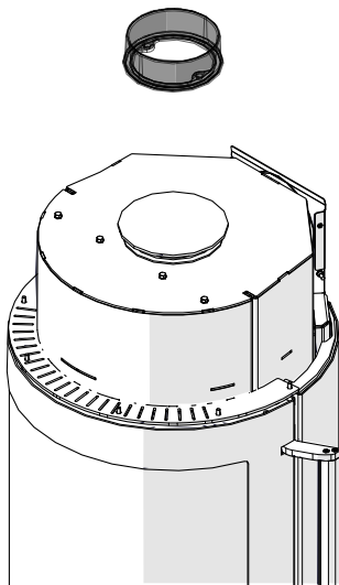
Abb. 34: Rauchrohrstutzen abmontieren
