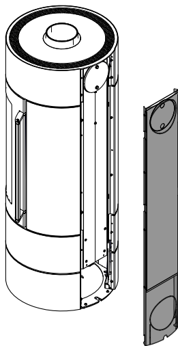
Abb. 28: Rückseite entfernen
