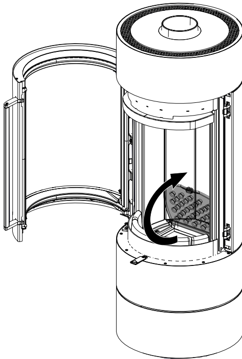
Abb. 51: Rost hochklappen
