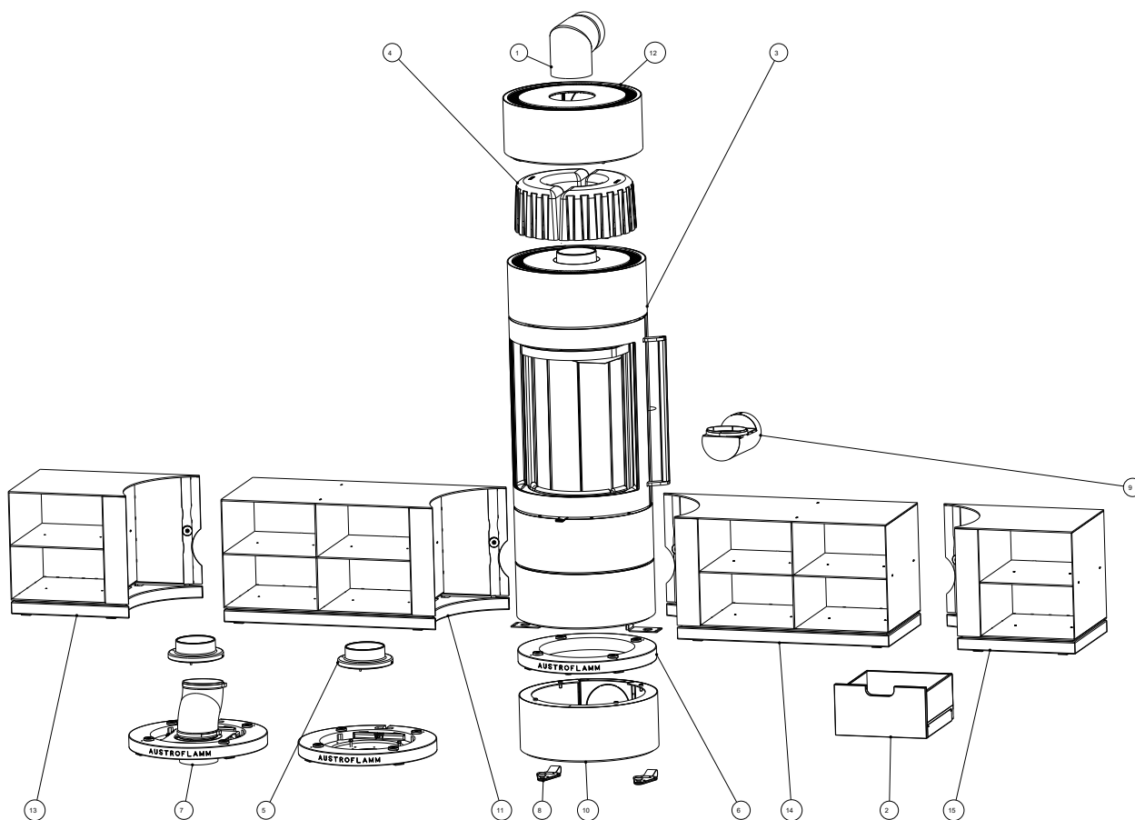
Abb. 55:
