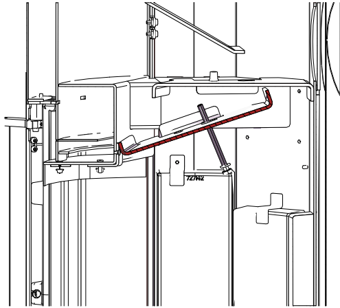
Abb. 63: Platte nach unten herausnehmen
