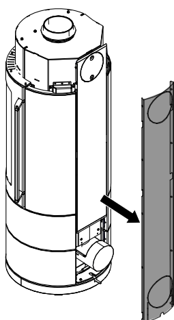
Abb. 40: Rückwand entfernen
