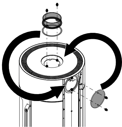
Abb. 12: Abdeckung und Stützen tauschen
