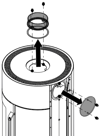
Abb. 11: Abdeckung und Rauchrohrstutzen demontieren
