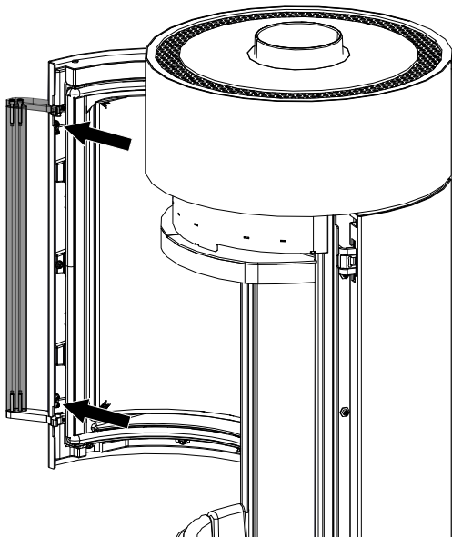
Abb. 46: Türgriffschließkraft einstellen
