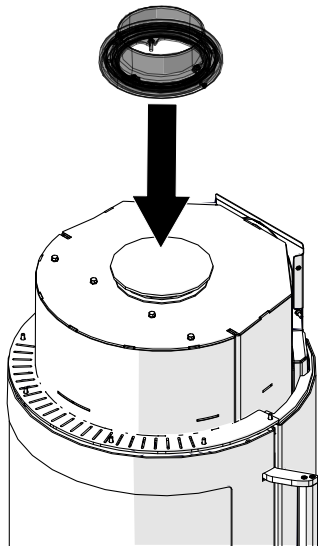
Abb. 35: Drehrauchrohrstutzen montieren
